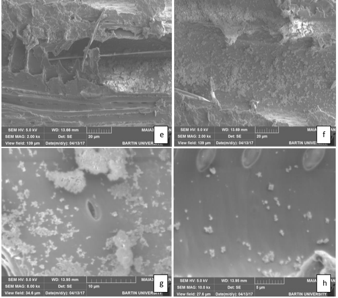
Şekil 3.14: Emprenyelenmiş Ahşap Malzemeye farklı açılardan SEM Görüntüleri (e-200 kx, f-200 kx, g-800 kx, h-100 kx).
