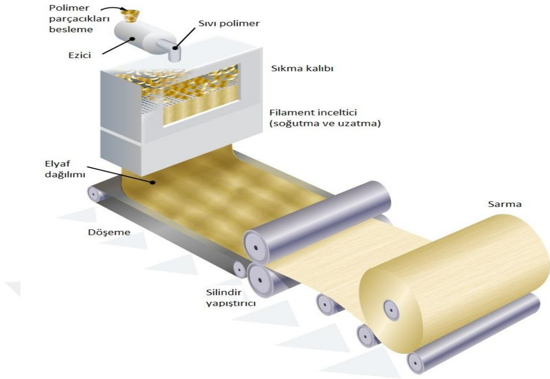
Şekil 2.4. Eriyik çekim yöntemi üretim aşamaları
