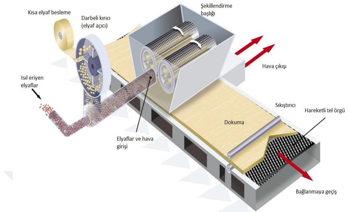
Şekil 2.2. Havalı serme yöntemi üretim aşamaları
