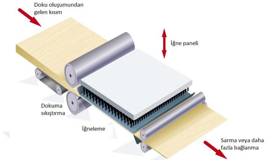
Şekil 2.7. İğneleme yönteminin üretim hattında uygulanması
