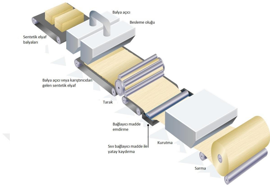
Şekil 2.1. Taraklama yöntemi üretim aşamaları
