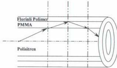
Şekil 3.9. Çok kaplamalı bir SciFi'nin şematik görünümü
