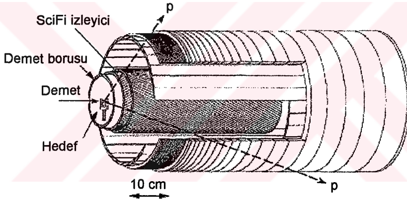
Şekil 4.5. COSY'deki EDDA dedektörünün Şematik Yapısı (Hinterberger, 1999)
