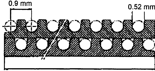
Şekil 4.11. H1 dedektöründe kullanılan kurşun-fiber yapıdaki elektromanyetik kalorimetrenin iki tabakasına ait kesit (Weber, 1997)
