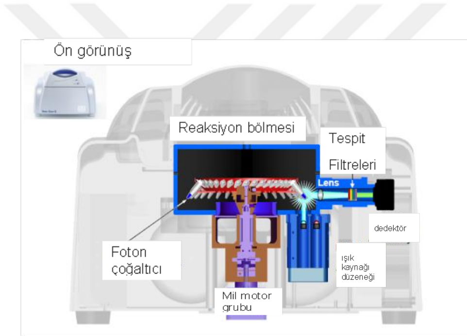
Şekil 2.5. Rotor Gene Q cihazının optik sisteminin illüstrasyonu. Işık kaynağı ve Dedektör filtreleri (Anonymous 3)
