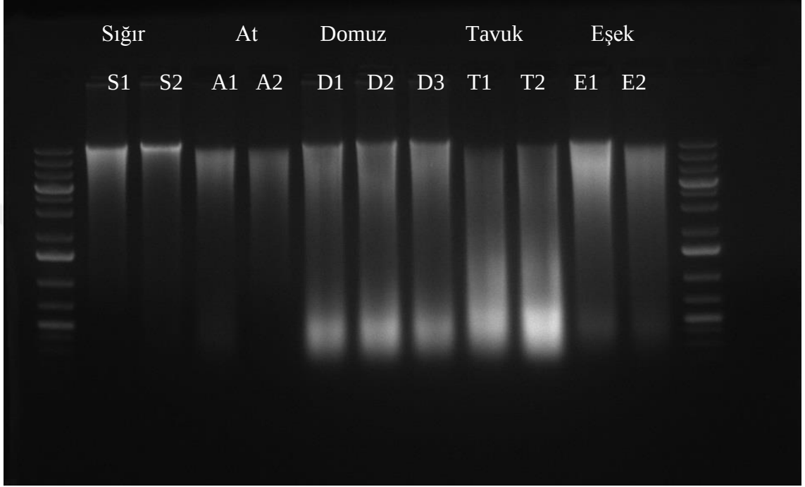
Şekil 4.1. Et türlerinden izole edilen genomik DNA'ların %1 agaroz jel görüntüsü. (S1: sığır DNA'sı, 240 ng/µl; S2: sığır DNA'sı, 107 ng/µl; A1: at DNA'sı, 220 ng/µl; A2: at DNA'sı, 100 ng/µl; D1: domuz DNA'sı, 1250 ng/µl; D2: domuz DNA'sı, 1130 ng/µl; D3: domuz DNA'sı, 500 ng/µl; T1: tavuk DNA'sı, 1150 ng/µl; T2: tavuk DNA'sı, 1275 ng/µl; E1: eşek DNA'sı, 635 ng/µl; E2: eşek DNA'sı, 385 ng/µl)
