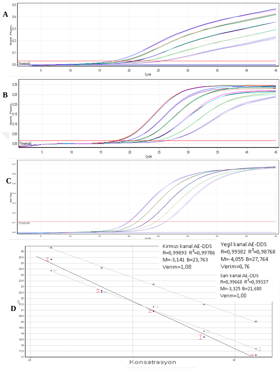
Şekil 4.13. Primer ve prob setlerinin AE-DDS (at ve eşek DNA'larının her birinden %16, %5, %1,6, %0,5, %0,16 ve %0,05 içeren) ile üçlü reaksiyon verimliliği analizi sonucu (A) Eşek primerleri amplifikasyon grafiği (Yeşil Kanal) (B) At primerleri amplifikasyon grafiği (Sarı Kanal) (C) 18S primerleri amplifikasyon grafiği (Kırmızı Kanal) (D) Standart eğri
