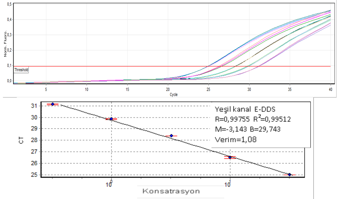
Şekil 4.7. Eşek primer ve prob setinin E-DDS ile 45°C bağlanma sıcaklığında gerçekleştirilen tekli GZ-PZR reaksiyon verimliliği analizi sonucu. (A) E-DDS ile eşek primerlerinin amplifikasyon grafiği, Yeşil Kanal; (B) Standart eğri (E: reaksiyon verimliliği, M: eğim, R^2 : korelasyon katsayısı)
