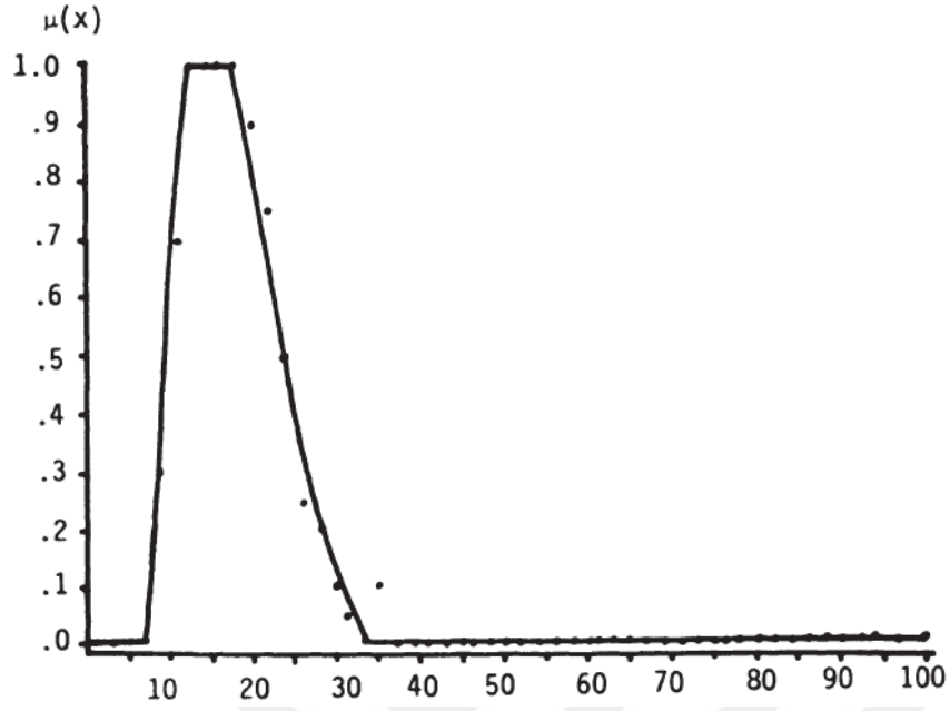
Şekil 3d: Genç İnsanlar (Gİ) kümesi üyelik fonksiyonu
