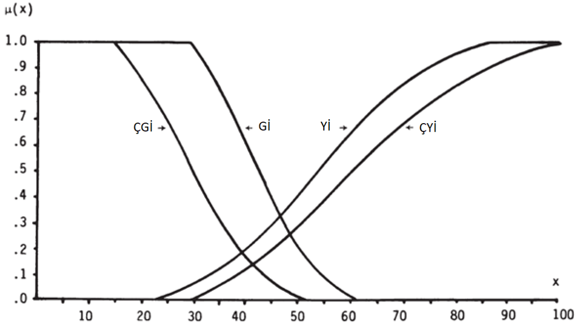
Şekil 3e: Genel üyelik fonksiyonları, Çok Genç İnsanlar (ÇGİ), Genç İnsanlar (Gİ), Yaşlı İnsanlar (Yİ), Çok Yaşlı İnsanlar (ÇYİ)
