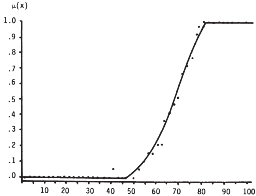
Şekil 3b: Çok Yaşlı İnsanlar (ÇYİ) kümesi üyelik fonksiyonu
