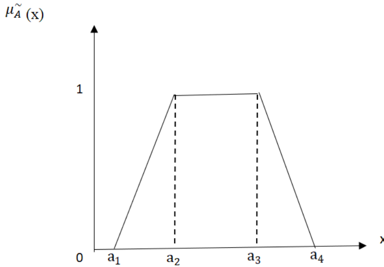
Şekil 4b: Yamuk üyelik fonksiyonu
