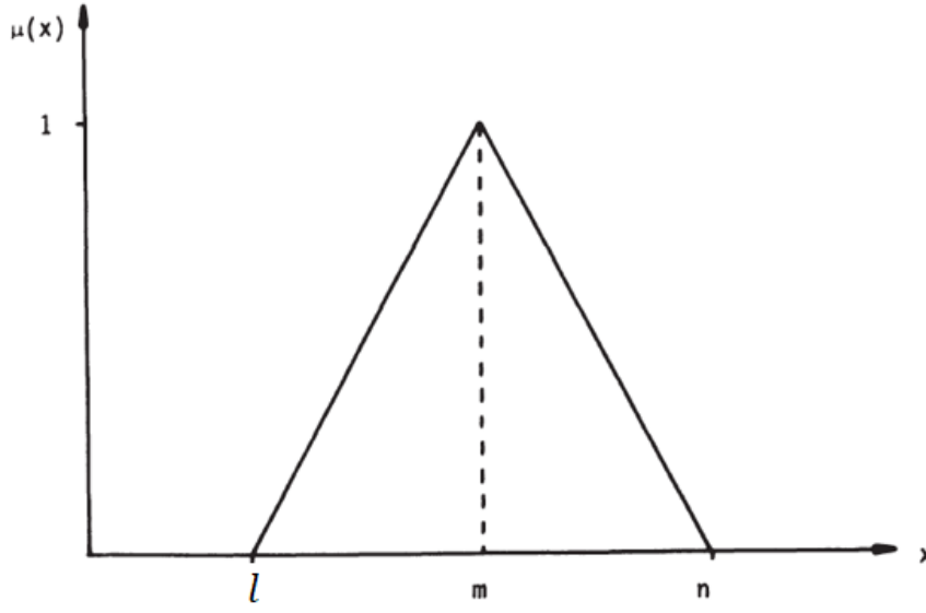
Şekil 4a. Bulanık Üçgensel Üyelik Fonksiyonu
