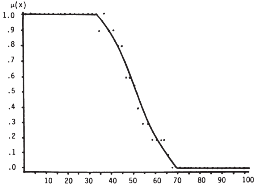
Şekil 3d: Genç İnsanlar (Gİ) kümesi üyelik fonksiyonu
