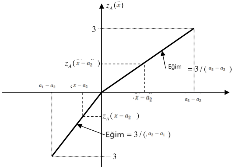
Şekil 4c: Logaritmik mümkünlik değeri
