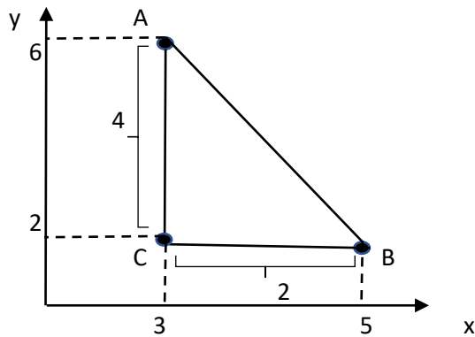
Şekil 4d. Noktalar arası uzaklıklar
