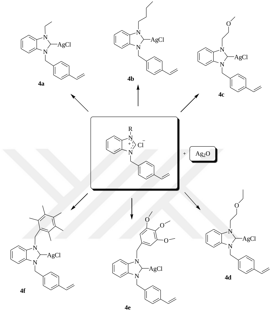
Şema 3.5. 4-vinilbezil süstitüentli Ag-(NHC) komplekslerinin sentezi.
