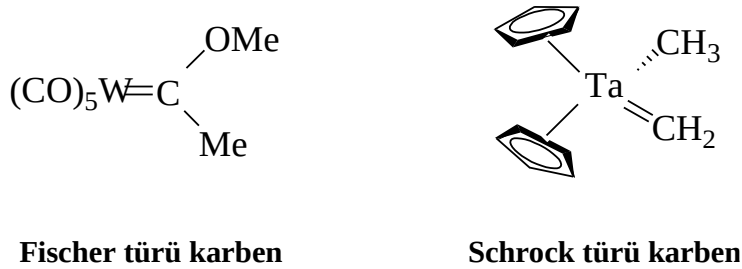
Şekil 1.6. Fischer ve schrock karben kompleksleri.
