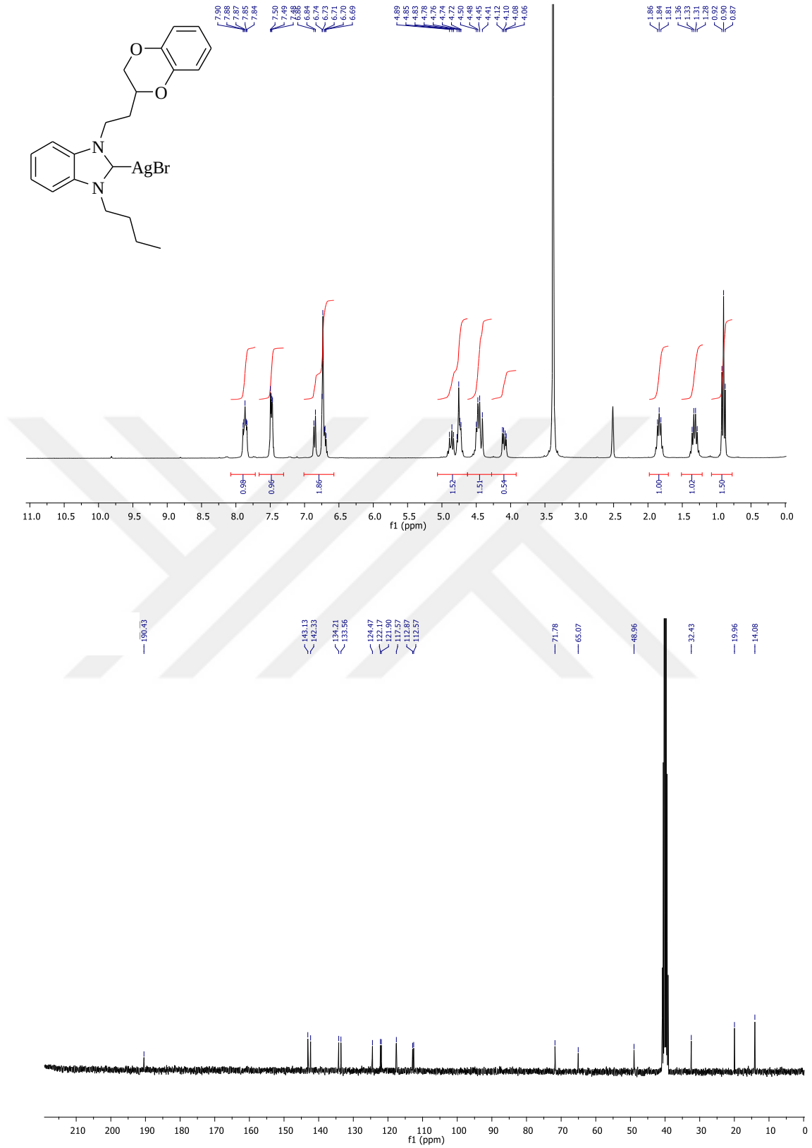
Şekil 3.4. [1-(2-metil-1,4-benzodioxan)-3-butylbenzimidazol-2-iliden] bromür gümüş (I) bileşiğine ait 1 H NMR ve 13 C NMR spektrumları.
