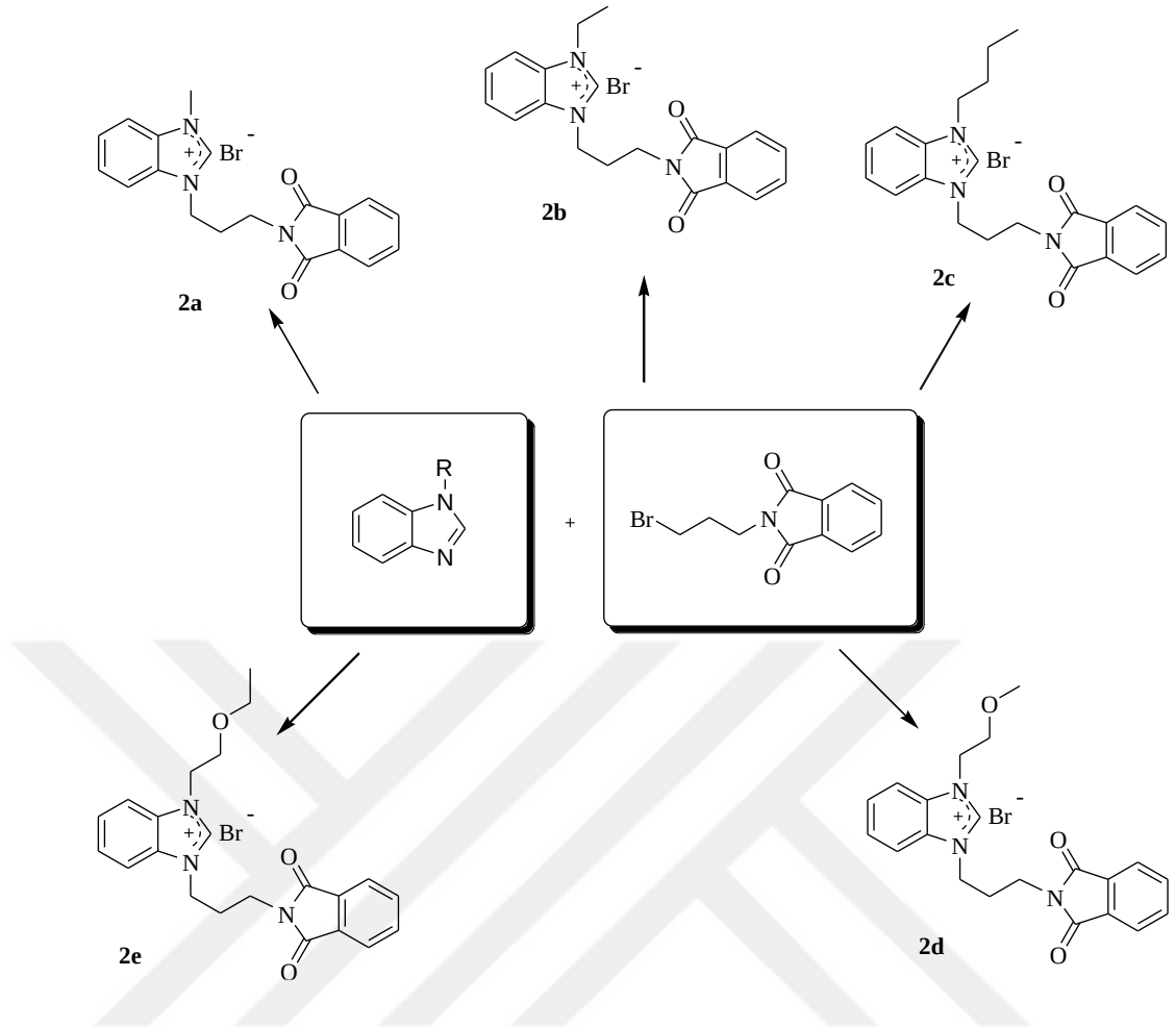
Şema 3.3. N-propilftalimit süstitüentli benzimidazolyum tuzlarının (2a-e) sentezi.
