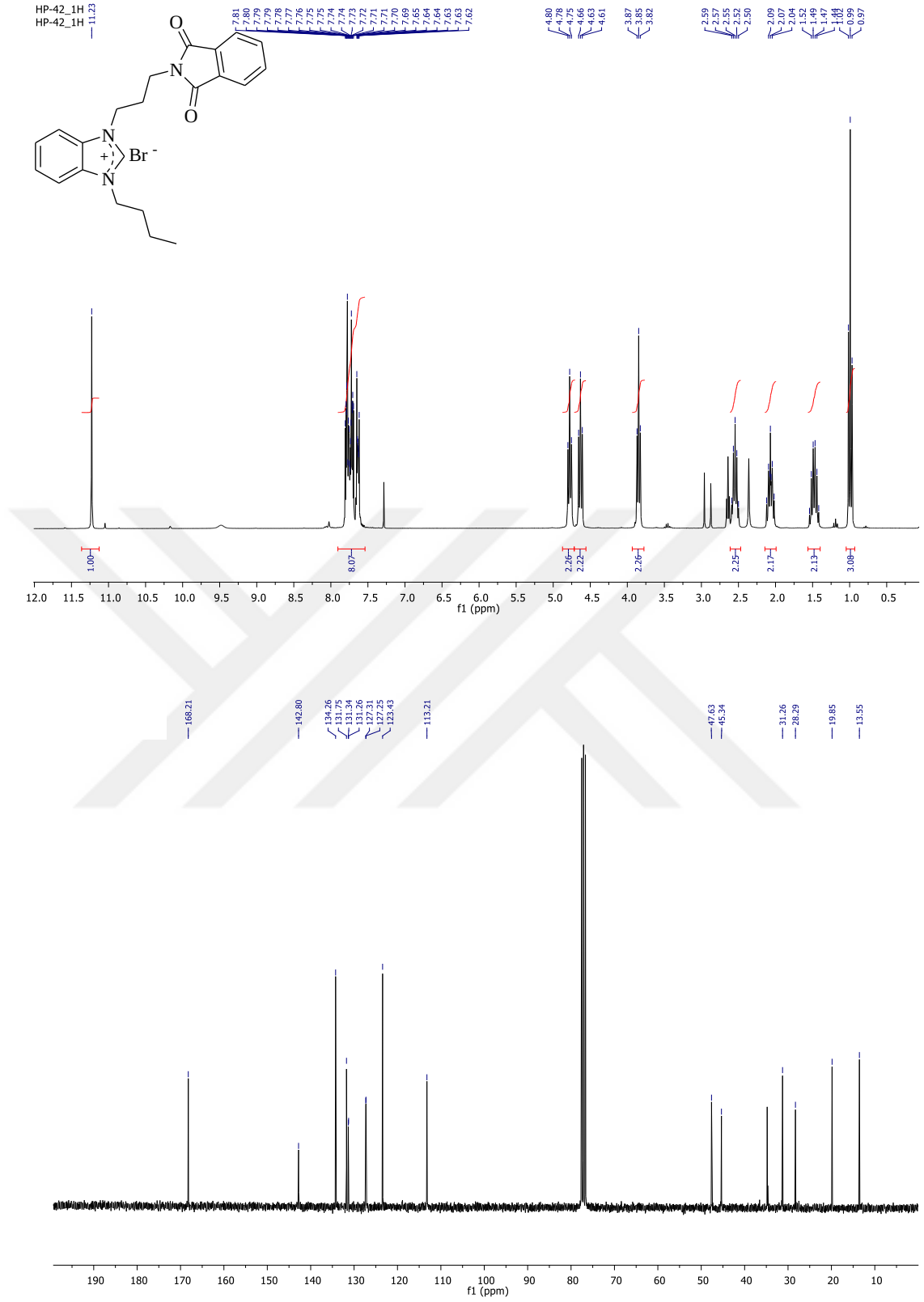
Şekil 3.1. 1-( N -propilfthalimit)-3-bütülbenzimidazolyum bromür bileşiğine ait 1 H NMR ve 13 C NMR spektrumları.
