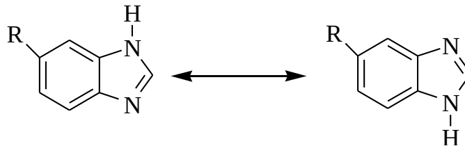
Şekil 1.1. Benzimidazollerde tautomerik denge.
