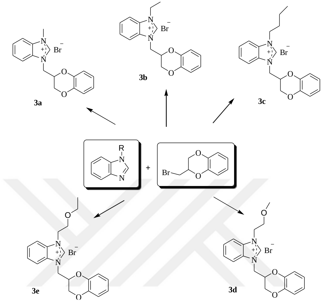
Şema 3.4. 2-metil-1,4-benzodioksan süstitüentli benzimidazolyum tuzlarının (3a-e) sentezi.
