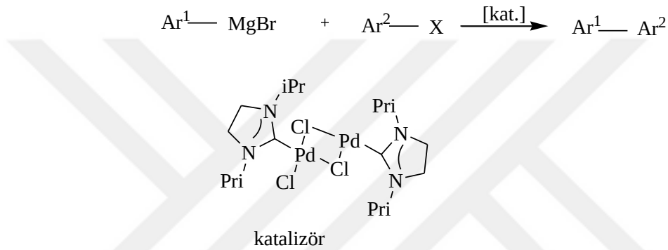
Şekil 1.11. Aril halojenürlerin Kumada-Tamao-Corriu çapraz eşleşme tepkimesi.
