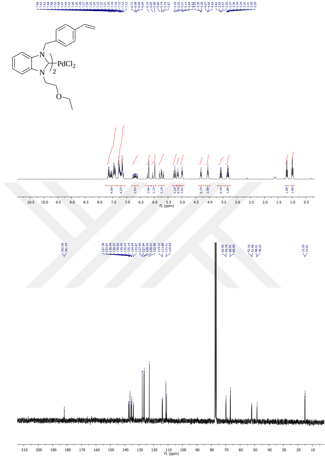
Şekil 3.5. Bis[1-(4-Vinilbenzil)-3-(2-etoksietil)benzimidazol-2-iliden]dikloro paladyum(II) bileşiğine ait 1 H NMR ve 13 C NMR spektrumları.
