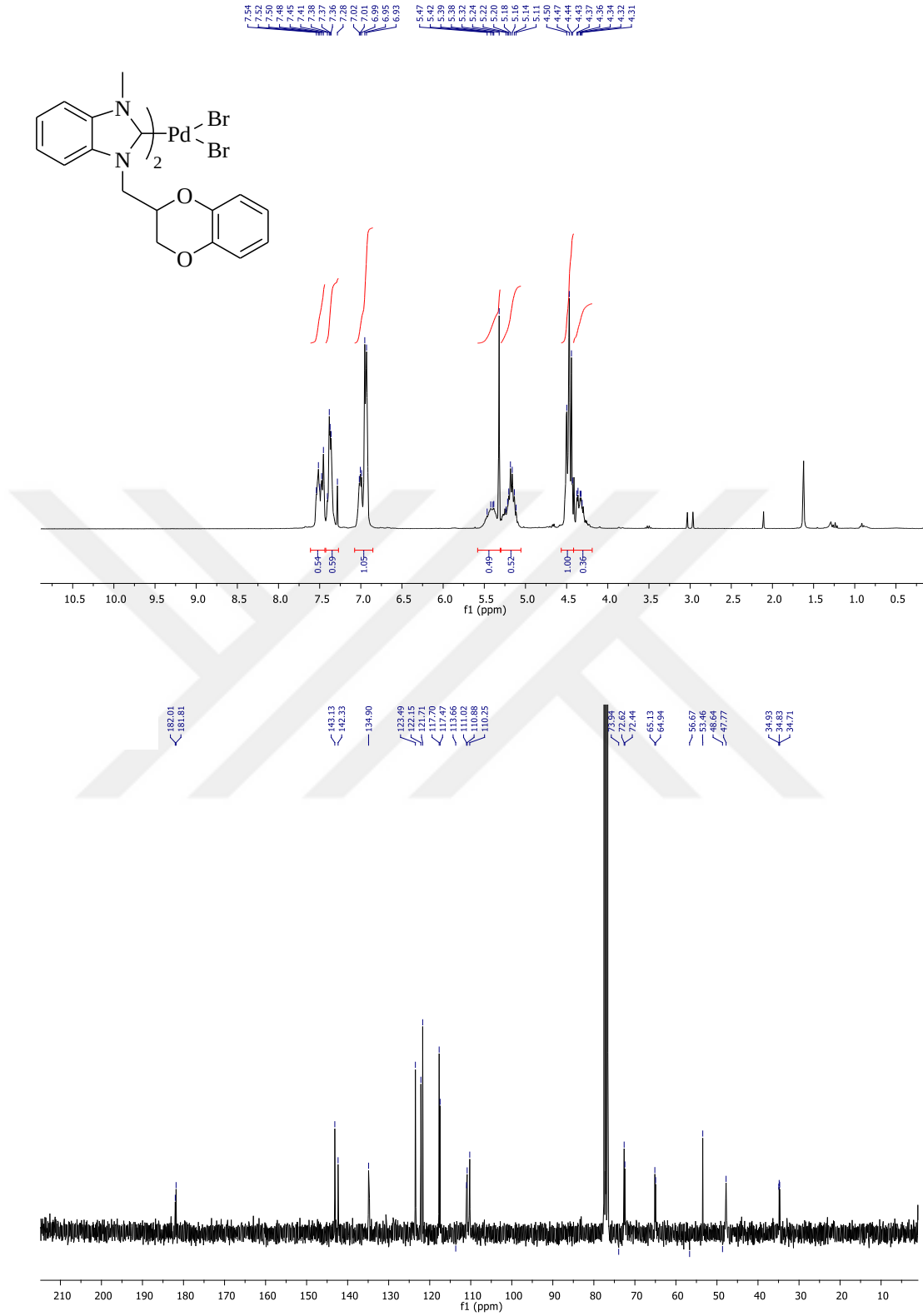
Şekil 3.6. Bis[1-(2-metil-1,4-benzodioxan)-3-metilbenzimidazol-2-iliden]dibromo paladyum (II) bileşiğine ait 1 H NMR ve 13 C NMR spektrumları.
