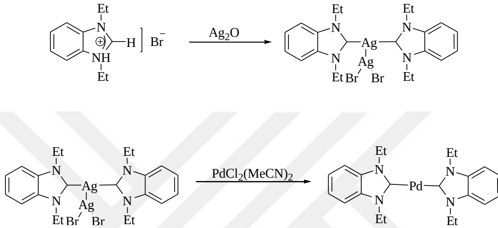
Şema 1.4. Ag-NHC üzerinden ilk transmetalasyon reaksiyonu.
