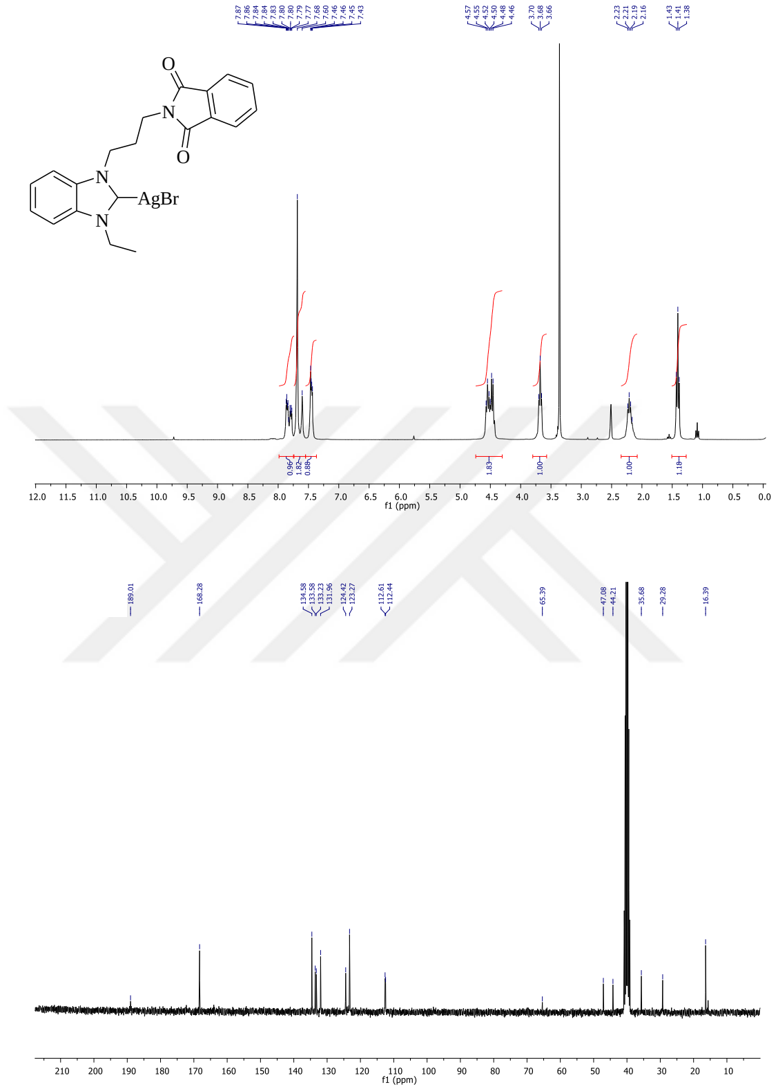
Şekil 3.3. [1-( N -propilftalimit)-3-etilbenzimidazol-2-iliden]bromür gümüş(I) bileşiğine ait 1 H NMR ve 13 C NMR spektrumları.
