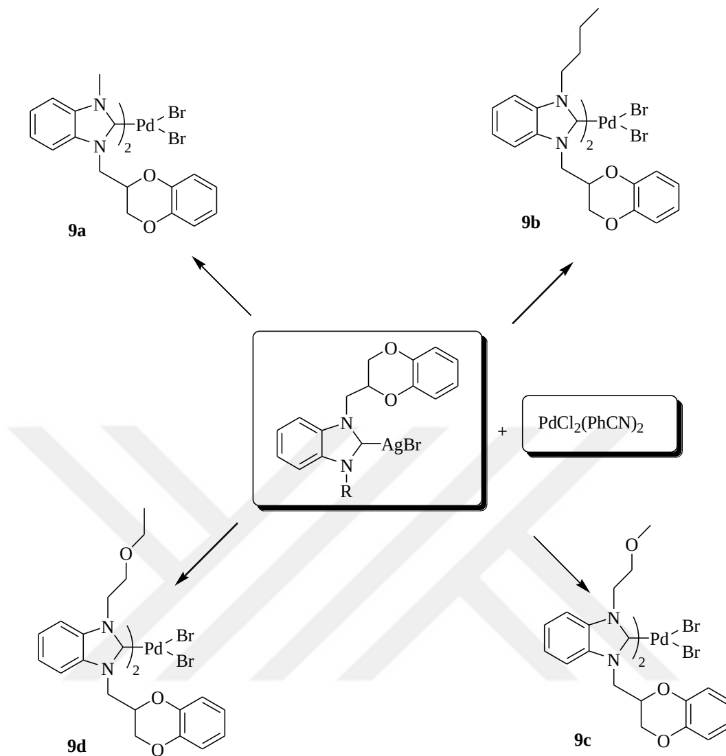
Şema 3.10. 2-metil-1,4-benzodioksan sübstitüentli Pd-NHC komplekslerinin ( 9a-d ) sentezi.
