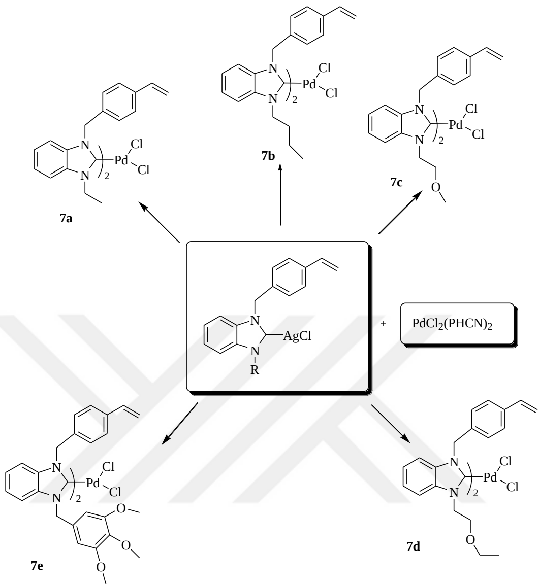
Şema 3.8. 4-vinilbenzil sübstitüentli Pd-NHC komplekslerinin ( 7a-e ) sentezi.
