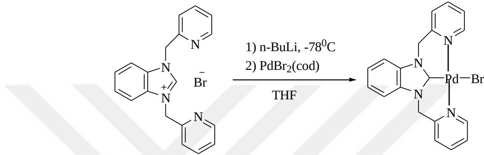
Şema 1.7. Benzimidazol türevinin deprotonasyonu ile metal kompleksi sentezi.
