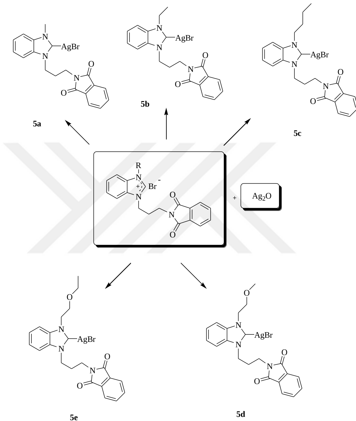
Şema 3.6. N-propilftalimit süstitüentli Ag-NHC komplekslerinin sentezi.
