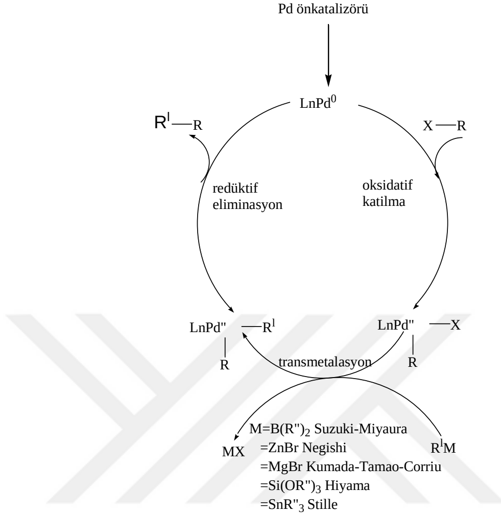
Şema 1.11. Transmetalatlamanın kullanıldığı genelleştirilmiş çapraz bağlanma mekanizması.
