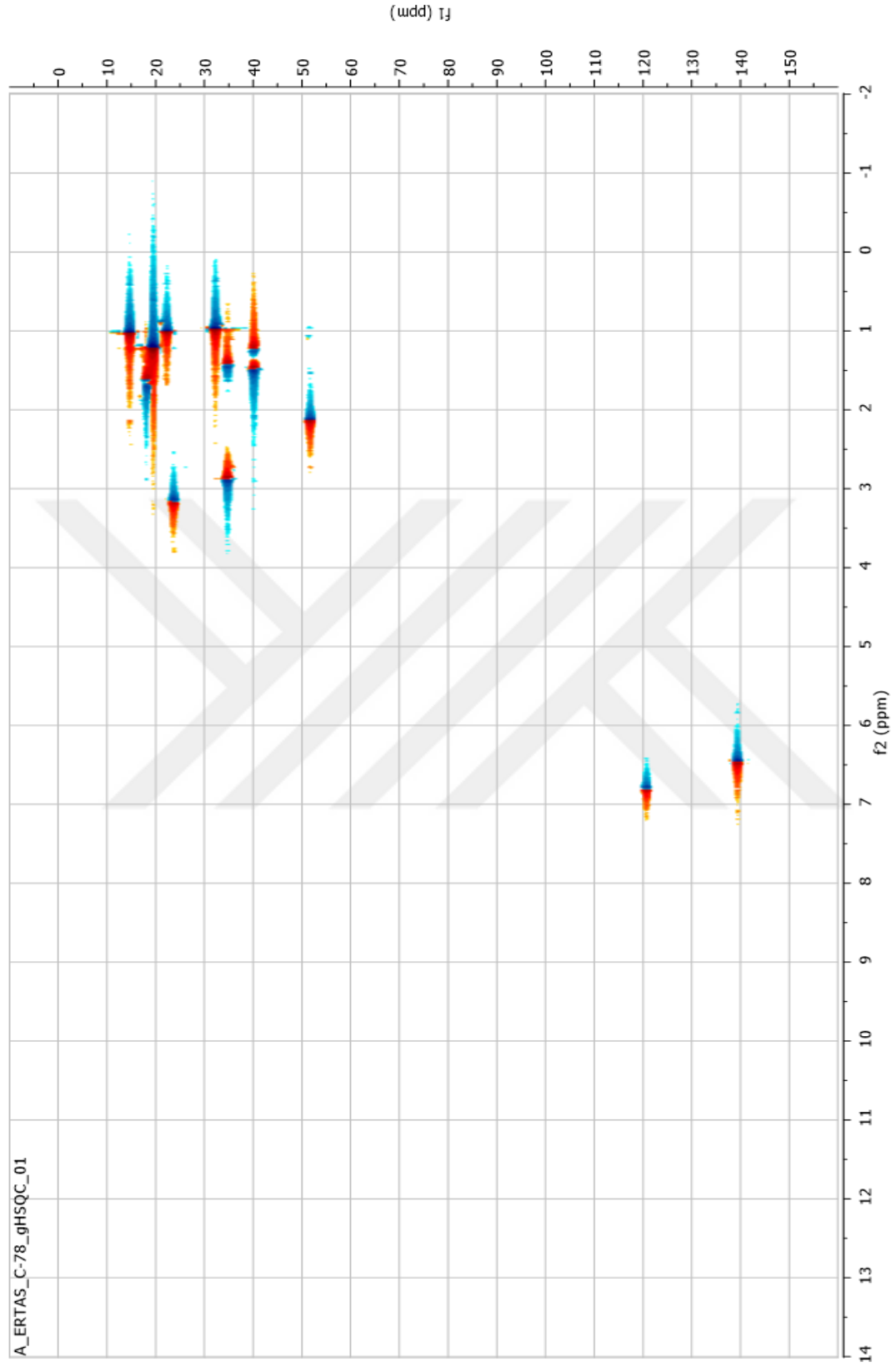
Şekil 76. 6,7-Dehidroroyleanon Bileşiğinin HMQC Spektrumu ( \text{CDCl}_3 , 600 MHz)
