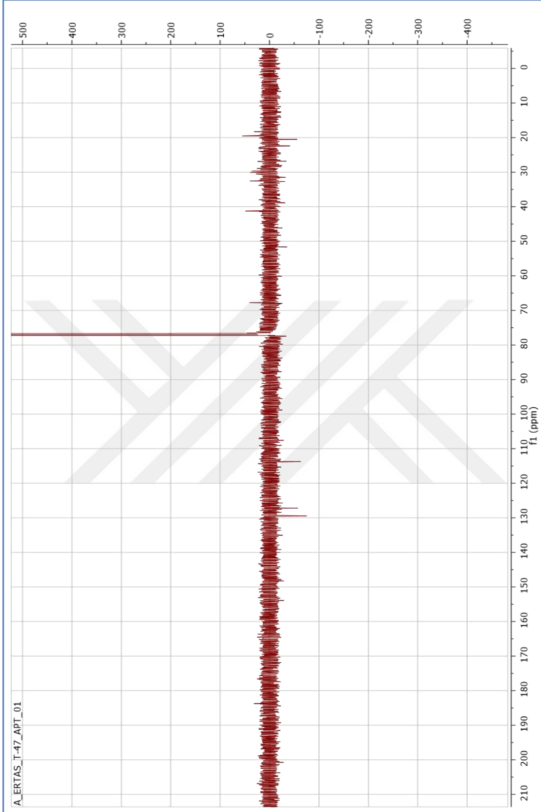
Şekil 110. Pisiferal Bileşiğinin APT Spektrumu (CDCl 3 , 600 MHz)
