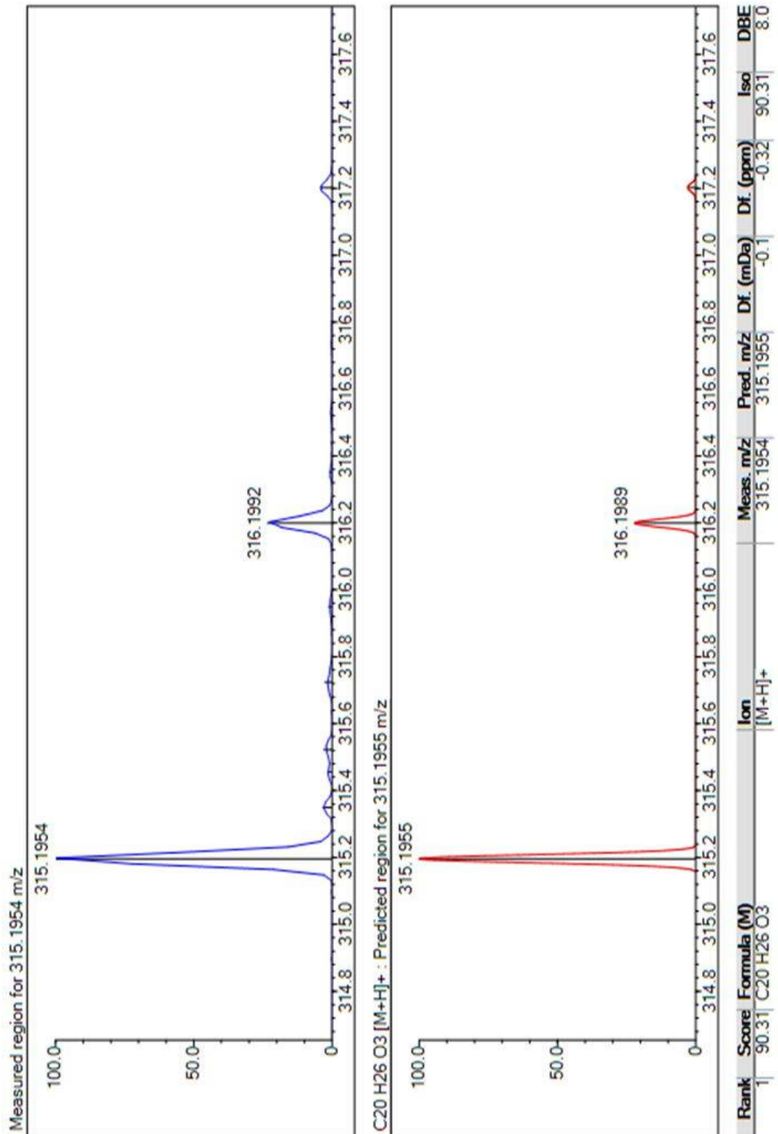
Şekil 78. 6,7-Dehidroroleanon bileşiğinin LC-MS-IT-TOF kromatogramı
