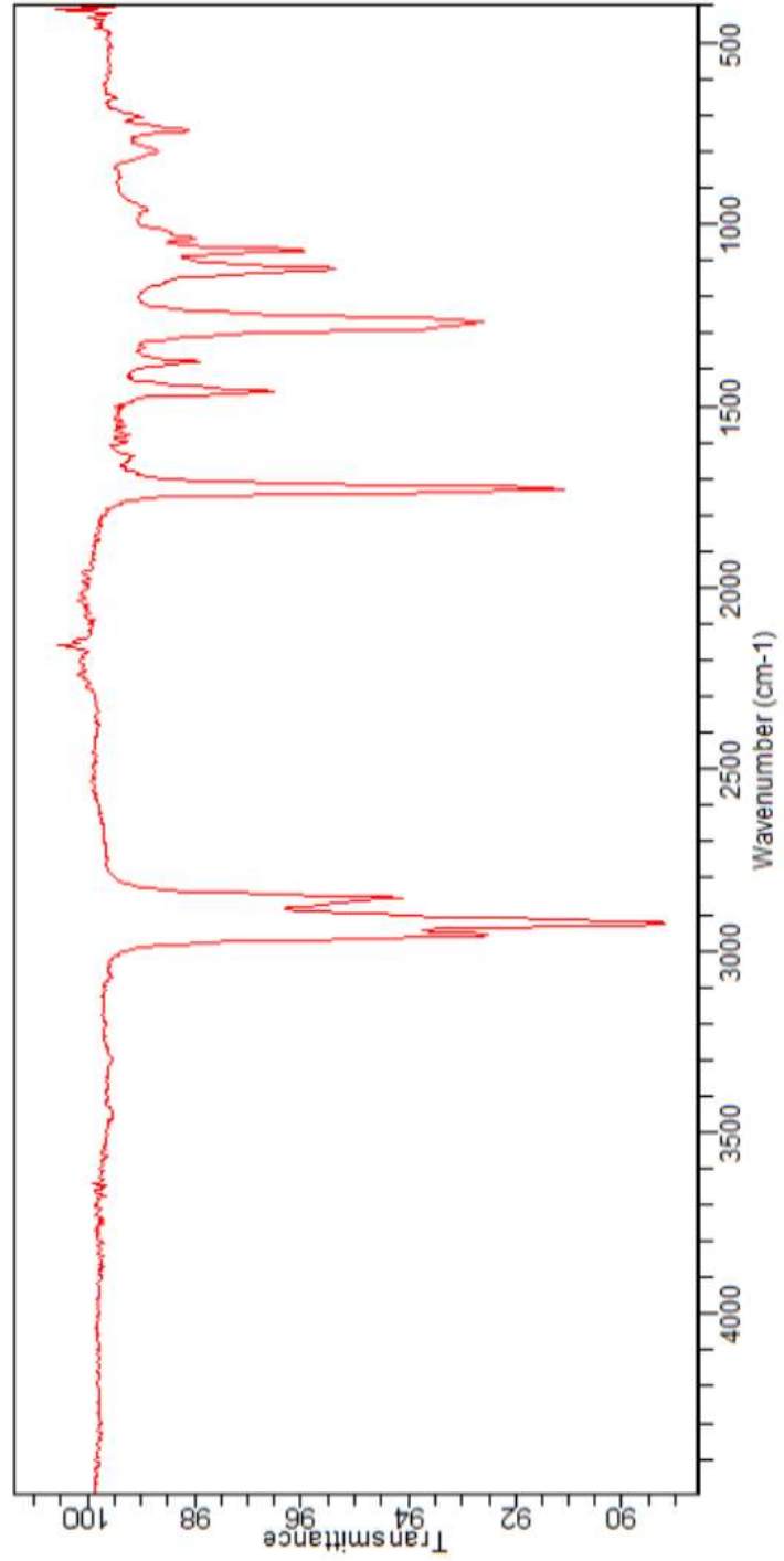
Şekil 97. Bis-(2-etil heksil) benzen-1,2 dikarboksilat bileşiğinin IR spektrumu
