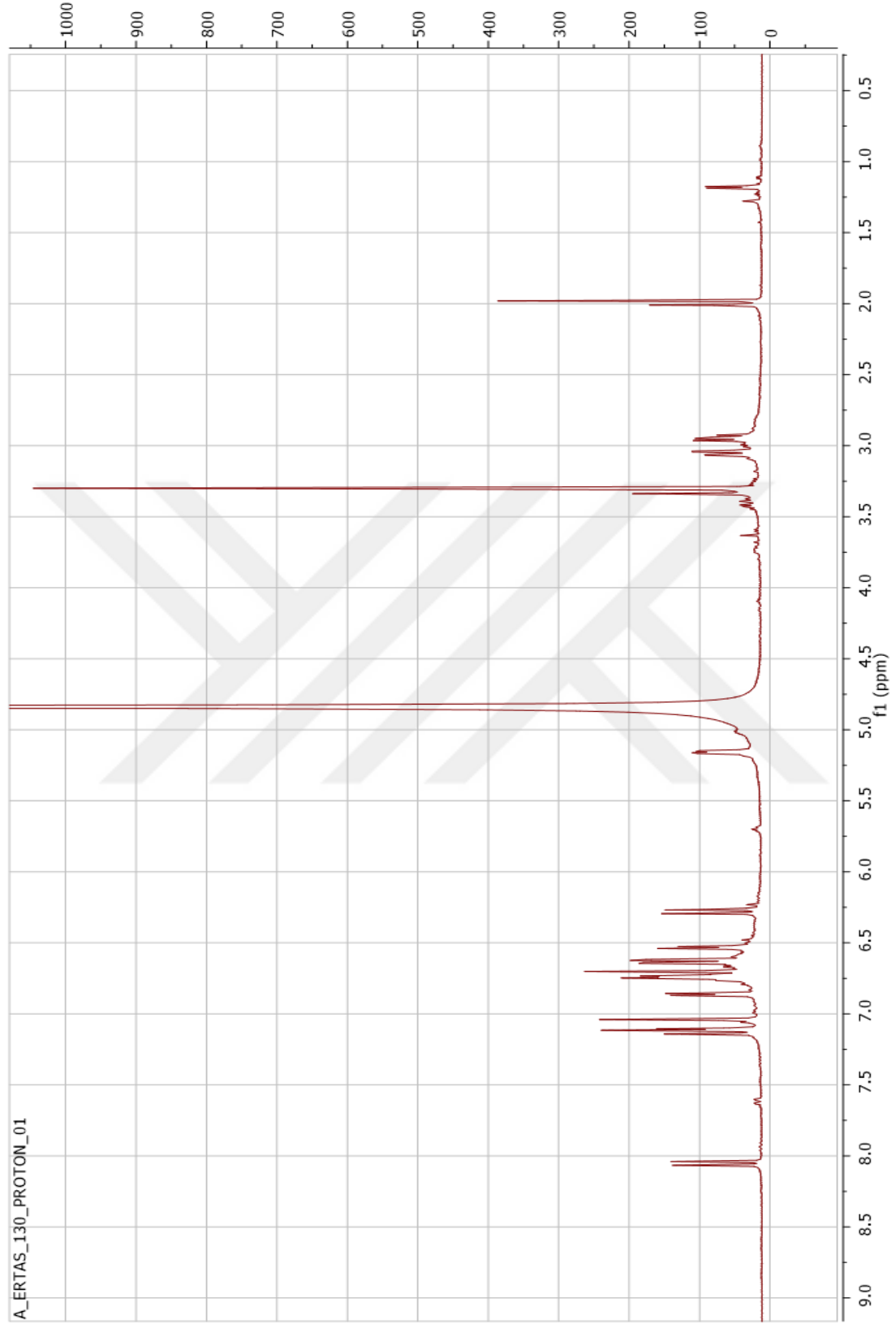
Şekil 90. Salvianolik Asit Abileşiginin ^1\text{H} NMR spektrumu ( \text{CD}_3\text{OD} , 600 MHz)
