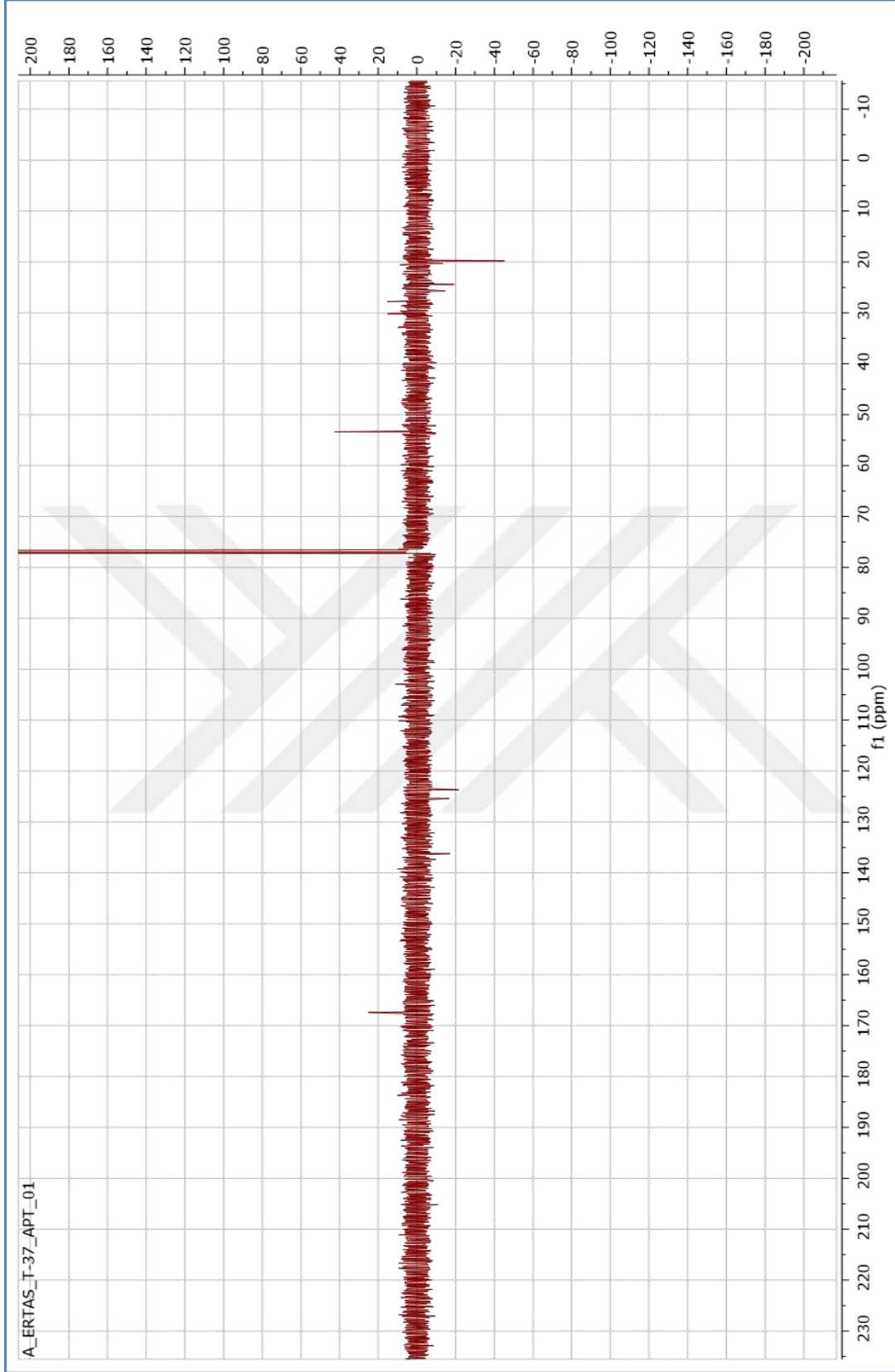
Şekil 136. Salvipison Bileşiğinin APT Spektrumu ( CDCl_3 , 600 MHz)
