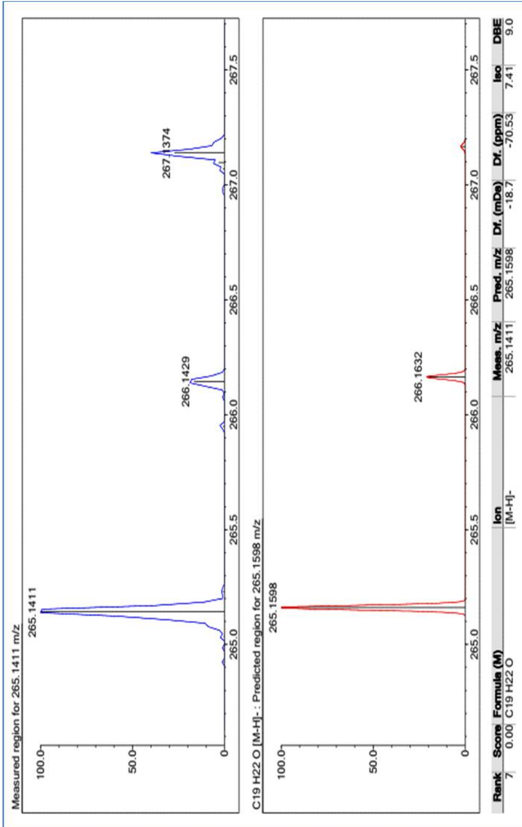
Şekil 133. 12-Demetil multikaulin Bileşiğinin LC-MS-IT-TOF Kromatogram
