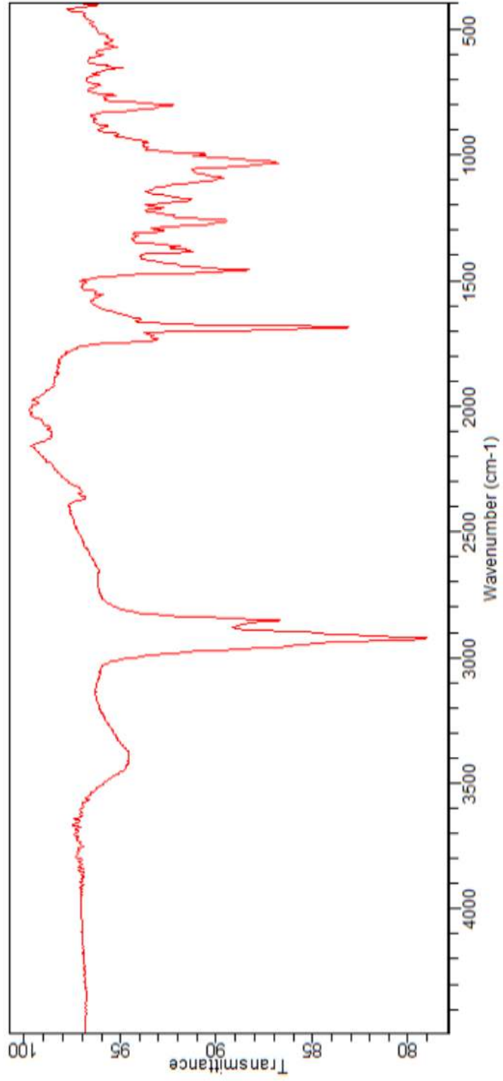
Şekil 88. Oleanolik asit bileşiğinin IR spektrumu
