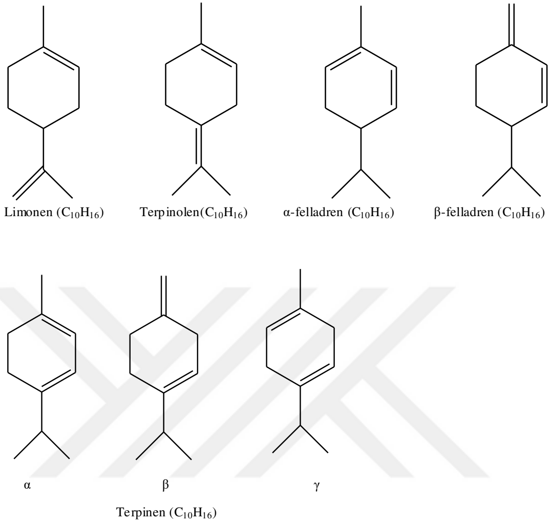
Şekil 4. Monosiklik monoterpenler
