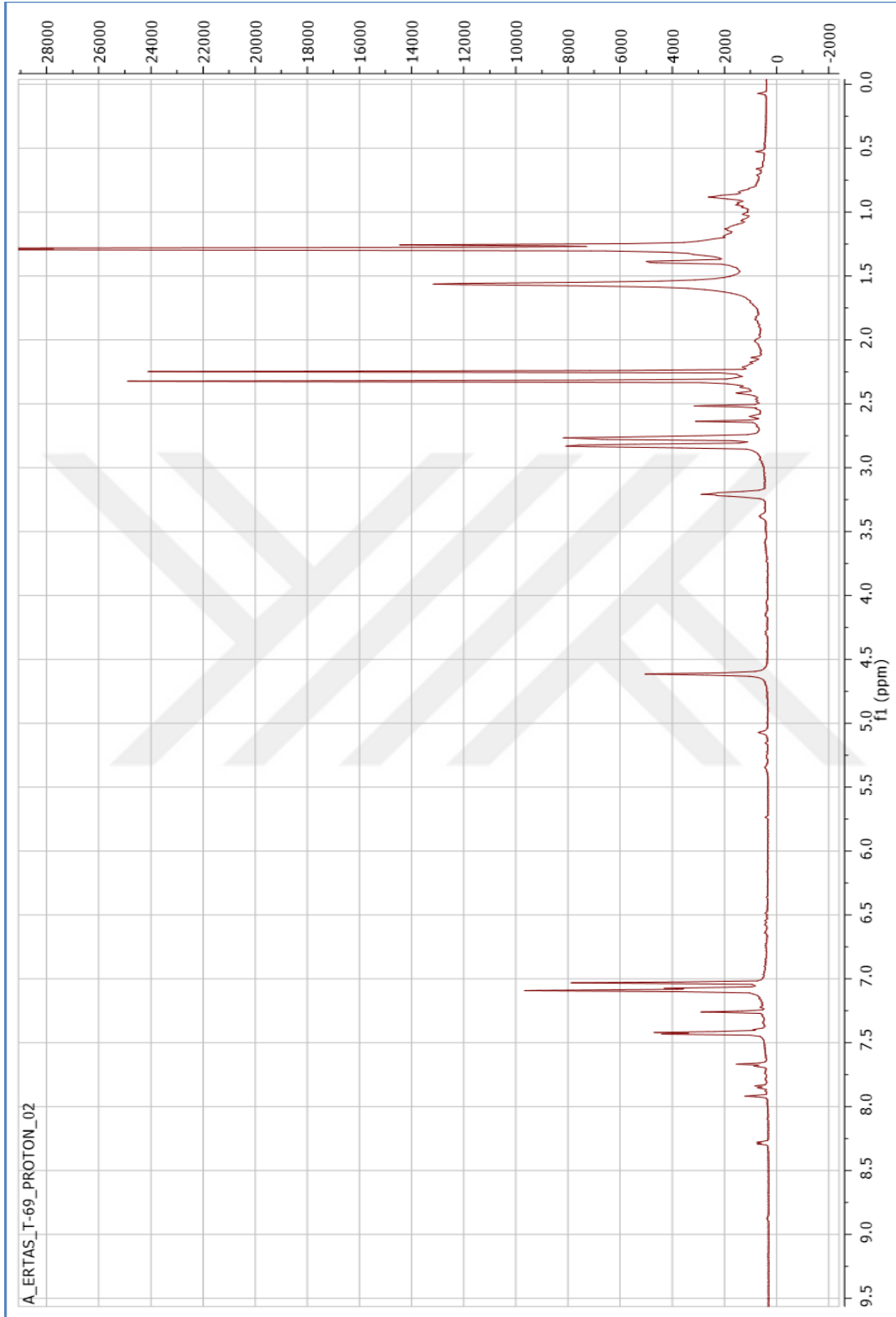
Şekil 121. 12-Hidroksi abieta 1,3,5(10), 8, 11, 13-hekzaen Bileşiğinin ^1\text{H} NMR Spektrumu ( \text{CDCl}_3 , 600 MHz)
