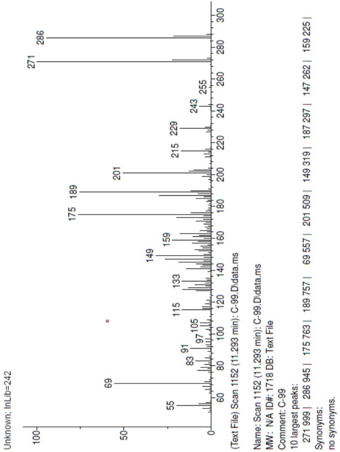
Şekil 64. Ferruginol bileşiğinin GC-MS kromatogramı
