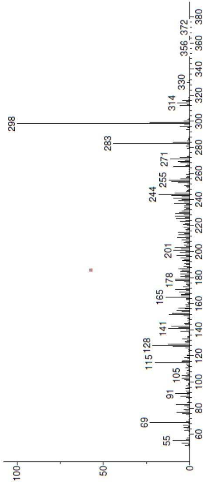
Şekil 77. 6,7-Dehidroroyleanon bileşiğinin GC-MS spektrumu
