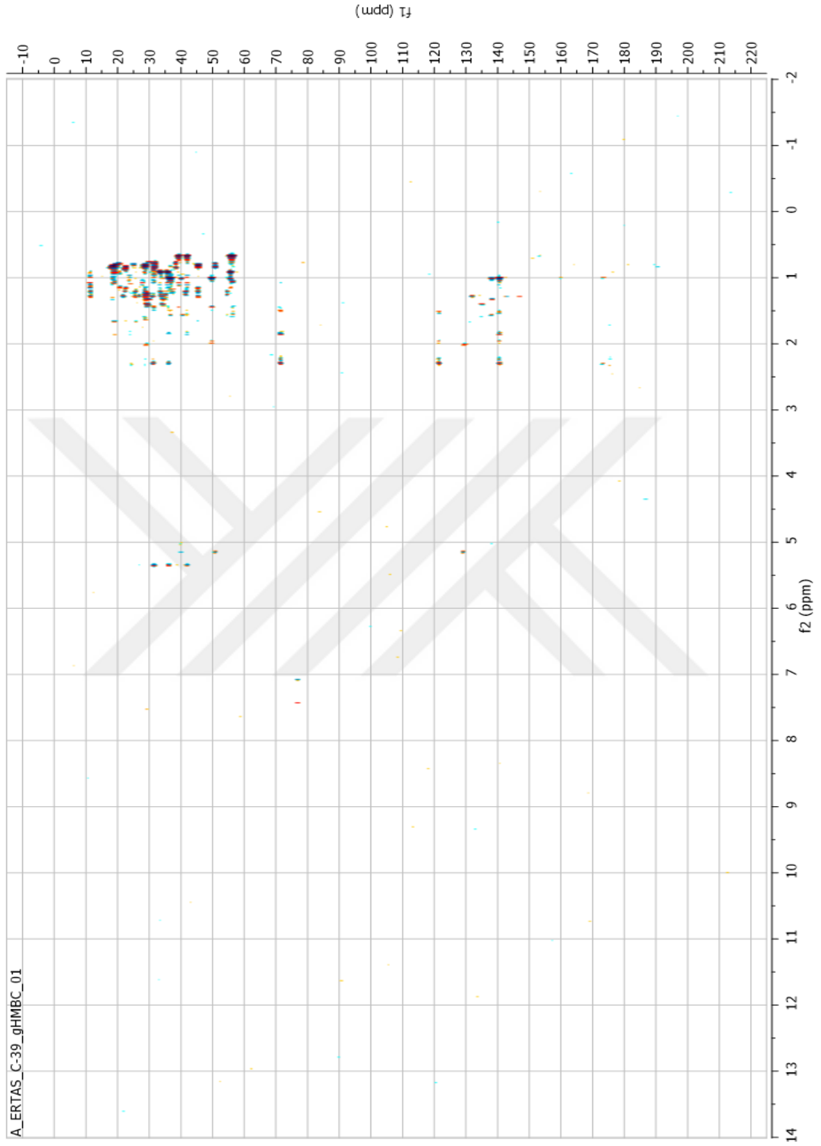
Şekil 54.β-Sitosterol bileşiğinin HMBC spektrumu ( \text{CDCl}_3 , 600 MHz)
