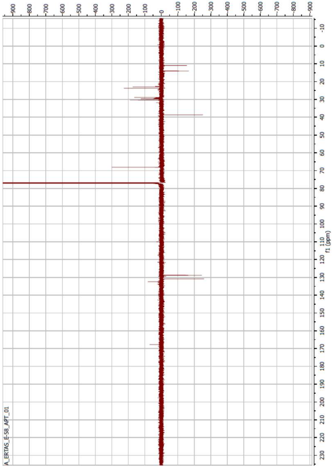
Şekil 104. Bis(2-etilheksil) tereftalat bileşiğinin APT s spektrumu ( \text{CDCl}_3 , 150 MHz)
