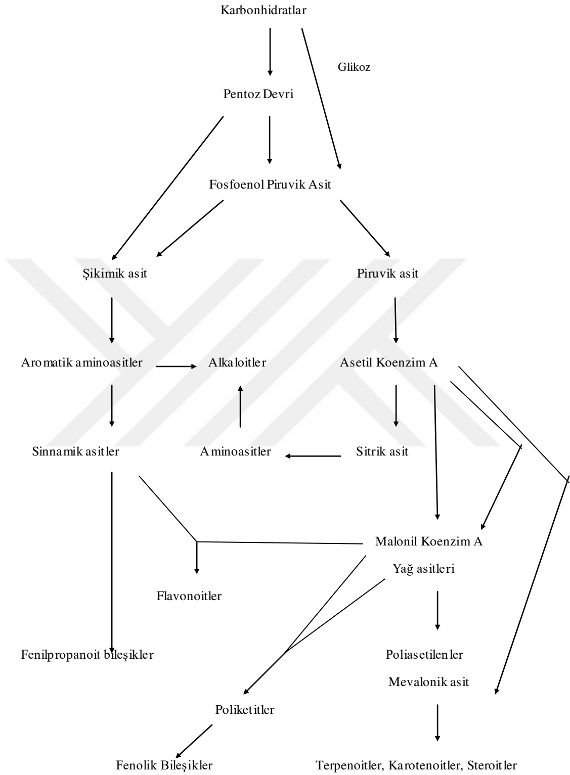
Şekil 1.Sekonder metabolitlerin oluşumu
