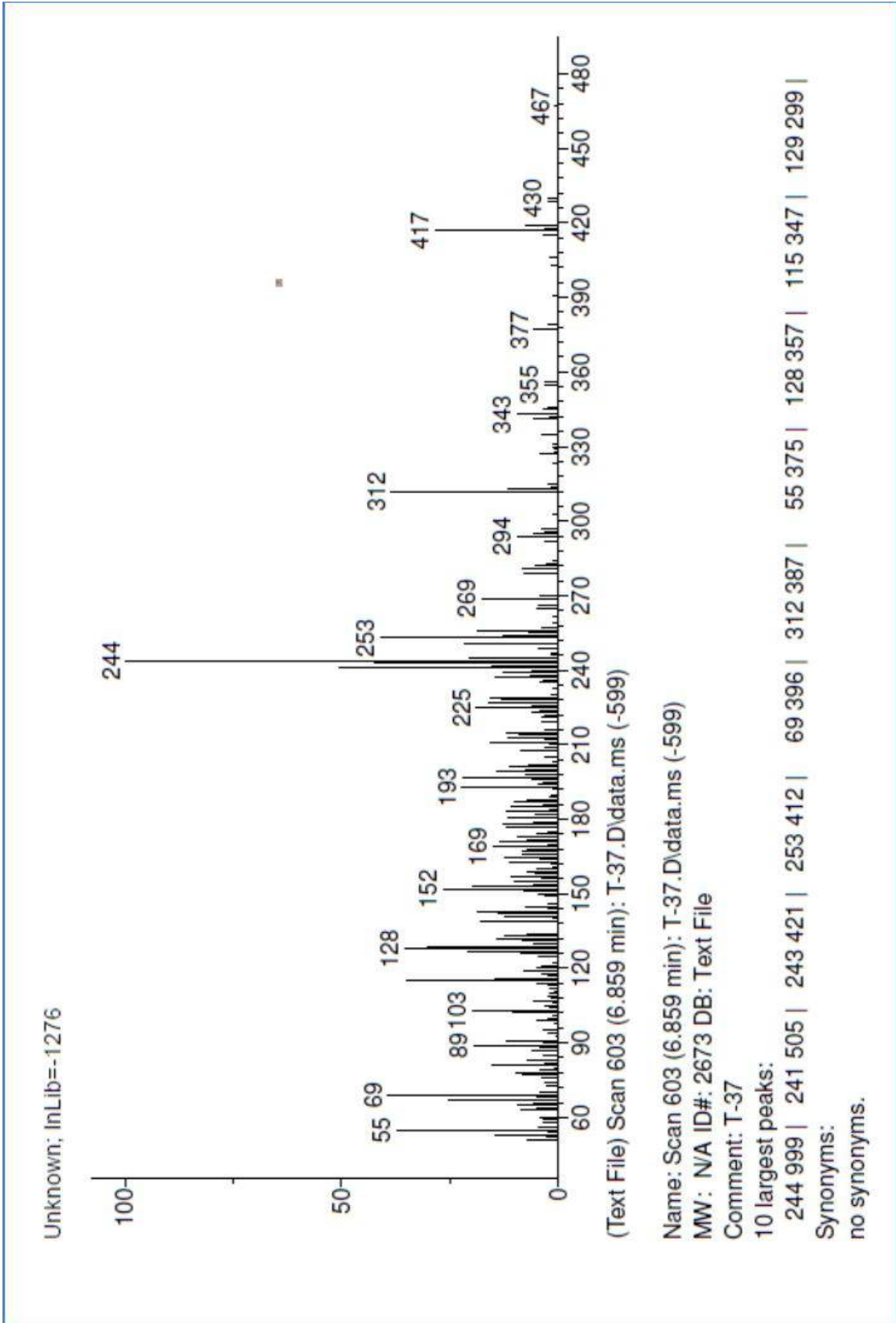
Şekil 138. Salvipison Bileşiğinin GC-MS Spektrumu
