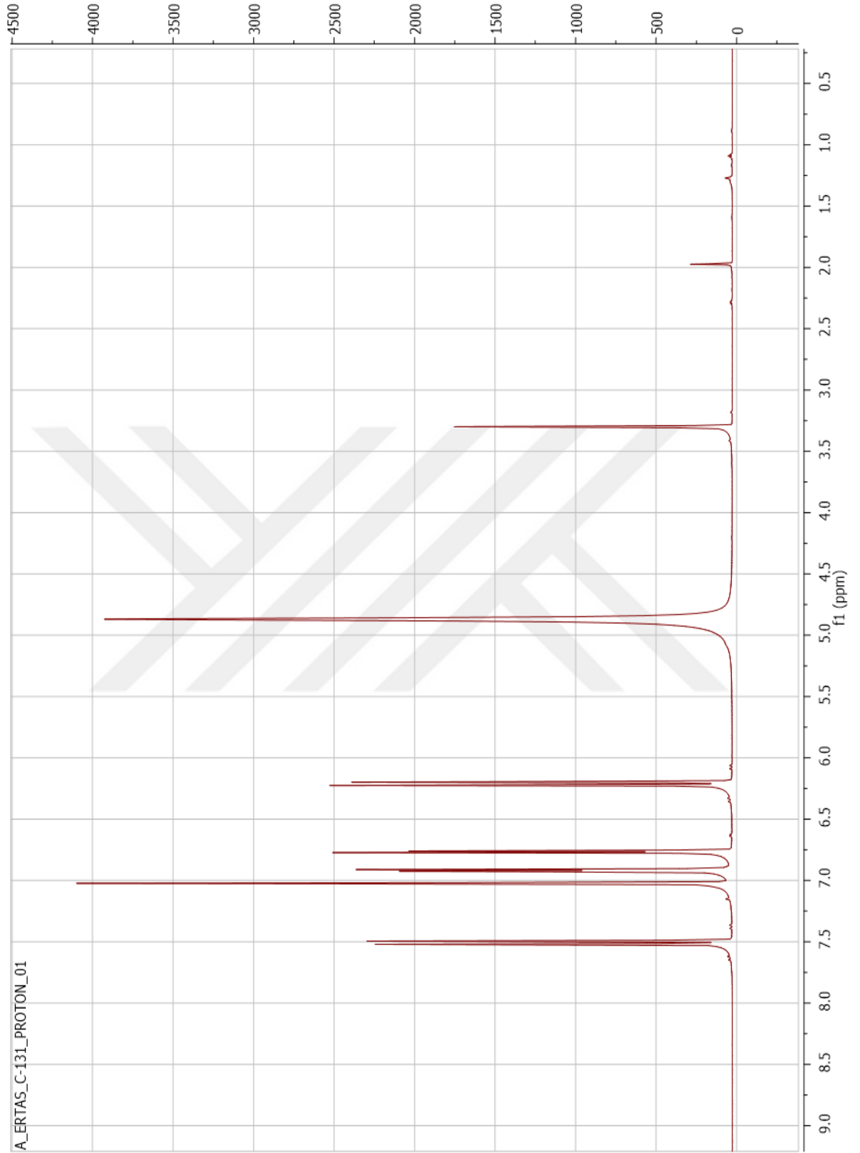
Şekil 36. Kaffeyk asit bileşığının ^1\text{H} NMR spektrumu ( \text{CD}_3\text{OD} , 600 MHz)
