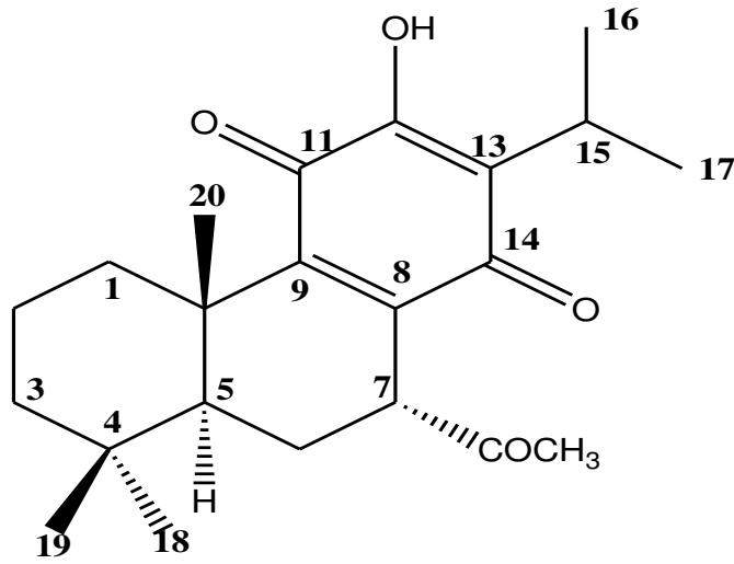
Şekil 45. 7-Asetil royleanon
