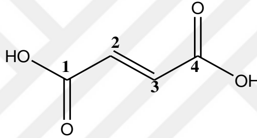
Şekil 32. Fumarik Asit
