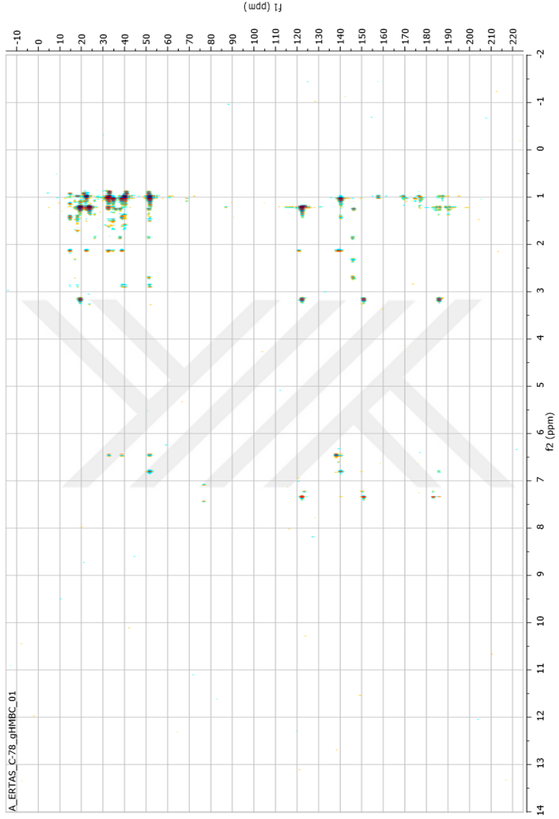
Şekil 75. 6,7-Dehidroroyleanon bileşiğinin HMBC spektrumu (CDCl 3 , 600 MHz)
