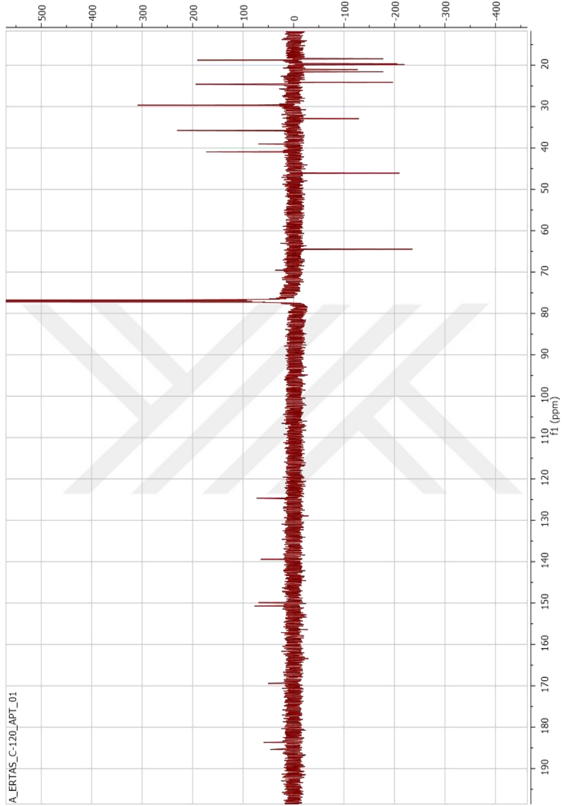
Şekil 47. 7-Asetil royleanon bileşiğinin ^{13}\text{C} NMR (APT) spektrumu ( \text{CDCl}_3 , 150 MHz)
