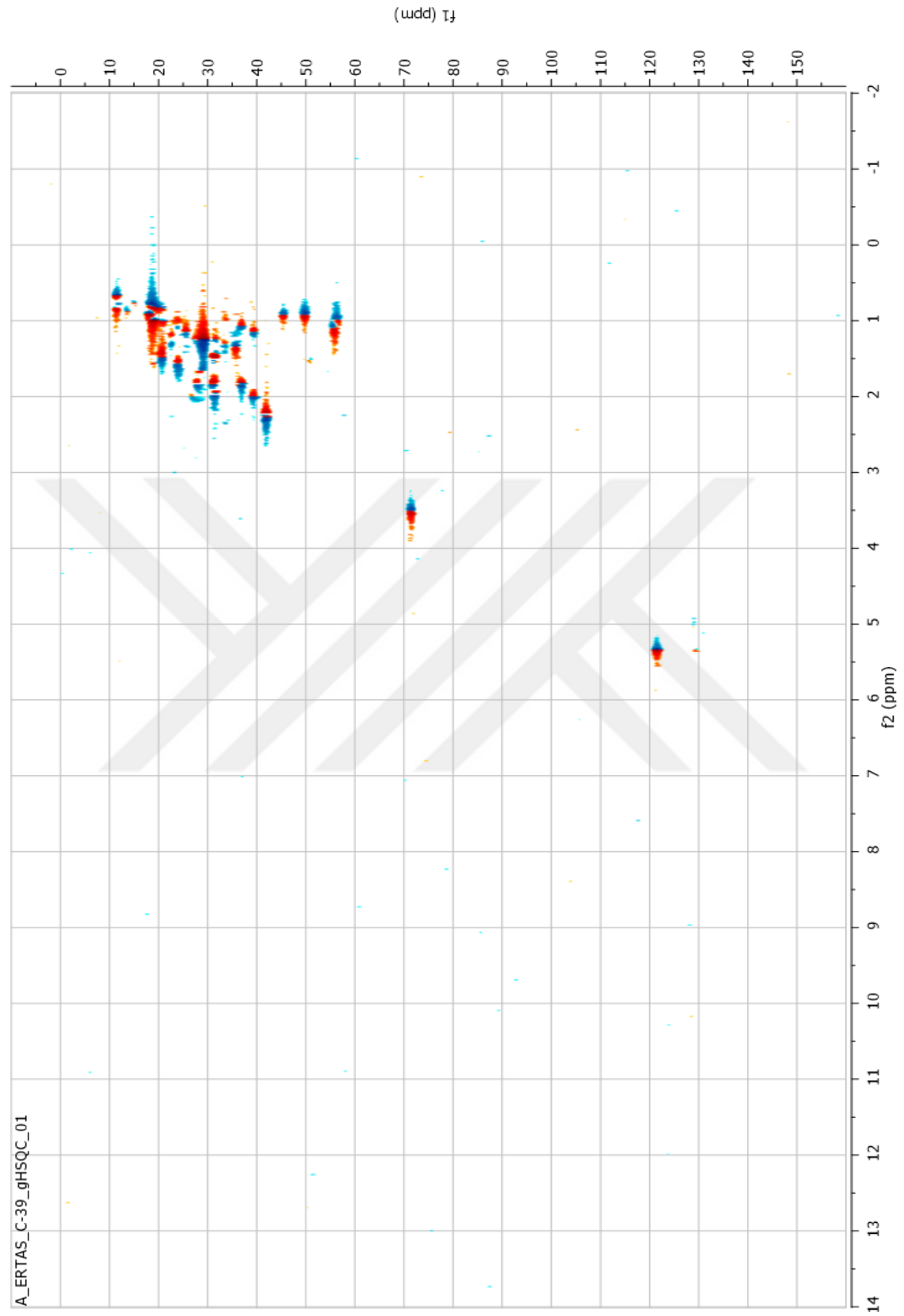
Şekil 55. \beta -Sitosterol bileşiğinin HMQC spektrumu ( \text{CDCl}_3 , 600 MHz)
