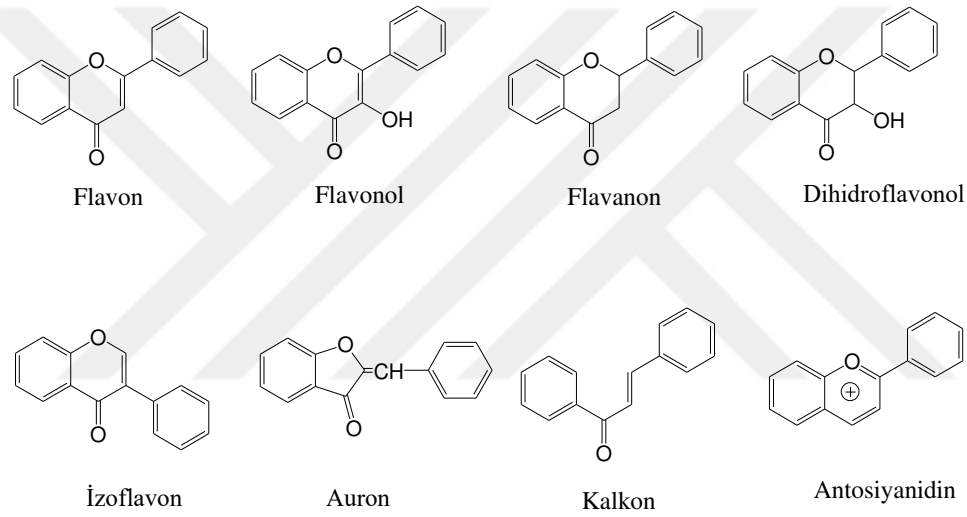
Şekil 15. Flavonoit iskeletleri
