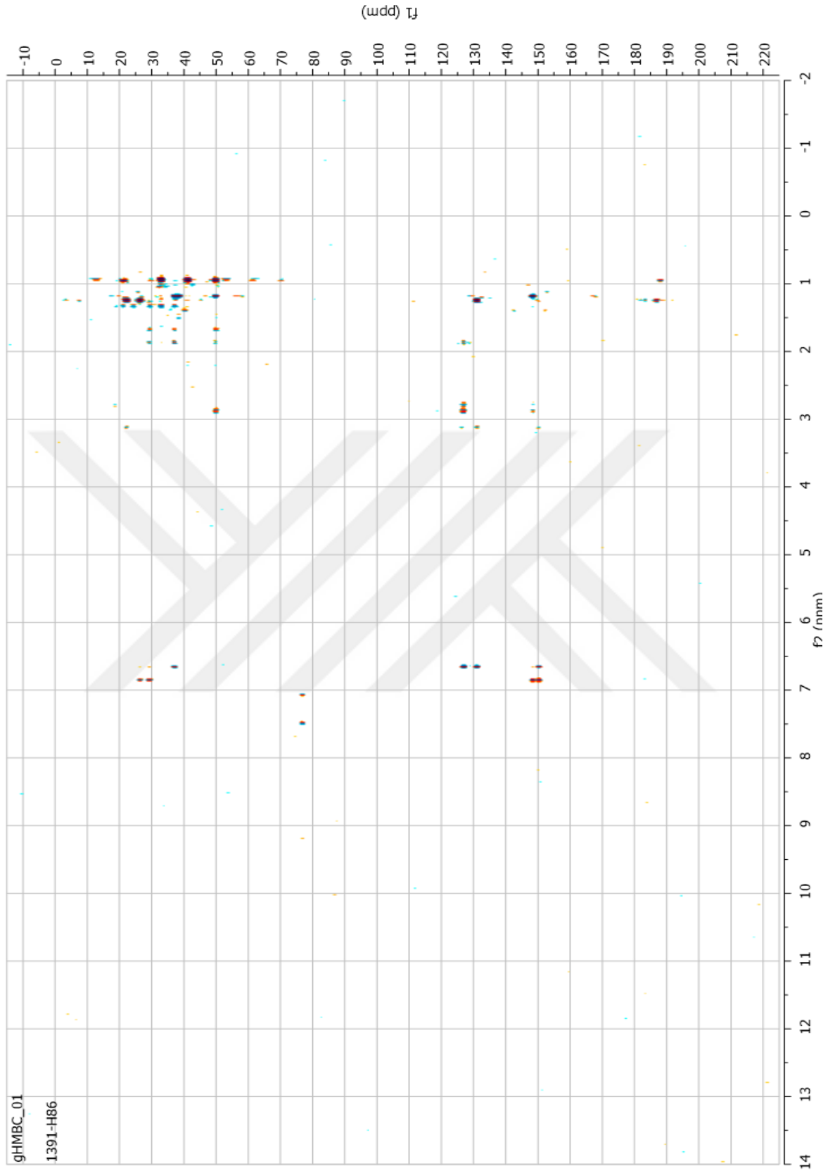
Şekil 62. Ferruginol bileşiminin HMBC spektrumu (CDCl 3 , 600 MHz)
