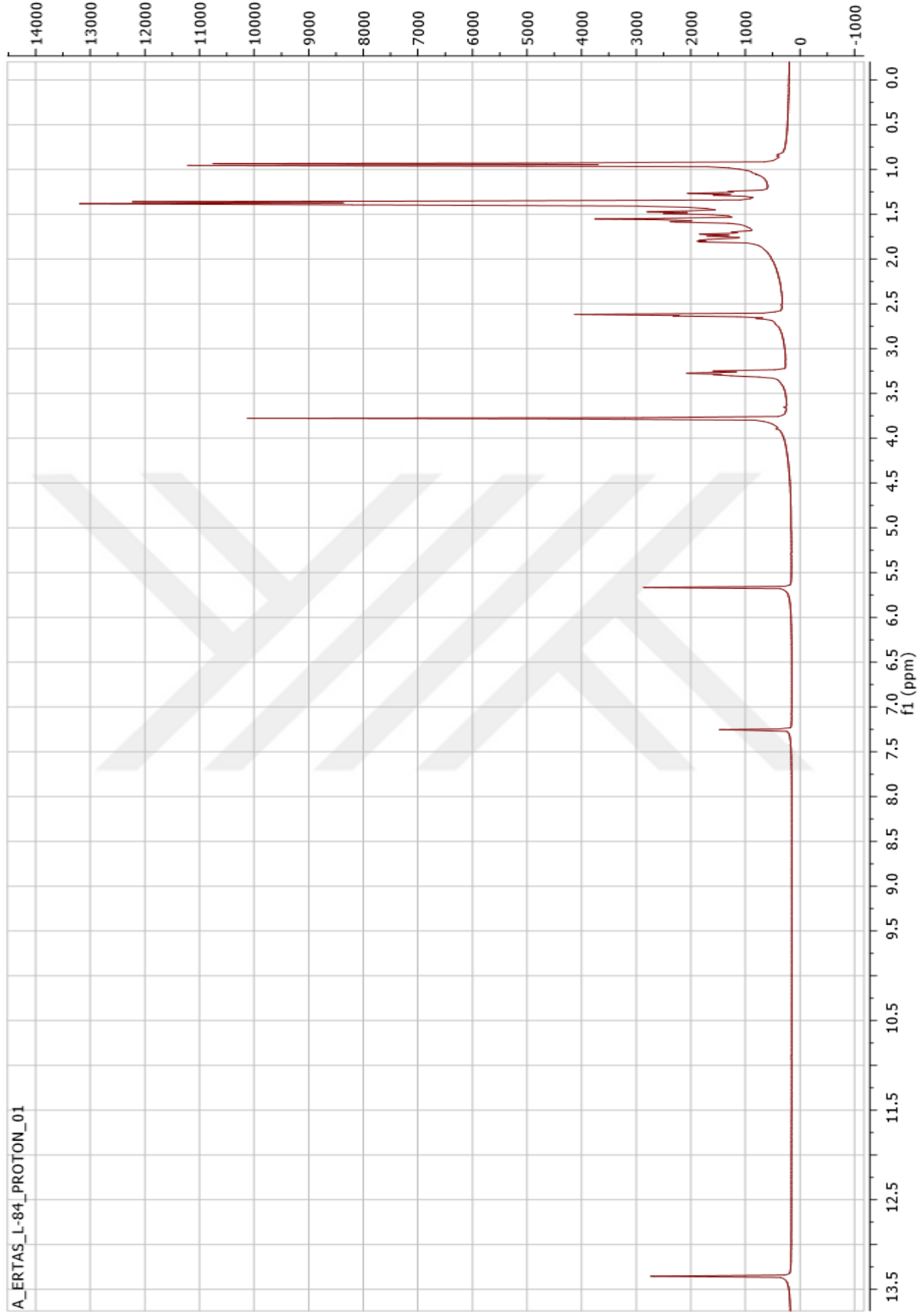
Şekil 67. Inuroyleanol bileşiğinin ^1\text{H} -NMR Spektrumu ( \text{CDCl}_3 , 600 MHz)
