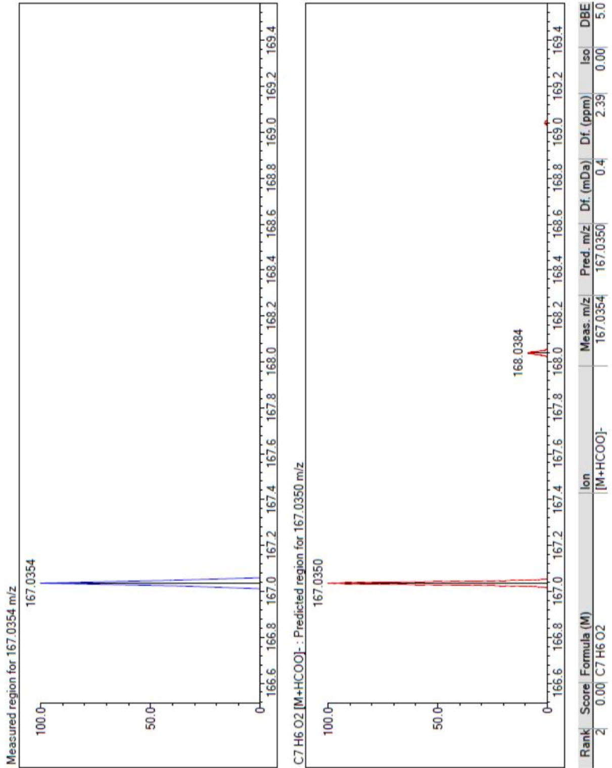
Şekil 43. 4-Hidroksi benzoik asit bileşiğinin LC-MS-IT-TOF kromatogramı
