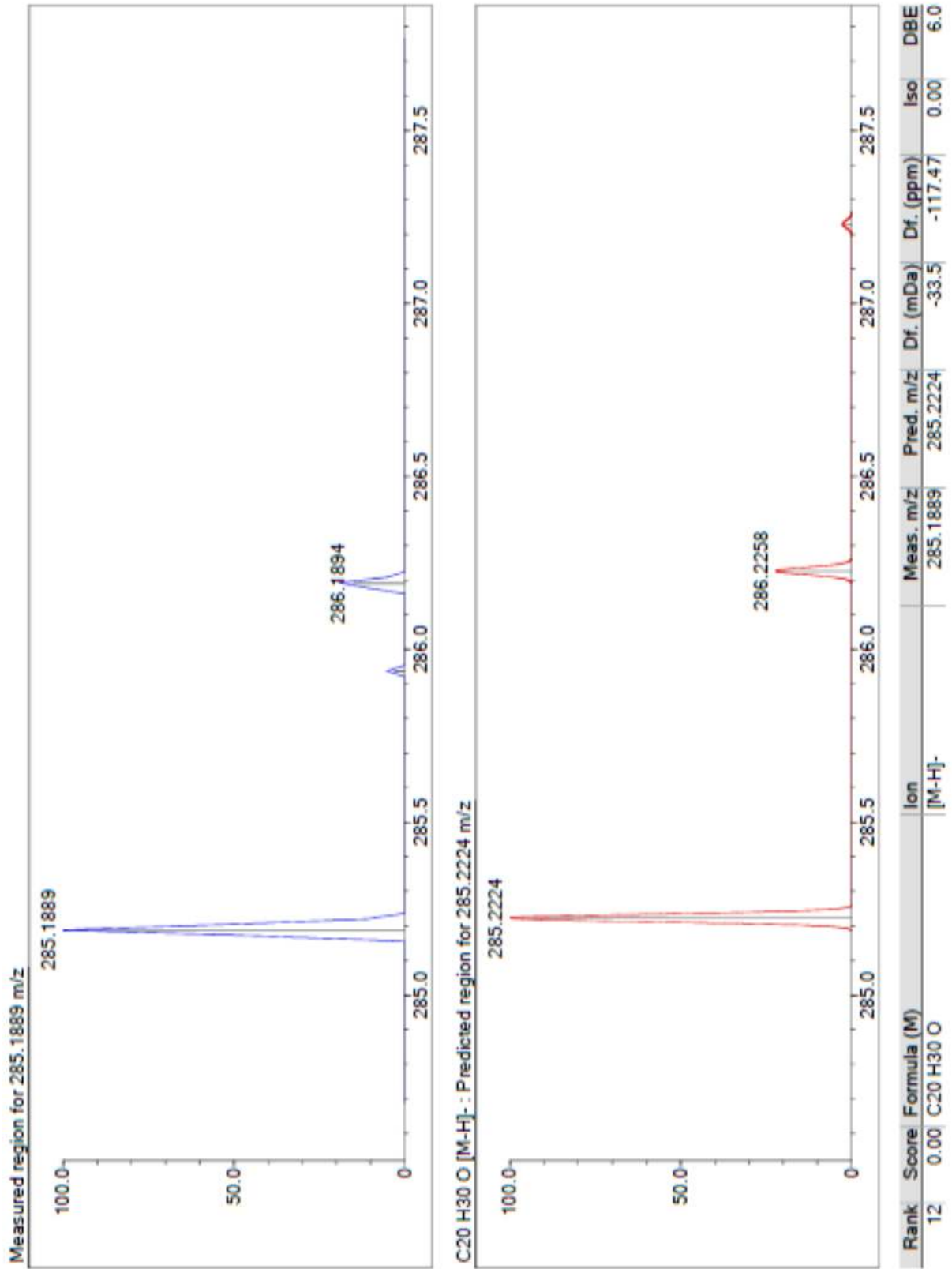
Şekil 65. Ferruginol bileşiğinin LC-MS-IT-TOF kromatogramı
