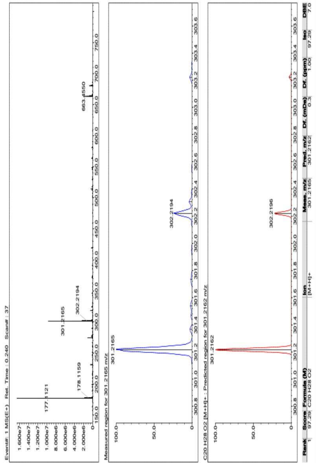
Şekil 119. Sugiol bileşiğinin LC-MS-IT-TOF kromatogramı
