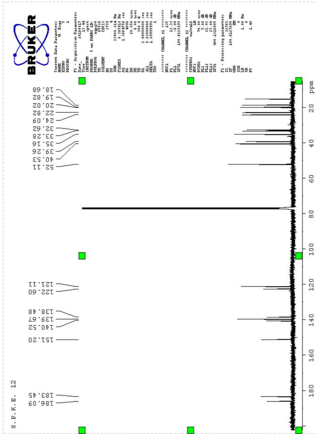
Şekil 73. 6,7-Dehydroroyleanon bileşiğinin ^{13}\text{C} NMR Spektrumu ( \text{CDCl}_3 , 150 MHz)
