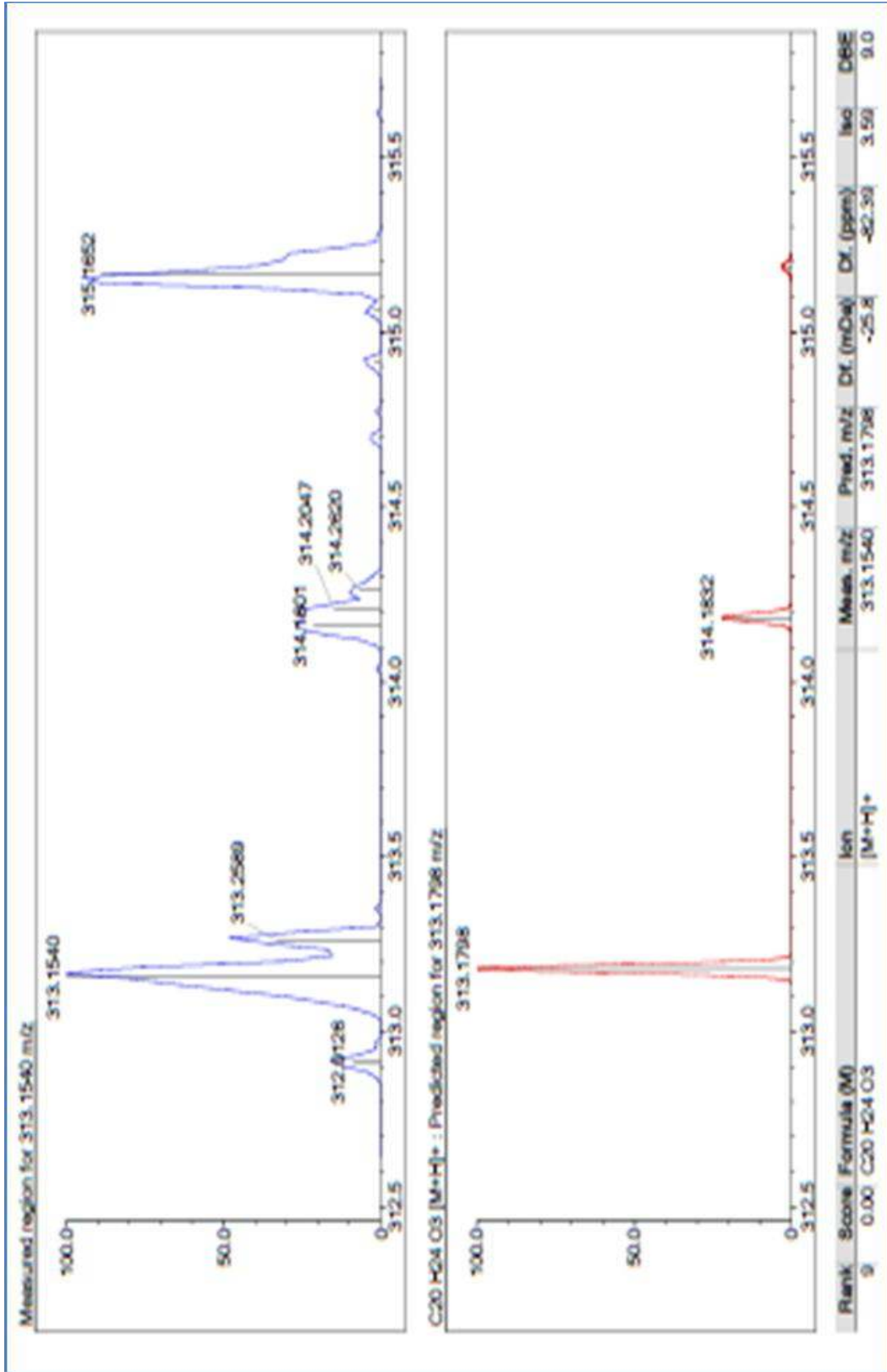
Şekil 139. Salvipison Bileşiğinin LC-MS-IT-TOF Kromatogramı
