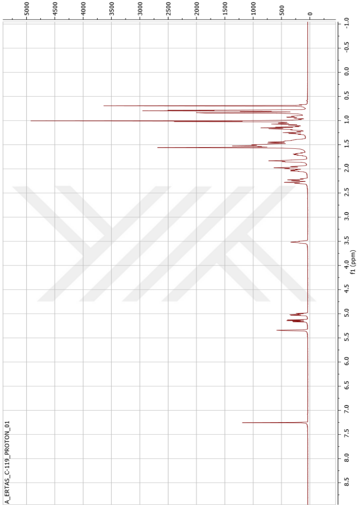
Şekil 99. Stigmasterol bileşiğinin ^1\text{H} NMR spektrumu ( \text{CDCl}_3 , 600 MHz)
