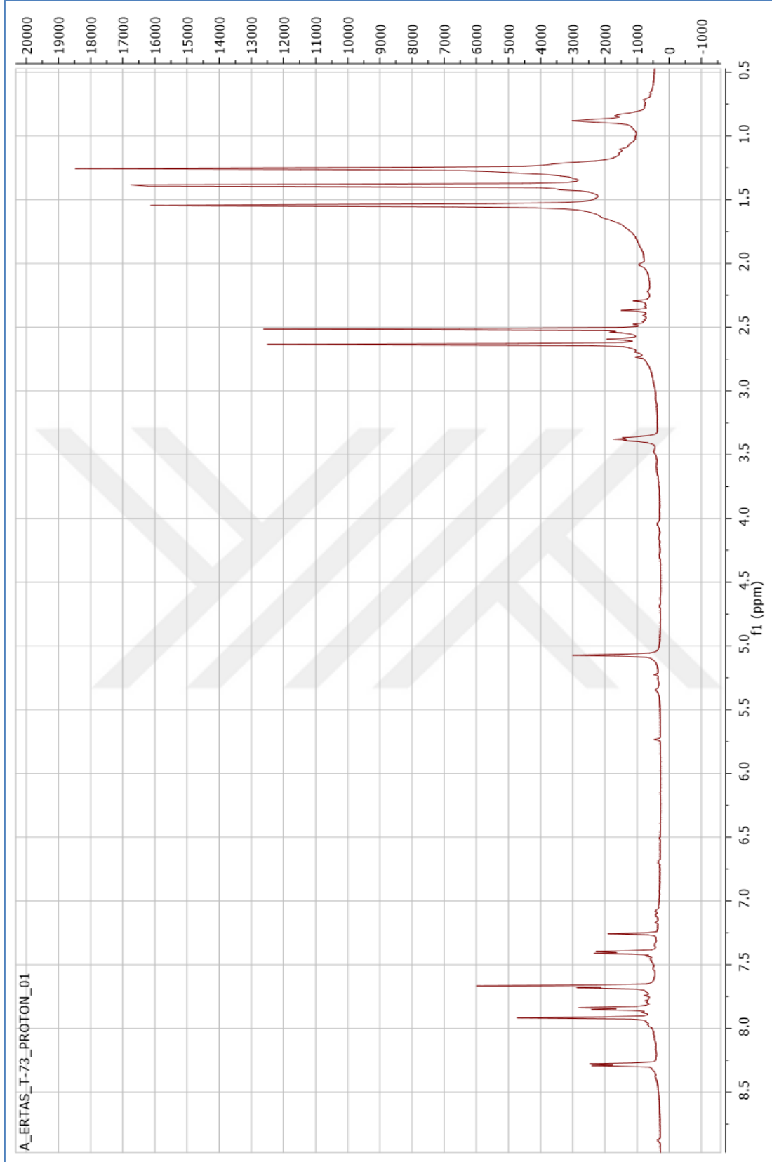
Şekil 128. 12-Demetilmultikaulin Bileşiğinin 1 H NMR Spektrumu (CDCl 3 , 600 MHz)
