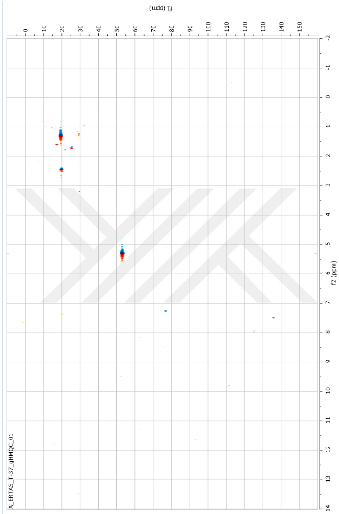
Şekil 137. Salvipison Bileşiğinin HMQC Spektrumu (CDCl 3 , 600 MHz)
