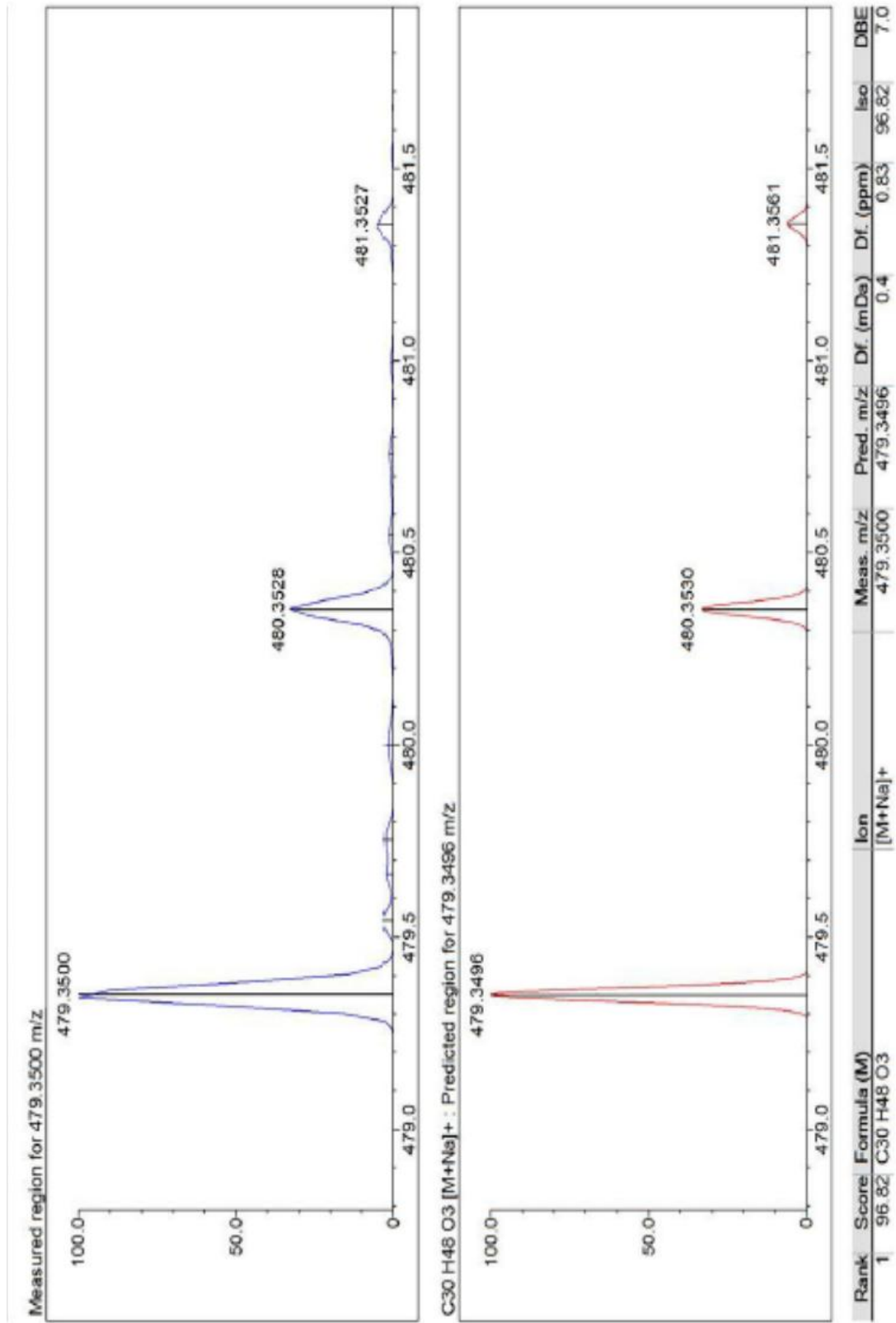
Şekil 83. Ursolik asit bileşiğinin LC-MS-IT-TOF kromatogramı
