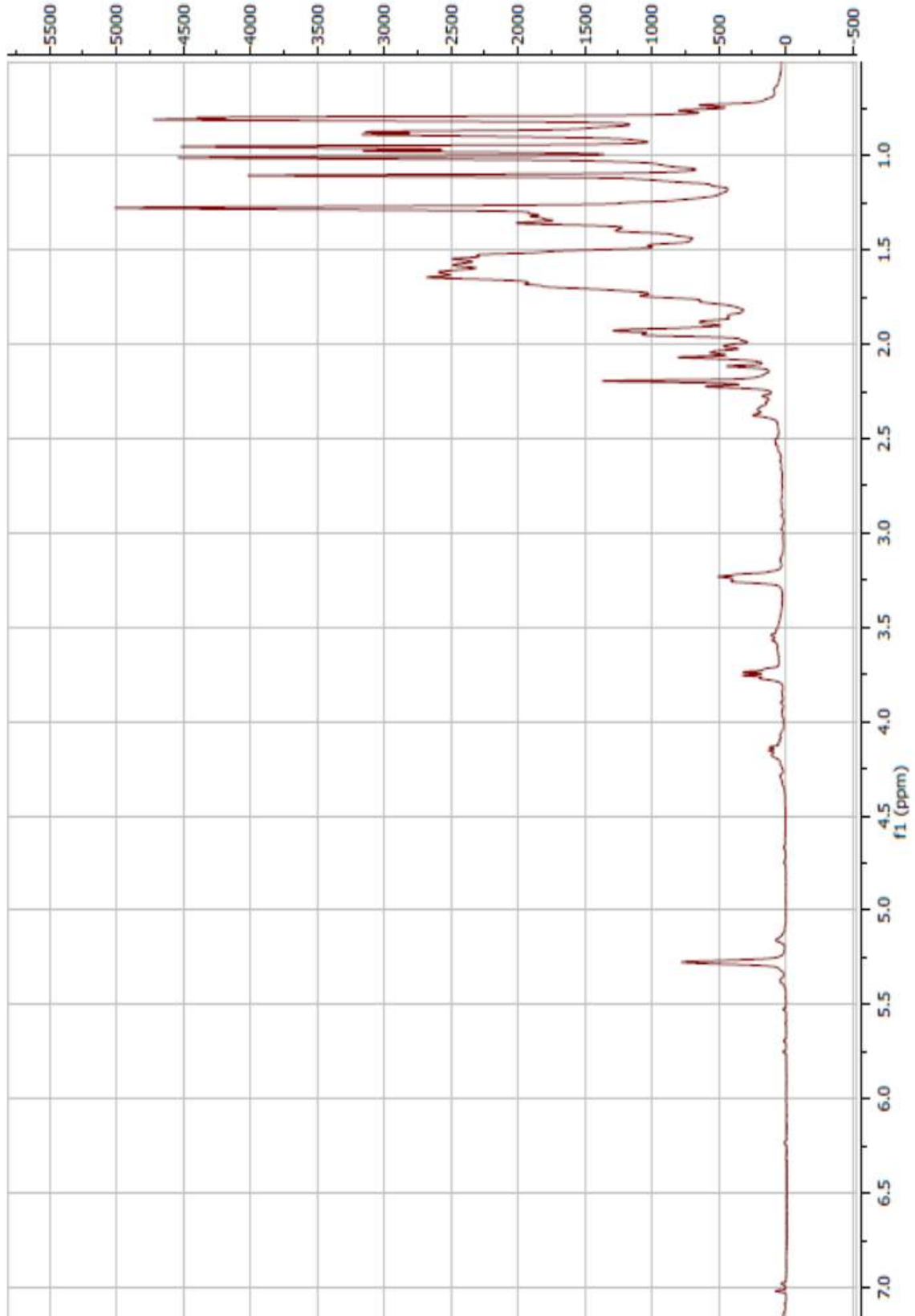
Şekil 81. Ursolik asit bileşiğinin ^1\text{H} -NMR Spektrumu ( \text{CDCl}_3 , 600 MHz)
