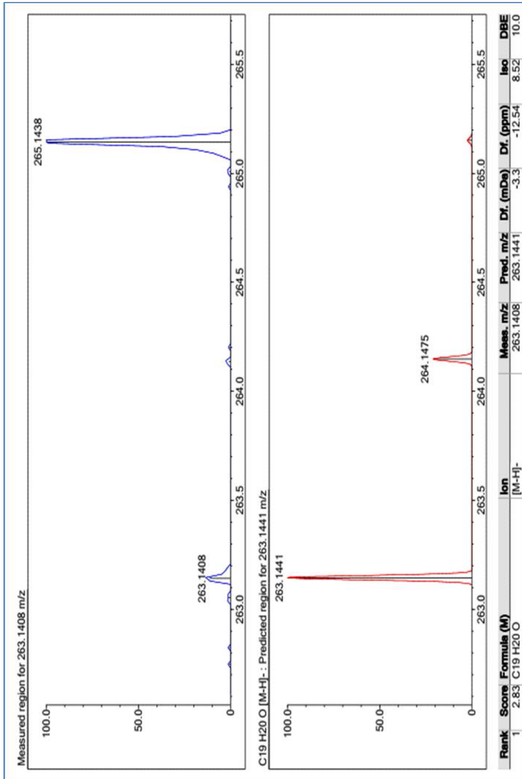
Şekil 126. 12-Hidroksi abieta 1,3,5(10), 8, 11, 13-hekzaen Bileşiğinin LC-MS-IT-TOF kromatogramı
