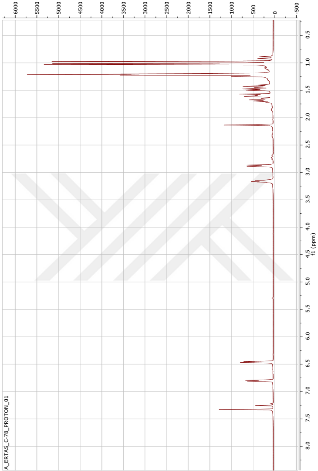
Şekil 72. 6,7-Dehydroroyleanon bileşiğinin 1 H NMR spektrumu (CDCl 3 , 600 MHz)
