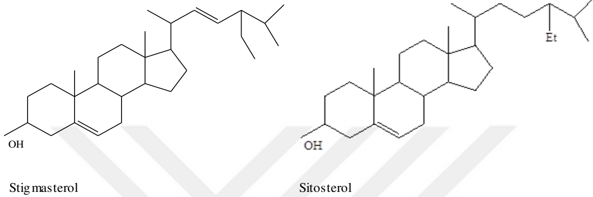
Şekil 11.Triterpen Örnekleri
