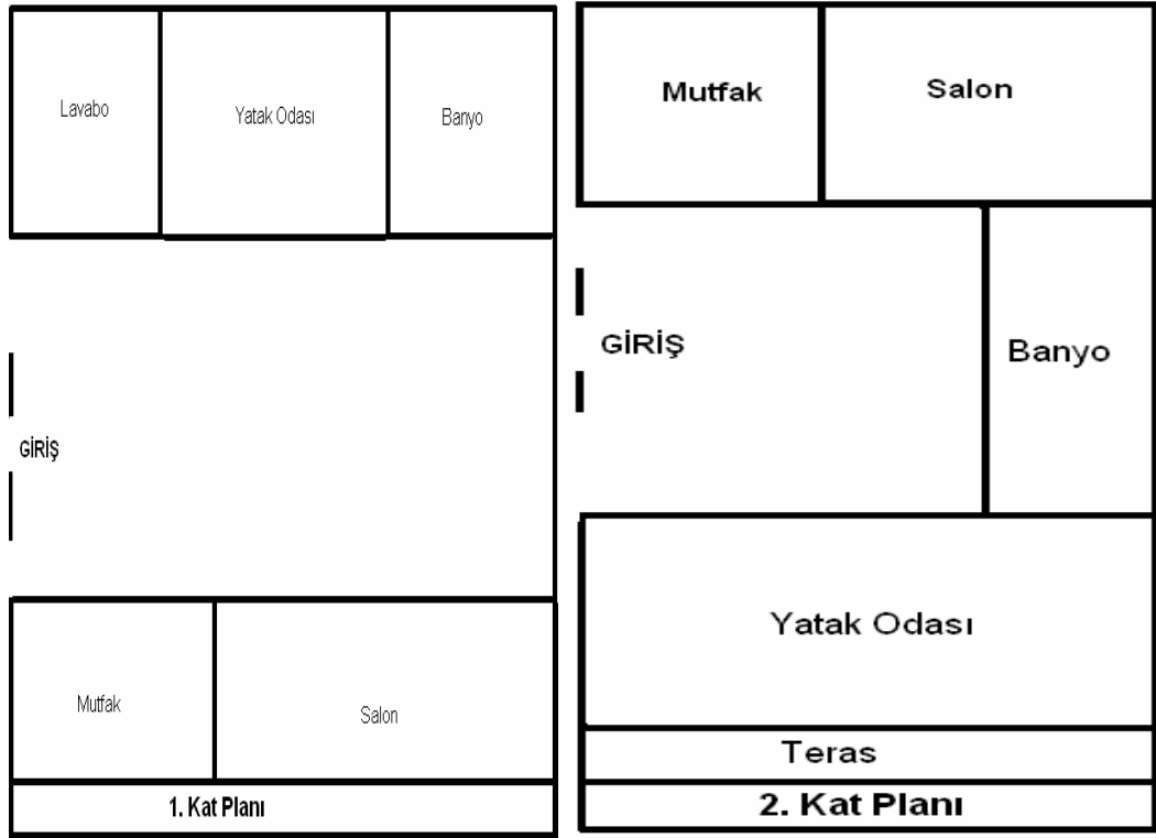
Şekil 2. Uluğbey kasabasındaki iki katlı bir evin planı (Ölçeksiz).
