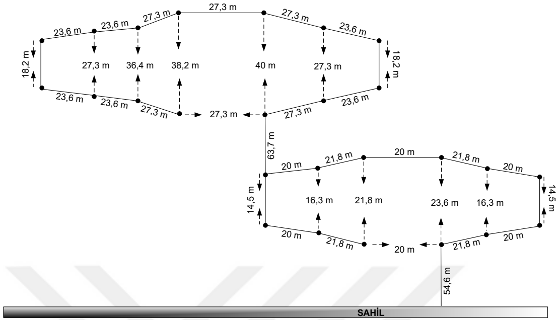
Şekil 3.2: Beykoz Dalı'nın teknik çizimi.
