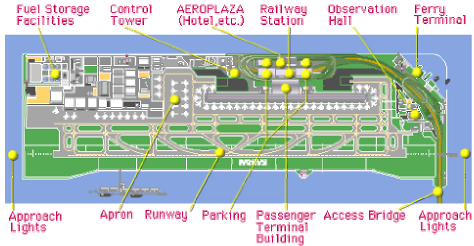
“Şekil 4. 28” Kansai havaalanı planı.
