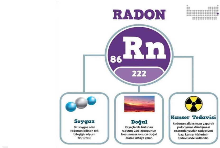
Şekil 1.1. Radon elementi ve özellikleri [bilimgenc.tubitak.gov.tr].
