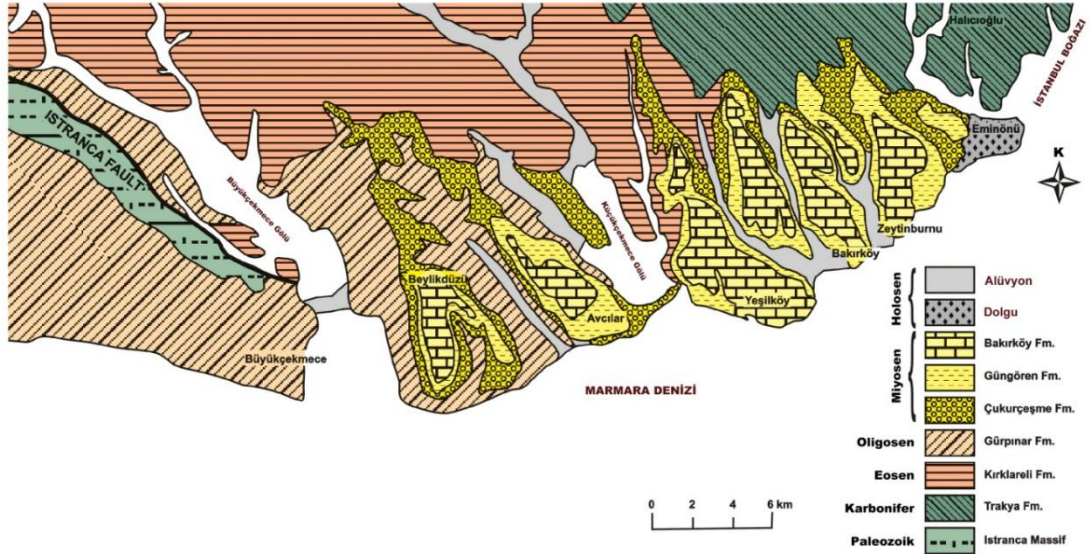
Şekil 2.2. İstanbul'un Avrupa yakasının genel jeoloji haritası (Arıç, 1955; Yalçınlar, 1976; Oktay ve Eren, 1999; Dalgıç, 2004; Dalgıç vd. 2009) [43-48].
