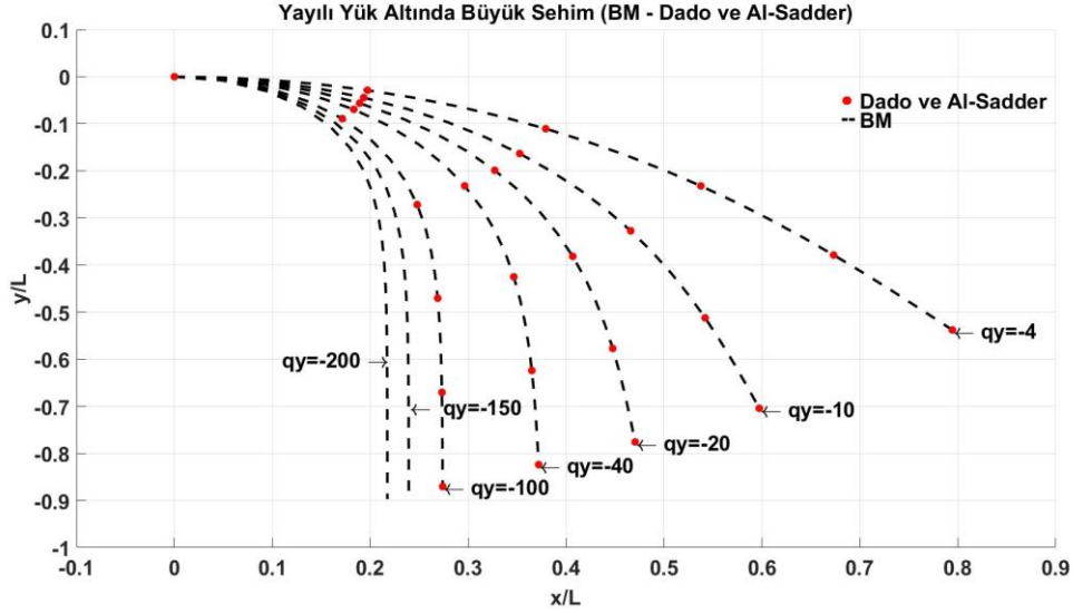
Şekil 3.6 Problem 1'in BM Çözümü ile Elde Edilen Büyük Sehim Diyagramları.
