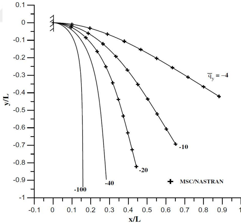
Şekil 3.7 Dado ve Al-Sadder (2005) Tarafından Gerçekleştirilen Çalışmanın Problem 1 Sonuçları (Dado and Al-Sadder, 2005).
