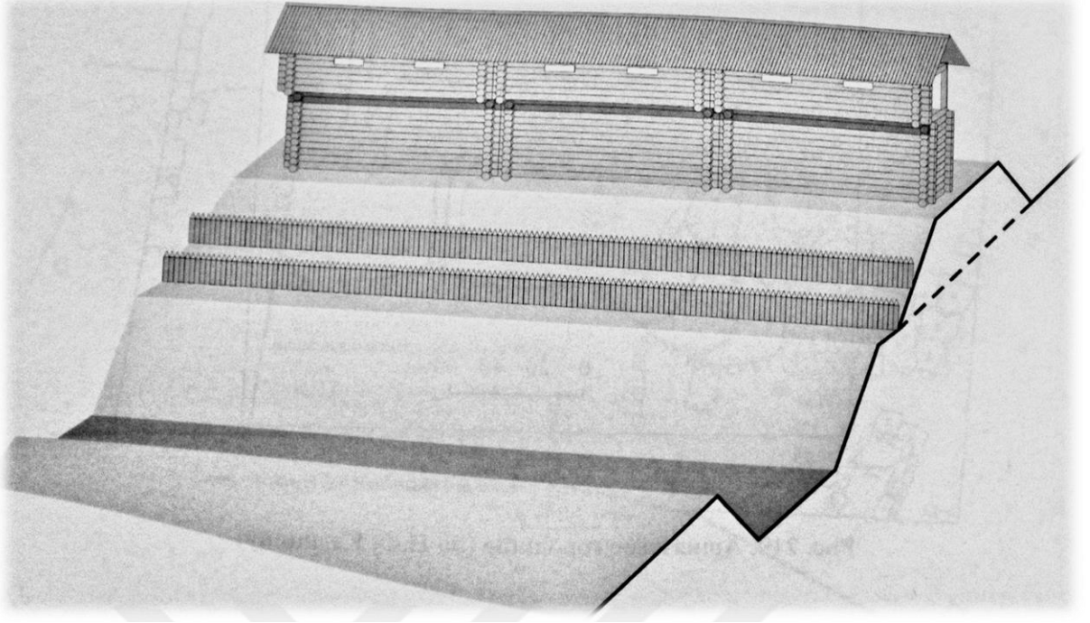
Levha 20. Kaşan Tahkimat Rekonstrüksiyonu
