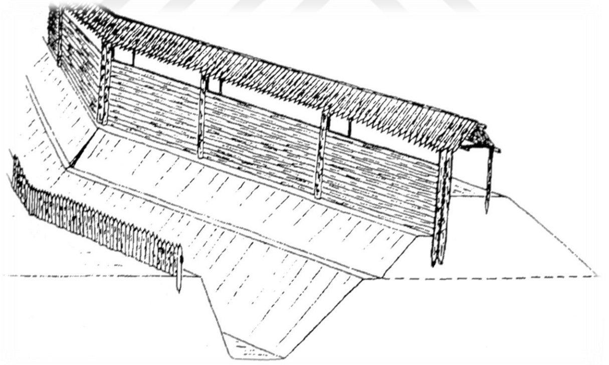
Levha 68. a. Bulgar kenti tahkimat rekonstrüksiyonu
