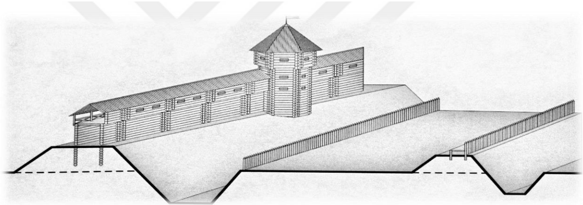
Levha 13.a. Suvar Tahkimat Rekonstrüksiyonu
