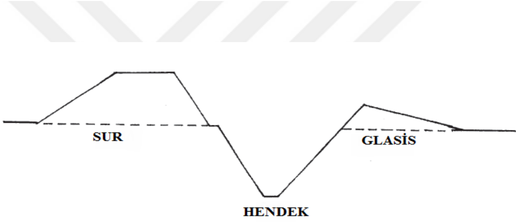
Levha 64. a. Glasis sistemi
