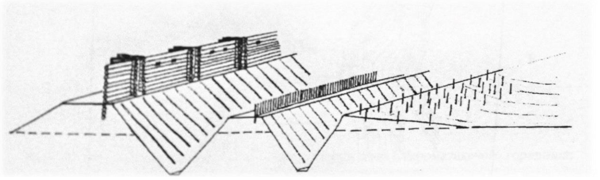
Levha 30. Şerben I Tahkimat Rekonstrüksiyonu
