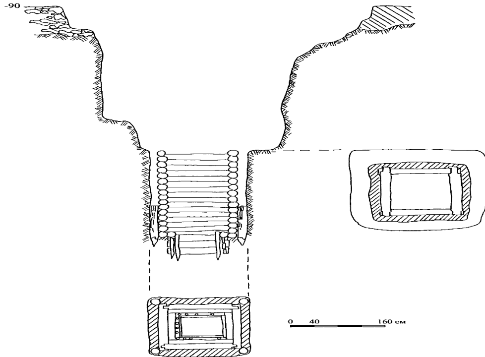
Levha 49. a. Biler Su Kuyuları
