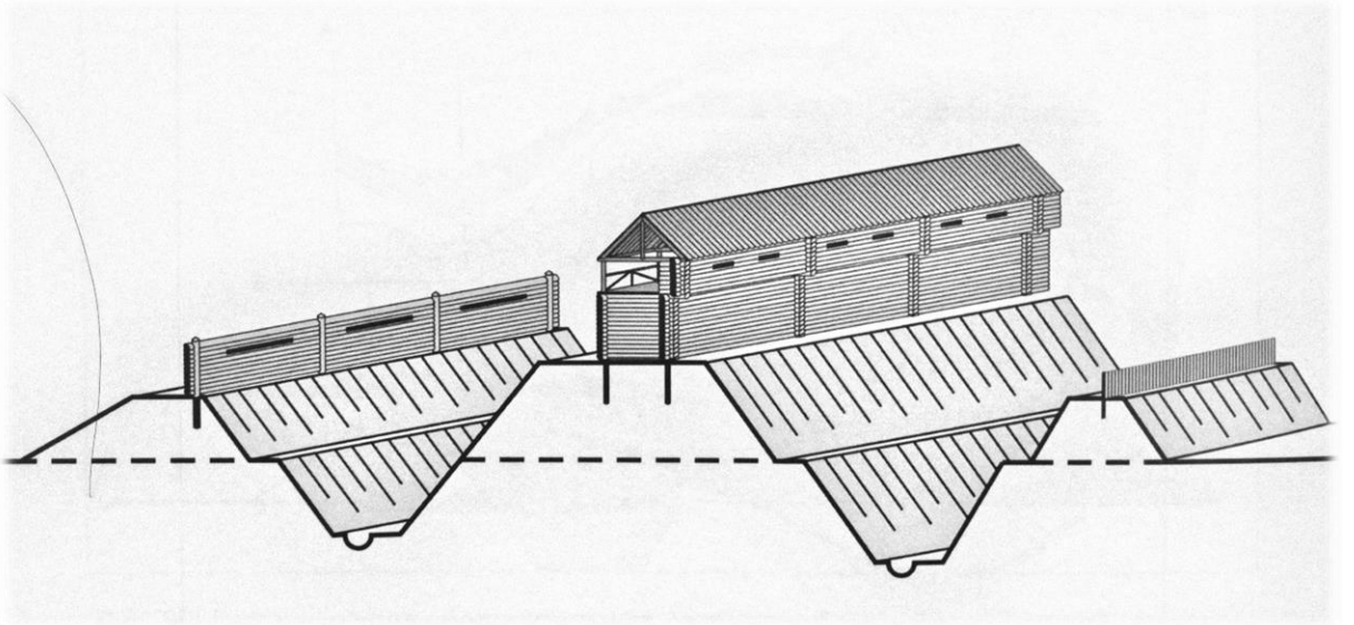
Levha 17. a. Cuketau Tahkimat Sistemi Rekonstrüksiyonu
