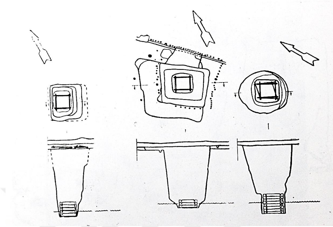
Levha 49. Biler Su Kuyuları
