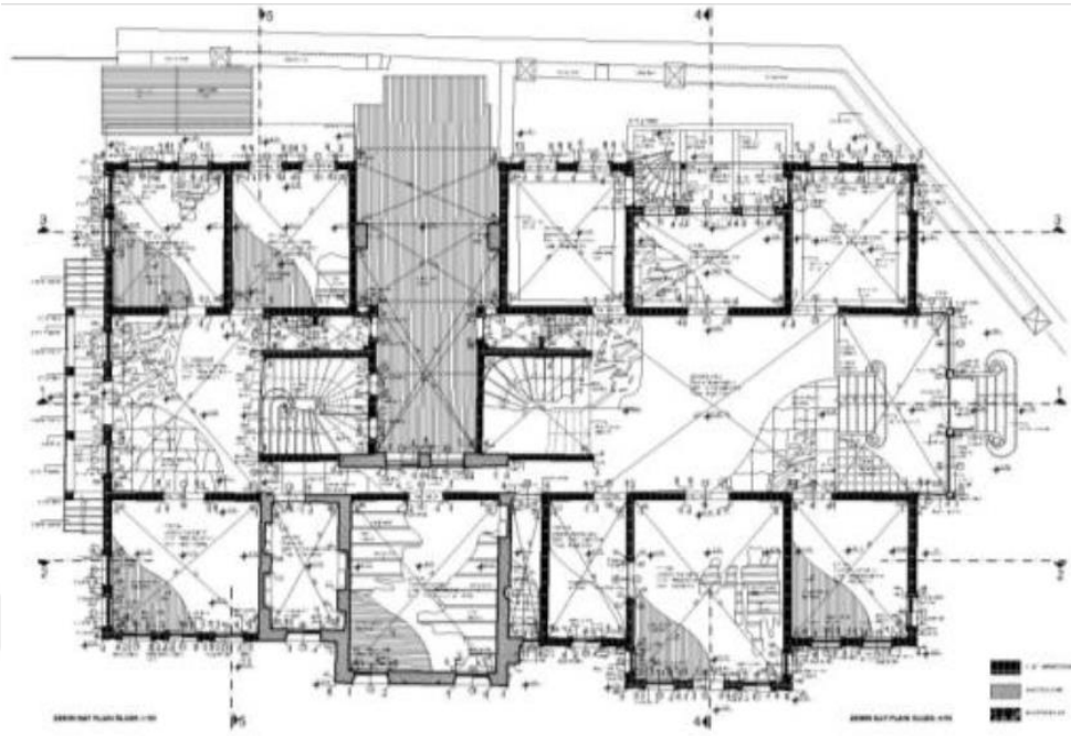
Şekil 7: Zemin Kat Döşeme Planı 170
