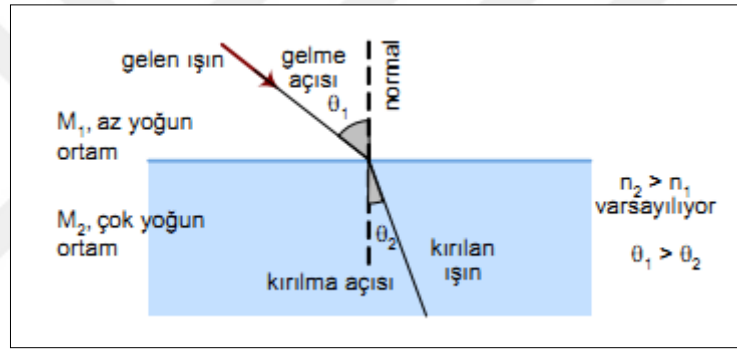
Şekil 3.3. Işığın kırılması [33].
