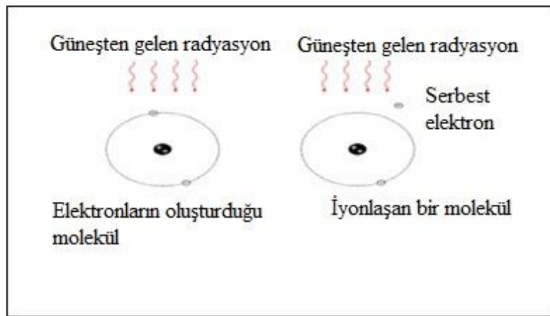
Şekil 2.2. İyonkürede iyonlaşma [17].
