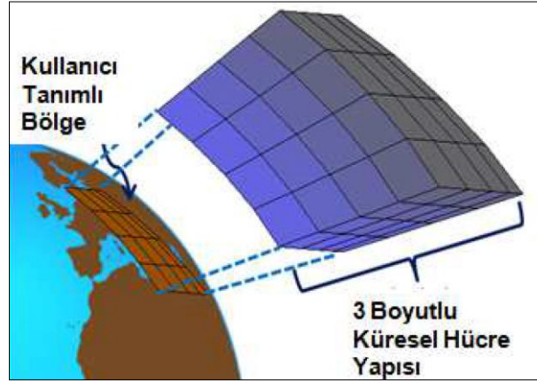
Şekil 3.7. İlgi alanı bölge üzerinde 3 boyutlu küresel ızgara modelinin gösterimi [4].
