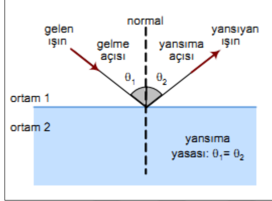
Şekil 3.5. Işın Yansıması [33].
