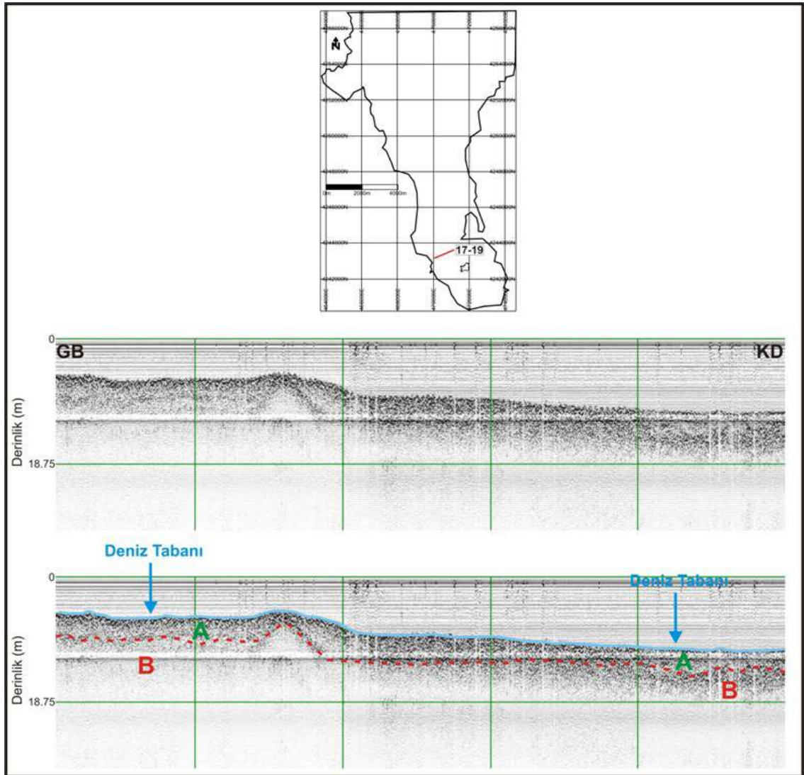
Şekil 5.32 17-19 nolu hat
