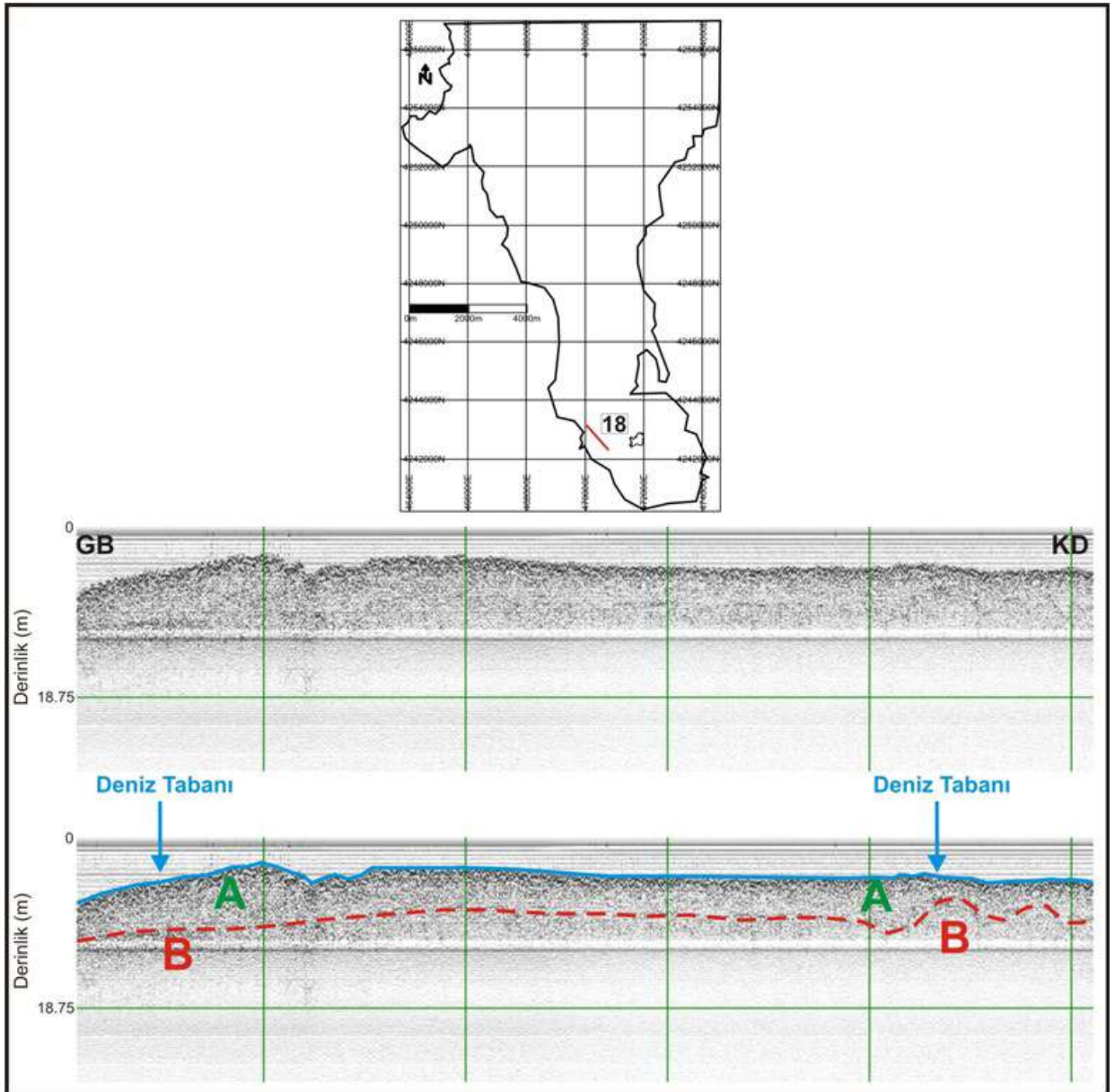
Şekil 5.33 18 nolu hat
