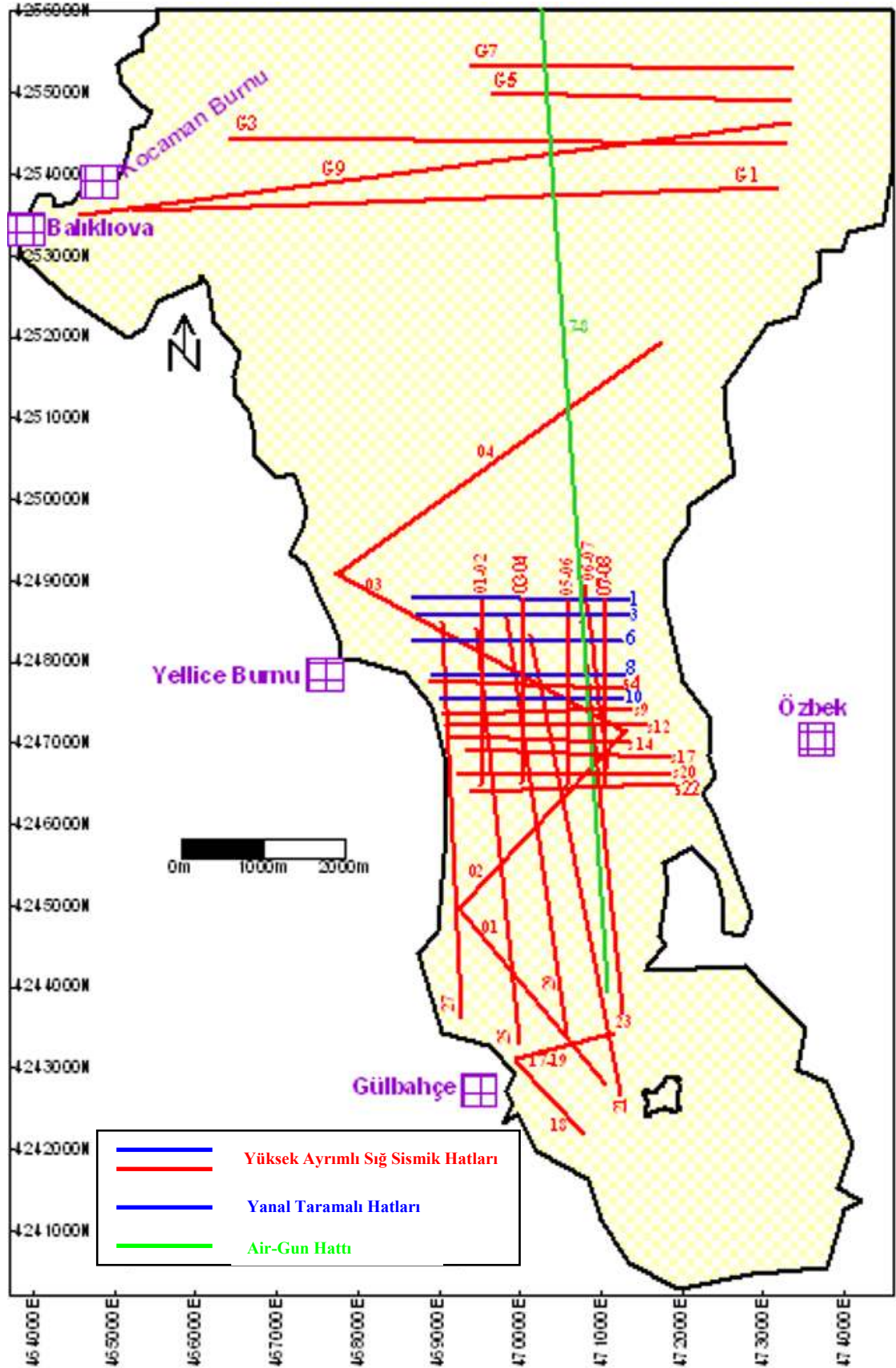
Şekil 5.11 Gulbahce Körfezinde yapılan batimetri, yüksek ayrımlı sığ sismik (3,5 kHz) ve yanıl taramalı sonar çalışmalarında koşulan hatları gösteren veri haritası
