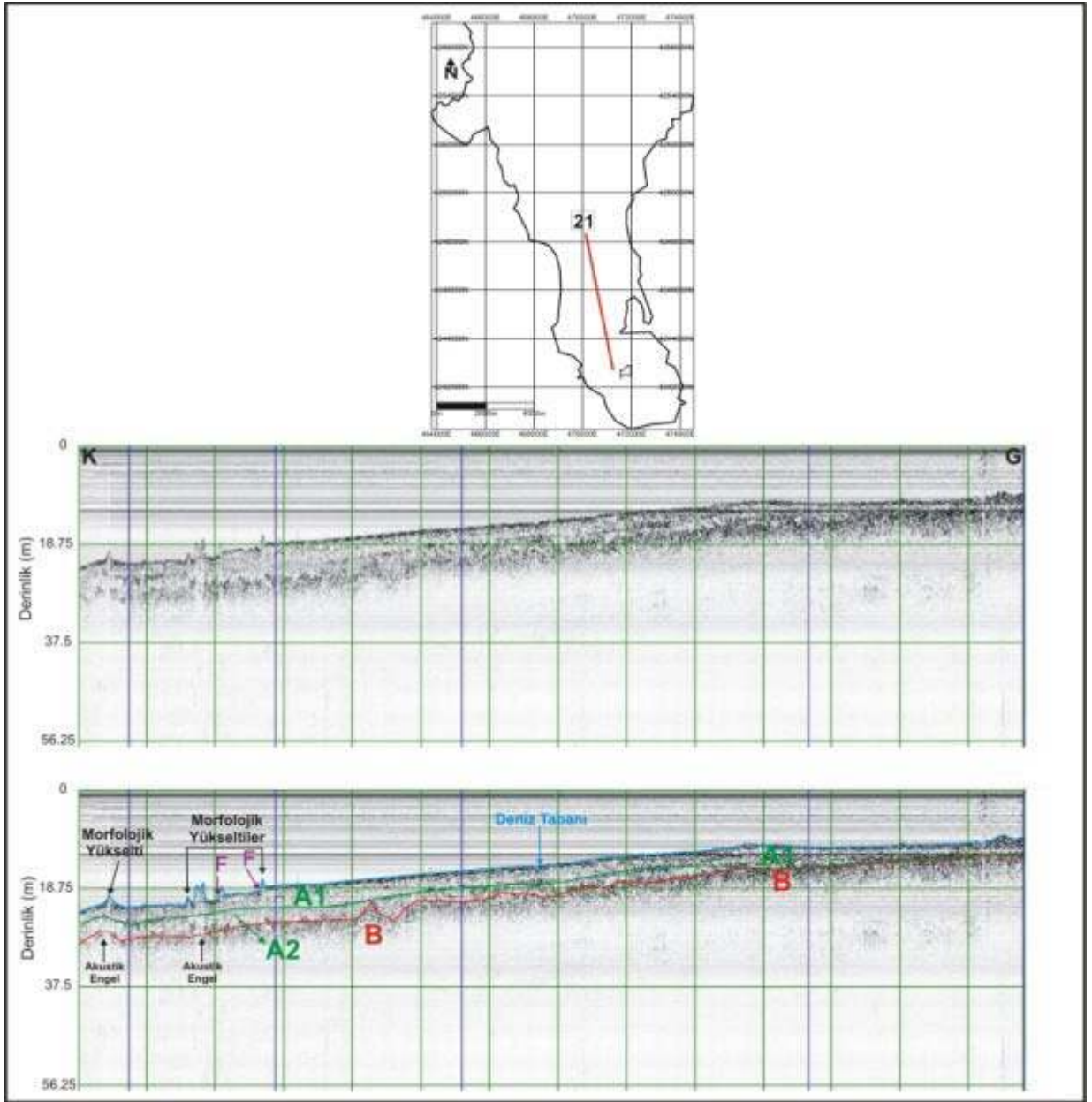
Şekil 5.29 21 nolu hat
