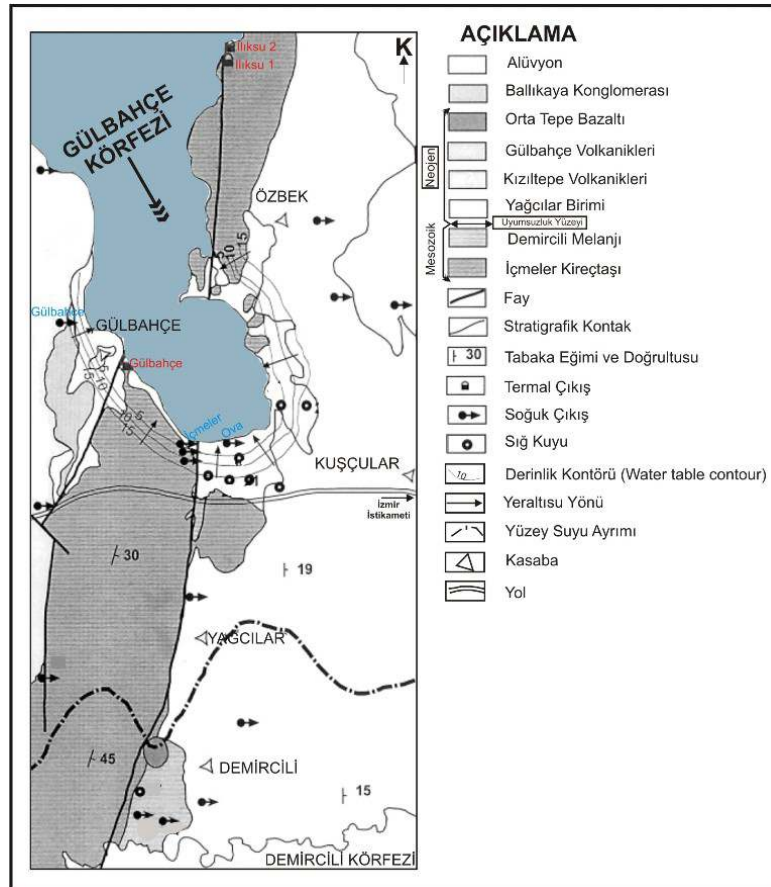
Şekil 5.2 Gülbahçe Körfezi jeoloji haritası (Tarcan, 2001)
