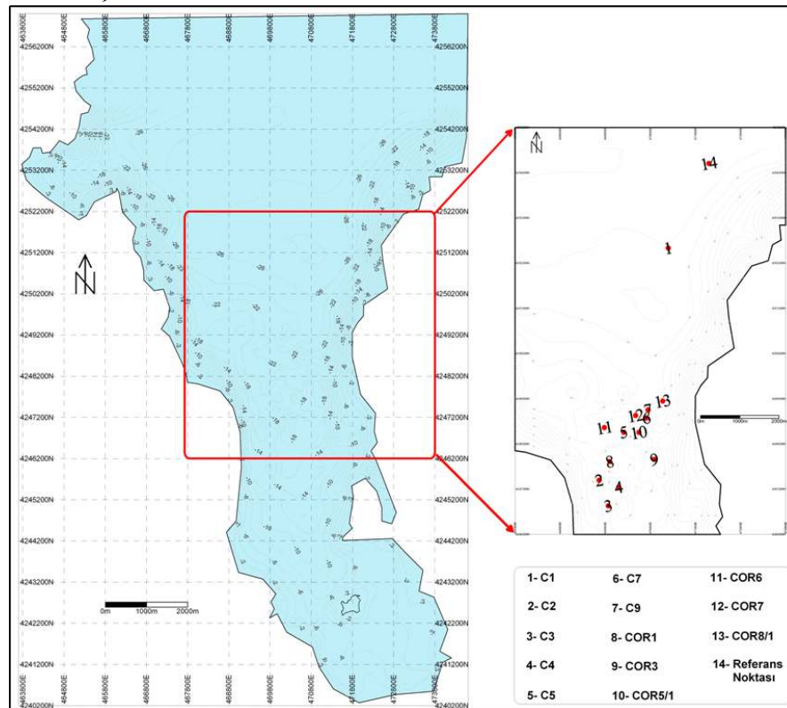
Şekil 5.47 Gravite önekleyicisiyle alınan deniz tabanı örnek lokasyonları
