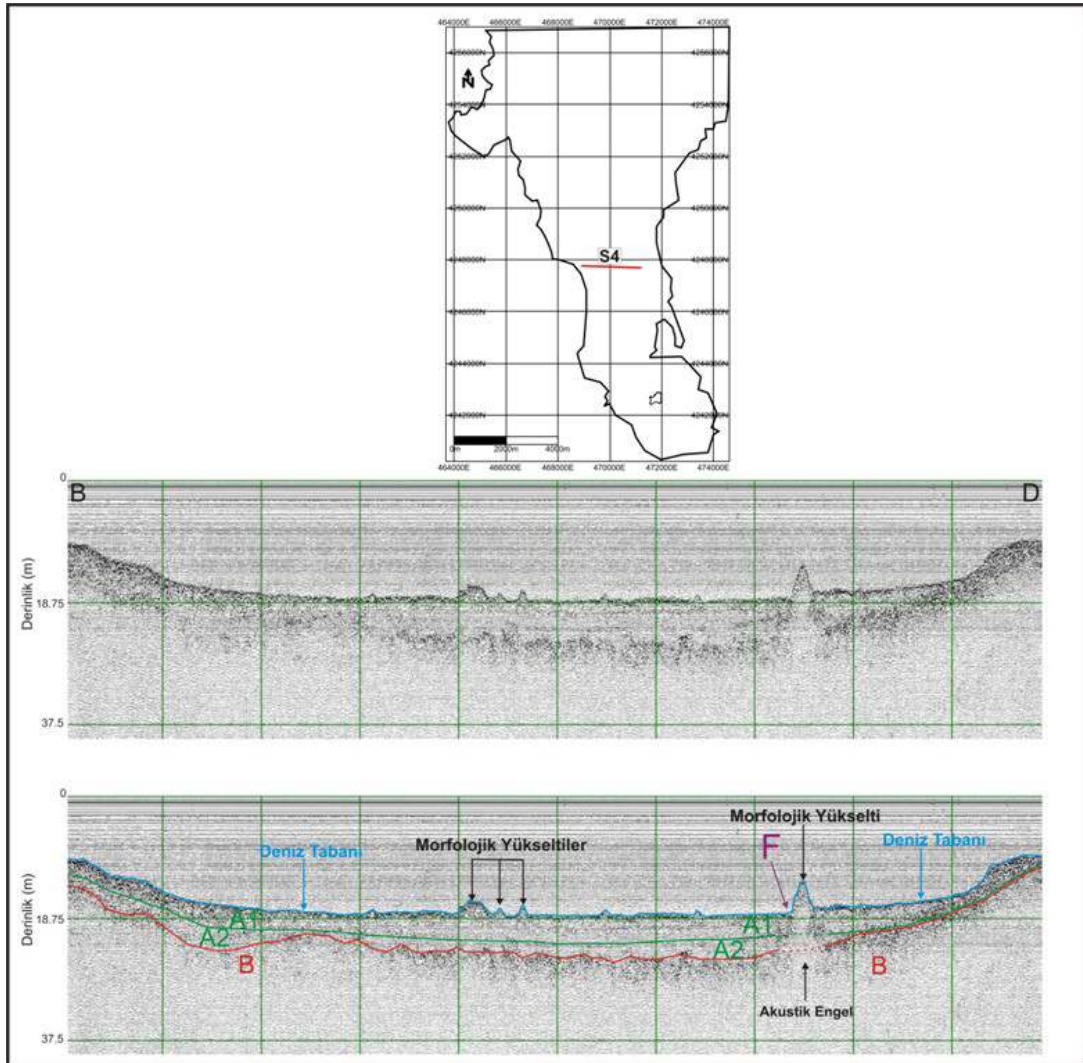
Şekil 5.37 S4 nolu hat
