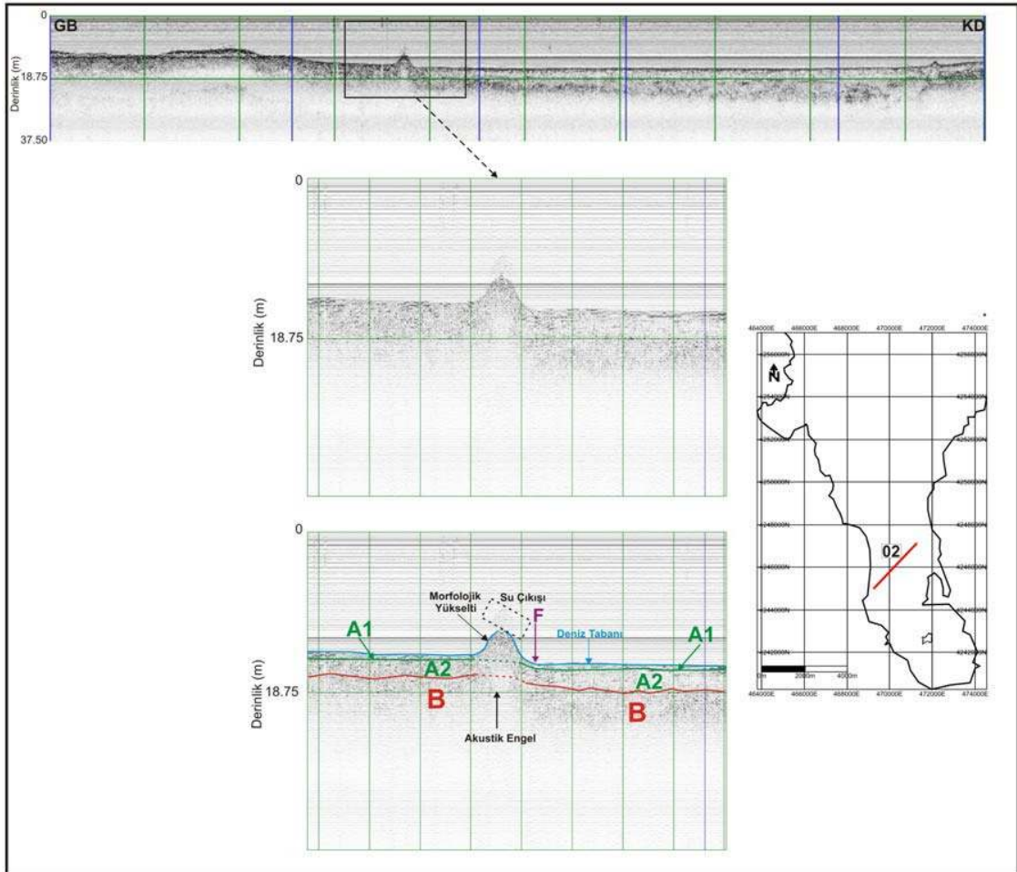
Şekil 5.18 02 nolu hat
