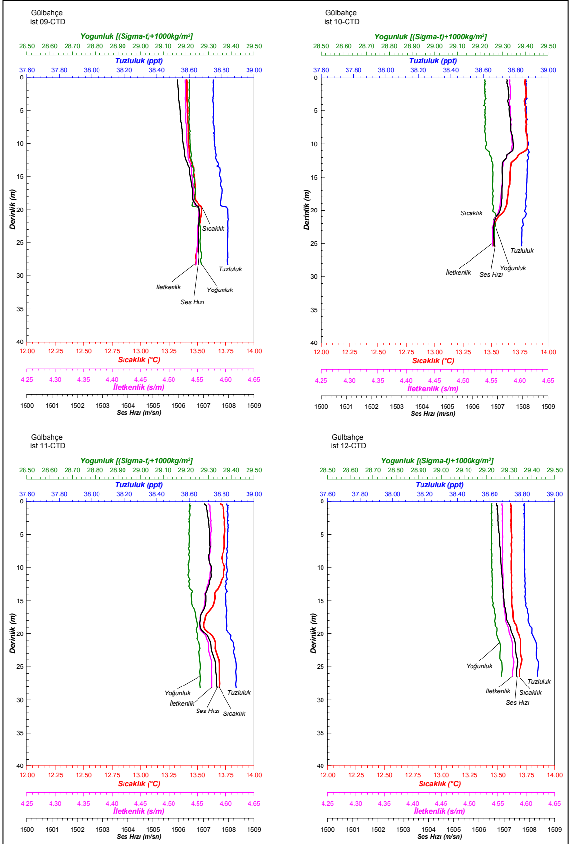
Şekil 5.65 devam ediyor
