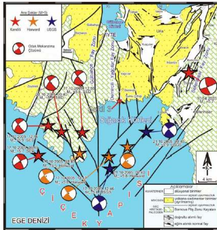
Şekil 5.44 Ekim-2005 ve Nisan-2003 depremlerinin ana şoklarını ve bu depremlere neden olan diri fayları gösteren jeoloji haritası. Değişik doğrultulardaki faylar Sığacık körfezinde birleşerek doğrultu atımlı faylara özgü çiçek yapısını oluşturmaktadır. Deprem verileri KOERI, USGS, Harward ve SED'den alınmıştır. Karada haritalanan fayların denizdeki uzanımları Ocakoğlu ve diğer., (2004, 2005)'nin sismik kesitlerinden yararlanılarak yeniden çizilmiştir. IYTE: İzmir Yüksek Teknoloji Enstitüsü (Sözbilir ve diğer., 2009).
