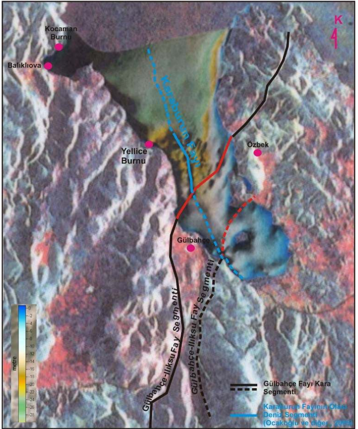
Şekil 5.46 Gulbahce Körfezindeki aktif fayların yüzey etkisinin üç boyutlu görünümü
