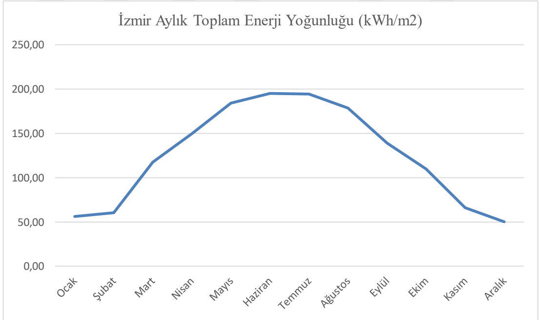
Şekil 3.5: İzmir İli Aylık Toplam Enerji Yoğunluğu
