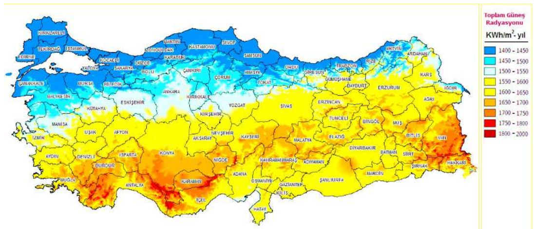
Şekil 2.1: Türkiye'nin Toplam Güneş Işıtım Miktarları ( kWh/m 2 -yıl)[36]
