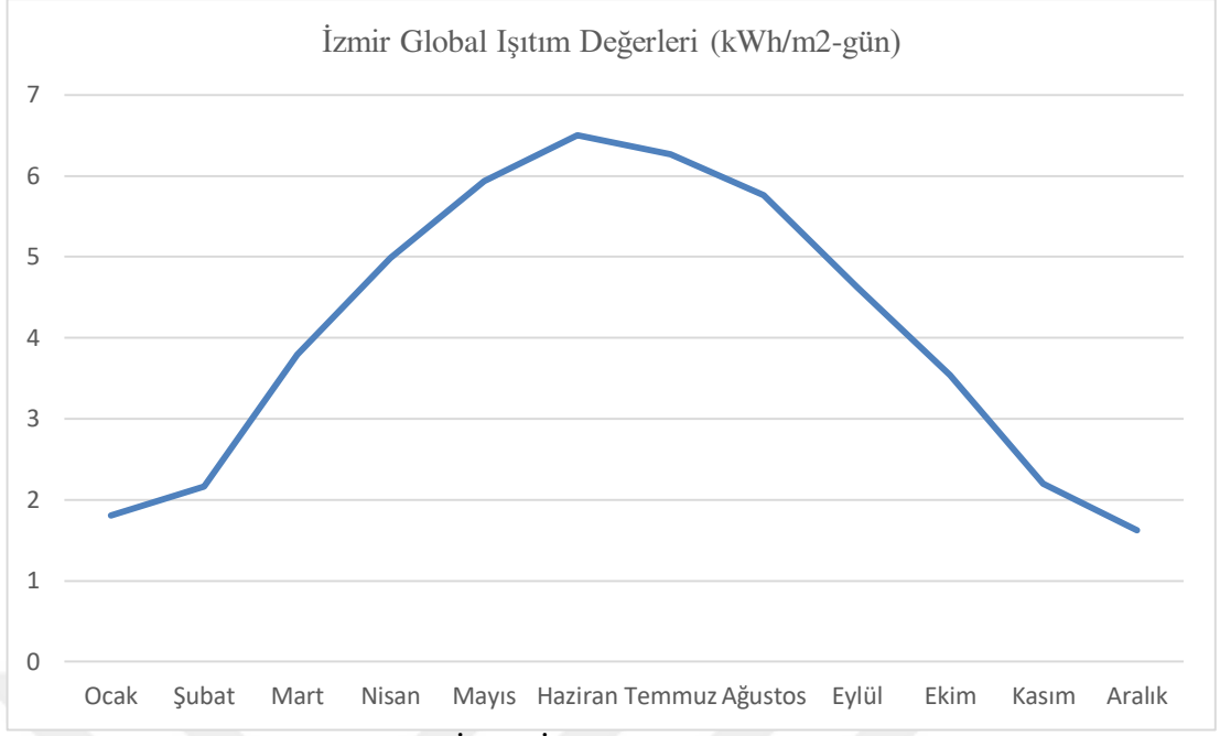
Şekil 3.4: İzmir İli Global Işıtım Değerleri
