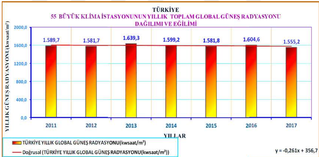
Şekil 2.5: Yıllık Ortalama Güneş Isıtım Verisinin 2011-2017 Yılları Arasında Dağılımı ve Eğilimi[43]
