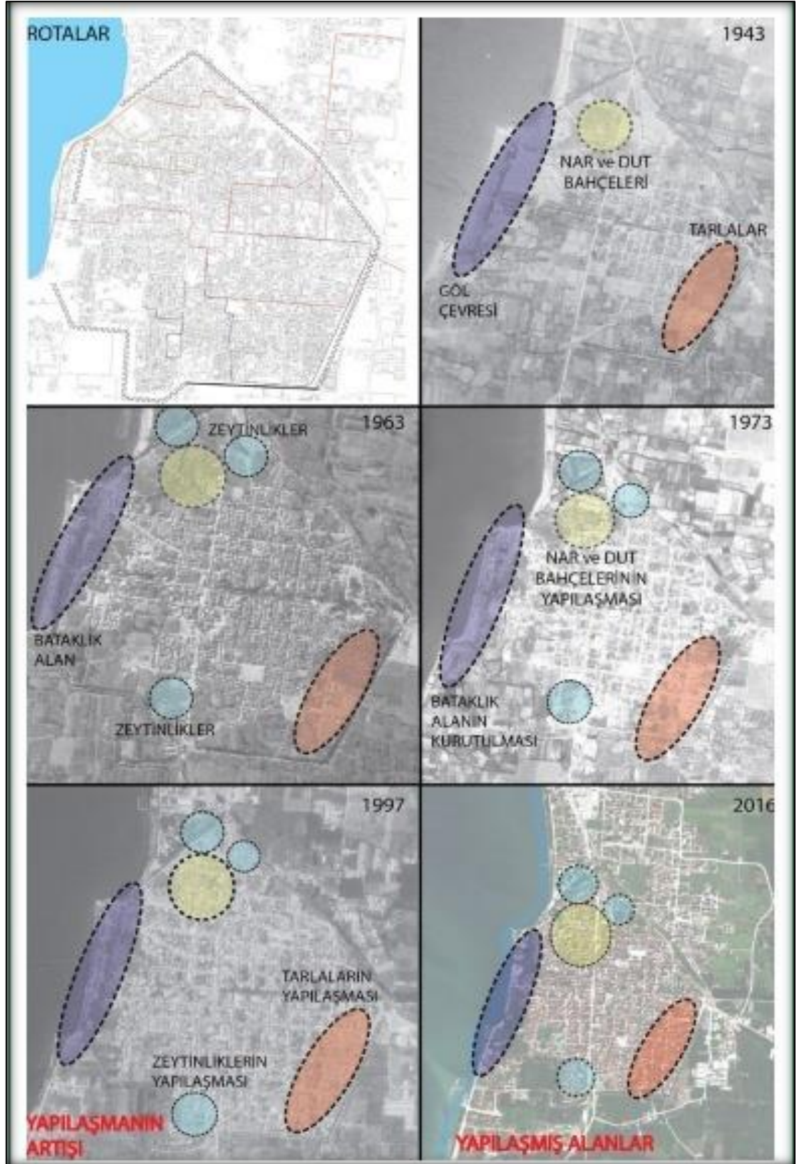
Şekil 6. 5. Çalışma Sahası Doğal Çevre Değişimleri
