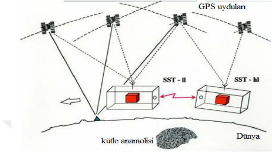
Şekil 4.2 SST-II ölçme tekniği (Rummel vd. 2002).
