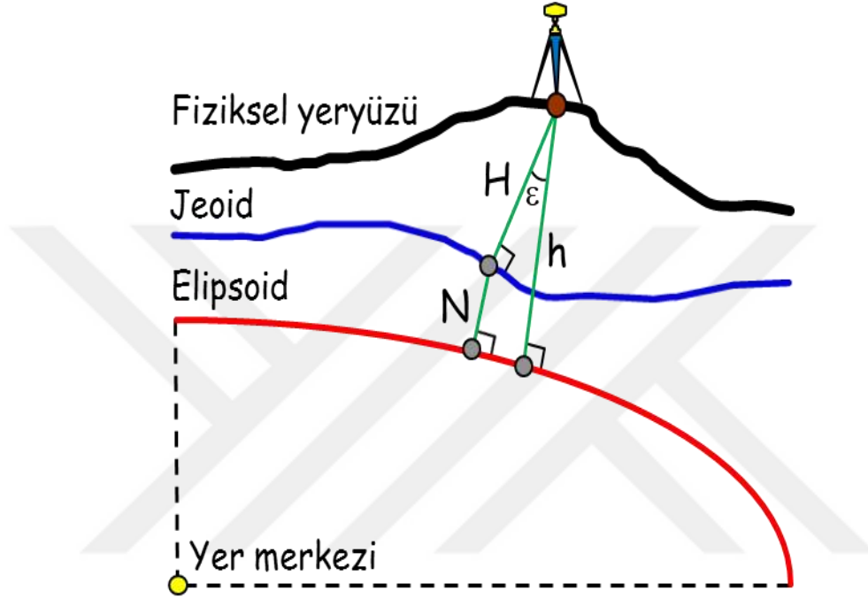
Şekil 2.4 Jeoid, elipsoid ve ortometrik yükseklik.
