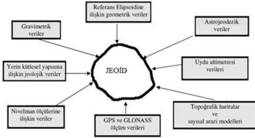
Şekil 2.2 Jeoid belirlemede kullanılan veri kaynakları (Akçın 2001).
