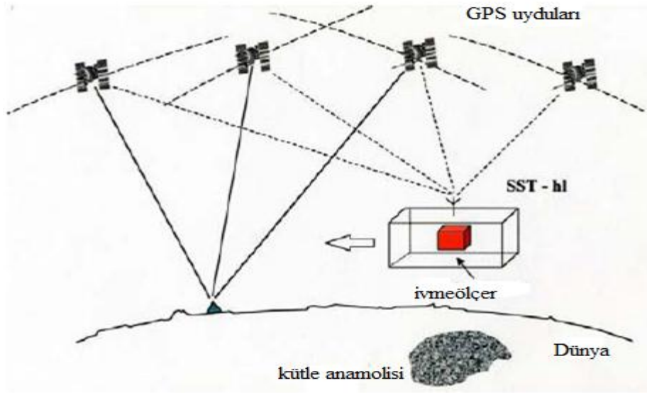
Őekil 4.1 SST-hI lme tekniđi (Rummel vd. 2002).
