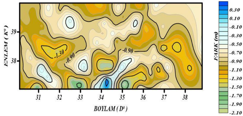
Şekil 5.12 GO_CONS_GCF_2_SPW_R4 modeline ait fark haritası.
