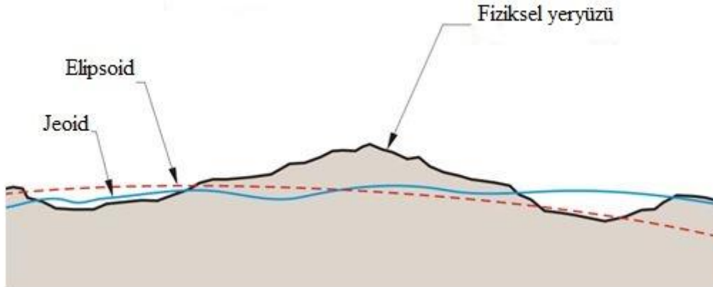
Şekil 2.1 Jeoid yüzeyi.
