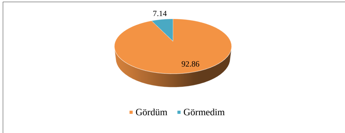
Şekil 35. Silisleşmiş ağacın görülme durumuna ilişkin yüzdeler
