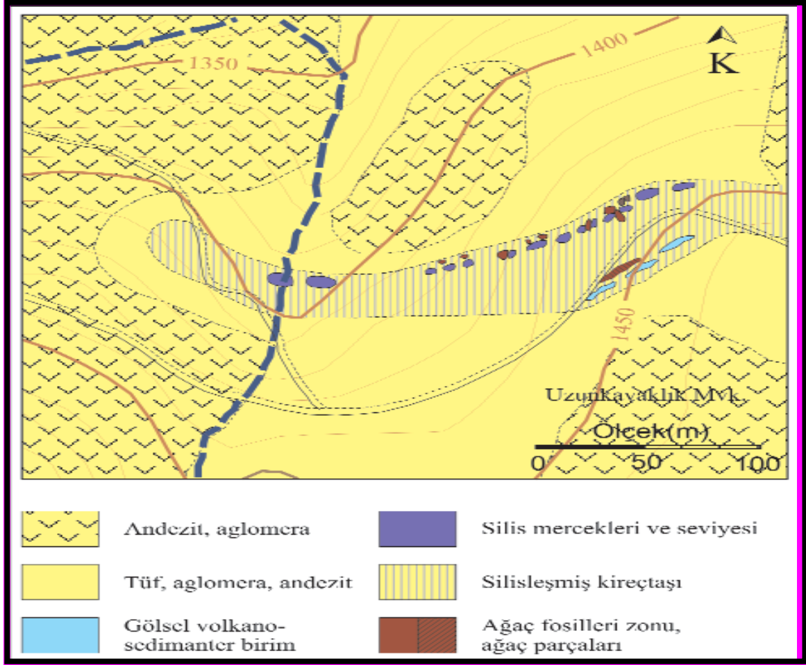
Şekil 5. Silisleşmiş ağaçların yayılış gösterdiği alanın jeoloji haritası ve fosilleşmiş ağaçların sahadaki dağılışı (Kaynak: https://www.jemirko.org.tr/download/soguksu-milli-parki-ve-cevresindeki-jeositleri/?wpdmdl=478 sayfasından erişilmiştir).
