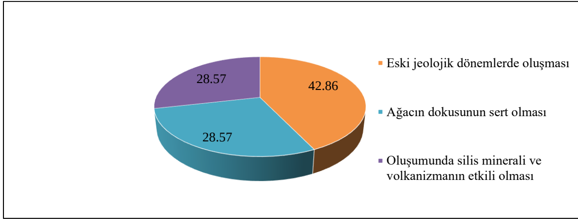
Şekil 36. Silisleşmiş ağaçların oluşumu ile ilgili dikkat çeken özelliklere ilişkin yüzdelik grafik
