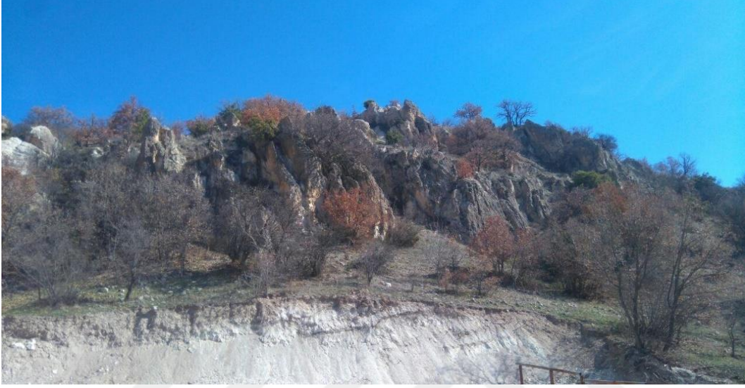
Şekil 20. Abacı peribacaları (Fotoğraf: Merve Ereli, 2017).
