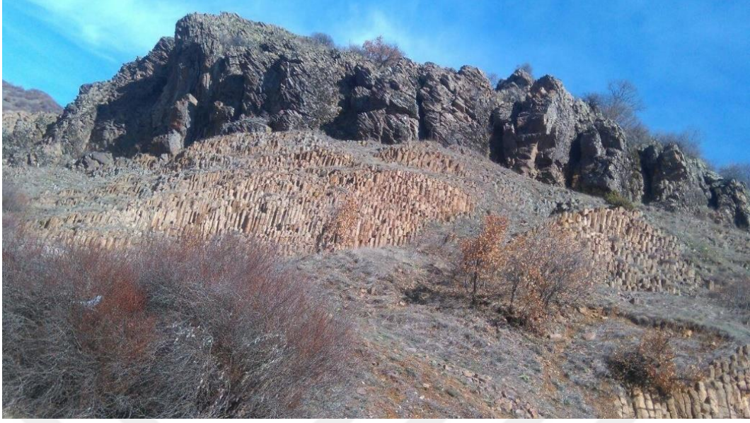
Şekil 9. Bazalt sütunlarından bir görünüm (Fotoğraf: Merve Ereli, 2017).
