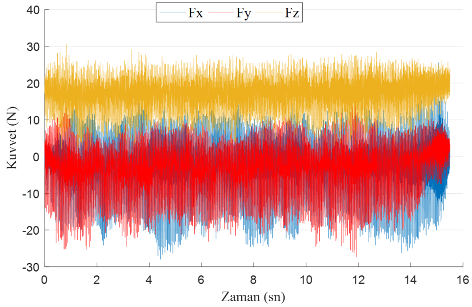
Şekil 24. Kompozit malzeme: JFT, Kesici takım: WC, Dönme devri: 5000 dev/dak ve İlerleme: 0,02 mm/dev
