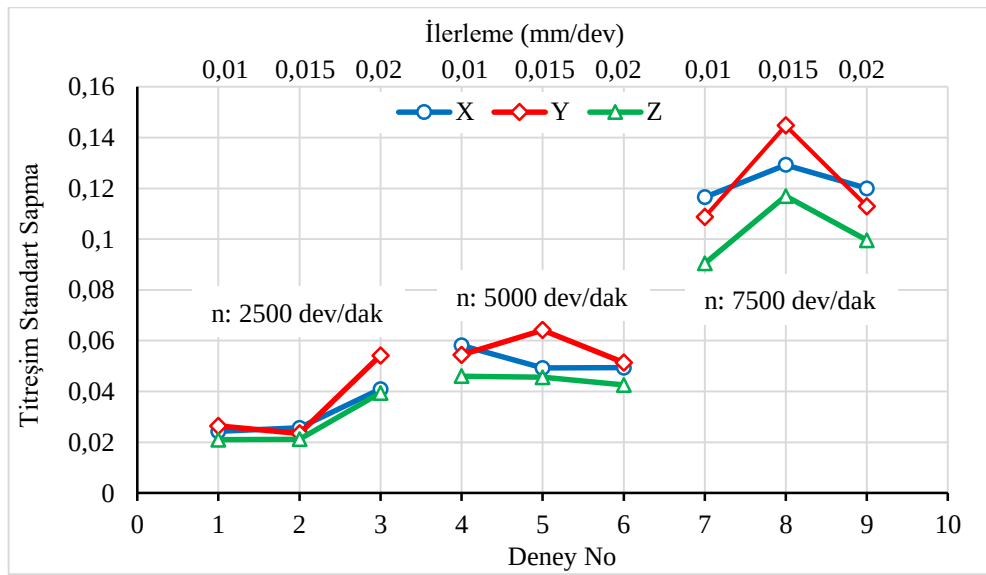
Şekil 4.16. JFTP kompozit malzemenin HSS parmak freze \dot{\text{c}}\text{a}}\text{k}\text{ı}\text{s}\text{ı} ile frezelenmesinde elde edilen titreşim standart sapma grafiği
