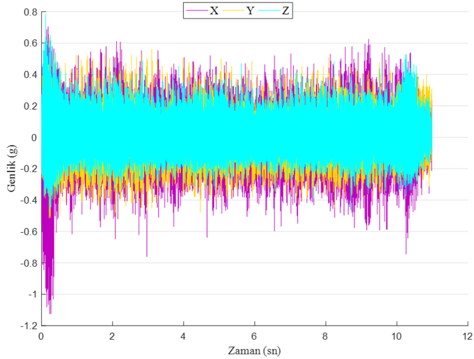
Şekil 54. Kompozit malzeme: KFT, Kesici takım: WC, Dönme devri: 7500 dev/dak ve İlerleme: 0,02 mm/dev
