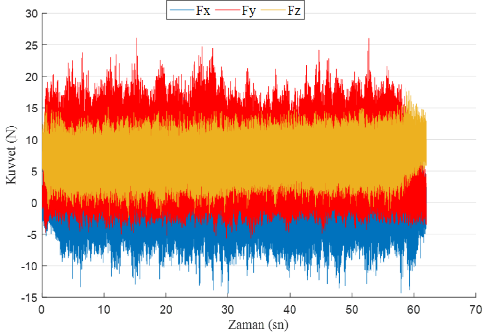
Şekil 46. Kompozit malzeme: KFT, Kesici takım: WC, Dönme devri: 2500 dev/dak ve İlerleme: 0,01 mm/dev
