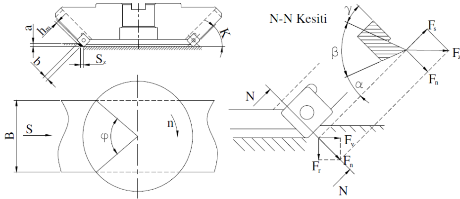
Şekil 1.6. Alın frezelemede açılar ve kesme kuvvetleri (Sarı, 2008)
