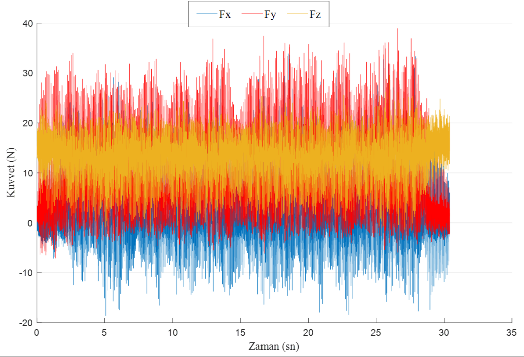
Şekil 21. Kompozit malzeme: JFT, Kesici takım: WC, Dönme devri: 2500 dev/dak ve İlerleme: 0,02 mm/dev
