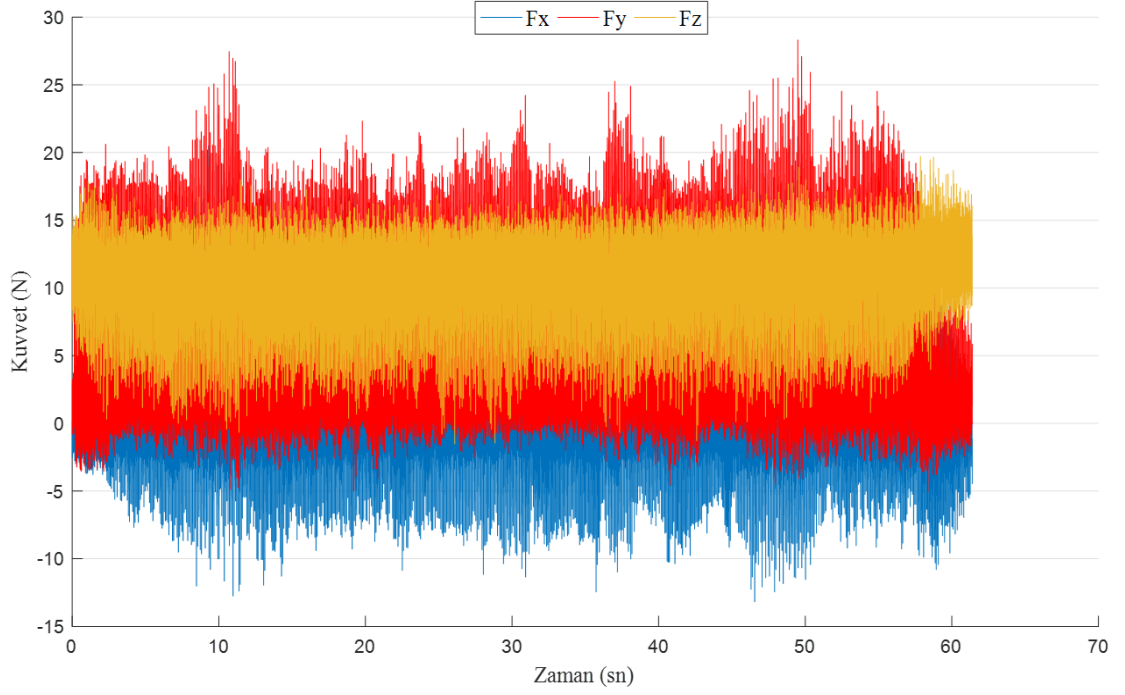
Şekil 19. Kompozit malzeme: JFT, Kesici takım: WC, Dönme devri: 2500 dev/dak ve İlerleme: 0,01 mm/dev
