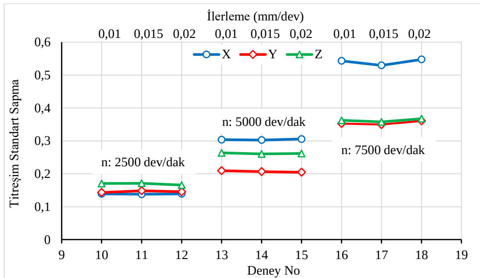
Şekil 4.20. KFTP kompozit malzemenin WC parmak freze akısı ile frezelenmesinde elde edilen titreşim standart sapma grafięi
