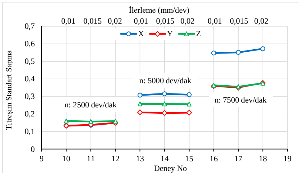
Şekil 4.17. JFTP kompozit malzemenin WC parmak freze çıkışı ile frezelenmesinde elde edilen titreşim standart sapma grafiği
