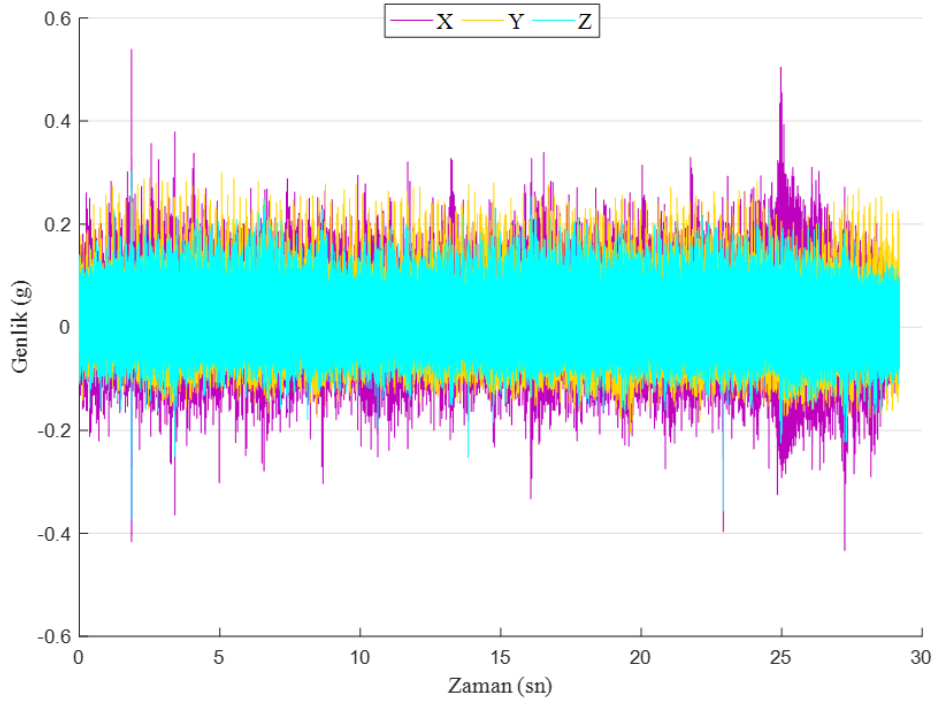
Şekil 49. Kompozit malzeme: KFT, Kesici takım: WC, Dönme devri: 5000 dev/dak ve İlerleme: 0,01 mm/dev
