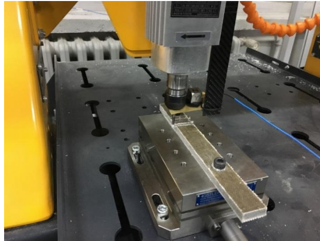
Şekil 3.15. Titreşim ölçüm cihaz aparatının görüntüsü
