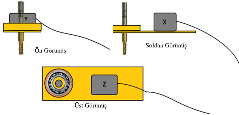
Şekil 3.14. Titreşim ölçüm aparatı için hazırlanan düzenek
