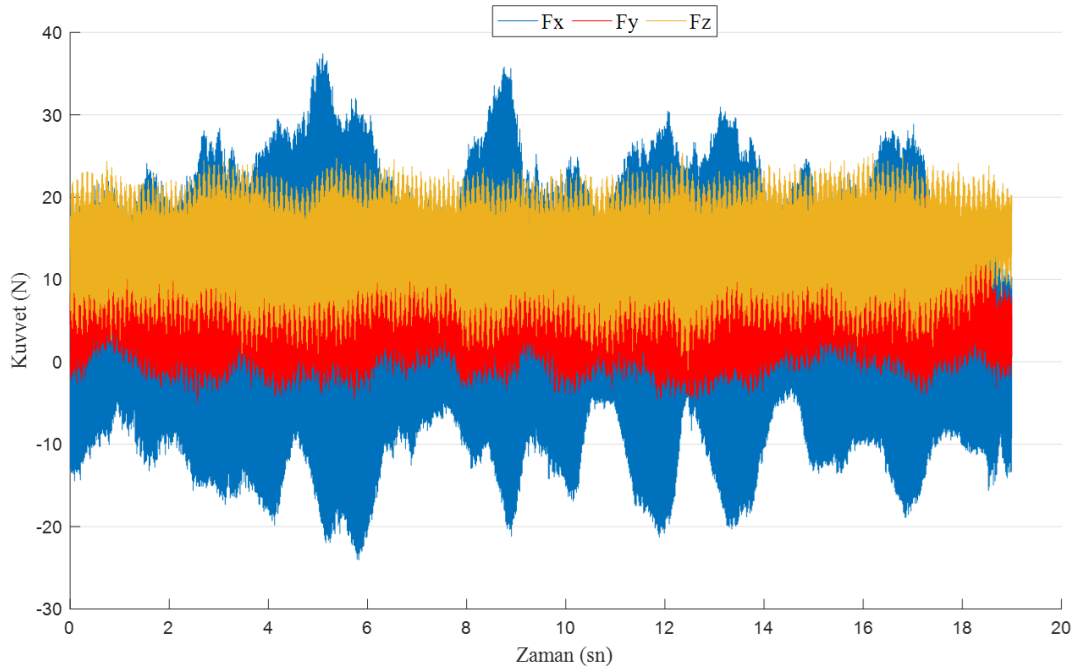
Şekil 16. Kompozit malzeme: JFT, Kesici takım: TiN Kaplı HSS, Dönme devri: 7500 dev/dak ve İlerleme: 0,01 mm/dev
