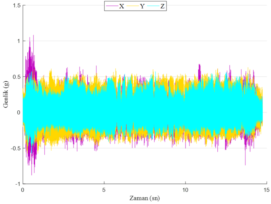
Şekil 53. Kompozit malzeme: KFT, Kesici takım: WC, Dönme devri: 7500 dev/dak ve İlerleme: 0,015 mm/dev
