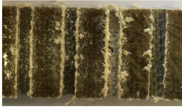
Şekil 4.26. KFTP kompozitin TiN kaplı HSS parmak freze çakısı ile frezelenmesinde oluşan deformasyon görüntüleri
