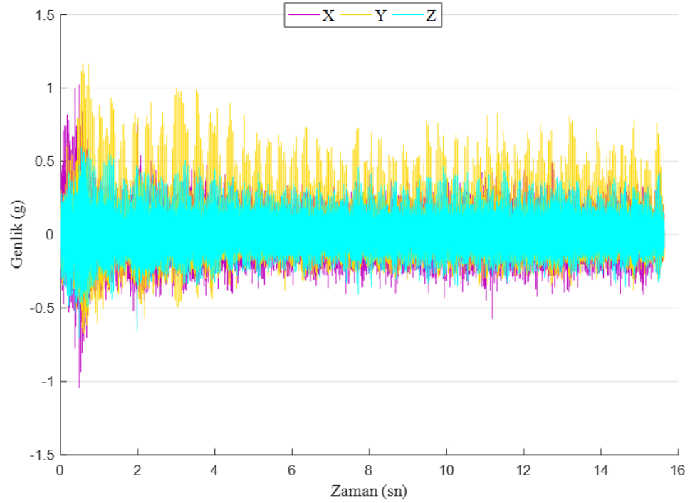
Şekil 42. Kompozit malzeme: KFT, Kesici takım: TiN Kaplı HSS, Dönme devri: 5000 dev/dak ve İlerleme: 0,02 mm/dev
