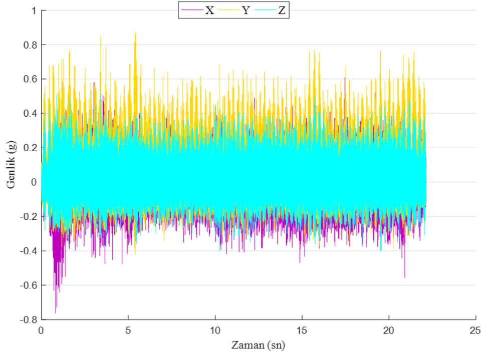
Şekil 41. Kompozit malzeme: KFT, Kesici takım: TiN Kaplı HSS, Dönme devri: 5000 dev/dak ve İlerleme: 0,015 mm/dev
