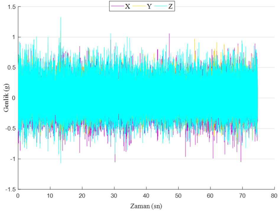
Şekil 19. Kompozit malzeme: JFT, Kesici takım: WC, Dönme devri: 2500 dev/dak ve İlerleme: 0,01 mm/dev
