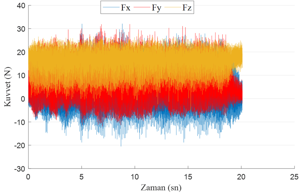
Şekil 23. Kompozit malzeme: JFT, Kesici takım: WC, Dönme devri: 5000 dev/dak ve İlerleme: 0,015 mm/dev
