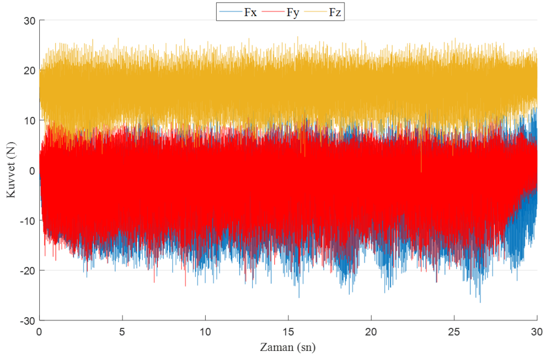
Şekil 22. Kompozit malzeme: JFT, Kesici takım: WC, Dönme devri: 5000 dev/dak ve İlerleme: 0,01 mm/dev
