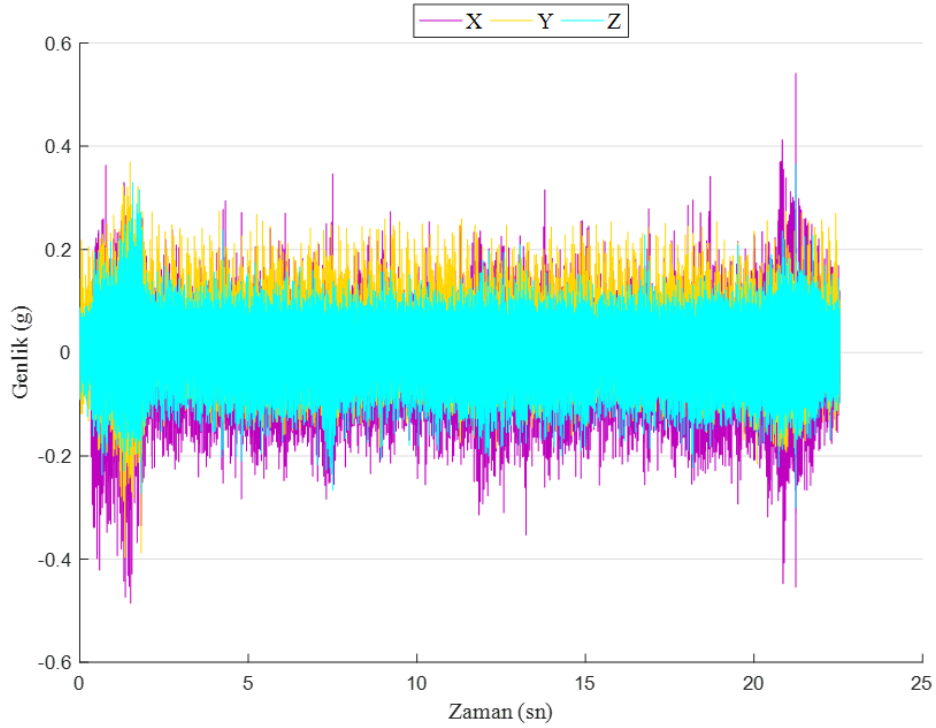
Şekil 50. Kompozit malzeme: KFT, Kesici takım: WC, Dönme devri: 5000 dev/dak ve İlerleme: 0,015 mm/dev
