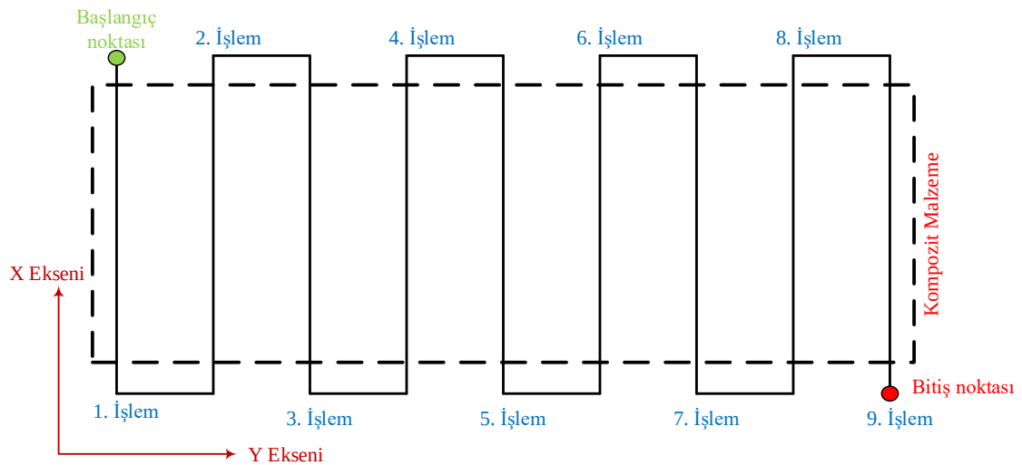
Şekil 3.7. Kesici takımın izlediği yol
