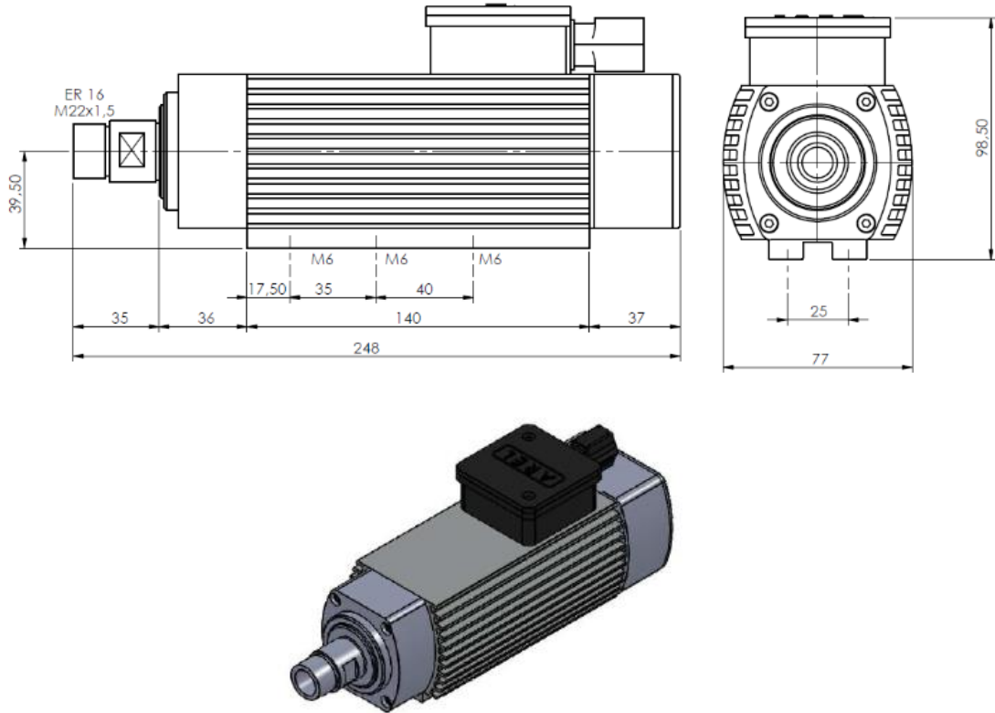
Şekil 3.6. ARFM 1Y-M4 model yüksek frekans motoru
