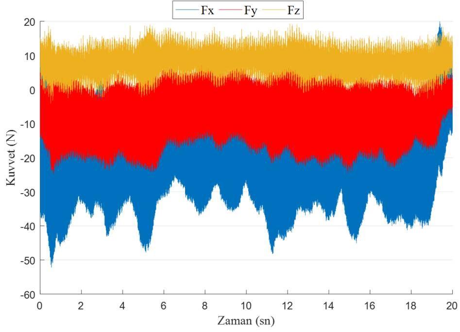
Şekil 7. Kompozit malzeme: JFT, Kesici takım: HSS, Dönme devri: 7500 dev/dak ve İlerleme: 0,01 mm/dev
