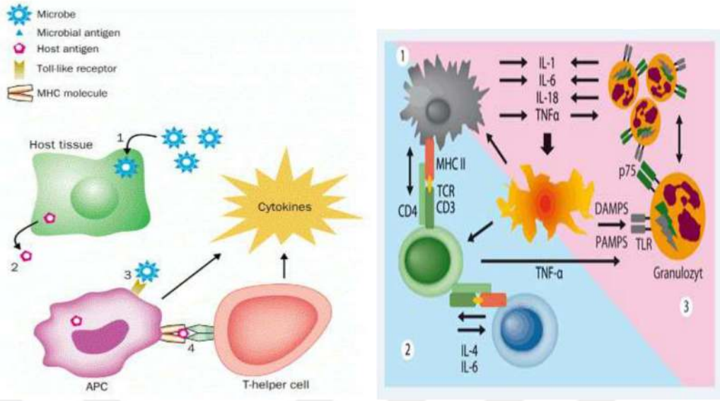
Şekil 2. JİA’da etyopatogenez (44)
