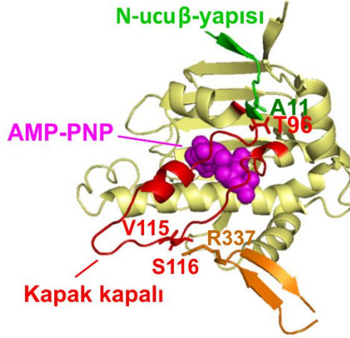
(A) Hsp-90-ND kapalı üç boyutlu yapısı
