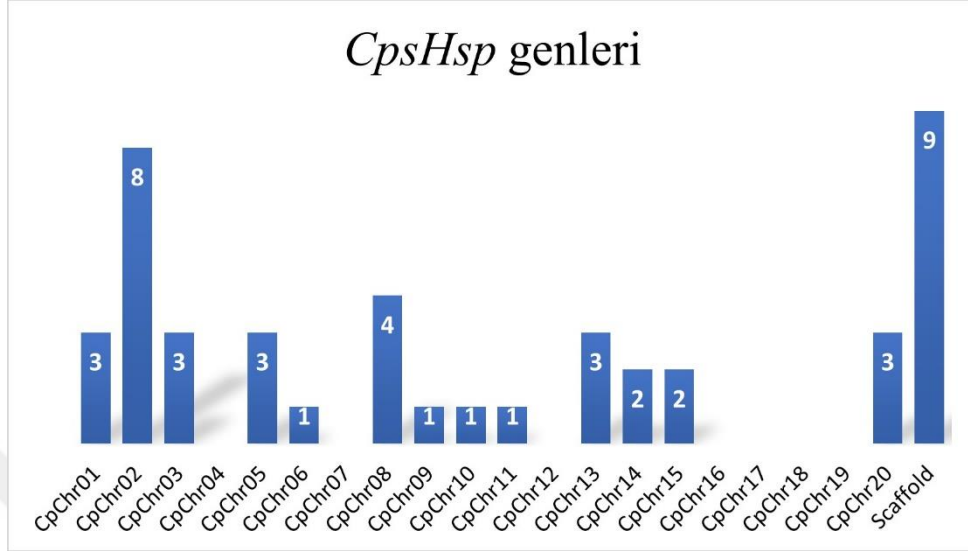
Şekil 5.1 CpsHsp genlerinin kabak kromozomları üzerinde dağılım grafiği
