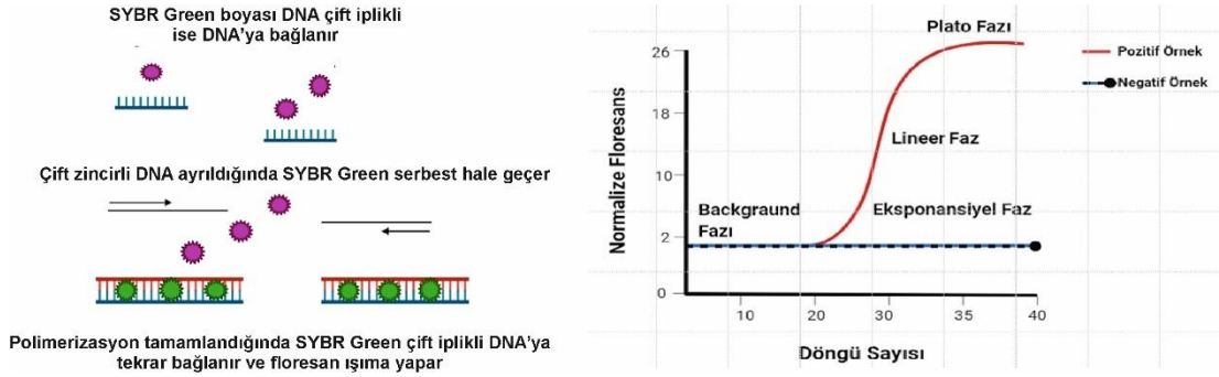
Şekil 2.11 SYBR Green yöntemi kullanılarak gerçek zamanlı PZR reaksiyonu ve grafiği (Wilhelm ve Pingoud, 2003)
