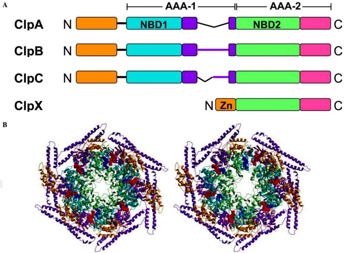
Şekil 2.8 Hsp100 proteini alt birimleri (a), Hsp100 proteini kristal yapısı (b) (S. Lee, Sowa, Choi ve Tsai, 2004)
