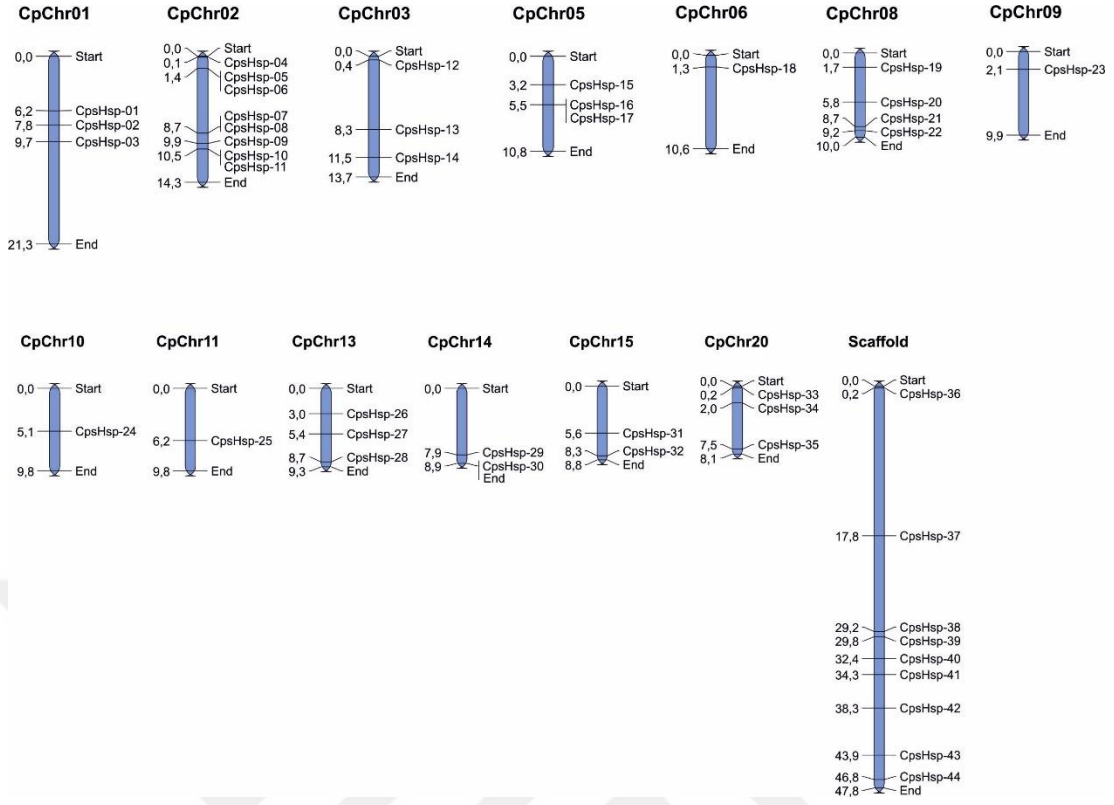
Şekil 5.2 CpHsp genlerinin kabak kromozomları üzerinde dağılımları
