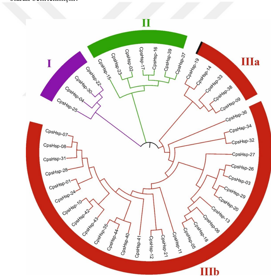
Şekil 5.29 CpsHsp ailesinin filogenetik ağacı
