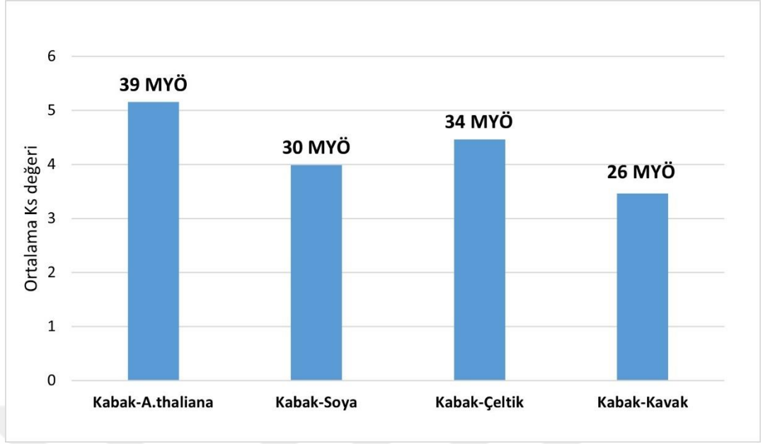
Şekil 5.38 CpHsp60 genlerinin diğer model organizmalar ile ortolog ilişkileri
