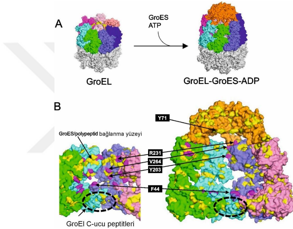
Şekil 2.5 Hsp60 proteinin yapısı (a), GroEL X-ray kristal yapısı (b) (Asea ve Kaur, 2018)
