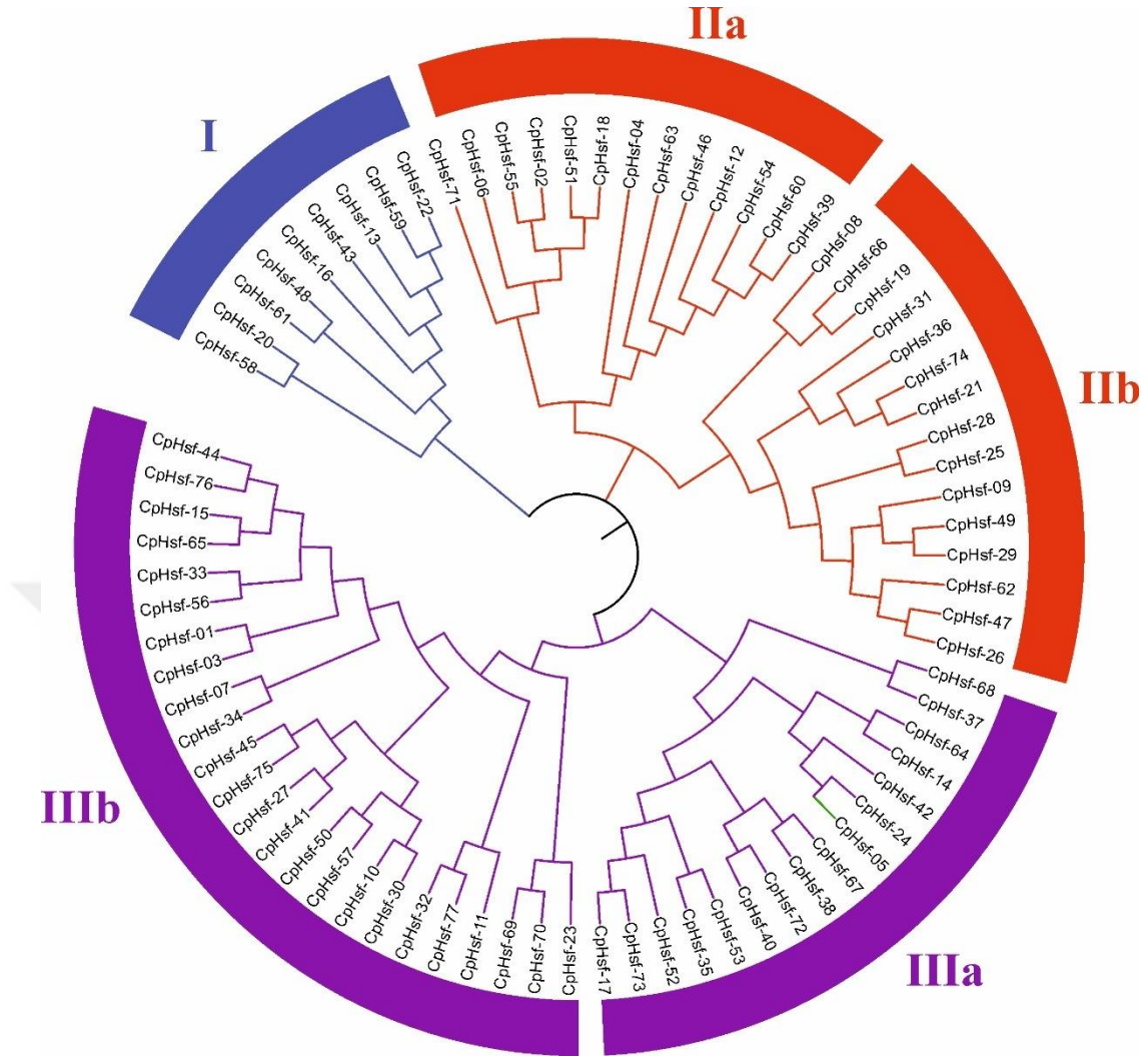
Şekil 5.35 CpHsf ailesinin filogenetik ağacı
