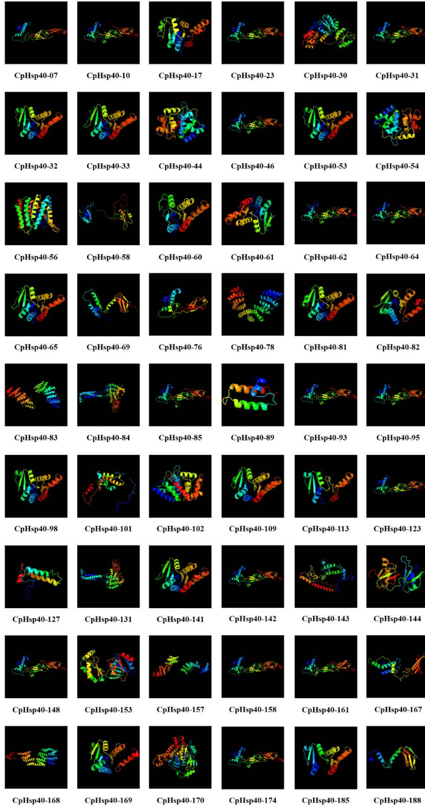
Şekil 5.44 CpHsp40 proteinlerinin tahmini üç boyutlu yapıları
