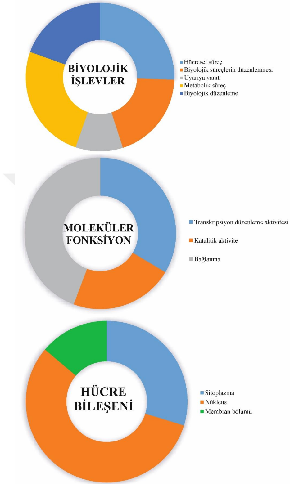
Şekil 5.70 CpHsf genlerinin gen ontoloji analizleri sonuçları
