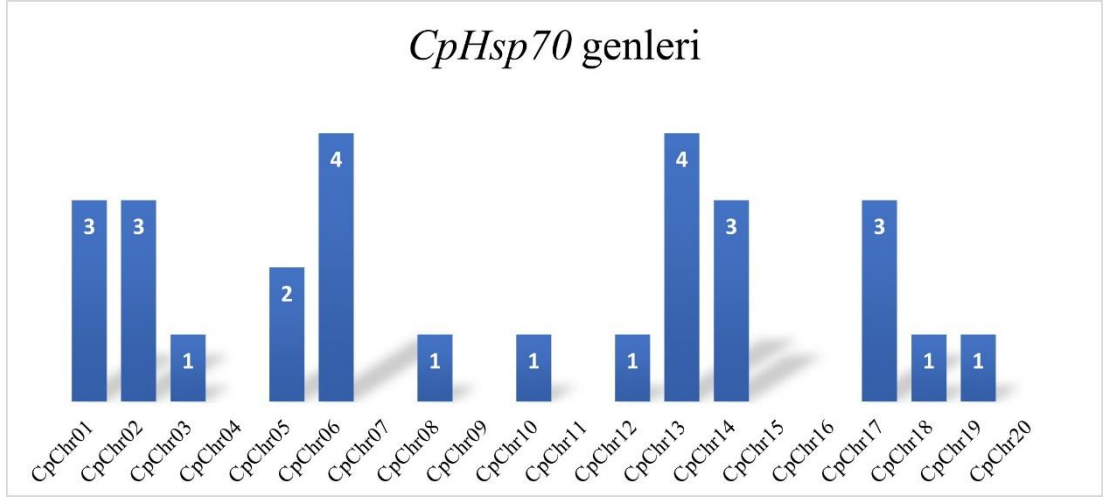
Şekil 5.7 CpHsp70 genlerinin kabak kromozomları üzerinde dağılım grafiği
