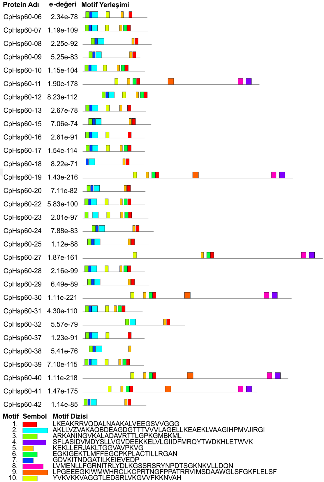
Şekil 5.17 CpHsp60 ailesine ait korunmuş motif organizasyonları
