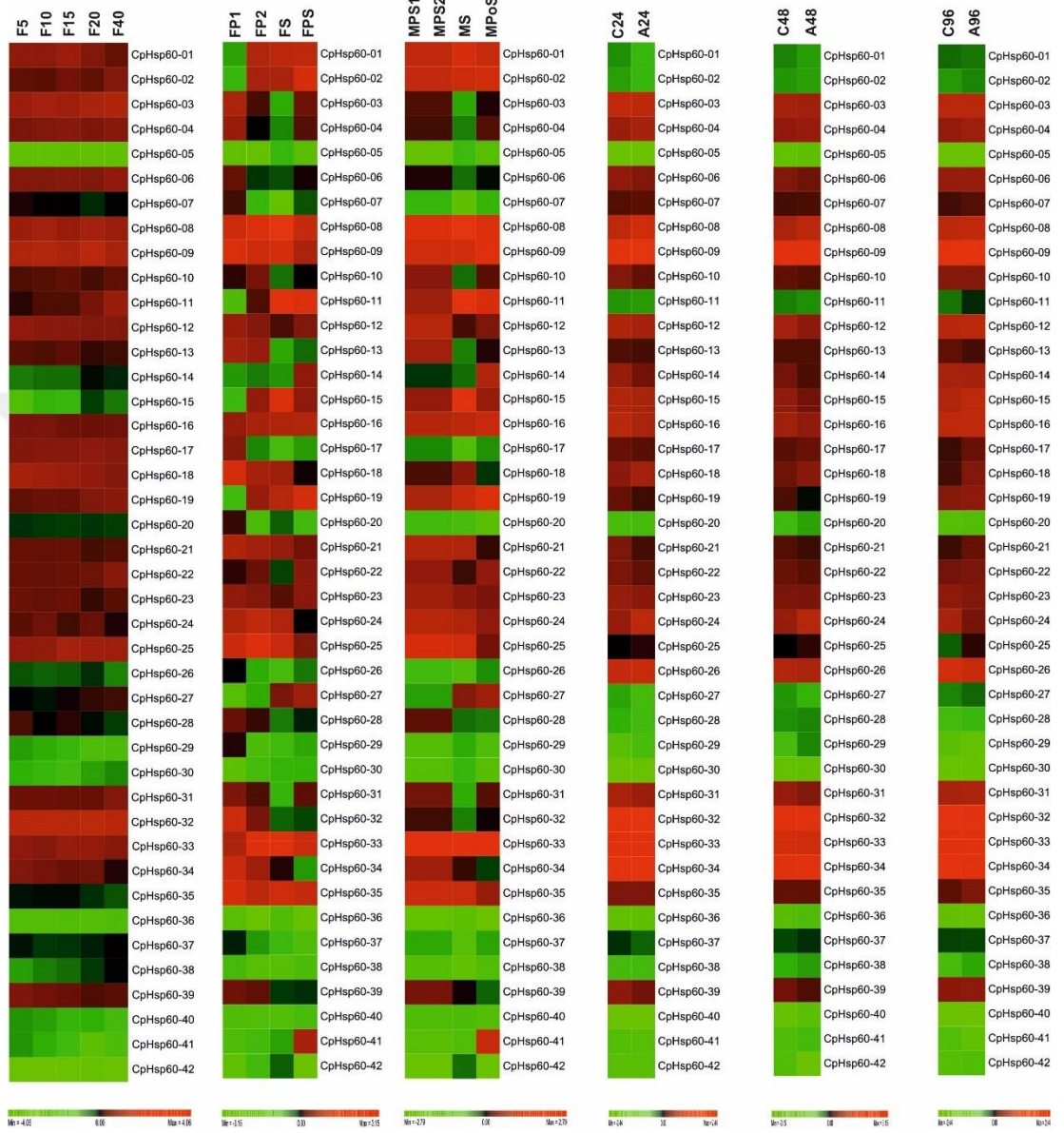
Şekil 5.73 Transkriptom verileri ile hazırlanmış CpHsp60 genlerine ait ısı haritaları
