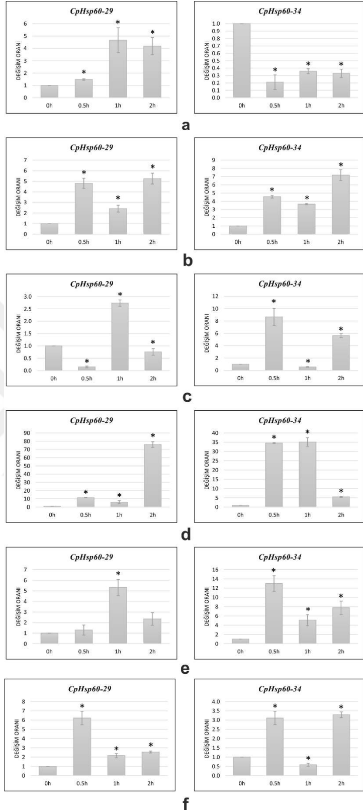
Şekil 5.80 CpHsp60-29 ve CpHsp60-34 genlerine ait (a) Cordelia çeşidi-yüksek sıcaklık stresi (b) Cordelia çeşidi-kuraklık stresi, (c) Cordelia çeşidi-yüksek sıcaklık-kuraklık kombine stresi, (d) Seyden çeşidi-yüksek sıcaklık stresi, (e) Seyden çeşidi-kuraklık stresi, (f) Seyden çeşidi-yüksek sıcaklık-kuraklık kombine stresi (* p < 0,05 'i ifade etmektedir)
