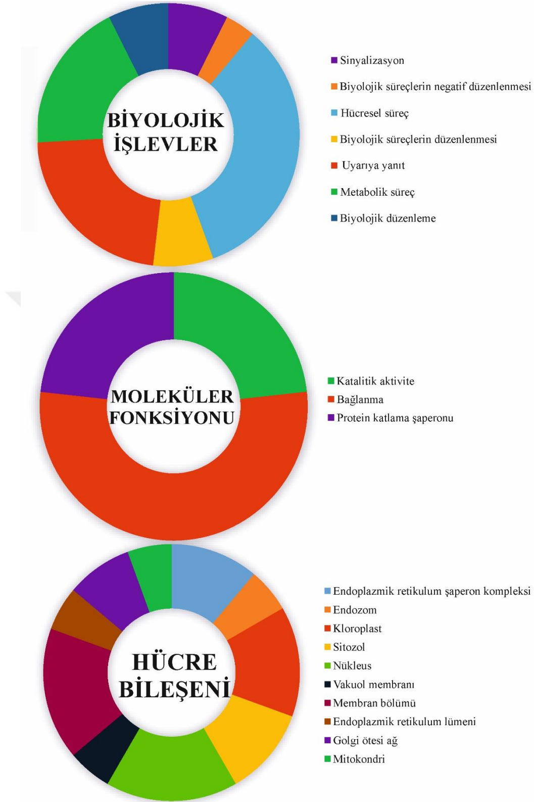
Şekil 5.67 CpHsp70 genlerinin gen ontoloji analizleri sonuçları
