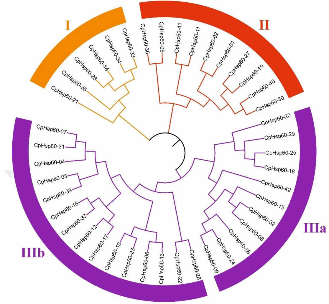
Şekil 5.31 CpHsp60 ailesinin filogenetik ağacı
