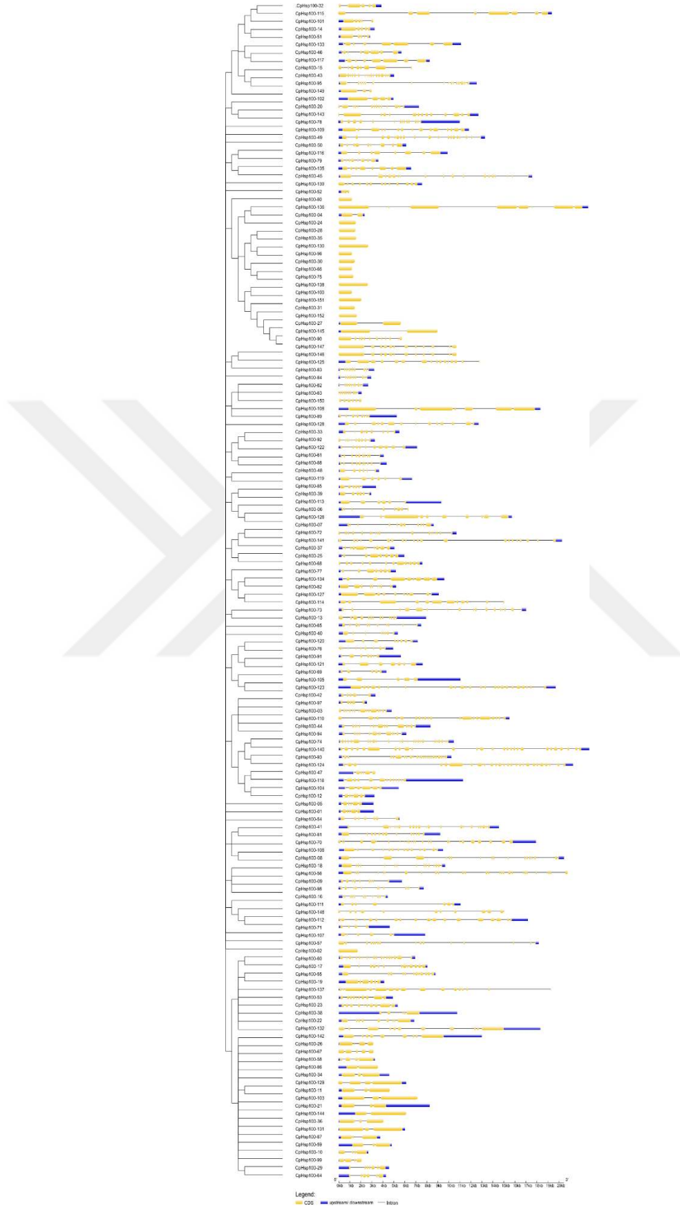
Şekil 5.27 CpHsp100 genlerinin ekzon-intron bölgeleri organizasyonu
