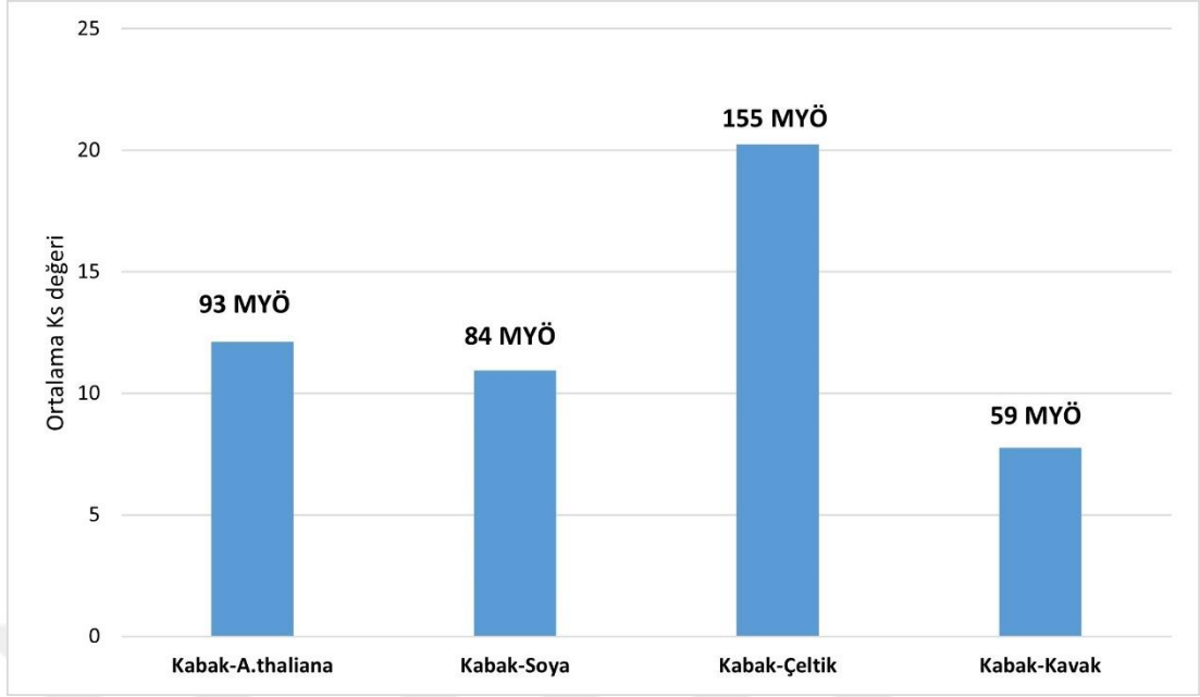
Şekil 5.37 CpHsp40 genlerinin diğer model organizmalar ile ortolog ilişkileri
