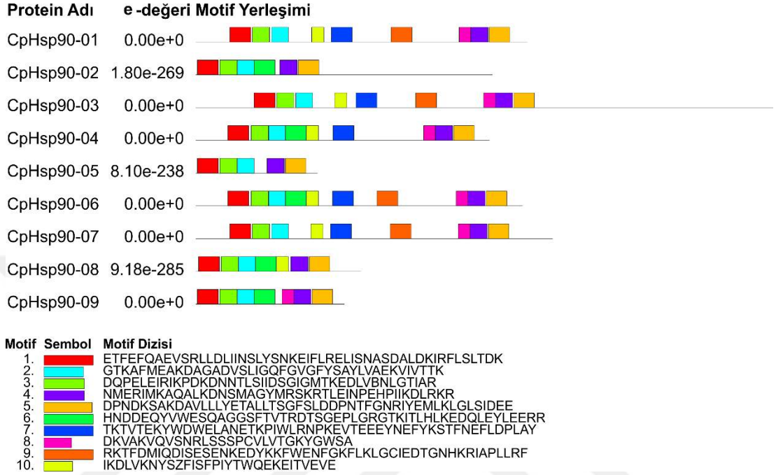
Şekil 5.19 CpHsp90 ailesine ait korunmuş motif organizasyonları
