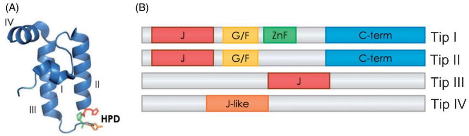
Şekil 2.4 Tipik J-domaini içeren Hsp40 proteini (a), Hsp40 proteinini yapısal olarak sınıflandırması (b) (A. K. Verma vd., 2019)
