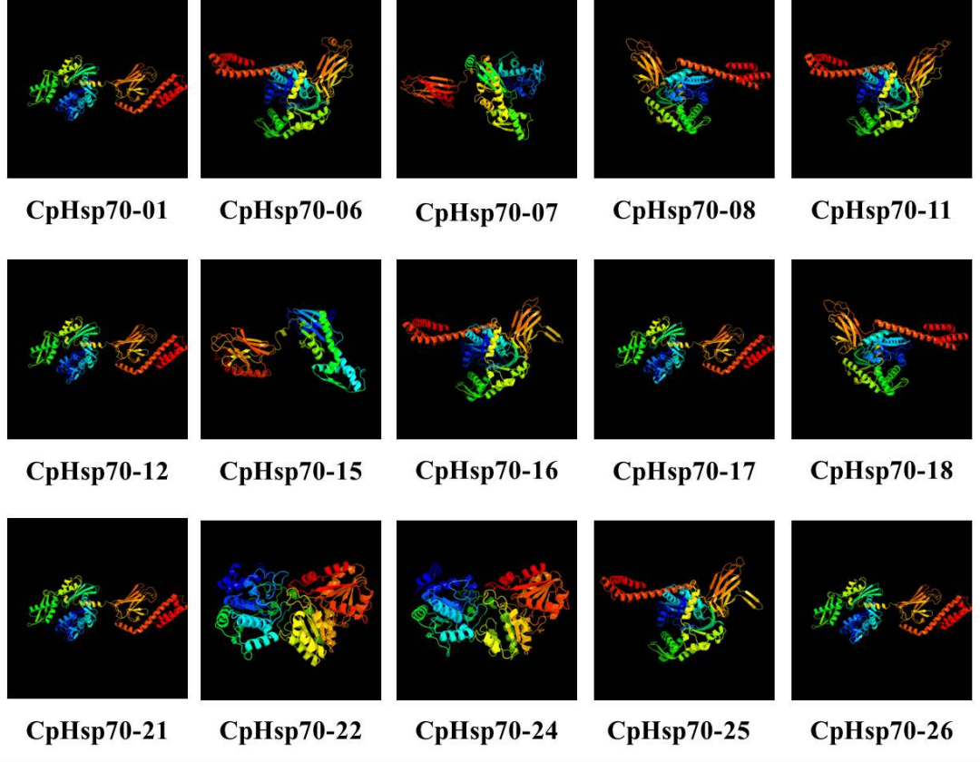
Şekil 5.46 CpHsp70 proteinlerinin tahmini üç boyutlu yapıları
