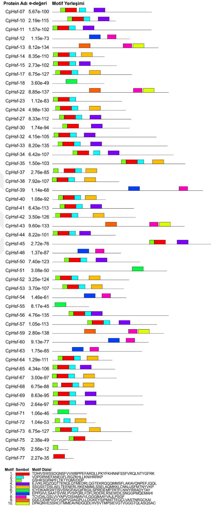
Şekil 5.21 CpHsf ailesine ait korunmuş motif organizasyonları
