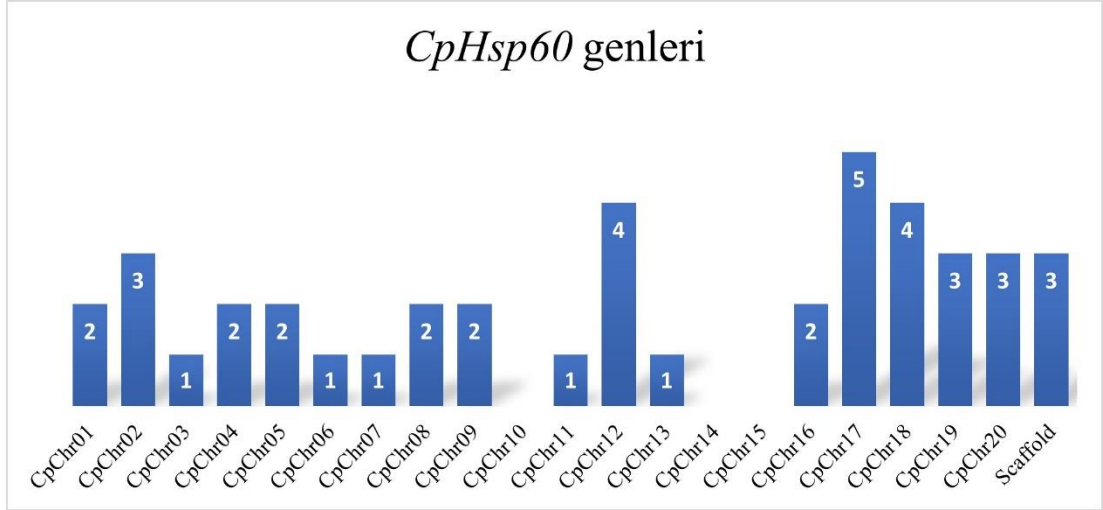
Şekil 5.5 CpHsp60 genlerinin kabak kromozomları üzerinde dağılım grafiği
