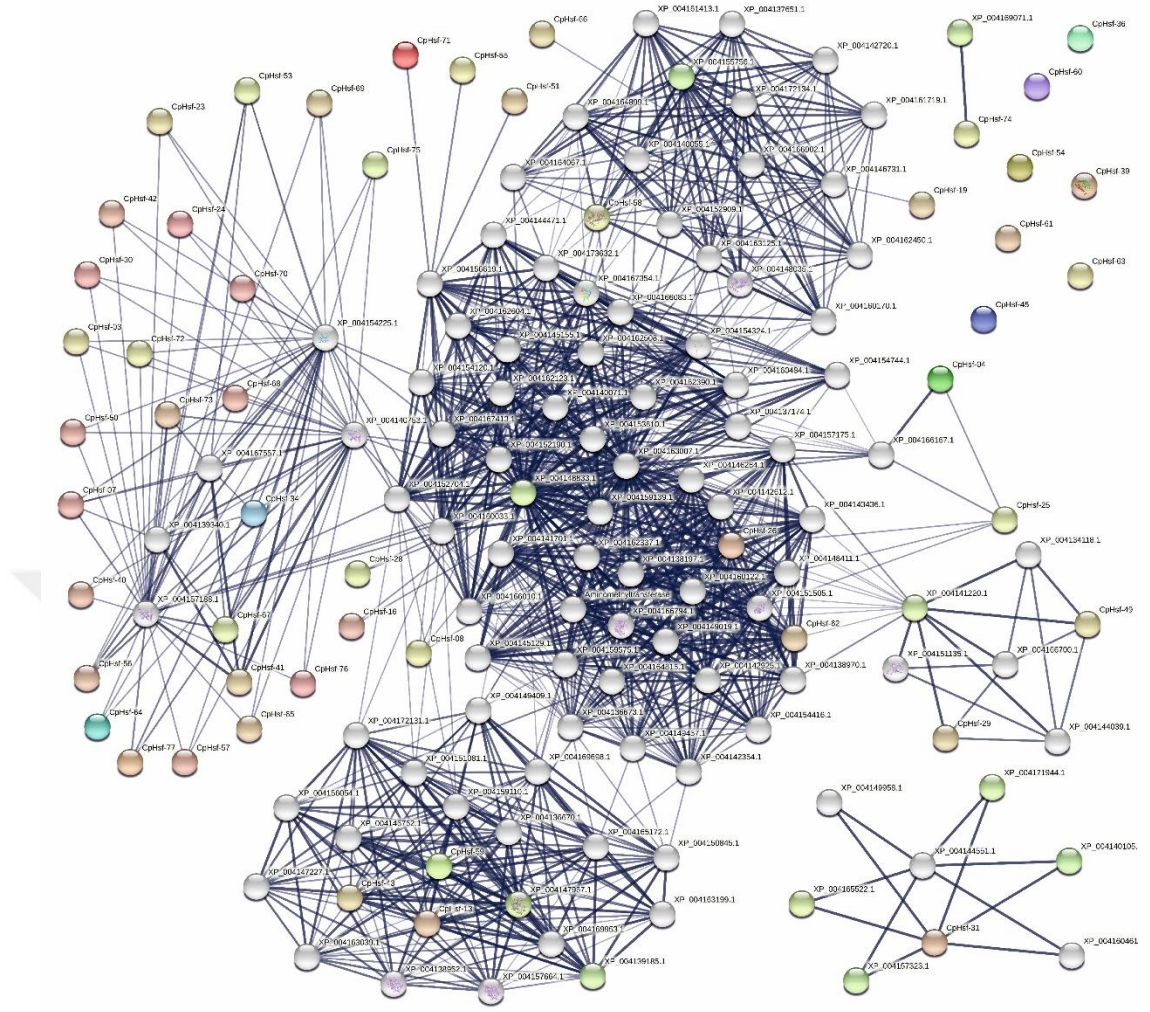
Şekil 5.63 CpHsf proteinlerinin protein-protein etkileşim haritası
