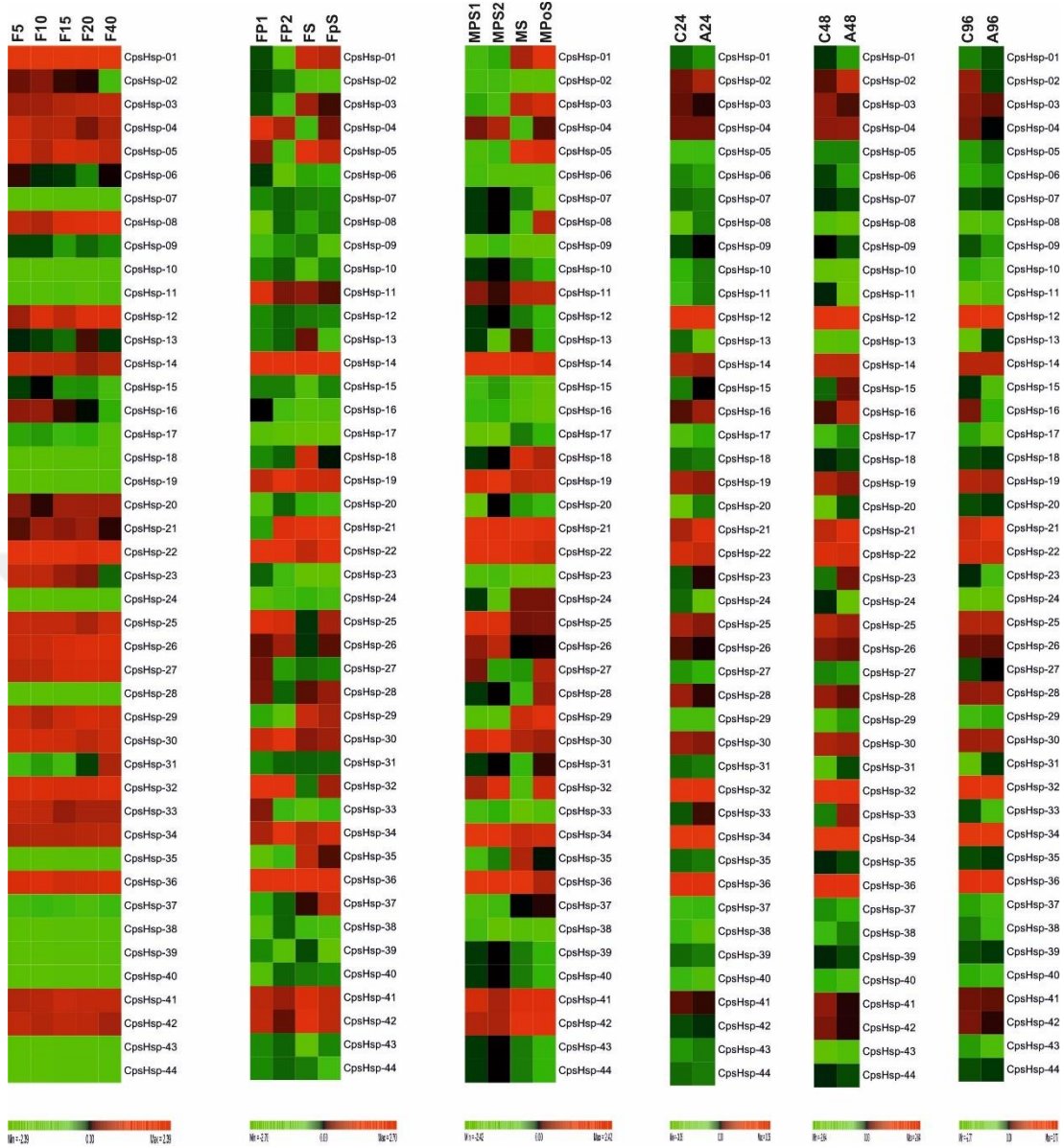
Şekil 5.71 Transkriptom verileri ile hazırlanmış CpsHsp genlerine ait ısı haritaları
