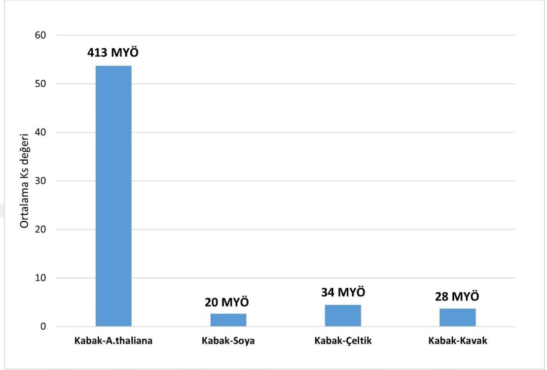
Şekil 5.36 CpsHsp genlerinin diğer model organizmalar ile ortolog ilişkileri
