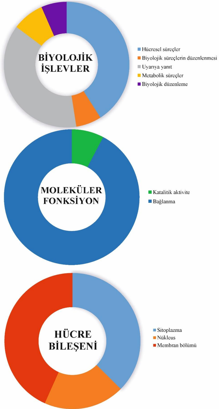
Şekil 5.64 CpsHsp genlerinin gen ontoloji analizleri sonuçları
