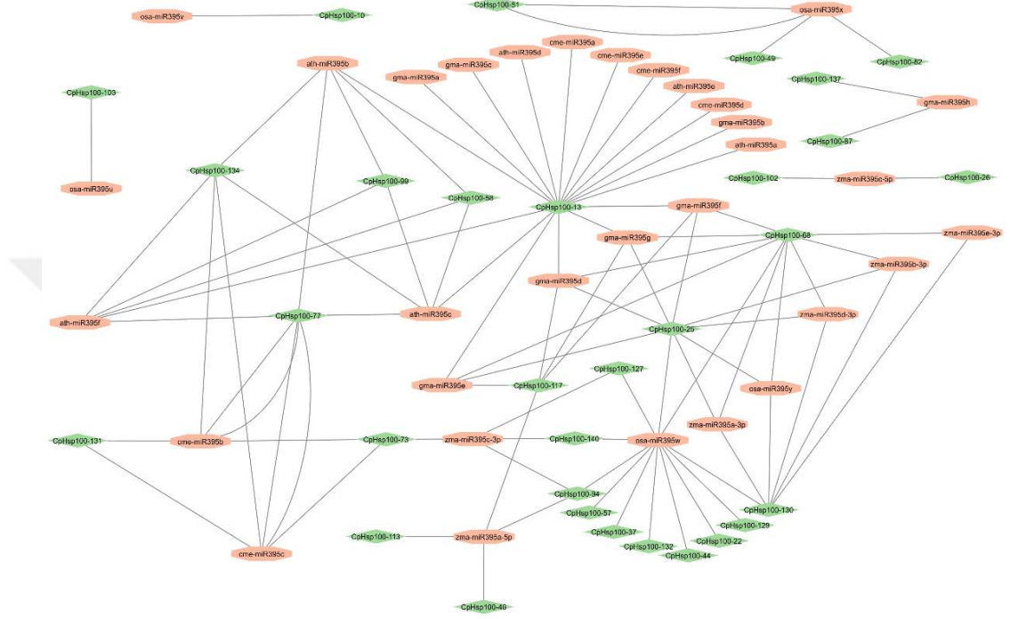
Şekil 5.55 CpHsp100 genlerini hedef alan miRNA'lar
