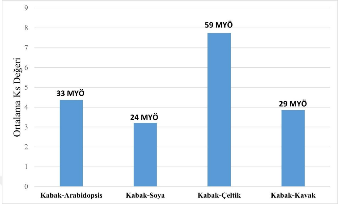
Şekil 5.41 CpHsp100 genlerinin diğer model organizmalar ile ortolog ilişkileri
