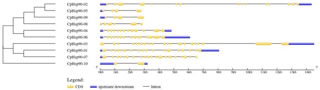
Şekil 5.26 CpHsp90 genlerinin ekzon-intron bölgeleri organizasyonu
