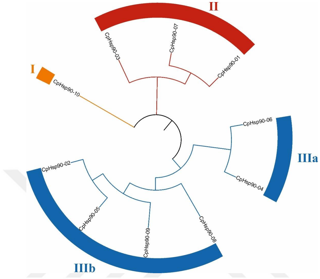
Şekil 5.33 CpHsp90 ailesinin filogenetik ağacı
