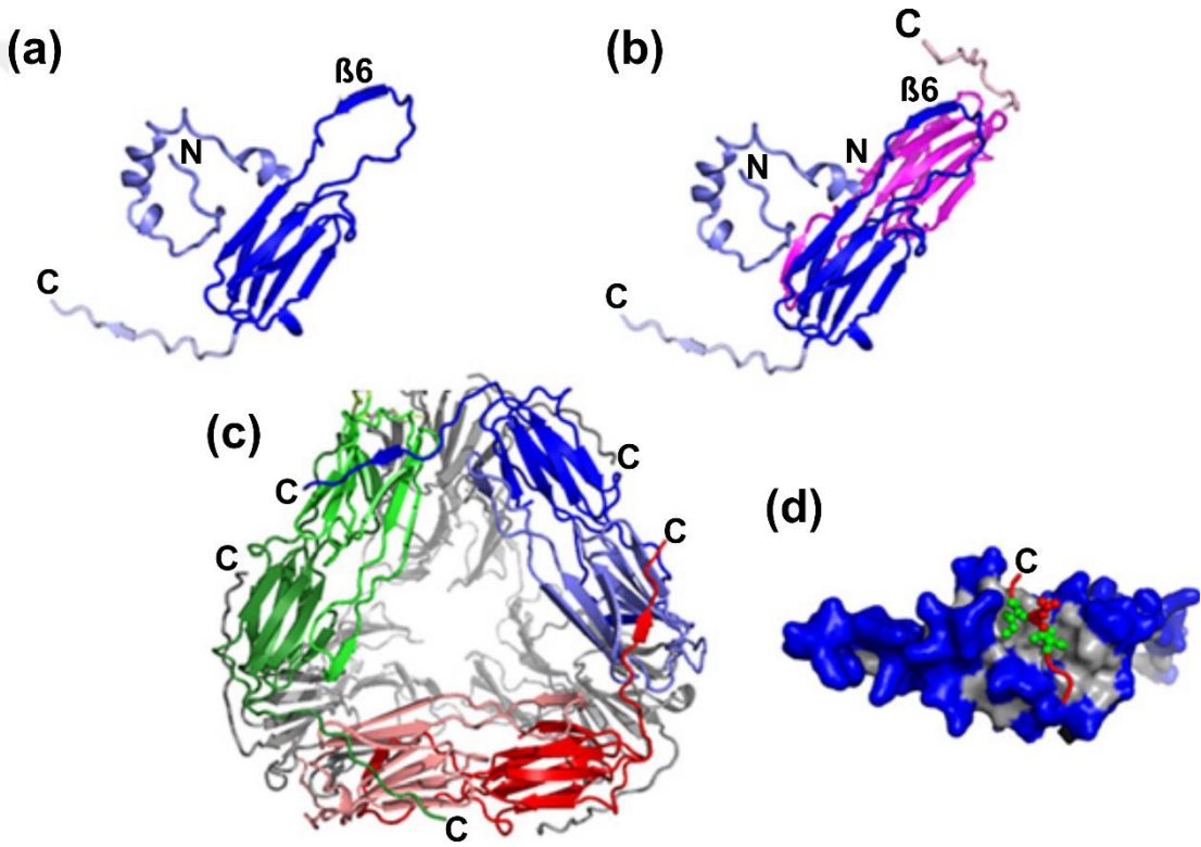
Şekil 2.3 sHsp proteine ait (a) monomer yapısı, (b) dimer yapısı, (c) üç boyutlu yapı, (d) üç boyutlu yapı (Waters ve Vierling, 2020)
