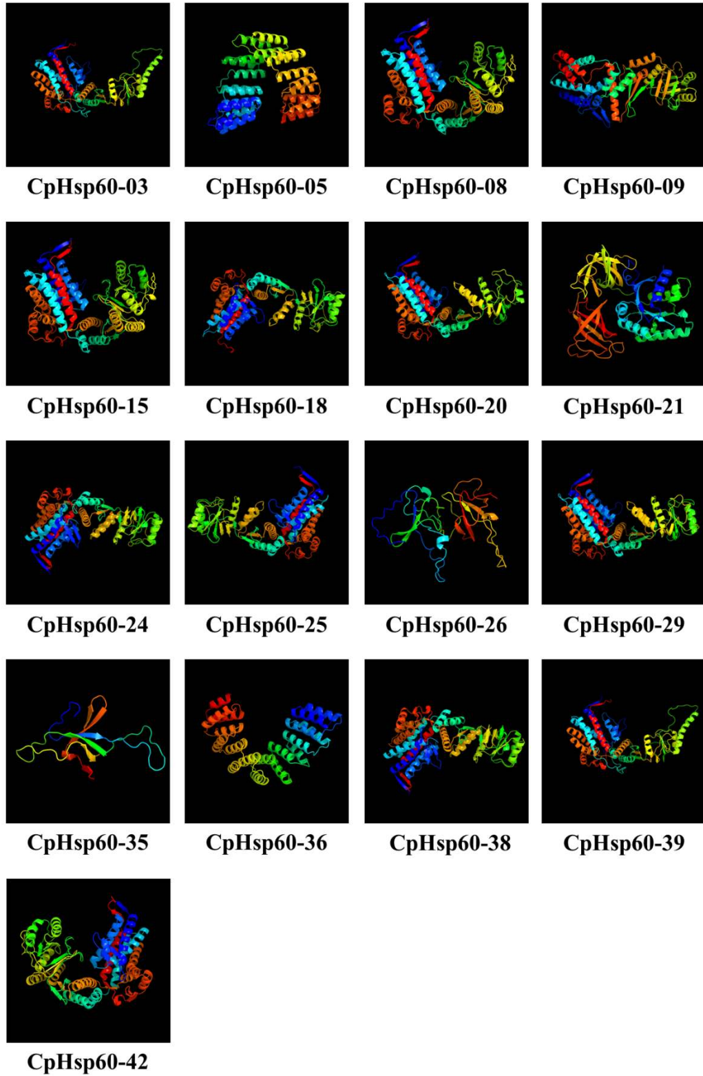
Şekil 5.45 CpHsp60 proteinlerinin tahmini üç boyutlu yapıları
