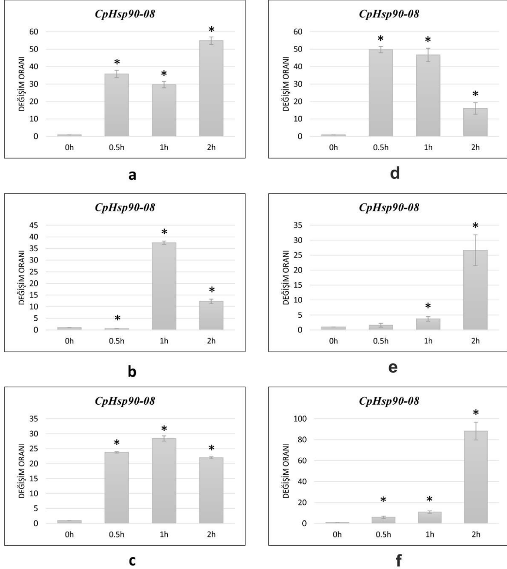
Şekil 5.82 CpHsp90-08 genine ait (a) Cordelia çeşidi-yüksek sıcaklık stresi (b) Cordelia çeşidi-kuraklık stresi, (c) Cordelia çeşidi-yüksek sıcaklık-kuraklık kombine stresi, (d) Seyden çeşidi-yüksek sıcaklık stresi, (e) Seyden çeşidi-kuraklık stresi, (f) Seyden çeşidi-yüksek sıcaklık-kuraklık kombine stresi (* p < 0,05 'i ifade etmektedir)
