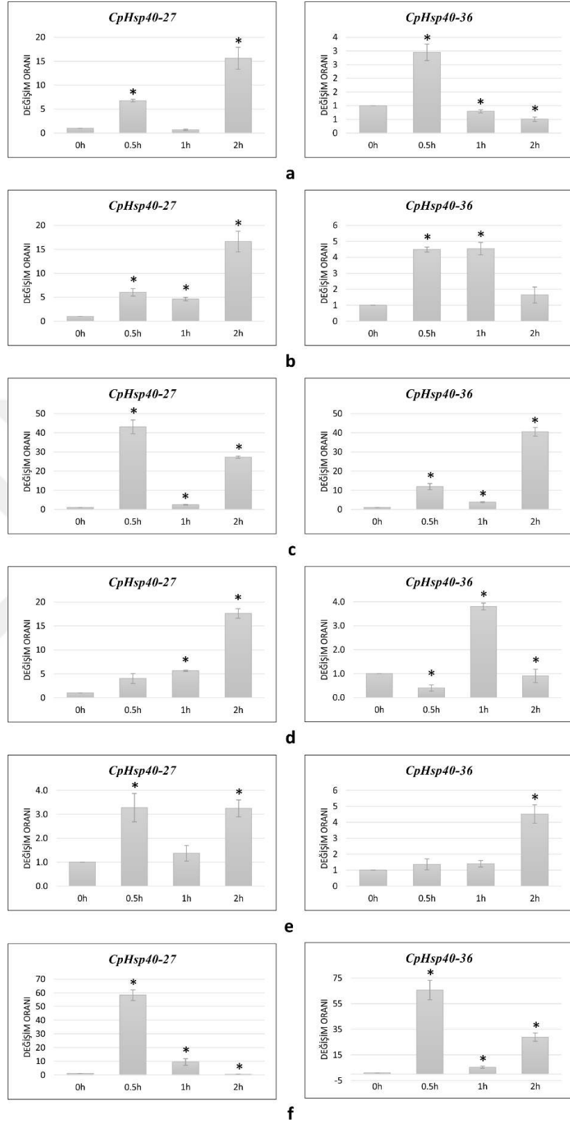
Şekil 5.79 CpHsp40-27 ve CpHsp40-36 genlerine ait (a) Cordelia çeşidi-yüksek sıcaklık stresi (b) Cordelia çeşidi-kuraklık stresi, (c) Cordelia çeşidi-yüksek sıcaklık-kuraklık kombine stresi, (d) Seyden çeşidi-yüksek sıcaklık stresi, (e) Seyden çeşidi-kuraklık stresi, (f) Seyden çeşidi-yüksek sıcaklık-kuraklık kombine stresi (* p < 0,05 'i ifade etmektedir)
