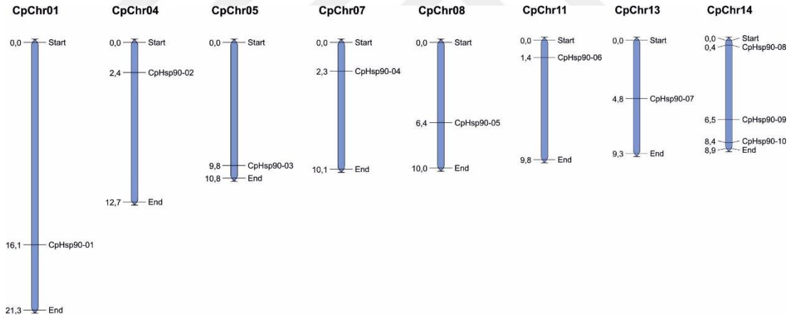
Şekil 5.10 CpHsp90 genlerinin kabak kromozomları üzerinde dağılımları
