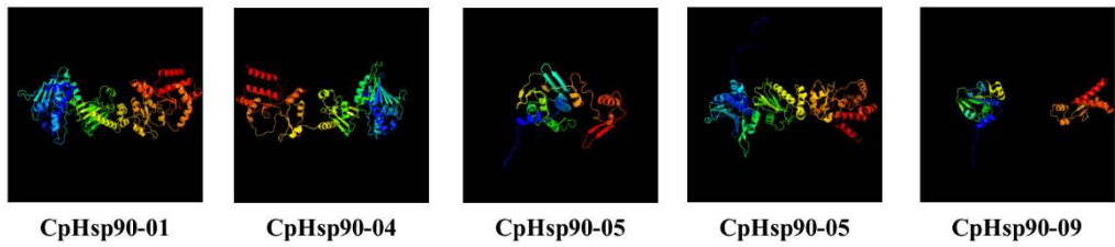
Şekil 5.47 CpHsp90 proteinlerinin tahmini üç boyutlu yapıları
