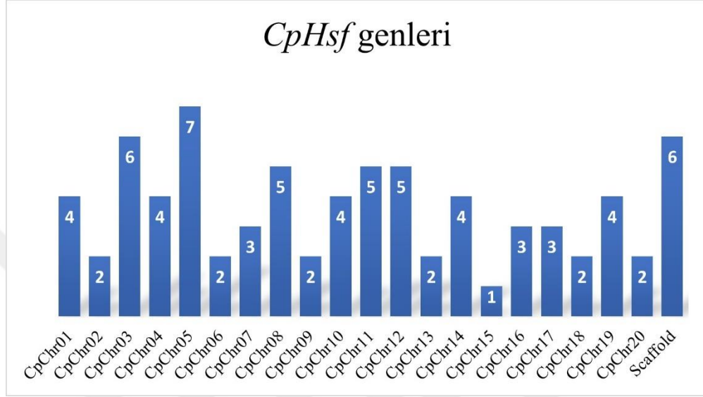
Şekil 5.13 CpHsf genlerinin kabak kromozomları üzerinde dağılım grafiği
