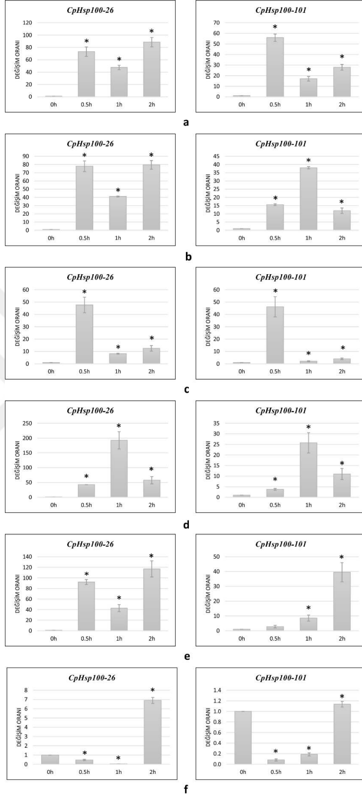
Şekil 5.83 CpHsp100-26 ve CpHsp100-101 genlerine ait (a) Cordelia çeşidi-yüksek sıcaklık stresi (b) Cordelia çeşidi-kuraklık stresi, (c) Cordelia çeşidi-yüksek sıcaklık-kuraklık kombine stresi, (d) Seyden çeşidi-yüksek sıcaklık stresi, (e) Seyden çeşidi-kuraklık stresi, (f) Seyden çeşidi-yüksek sıcaklık-kuraklık kombine stresi (* p < 0,05 'i ifade etmektedir)
