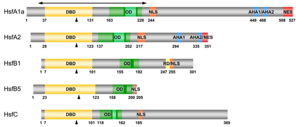
Şekil 2.9 Domates bitkisinde örneklenen Hsf'nin temel yapısı. Oklar ile korunmuş intron bölgesi gösterilmiştir. DBD: DNA bağlanma alanı; OD: Oligomerizasyon alanı (HR-A/B); NLS: Nükleer lokalizasyon sinyali, AHA: Etkinleştirici motif (Asea ve Kaur, 2018)
