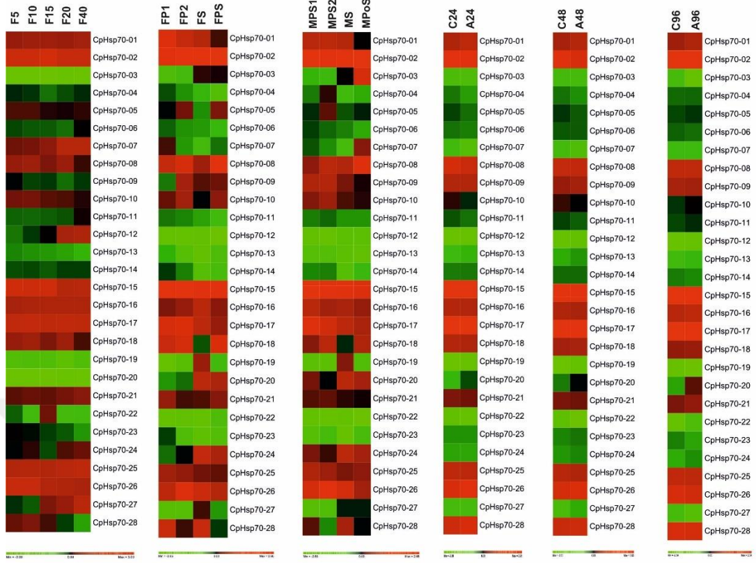
Şekil 5.74 Transkriptom verileri ile hazırlanmış CpHsp70 genlerine ait ısı haritaları
