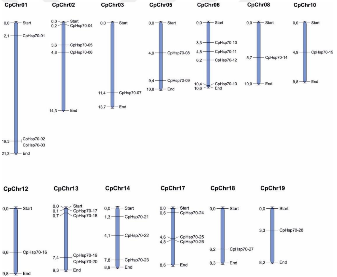
Şekil 5.8 CpHsp70 genlerinin kabak kromozomları üzerinde dağılımları
