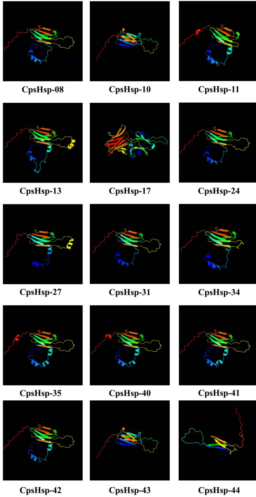
Şekil 5.43 CpsHsp proteinlerinin tahmini üç boyutlu yapıları
