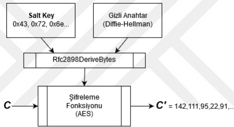
Şekil 6.5 Şifreleme.
