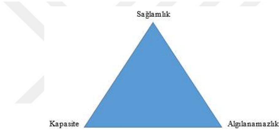
Şekil 7.1 Fridrich üçgeni.
