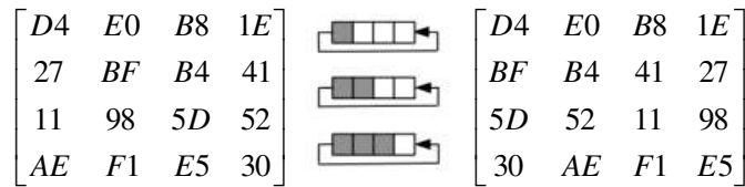
Şekil 3.8 Satır Kaydırma.
