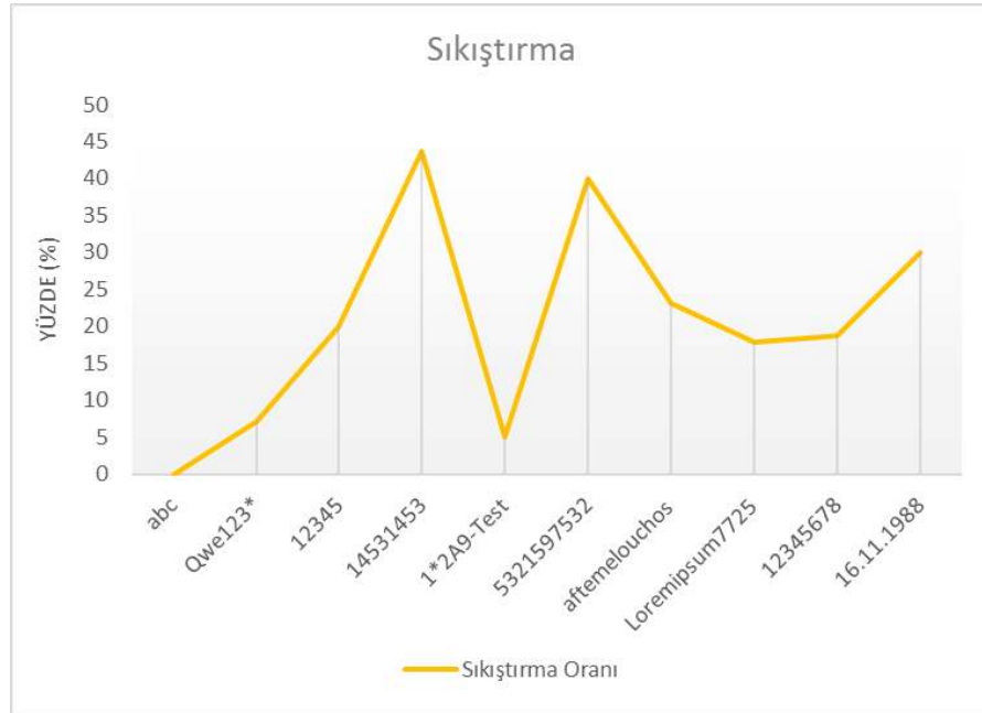
Şekil 7.3 Sıkıştırma oranları (%).
