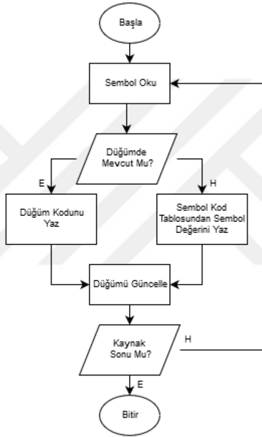
Şekil 4.3 Uyarlanırlı Huffman sıkıştırma akış diyagramı.
