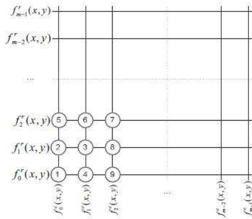
Şekil 3.6. Şebeke bazlı anahtar ön dağıtımını [74].
