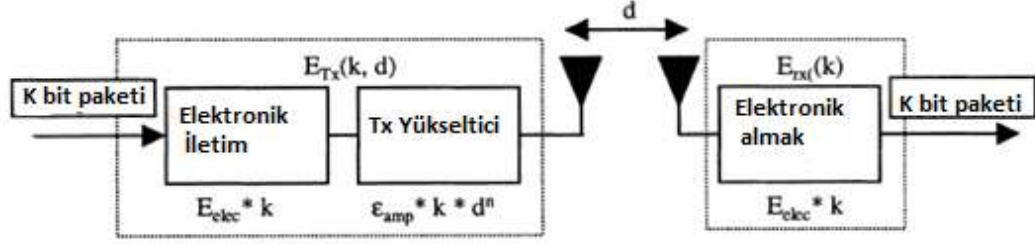
Şekil 3.1. Radyo modeli.
