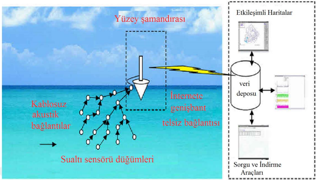
Şekil 2.3. Sualtı WSN
