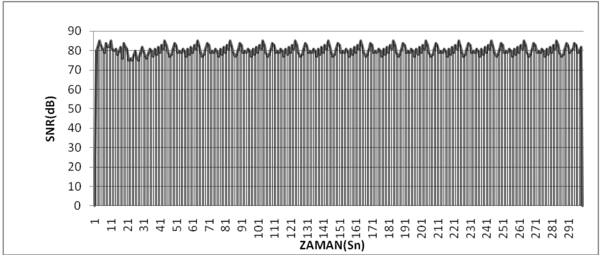
Şekil 24. Kablolu IP telefonda ses sinyali
