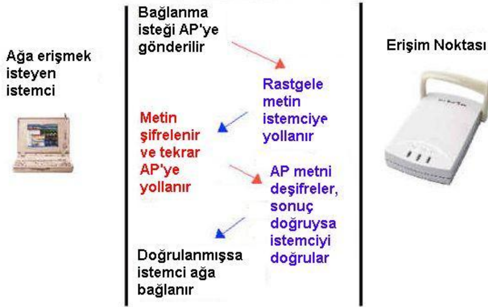
Şekil 8. Paylaşılan Anahtarlı Doğrulama[7].
