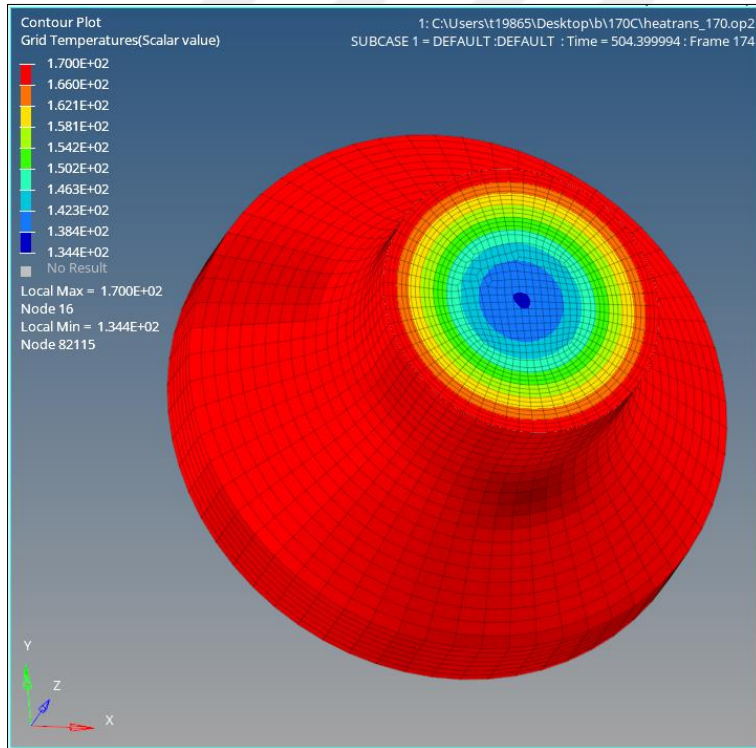
Şekil 5.43. 170 °C kürlenme 504. saniye numune içi dinamik sıcaklık dağılımı
