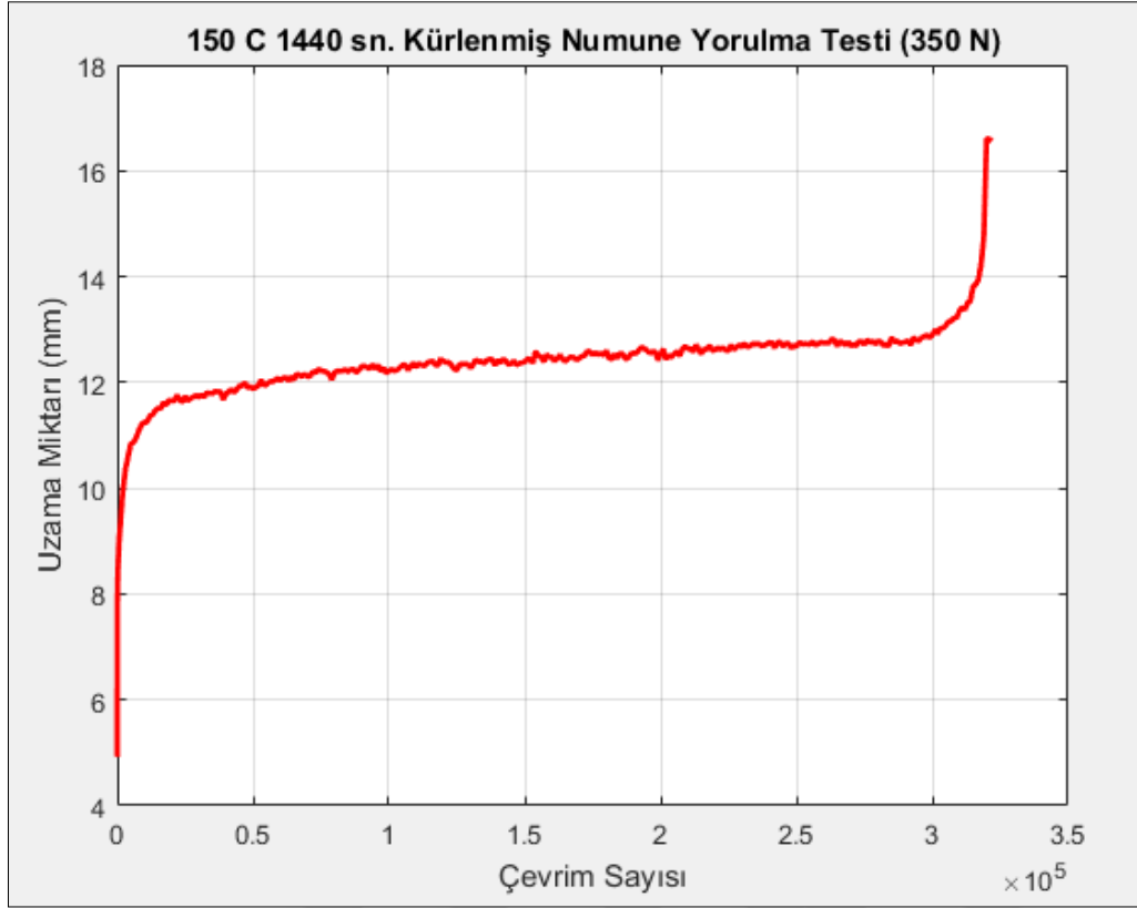
Şekil 5.49. 150 °C 1440 sn kürlenmiş numune yorulma testi uzama miktarı grafiği
