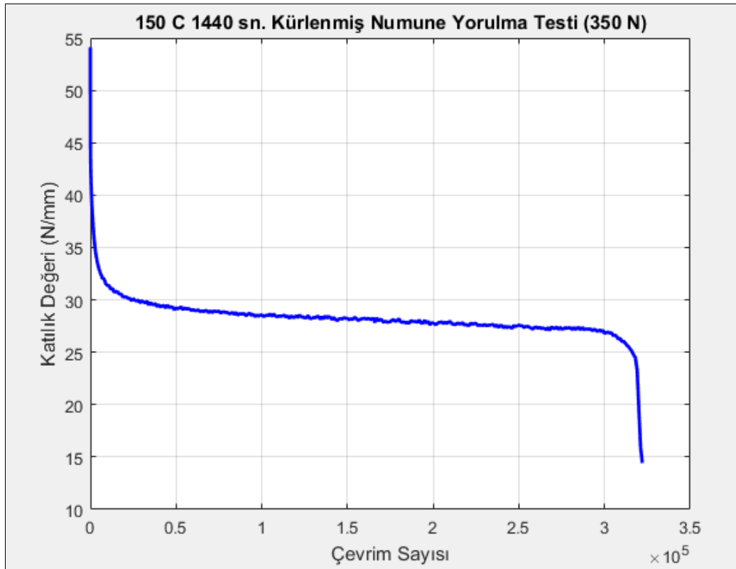
Şekil 5.50. 150 °C 1440 sn kürlenmiş numune yorulma testi katılık değeri grafiği
