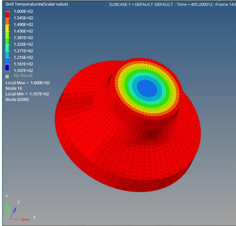
Şekil 5.34. 160 °C kirlenme 405. saniye numune içi dinamik sıcaklık dağılımı
