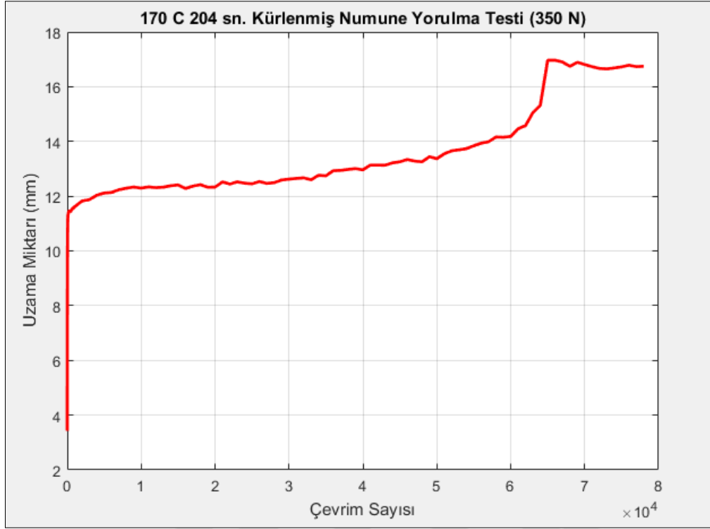
řekil 5.58. 170 °C 204 sn k rlenmiř numune yorulma testi uzama miktarı grafiđi
