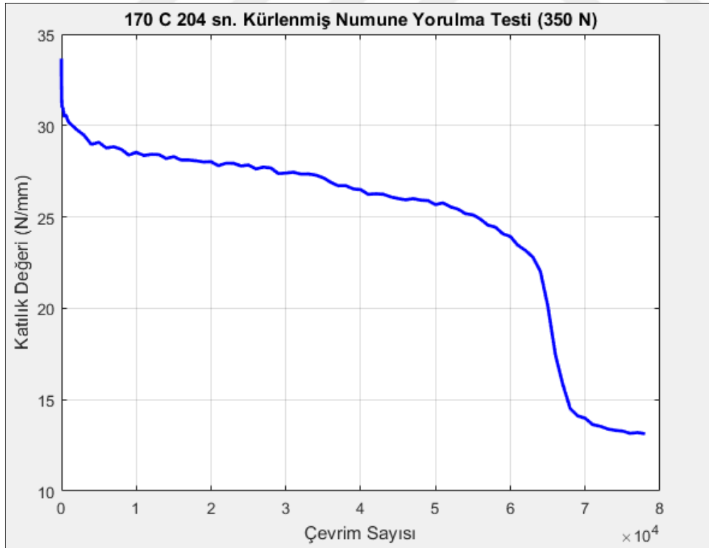
řekil 5.59. 170 °C 204 sn k rlenmiř numune yorulma testi katılık deđeri grafiđi
