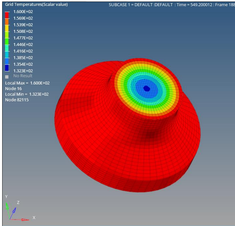
Şekil 5.35. 160 °C kirlenme 550. saniye numune içi dinamik sıcaklık dağılımı
