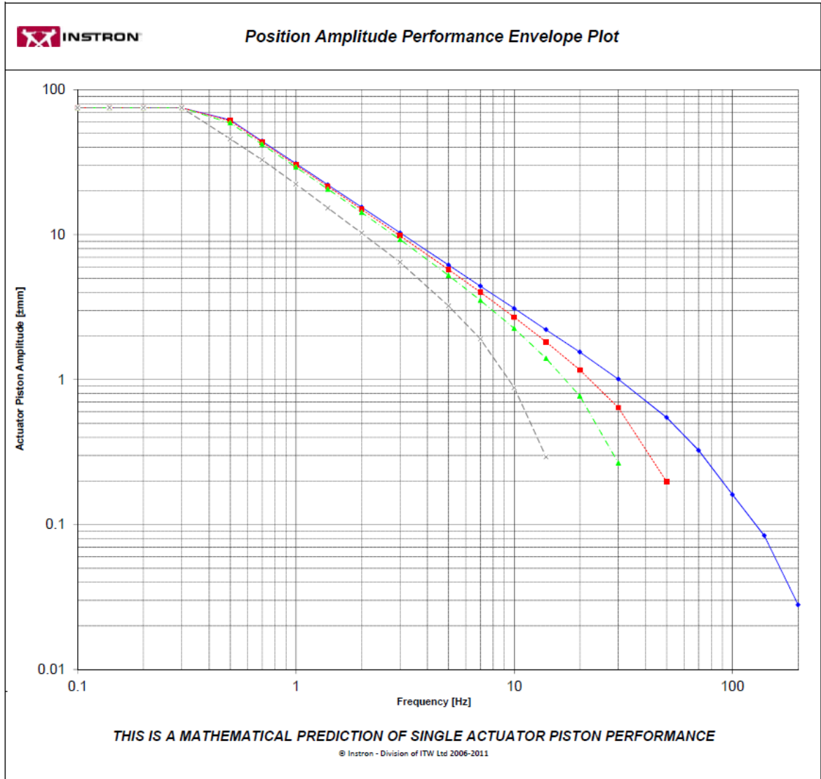
Şekil E1.1. Instron servohidrolik eksenel test cihazı frekans yer değiştirme değerleri
