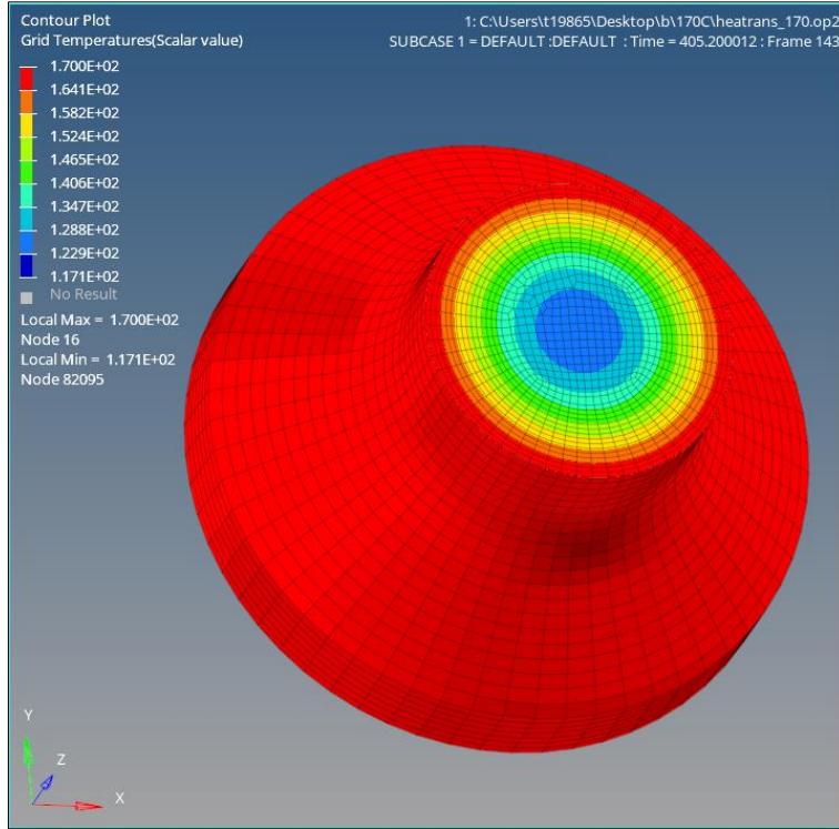
Şekil 5.42. 170 °C kürlenme 404. saniye numune içi dinamik sıcaklık dağılımı
