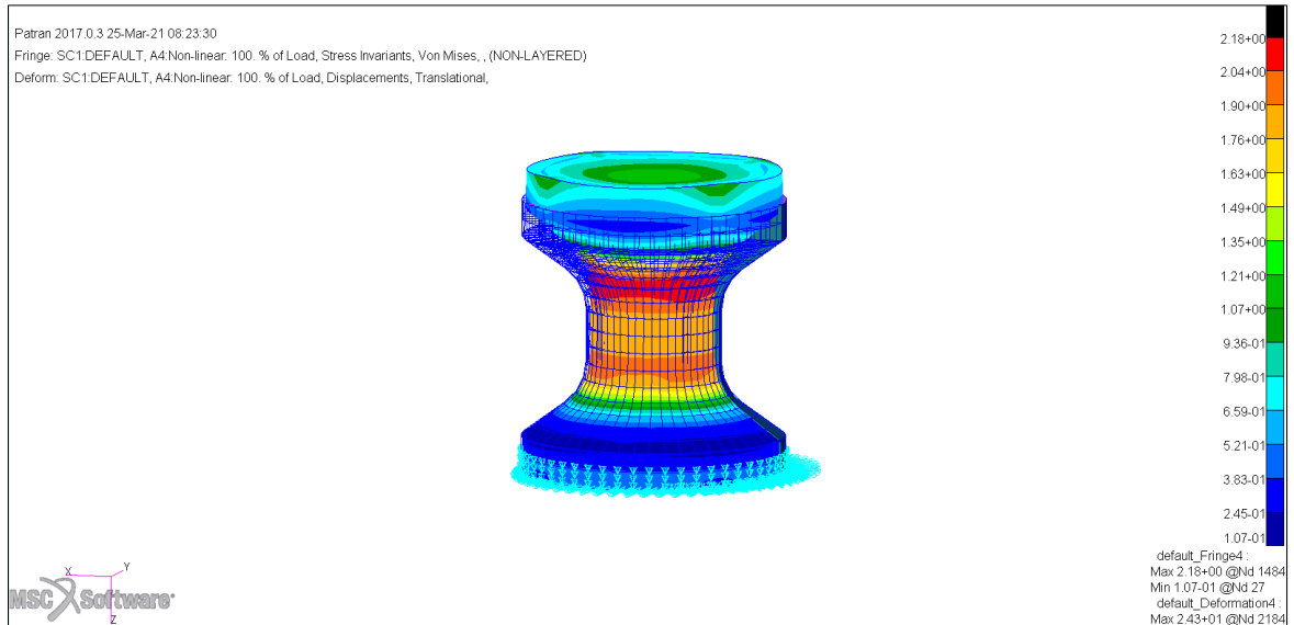
Şekil 5.20. Doğal kauçuk test numunesi 1250 N yük altındaki gerilim dağılımı
