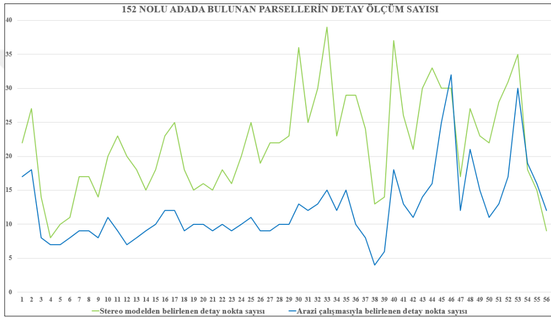
Şekil 4.18. Parseller ilişkin belirlenen detay noktalarının karşılaştırılması.
