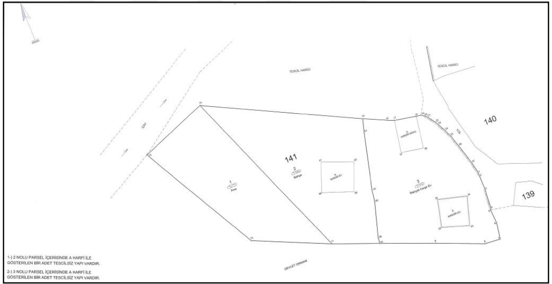
Şekil 4.10. Ölçü krokisi.
