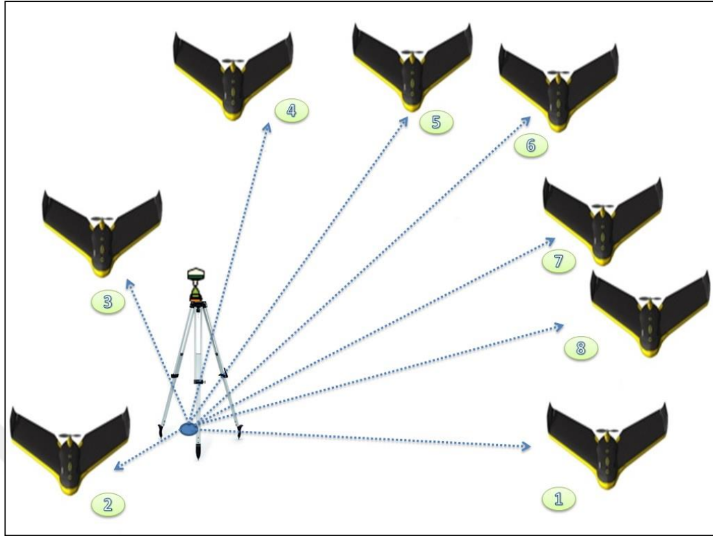
Şekil 3.18. İHA ile görüntü elde etmenin şematik görünümü.
