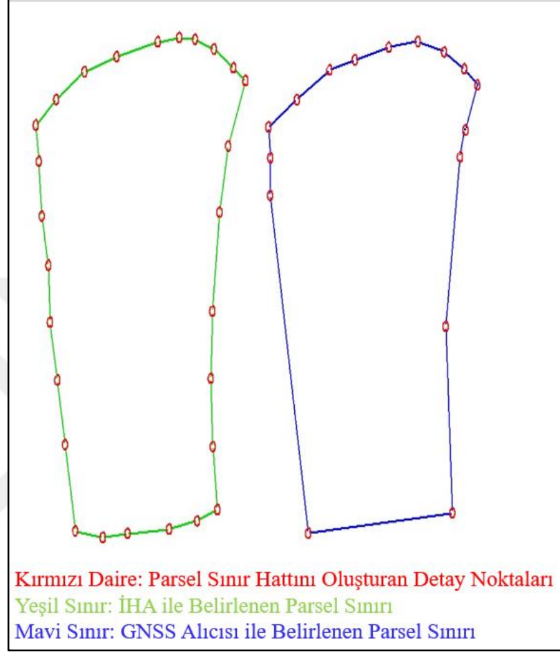
Şekil 4.5. Parseli meydana getiren sınır hattındaki detay noktalarının gösterimi.
