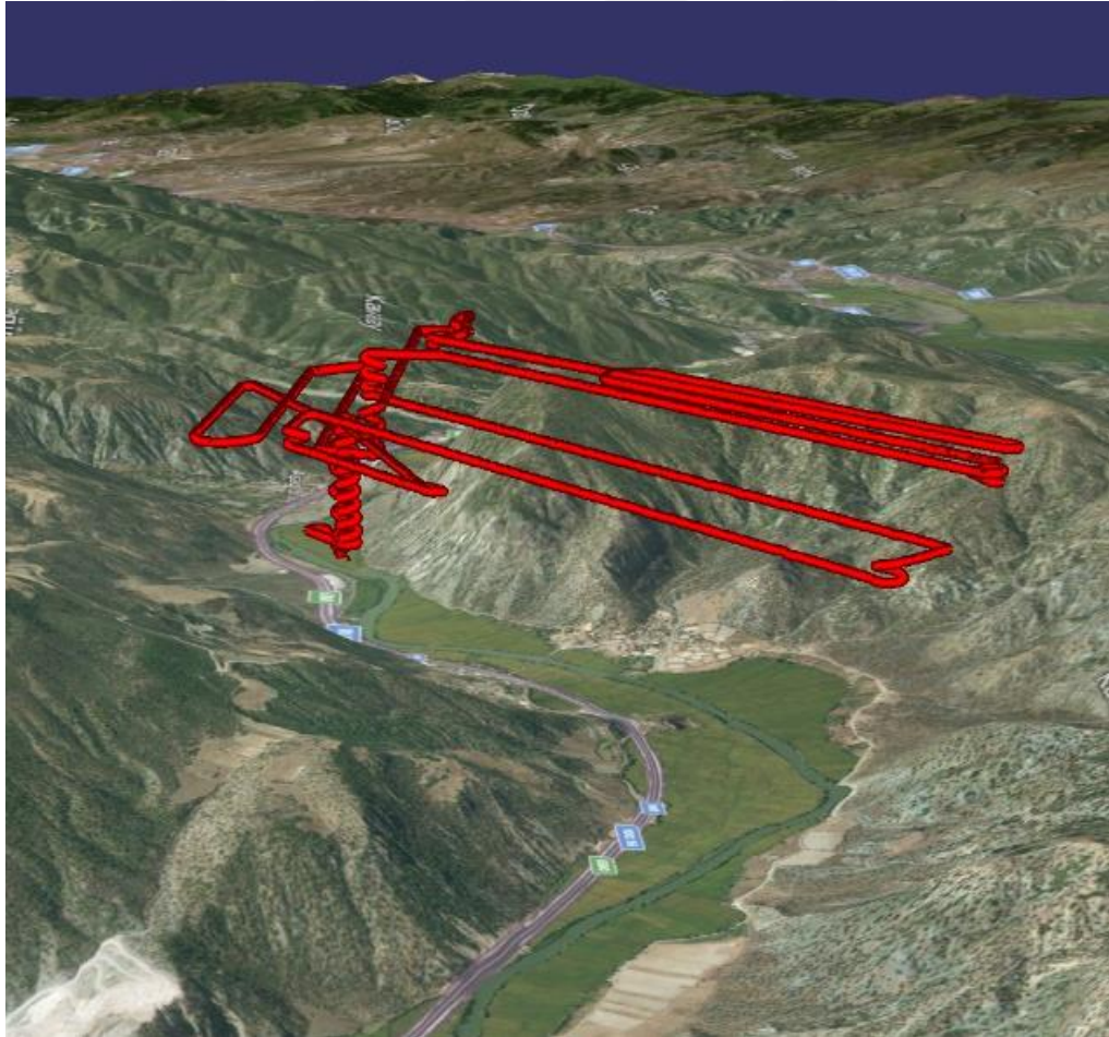
Şekil 3.16. eMotion3 yazılımında uçuş planlaması.
