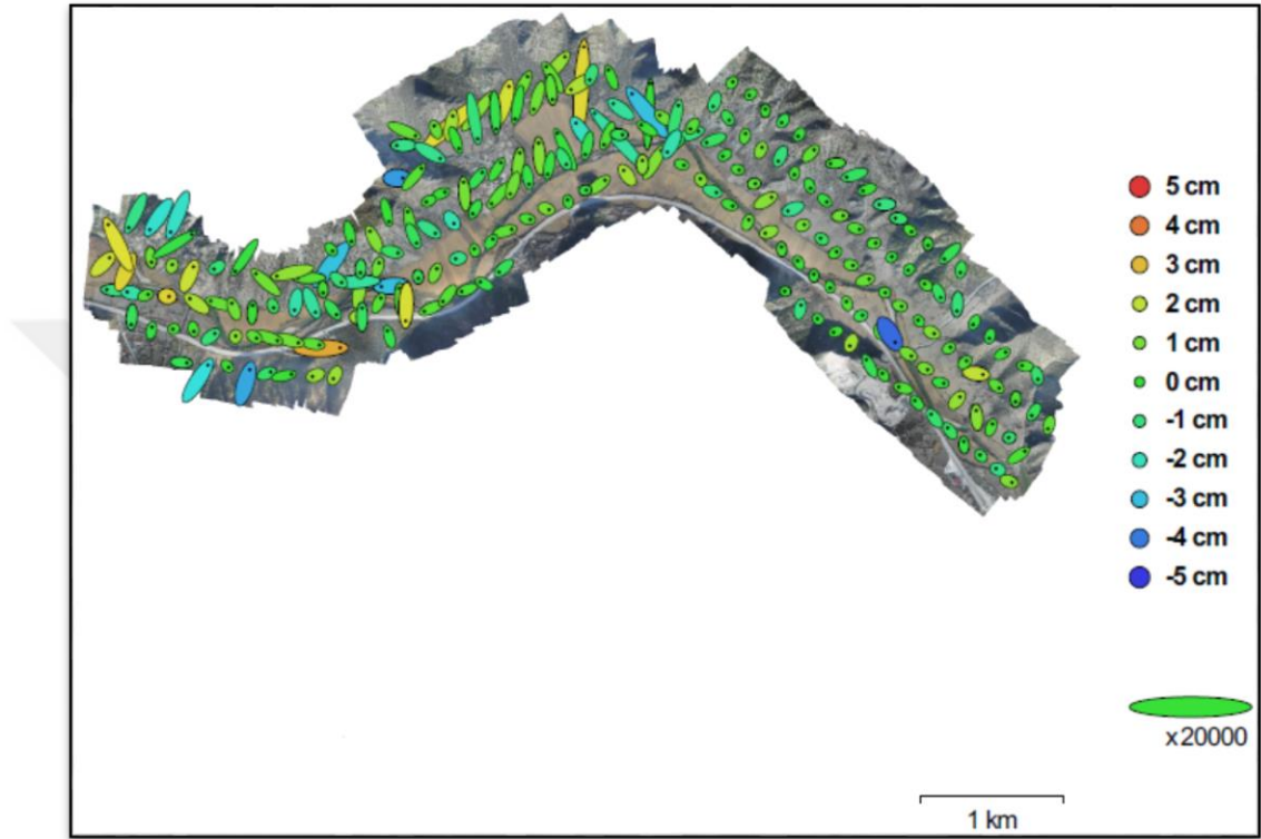
Şekil 3.26. Kamera yerleri ve hata tahminleri.
