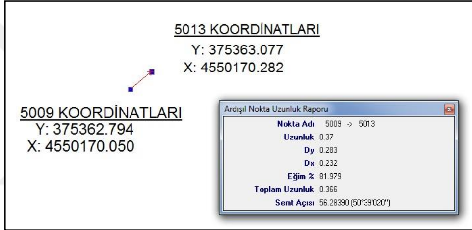
Şekil 4.7. Aynı doğrultuda detayın bir kaç kez ölçülmesi.
