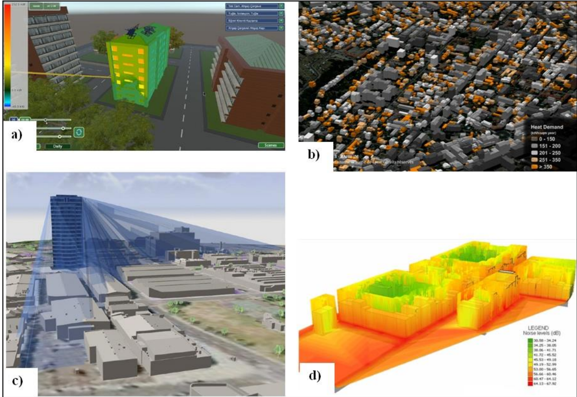
Şekil 1.6. 3B modeller ile yapılabilecek analizler. a) Güneşlenme süresinin analizi, b) Enerji tüketimi analizi, c) Kentsel nesnelere tarafından gölgelendirilen bölgelerin analizi, d) Gürültü kirliliği analizi (Biljecki vd., 2015).
