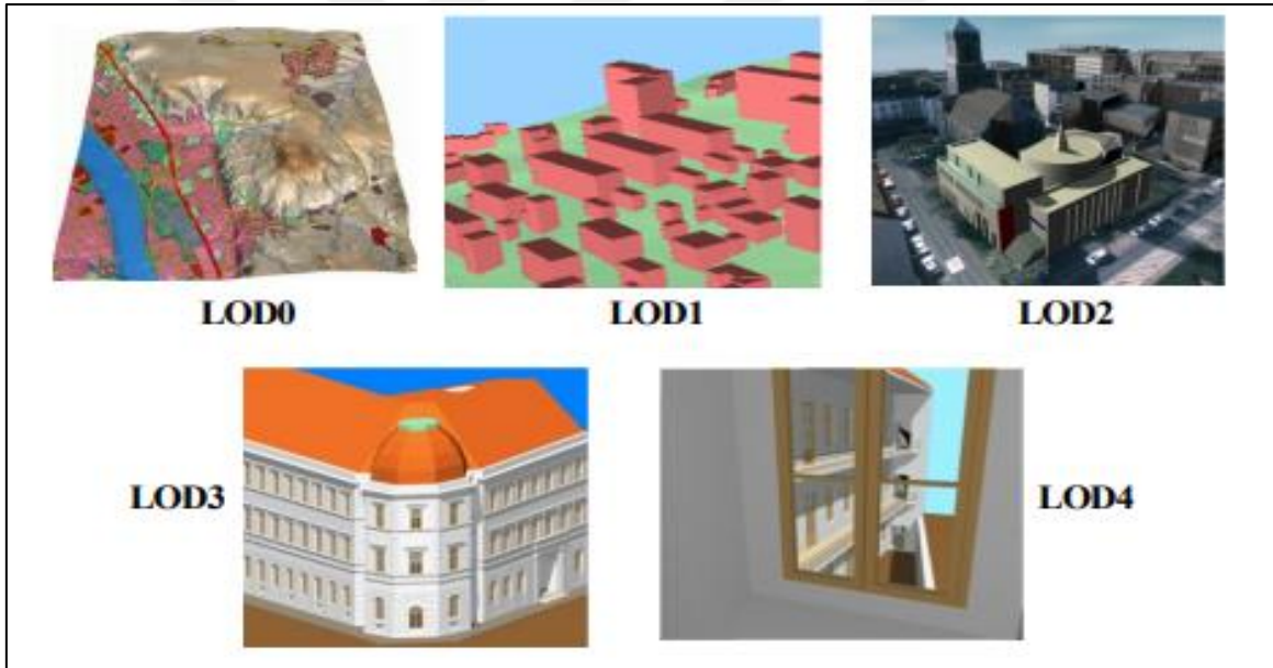
Şekil 2.11. CityGML tarafından tanımlanan beş ayrıntı seviyesi (OGC 12-019, (2012). City Geography Markup Language (CityGML) Encoding Standard, OGC.)
