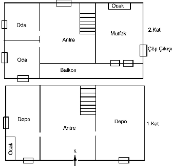
Şekil: 3.13 Topraktepe Köyü Karalar Mahallesi’nde İki Katlı Mesken Planı
