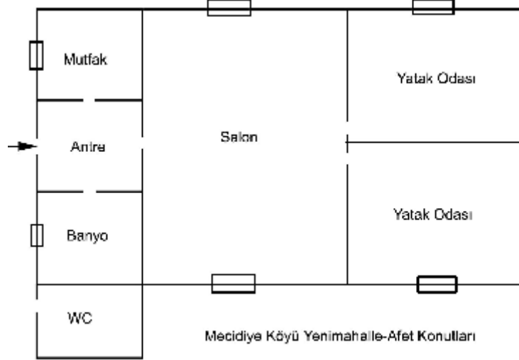
Şekil: 3.12. Mecidiye Köyü Yenimahalle'de Devlet Tarafından Yaptırılan Afet Konutları Planı
