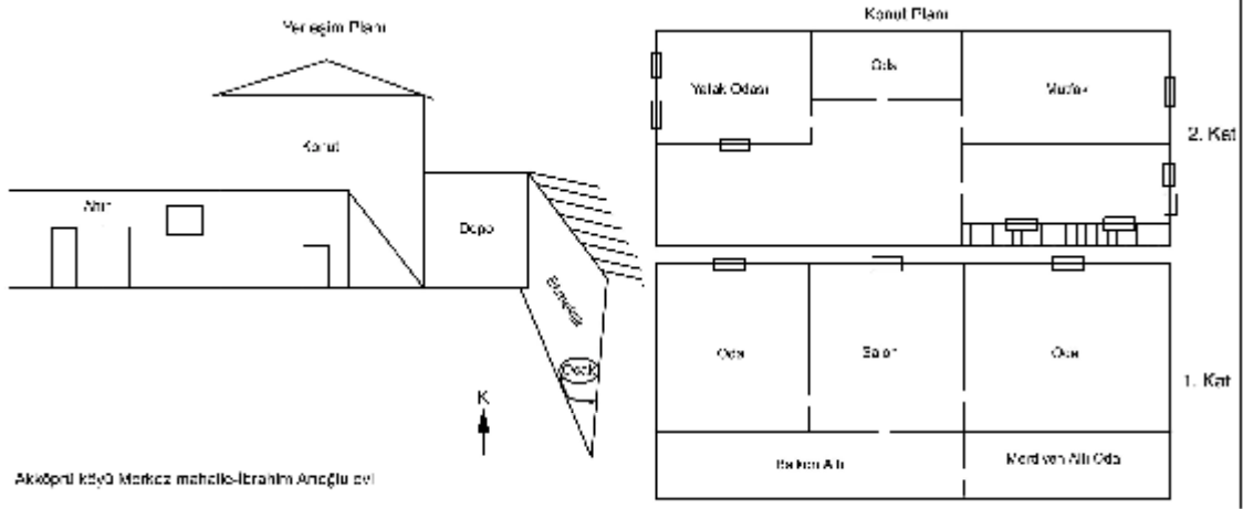
Şekil: 3.10. Akköprü Köyü Merkez Mahallede Bulunan İki Katlı Mesken Planı Örneği
