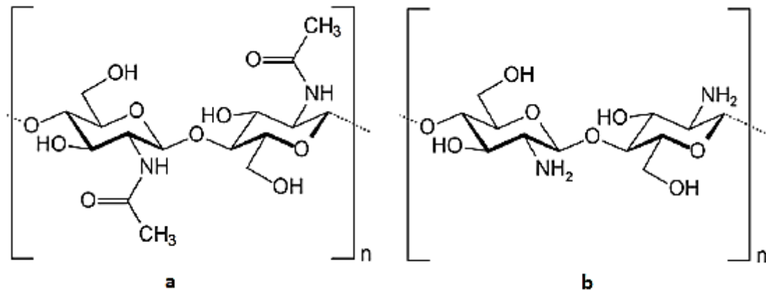
Şekil 2.1. Kitin (a) ve kitosan (b) kimyasal yapısı [8]
