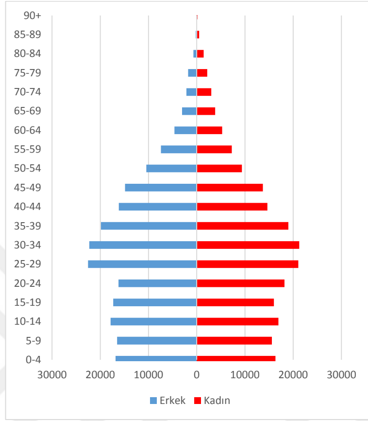
Şekil 15: Kâğıthane İlçesi 2010 Yılı Nüfus Piramidi
