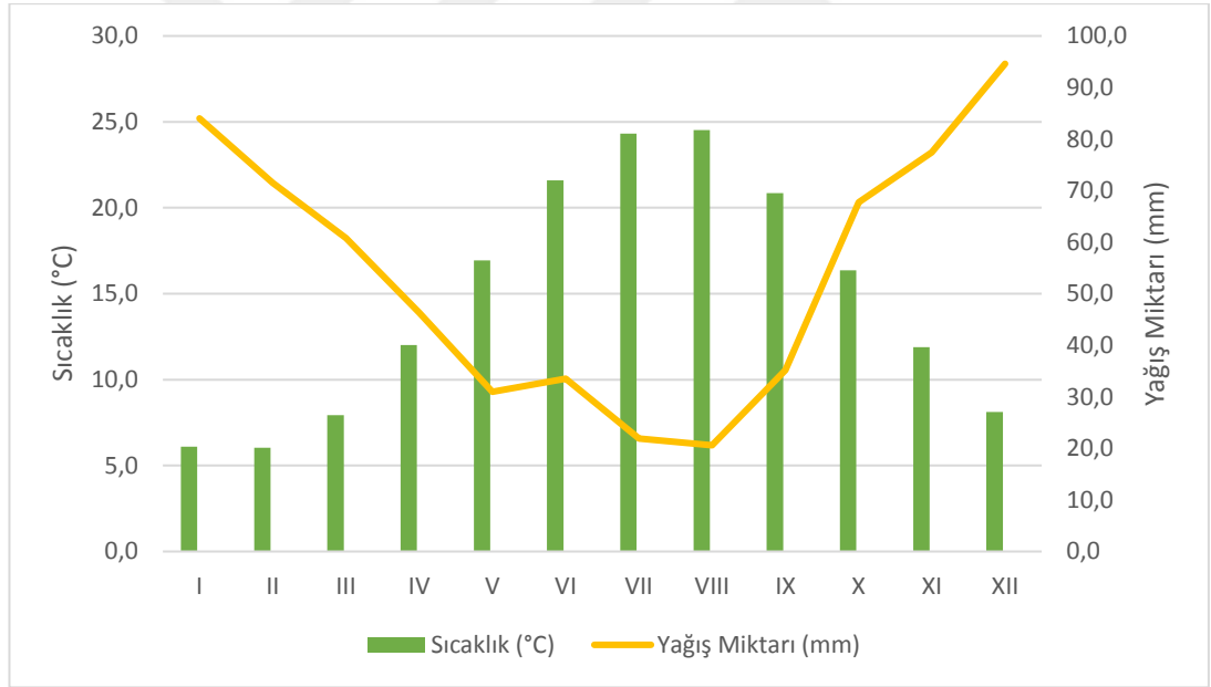
Şekil 2: Kâğıthane İlçesi'nde Sıcaklık ve Yağış Değerleri (1980 Ocak – 2021 Kasım)
