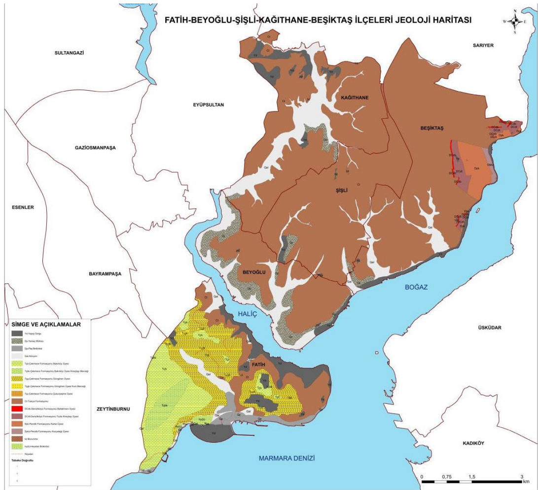
Harita 3: Fatih-Beyoğlu-Şişli-Kâğıthane-Beşiktaş İlçeleri Jeoloji Haritası
