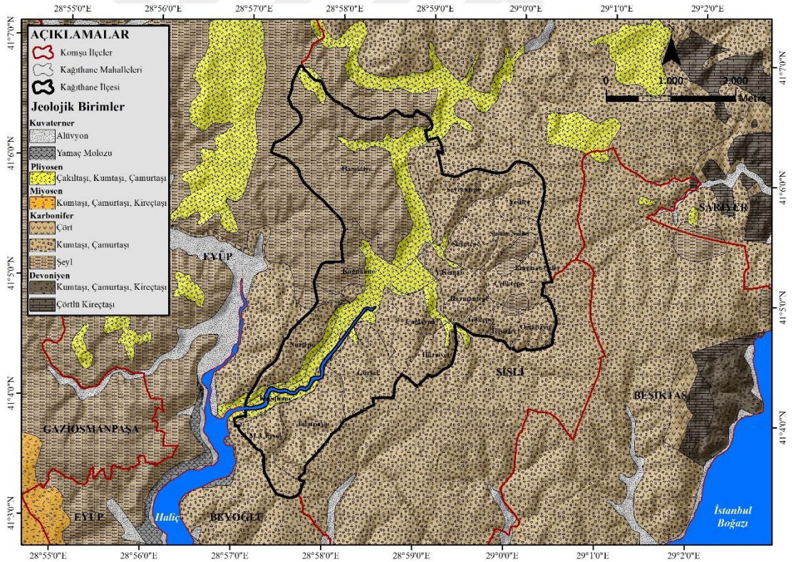
Harita 2: Kâğıthane İlçesi Jeoloji Haritası
