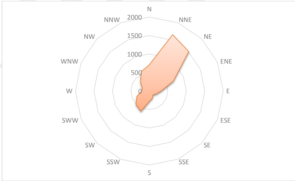
Şekil 11: Kâğıthane İlçesi'nin Hâkim Rüzgâr Yönü Diyagramı
