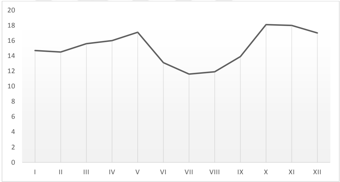
Şekil 4: Kâğıthane İlçesi’nde Bulutlu Günlerin Aylık Dağılışı (1980-2006)
