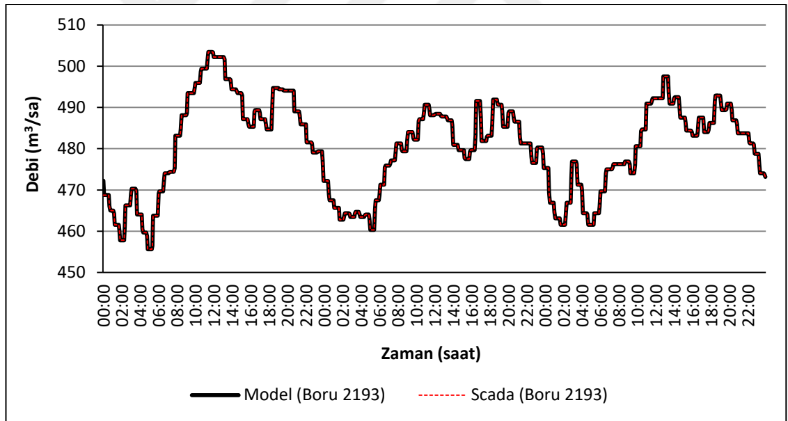
Şekil 4.25. Verifikasyon periyodunda Node 10198'in bağlı olduğu boru için model debi tahminleri ve SCADA ölçümlerinin karşılaştırması (Başlangıç Tarihi: 07.04.2011, Başlangıç Saati:00:00) MAE:0,013 m³/sa
