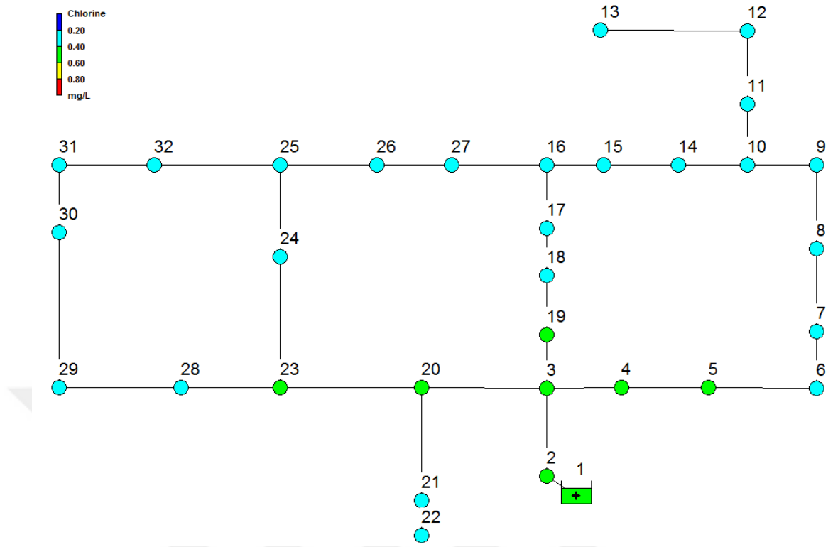
Şekil 2. Klor konsantrasyonlarının dağılımı, kaynak klor konsantrasyonu 0,5 mg/l (Saat 240:00)
