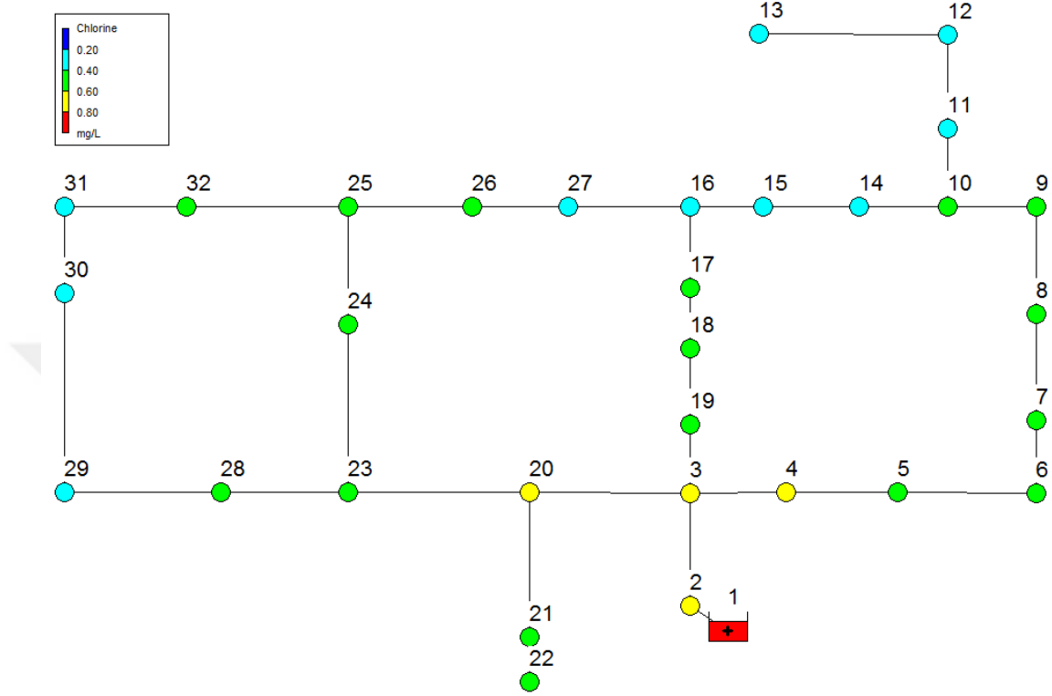
Şekil 12. Klor konsantrasyonlarının dağılımı, kaynak klor konsantrasyonu 0,8 mg/l (Saat 240:00)
