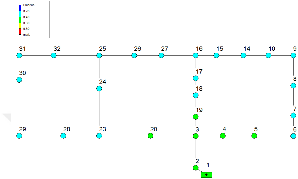
Şekil 14. Klor konsantrasyonlarının dağılımı, kaynak klor konsantrasyonu 0,5 mg/l (Saat 240:00)
