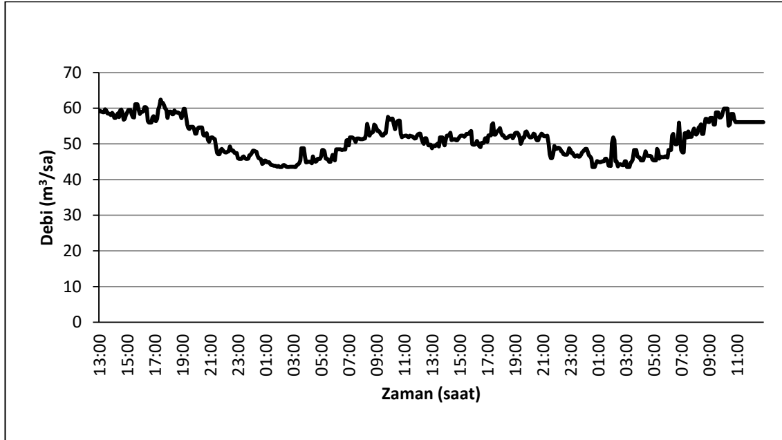
Şekil 2. Üçüncü kalibrasyon periyodu (KP 3) OKDMA debi grafiği (Başlangıç Tarihi: 19.04.2011, Başlangıç Saati:13:00)
