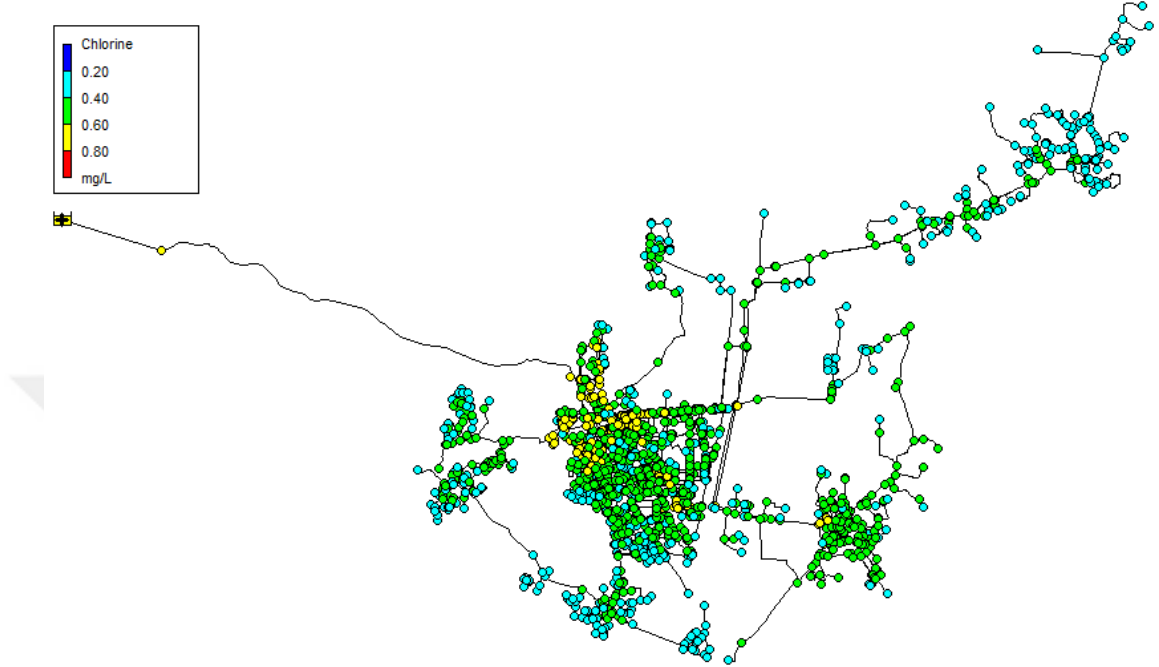
Şekil 4.70. Kaynak klor konsantrasyonu 0,7 mg/l için ara klor istasyonlarının yerleri ve klor dağılımı (Saat 240:00)
