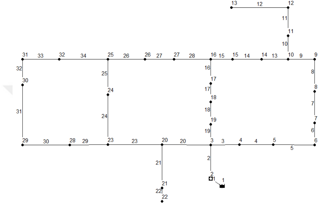
Şekil 1. Hanoi Şebekesi
