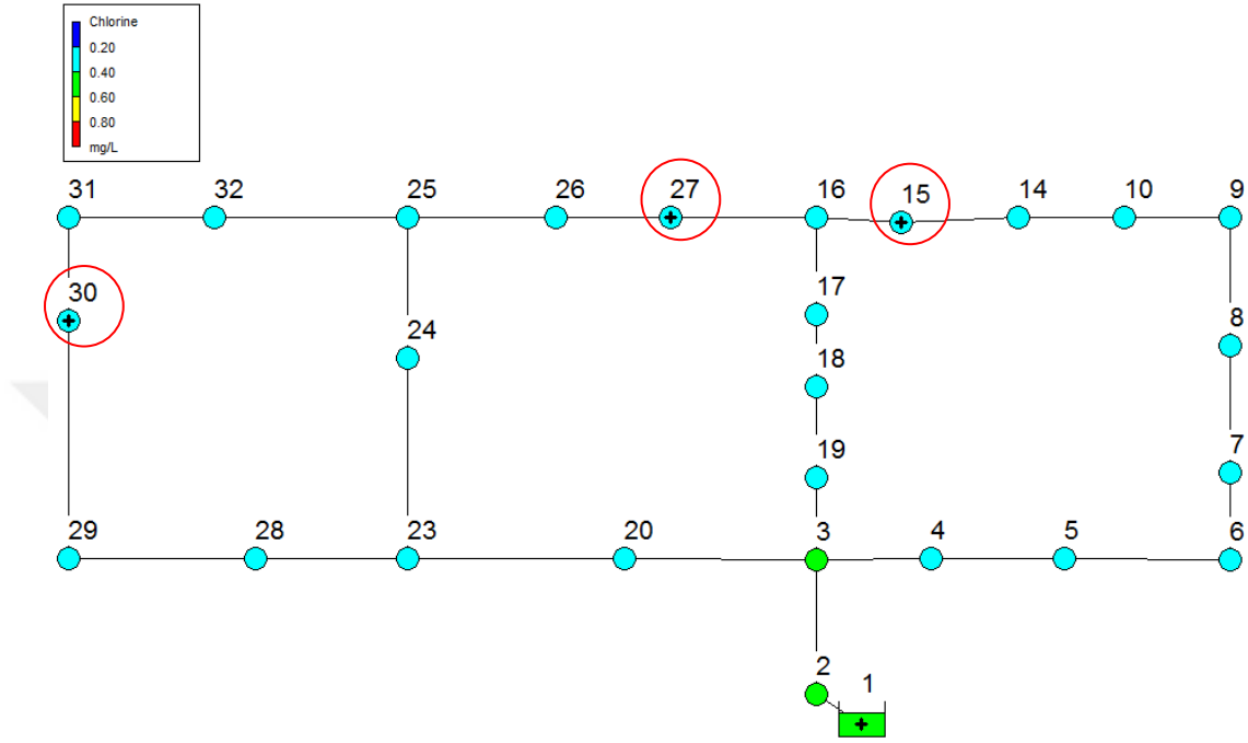
Şekil 16. Kaynak klor konsantrasyonu 0,5 mg/l için ara klor istasyonlarının yerleri ve klor dağılımı (Saat 240:00)
