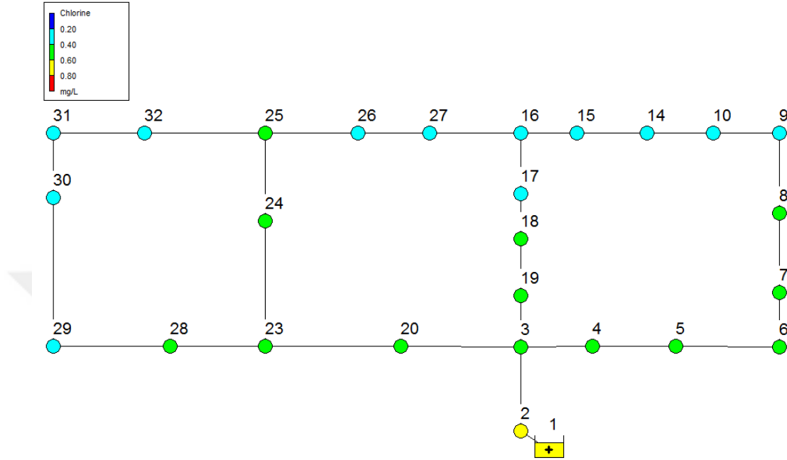
Şekil 19. Klor konsantrasyonlarının dağılımı, kaynak klor konsantrasyonu 0,7 mg/l (Saat 240:00)
