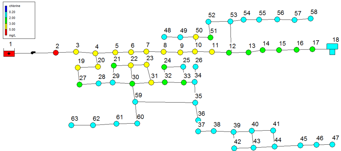
Şekil 9. Kaynakta 5 mg/l klor verildiğinde Sentetik Şebeke I'de klor dağılımı (Saat 101:30)
