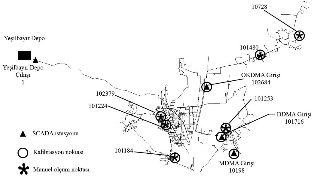
Şekil 3.13. Çalışma bölgesi için klor modeli kalibrasyon noktaları
