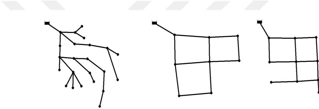
Şekil 2.1. İçme suyu şebeke yapıları a) Dal şebeke b) Ağ şebeke c) Ağ ve dal yapısında şebeke
