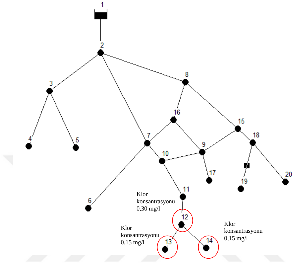
Şekil 3.16. Fiktif şebeke görünümü
