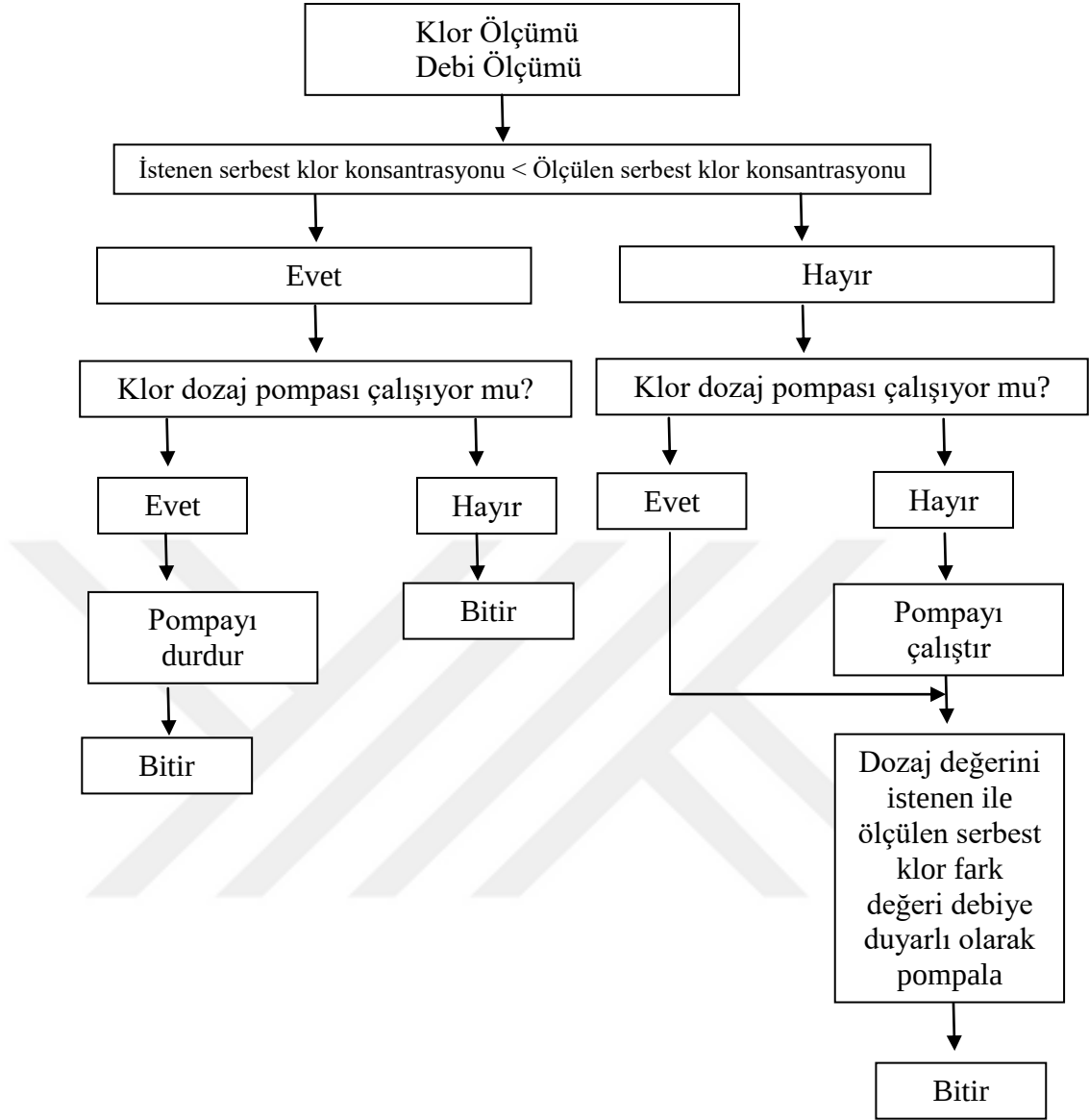
Şekil 4.79. Ara klor istasyonlarında klor dozaj pompasının çalıştırılması için bir algoritma örneği
