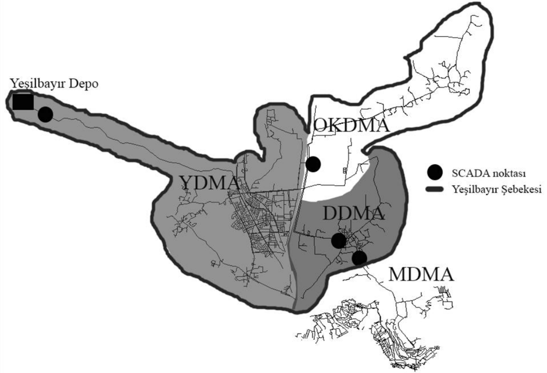
Şekil 3.4. Tez çalışmasında kullanılan SCADA istasyonları
