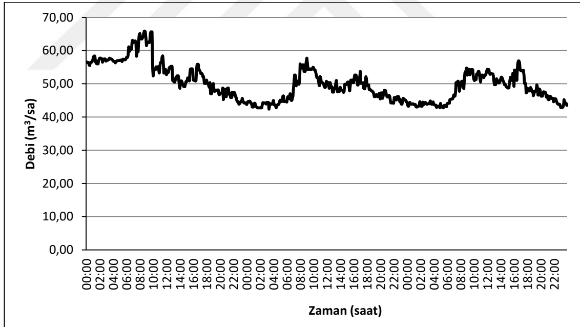
Şekil 4. Verifikasyon periyodu OKDMA debi grafiği (Başlangıç Tarihi: 07.04.2011, Başlangıç Saati:00:00)
