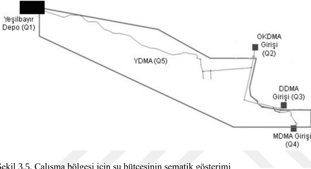
Şekil 3.5. Çalışma bölgesi için su bütçesinin şematik gösterimi
