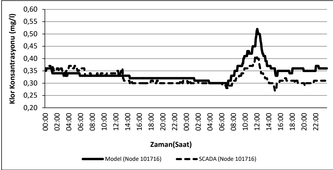
Şekil 4.44. KKP2 Duacı Girişi (Node 101716) ölçüm noktasında serbest klor ölçümleri ve model tahminleri(Başlangıç Tarihi: 05.05.2011, Başlangıç Saati:00:00) MAE:0,028 mg/l
