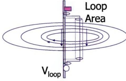
Şekil 6.8. Kalkan eklenmiş kablonun gösterimi [46]
