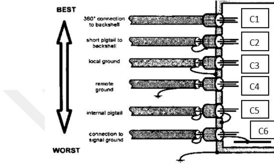
Şekil 11.1. EMU mühendisliği açısından farklı kalkan sonlandırma yöntemlerinin genel değerlendirmesi
