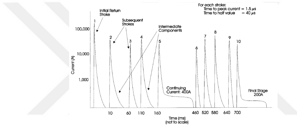
Şekil 3.4. Negatif yıldırım darbesinin dalga formu modeli [30]
