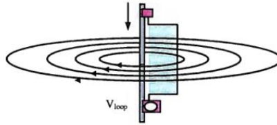
Şekil 6.5. Kablunun iki noktadan bağlı olduğu durumda indüklenen manyetik akı [46]
