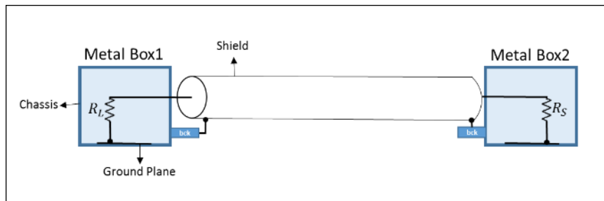
Şekil 13.1. Konfigürasyon 1
