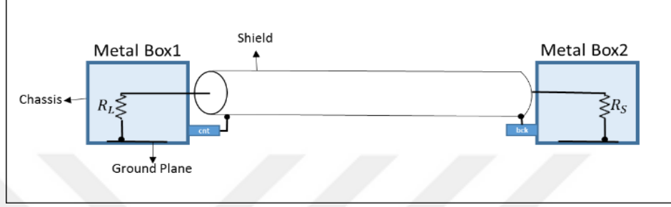
Şekil 13.2. Konfigürasyon 2
