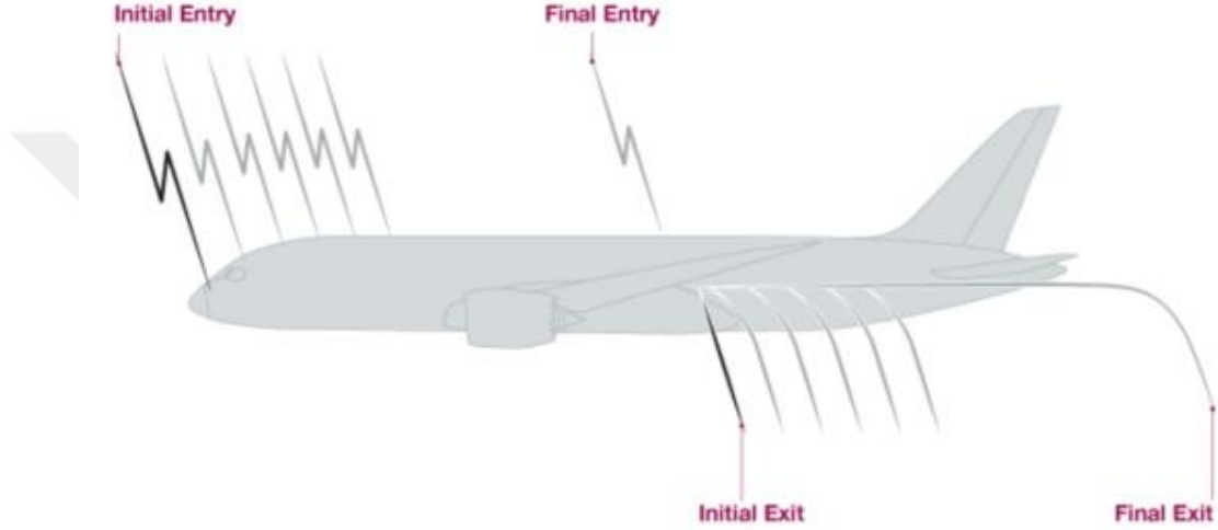
Şekil 4.5. Uçak üzerindeki süpürülmüş kanal tutunma noktalarının tipik gösterimi [39]
