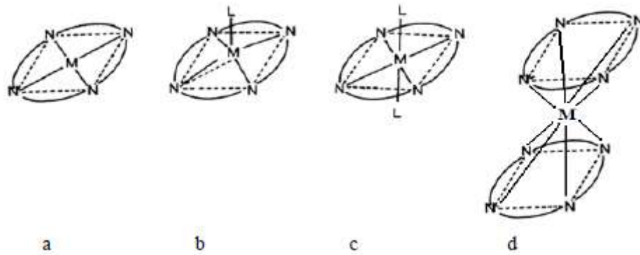
Şekil 2.4. Ftalosiyanın molekülünün geometrik yapısının şematik gösterimi
