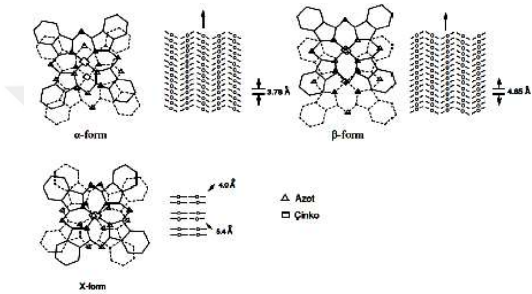
Şekil 2.5. Metallo ftalosiyaninlerin kristal yapısının geometrik gösterimi
