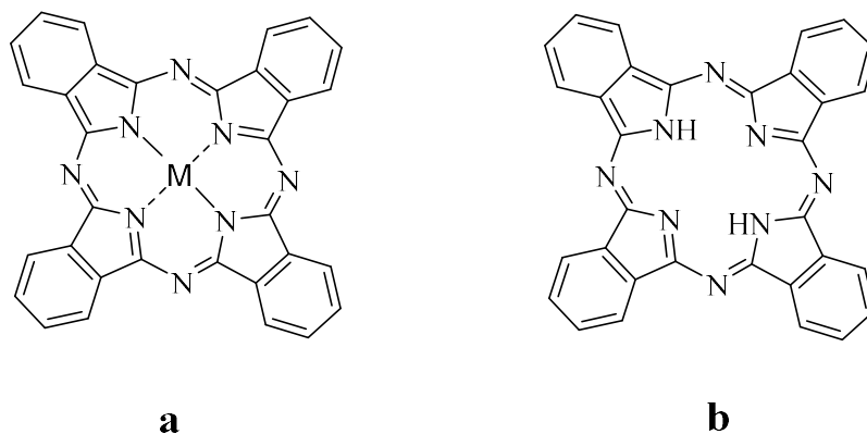
Şekil 2.2. a) Metallsız ftalosiyenin, b) Metalli ftalosiyenin
