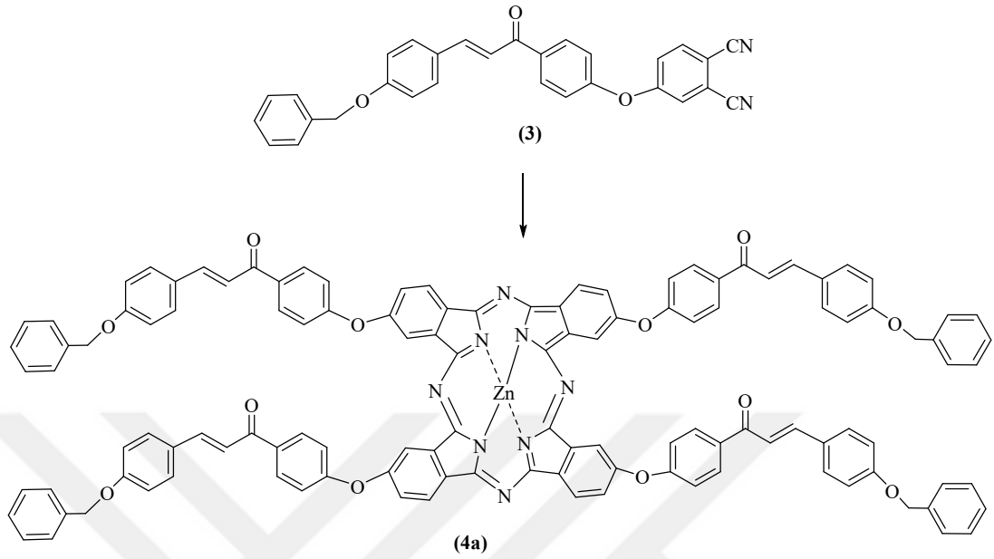
Şekil 3.4. 4a nolu bileşiğin sentezi
