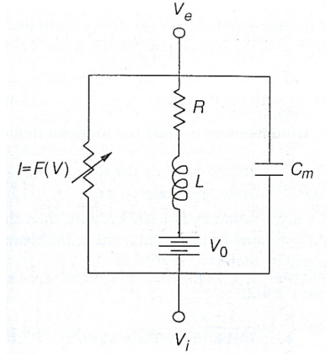
Şekil 3.3 FHN modeli hücre zarı elektriksel eşdeğer devresi.
