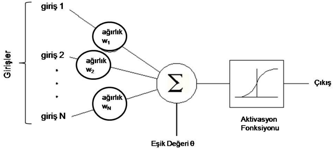
Şekil 2.13 Perseptron yapısı.
