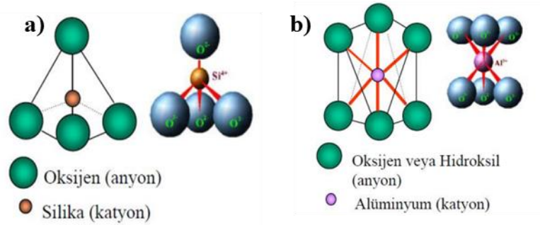
Şekil 3.1. Oktahedral ve tetrahedral yapı (Hancıoğlu, 2015)
