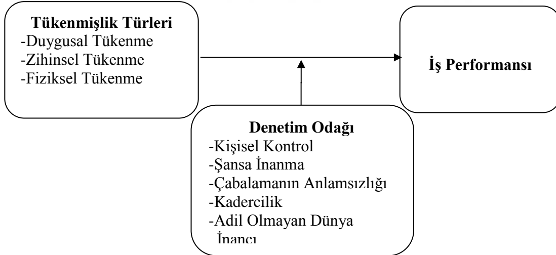
Şekil 2.1. Araştırmanın Modeli
