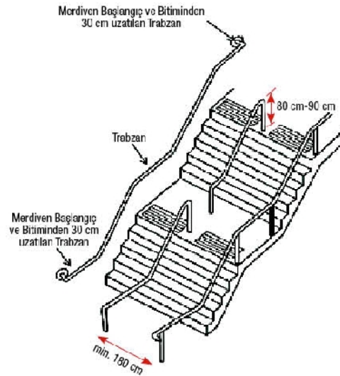
Şekil 2.5. Merdiven Ölçüleri
