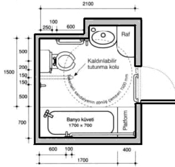
Şekil 2.15. Özürllüler İçin WC-Banyonun Bir Arada Olması Durumunda Gerekli Alanlar(39)
