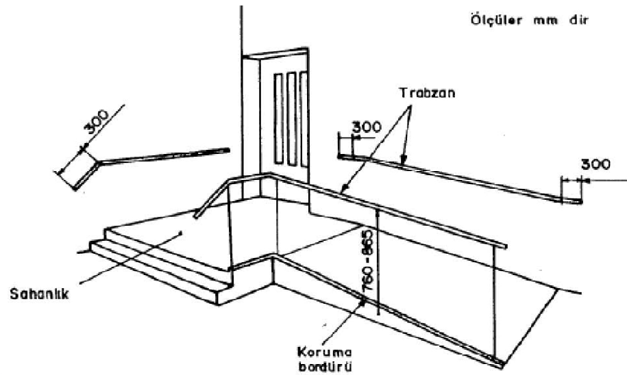
Şekil 2.4. Bina Giriş Rampası
