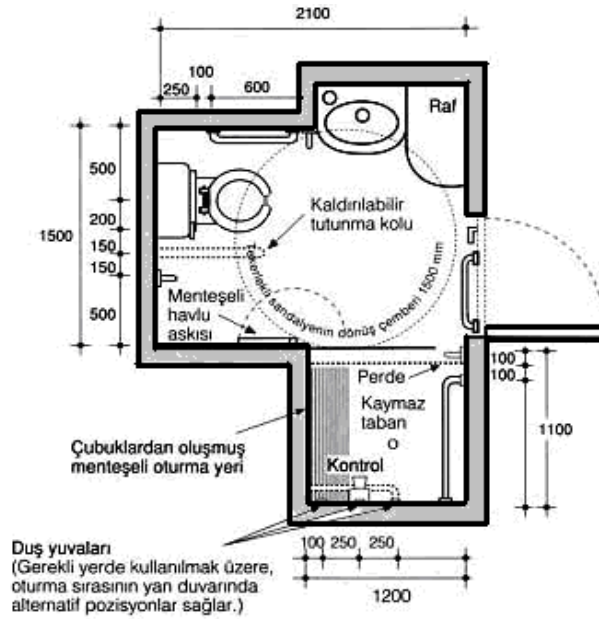
Şekil 2.16. Özürllüler İçin WC-Banyo Bir Arada Düzenlenmiş Alanlar (39)
