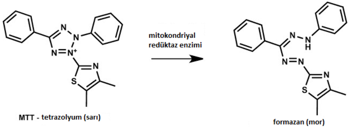
Şekil 3-MTT yapısında tetrazolyum tuzlarının formazan kristallerine dönüşmesinin şematik gösterimi.
