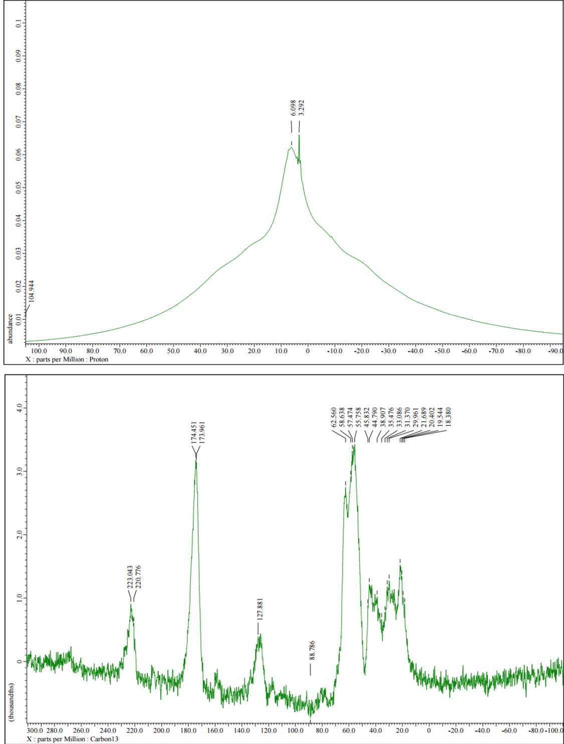
Şekil 4-23 Serisin partiküllerinin a) 1 H-NMR ve b) 13 C-NMR Spektrumları
