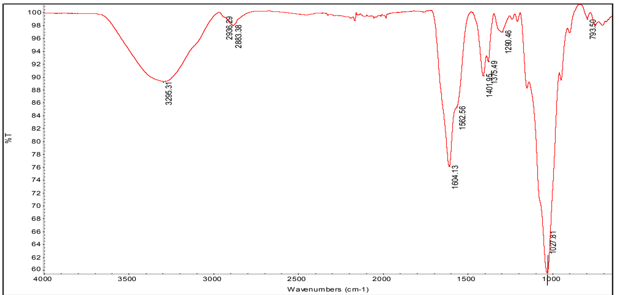
Şekil 4-14 Hyaluronik asit (HA) FTIR spektrumu
