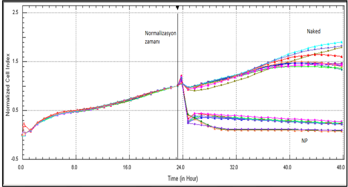
Şekil 4-47 HEp-2 hücrelerinin proliferasyonu üzerine tüm test numunelerinin (ASHL2, CSKN, CD1, NASHL2, NCSKN, NCD1 siRNA) ve tüm konsantrasyonlarının 24 saatlik etkisinin normalize hücre indeksi ile gösterilmesi (Normalizasyon zamanı; 23:18:20)
