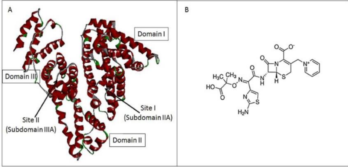
Şekil 2-2 Albuminin kimyasal yapısı ve domainleri
