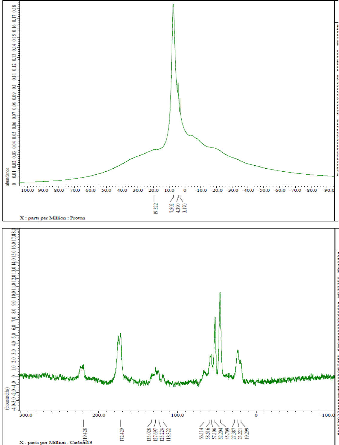
Şekil 4-19 Fibroin nanopartiküllerin a) 1 H-NMR ve b) 13 C-NMR Spektrumları
