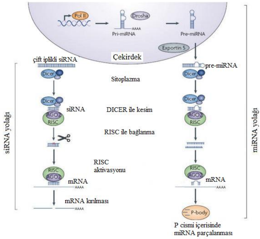
Şekil 2-1 miRNA ve siRNA yolları [48]
