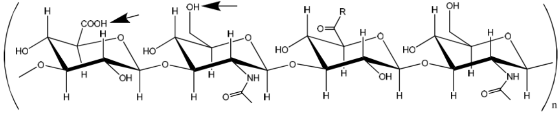
Şekil 2-6 Hyalüronik Asitin kimyasal yapısı
