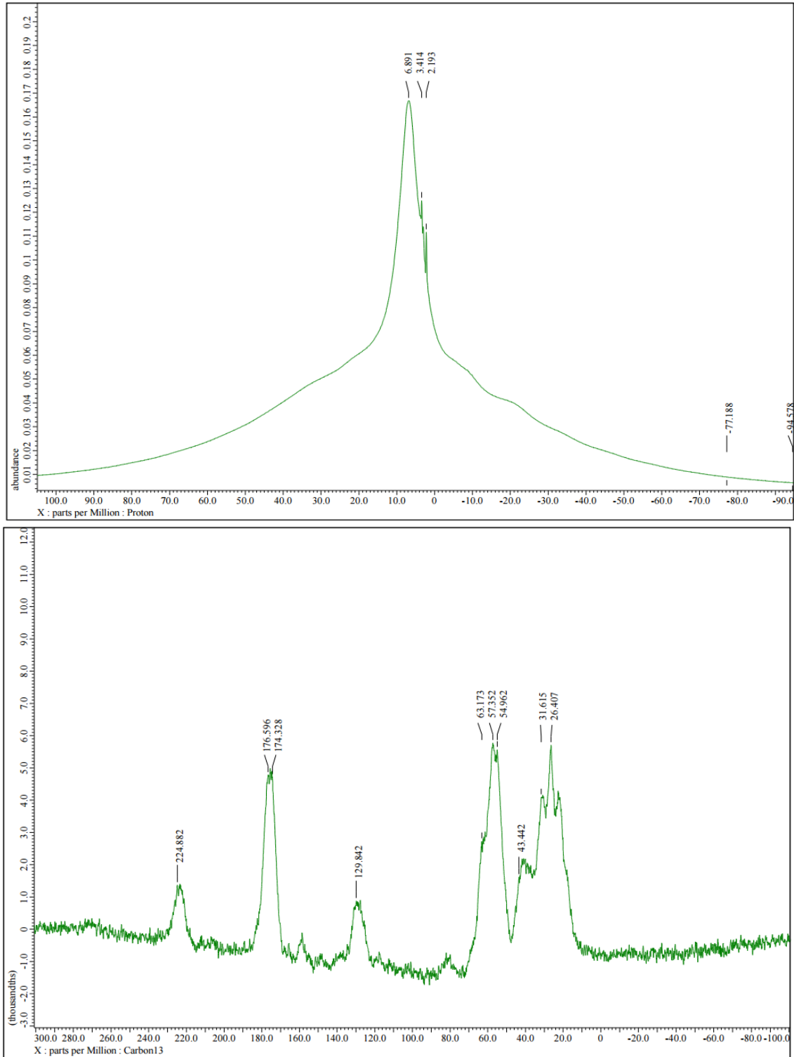
Şekil 4-24 Alb-Ser(1:1 w/w) partiküllerinin a) 1 H-NMR ve b) 13 C-NMR Spektrumları
