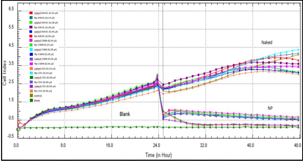
Şekil 4-61 HEp-2 hücrelerinin proliferasyonu üzerine nanopartiküllü ve nanopartikülsüz siRNA test numunelerinin ve tüm konsantrasyonlarının 24 saatlik etkisinin 21. saatten itibaren normalize hücre indeksi ile gösterilmesi (Normalizasyon zamanı; 23:18:20)
