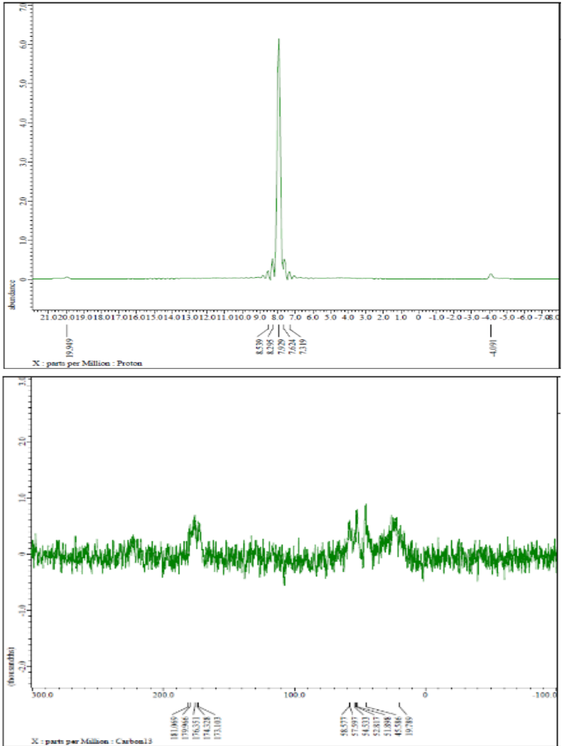
Şekil 4-22 Alb-fib (1:2 w/w) partiküllerinin a) ^1\text{H} -NMR ve b) ^{13}\text{C} -NMR Spektrumları
