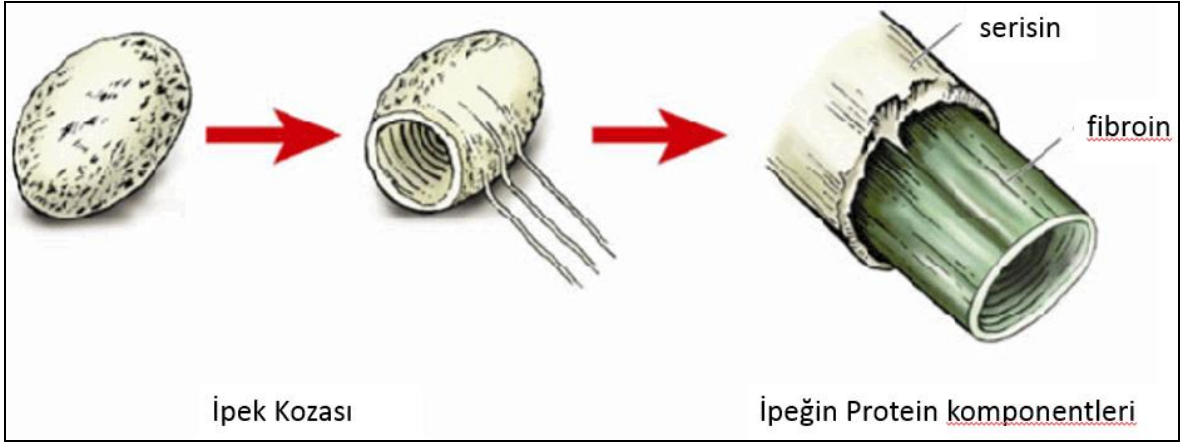
Şekil 2-3 İpek Proteinleri fiziksel yapısı
