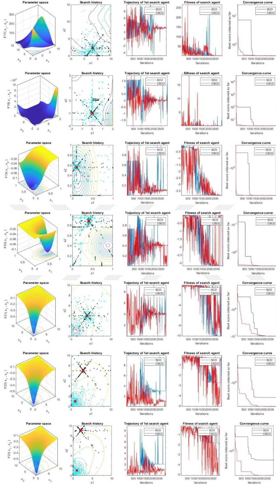
Şekil 3.1. SCO ve CSCO Algoritmalarının Analiz Sonuçları: Parametre Uzaklı, Search history: Arama Geçmişi, Trajectory of 1 st Agent: Aday Çözümlerin Yörüngesi, Fitness of Search Agent: Aday Çözümlerin Uygunluğu, Convergence Curve: Yakınsama Eğrisi
