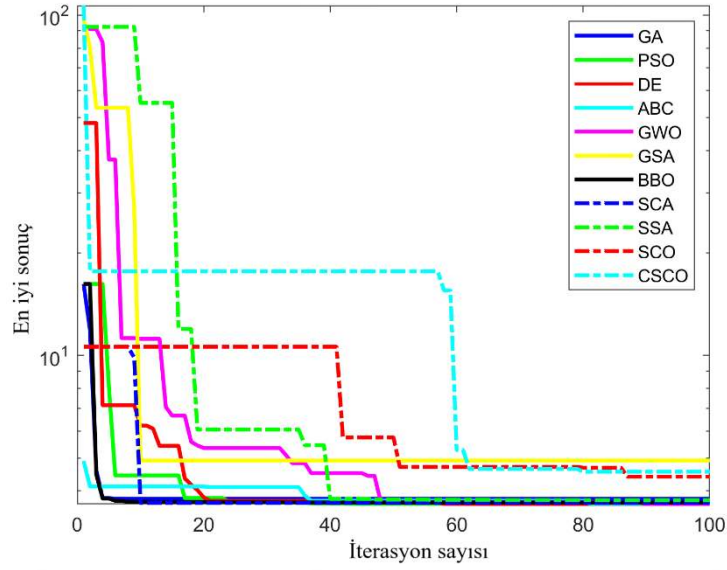
Şekil 3.3. Sıkıştırma Yayı Tasarım Problemi İçin CSCO ve Sezgisel Yöntemlerin Karşılaştırılması
