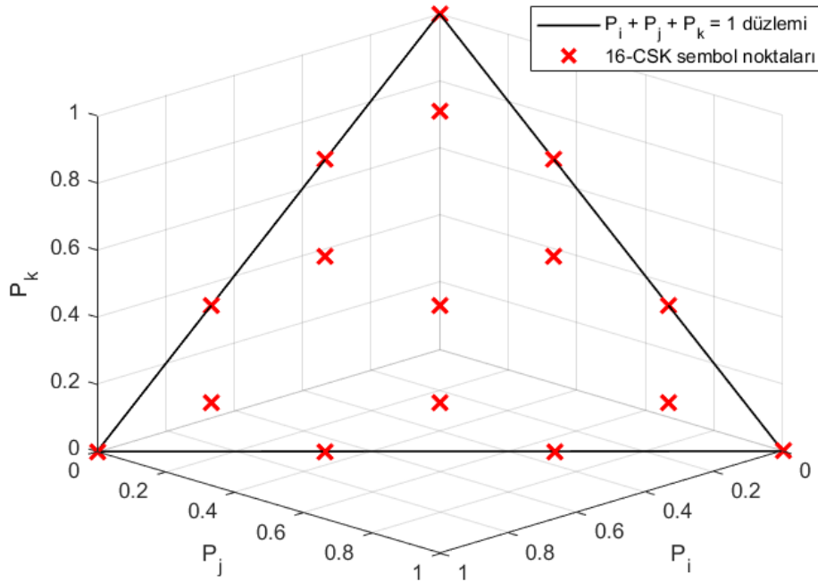
Şekil 1.3. 16-CSK modülasyonu sembol noktaları
