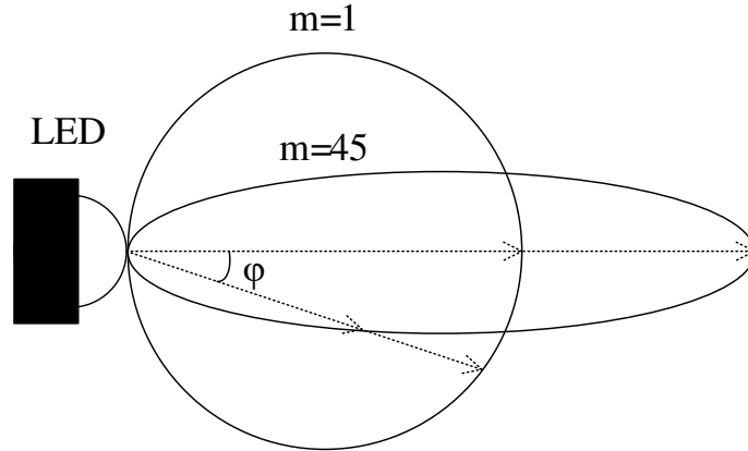
Şekil 1.5. Lambert indeksine göre ışıma şekli
