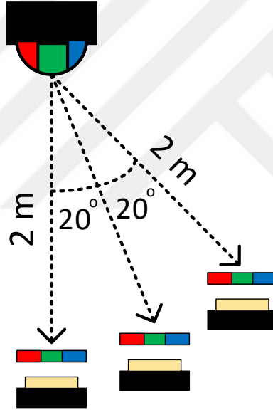
Şekil 2.1. Tek verici LED kullanılan model
