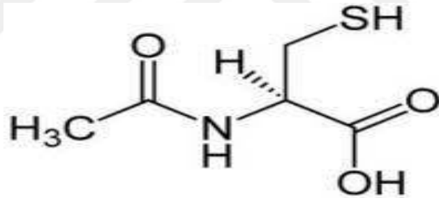
Şekil-36: N-asetil sisteinin kimyasal yapısı
