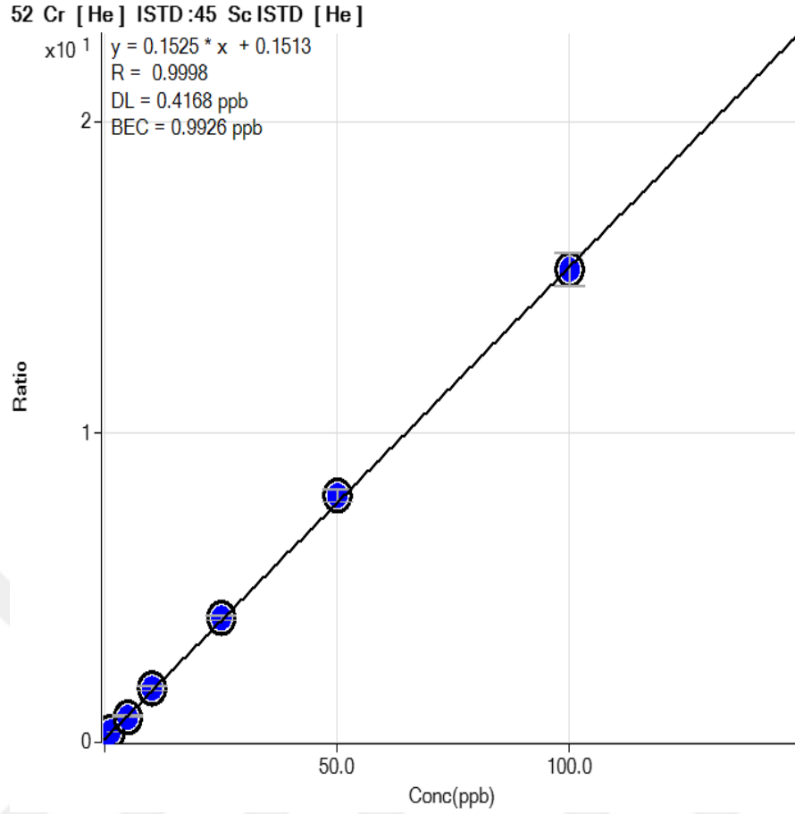
Şekil-61: Krom elementi için yapılan altı farklı standart çözeltiyle hazırlanan kalibrasyon grafiği
