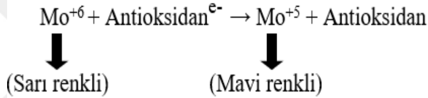
Şekil-44: Molibdenyumun antioksidan tarafından indirgenmesi sonucu oluşan renk değişikliği
