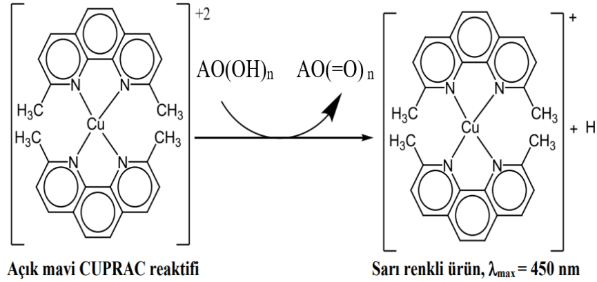
Şekil-48: CUPRAC Yönteminde \text{Cu}^{+2} -Nc reaktifinin antioksidanlarla ( \text{AO}(\text{OH})\text{N} ) reaksiyonu neticesinde sarı renkli \text{Cu}^{+1} -Nc'in oluşumu (764)
