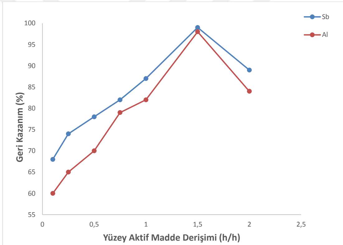
Şekil 5.3. Yüzey aktif madde derişiminin metal iyonlarının geri kazanım yüzdelere olan etkisi.
