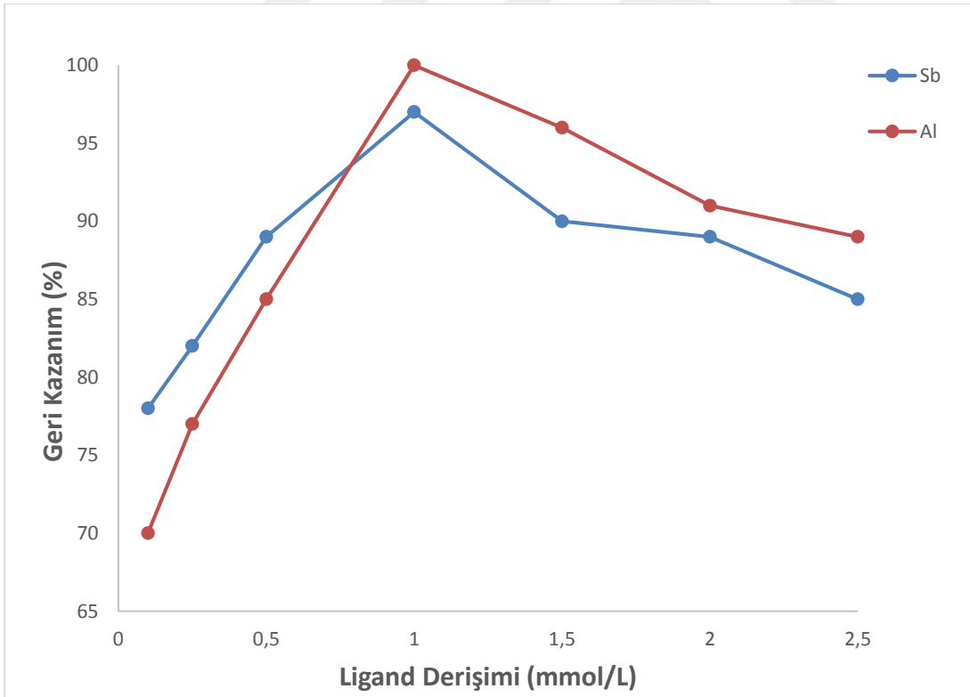
Şekil 5.2. Ligand derişiminin metal iyonlarının geri kazanım yüzdelere olan etkisi.
