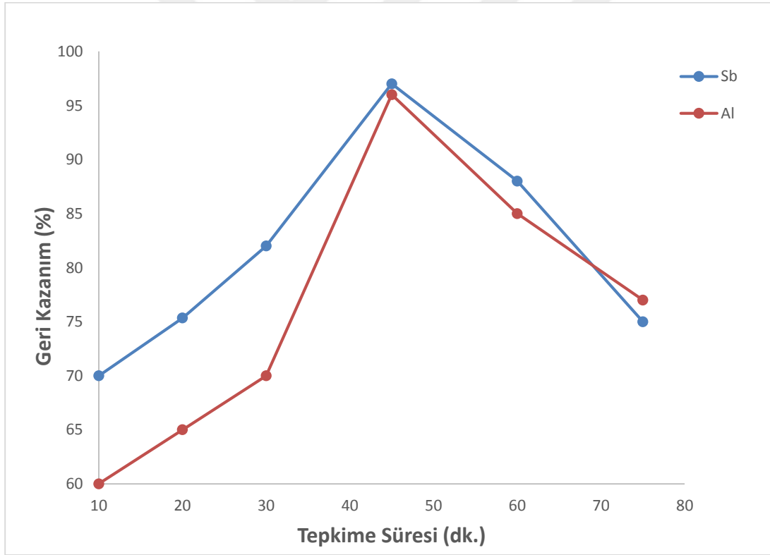
Şekil 5.4. Tepkime süresinin metal iyonlarının geri kazanım yüzdelere olan etkisi.
