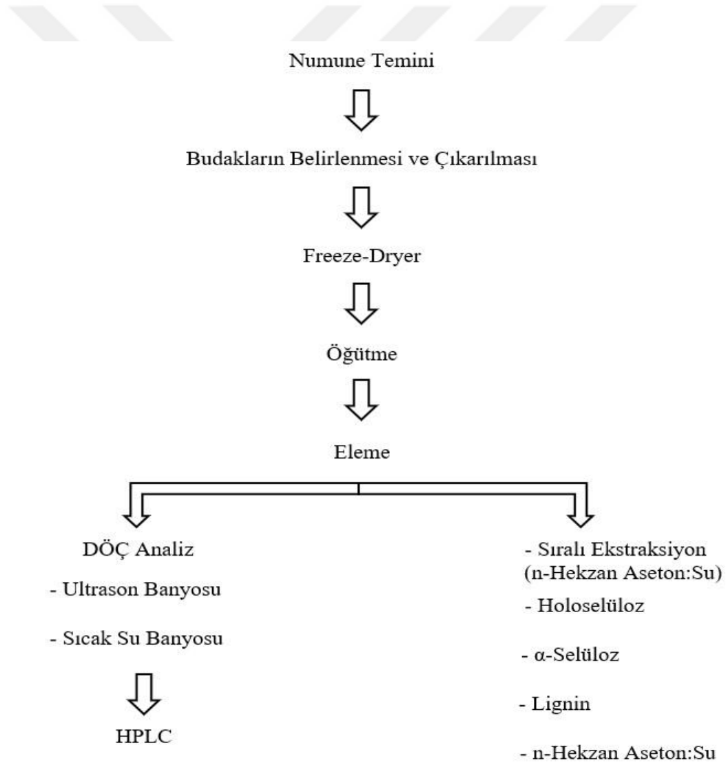
Şekil 3.3: Karaçam budaklarına ait deney akış şeması
