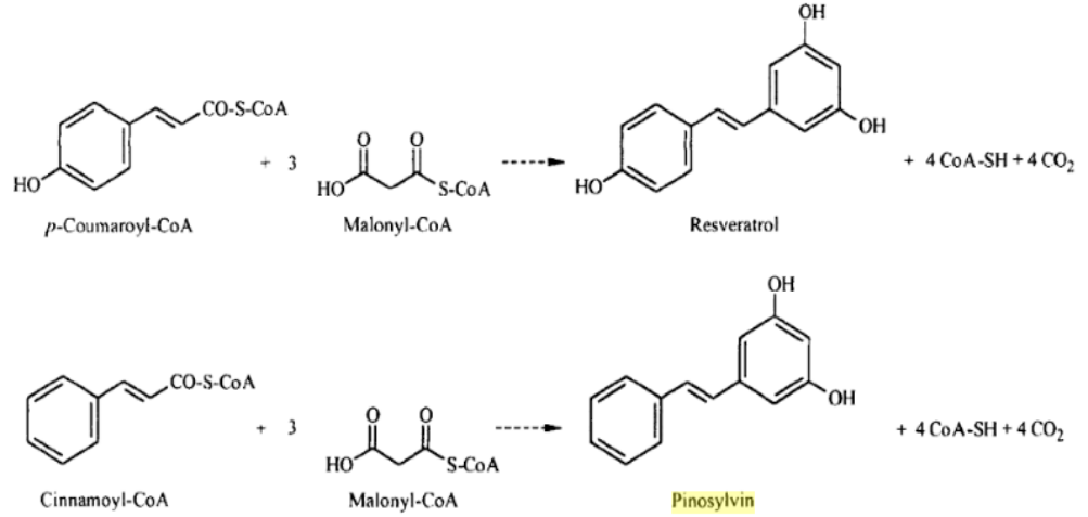
Şekil 1.6: Pinosilvin sentezine ait reaksiyon zinciri. (Nisula ,2003)
