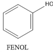
Şekil 1.4: Bir fenol ünitesine ait kimyasal yapı.
