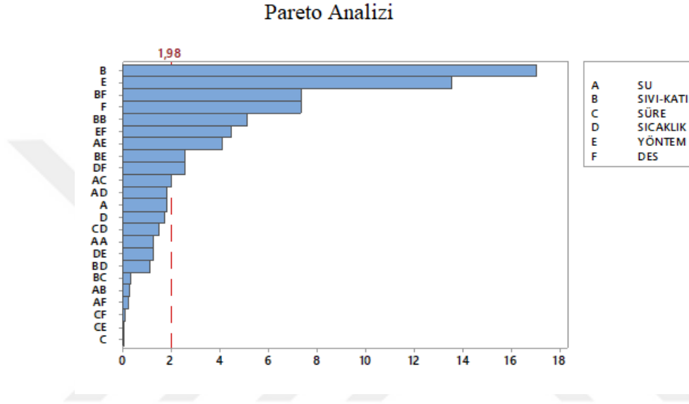
Şekil 4.14: Pareto Analizi
