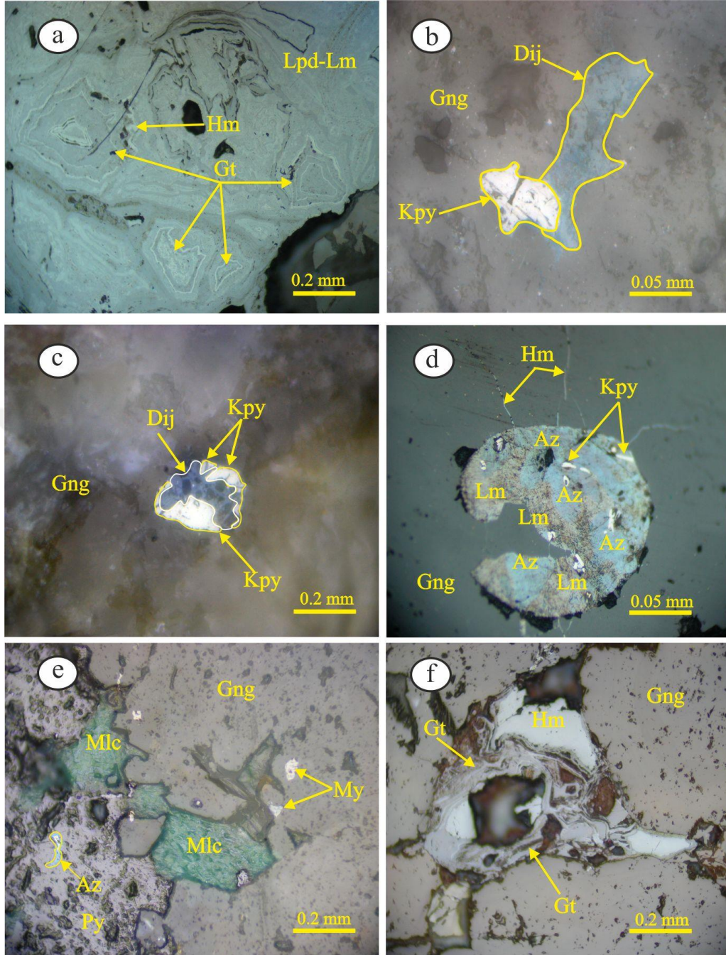
Şekil 3.30. İkincil cevher minerallerinin mikroskoftaki görünüşleri a) Hematitleşmiş manyetitler üzerinde konsantrik halkalar şeklinde götit ve lepidokrozit-limonit oluşumları (Örn. No.: 20-M), b) Kalkopirit etrafında gelişen dijenitler (Örn.No.: 20), c) Kalkopiritin içinde dijenit oluşumu (Örn.No.:20), d) Manyetit tanesi üzerinde hematit damarcıkları, limonit ve azurit ile birlikte küçük kalkopiritler (Örn. No.: S-47.1), e) Düzensiz şekilli piritler üzerinde ve kırıklarda malakit, azurit, hematit oluşumları (Örn. No.: 20), b), f) Gangın kırıklarında hematitten gelişen götit oluşumları (Örn. No.: 21-F). Gt: Götit, Lm: Limonit, Lep: Lepidokrozit, Hm: Hematit, Dij: Dijenit, Kpy: Kalkopirit, Gng: Gang, Mlc: Malakit, Az: Azurit
