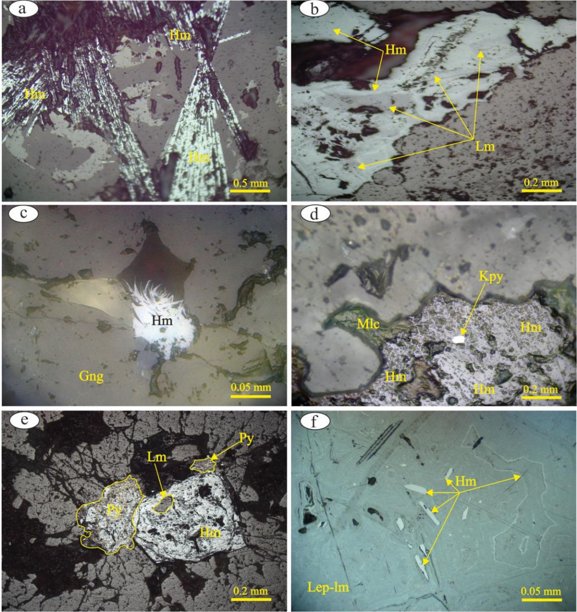
Şekil 3.25. Hematitin cevher mikroskobisindeki görünümleri. a) İğnemsu çubuksu spekülarit hematit lataları (Örn. No.: 26), b) Yarı özşekilli – düzensiz şekilli geniş yüzeyli hematit taneleri (Örn. No.: 21-E), c) Gang içerisinde tüy dokusu gösteren limonitleşmiş hematit (Örn. No.: 21-E), d) Öz şekilsiz hematit tanesi üzerinde kalkopirit ve malakit oluşumları (Örn. No.: 20), e) Öz şekilsiz ve yarı öz şekilli pirit taneleri üzerinde limonitle birlikte hematit oluşumu (Örn. No.: 20), f) konsantrik halkalar şeklinde gelişen hematit oluşumları (Örn. No.: 20-M). Hm: Hematit, Lm: Limonit, Kpy: Kalkopirit, Mlc: Malakit, Py: Pirit, Lep: Lepidokrozit
