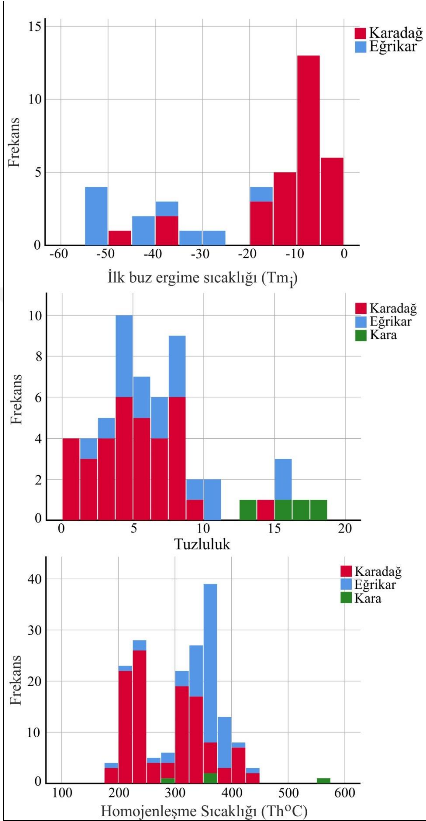
Şekil 4.7. Karadağ Fe-Cu skarn yatağı, Eğrikar Fe-Cu skarn yatağı ve Kara Fe skarn yatağının; İlk buz ergime (T m ), tuzluluk ve homojenleşme sıcaklık (Th °C) değerleri
