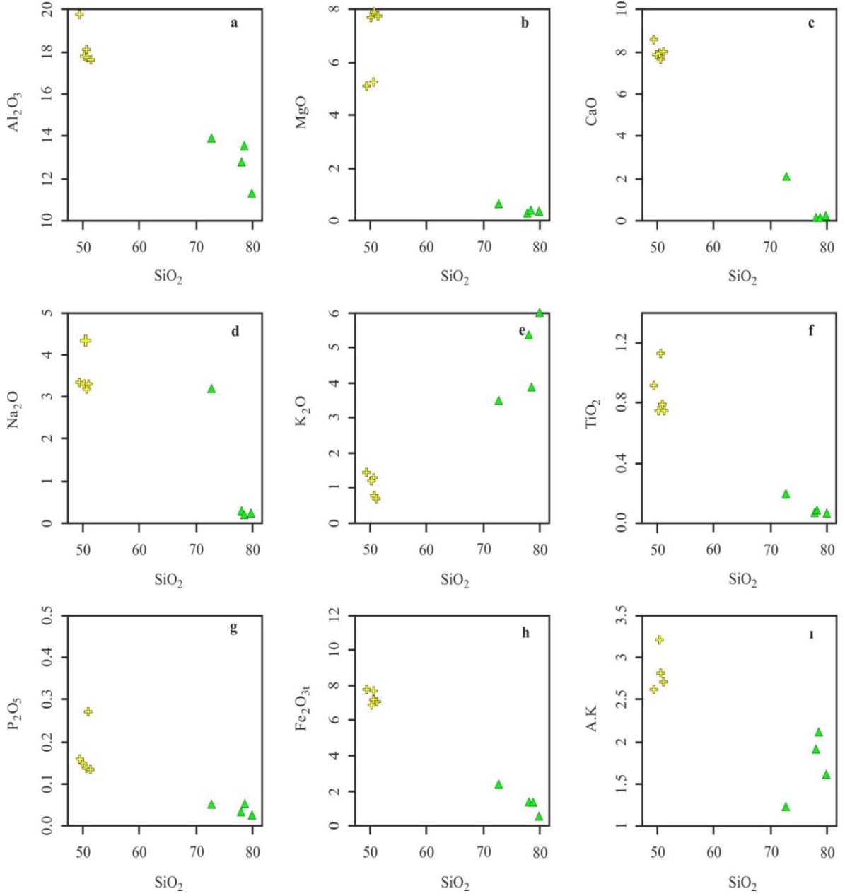
Şekil 3.16. Karadağ Fe-Cu skarn cevherleşmesindeki granitoidik kayaç örneklerinin SiO 2 'ye karşı ana oksit değişim diyagramları (semboller için Şekil 3.15a'ya bakınız).
