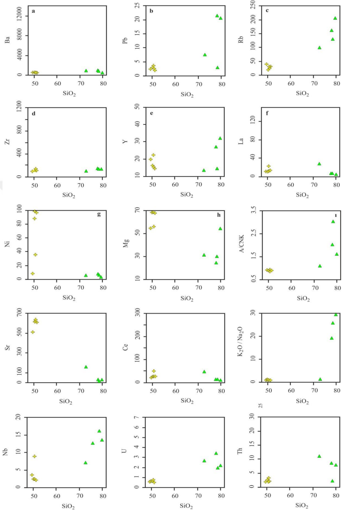
Şekil 3.17. Karadağ Fe-Cu skarn cevherleşmesindeki granitoidik kayaç örneklerin SiO 2 'ye karşı iz element değişim diyagramları (semboller için Şekil 3.15a'ya bakınız).
