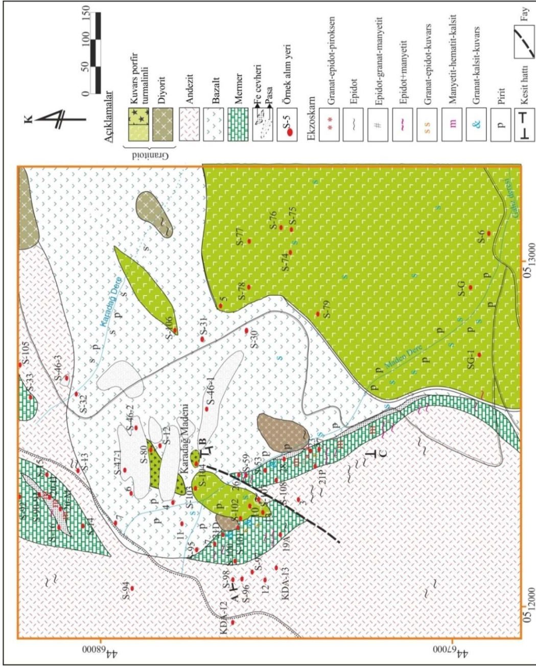
Şekil 3.2. İnceleme alanının jeolojik haritası, Karadağ Fe- Cu skarn cevherleşmesi ve skarn mineral birlikteliklerini gösteren harita
