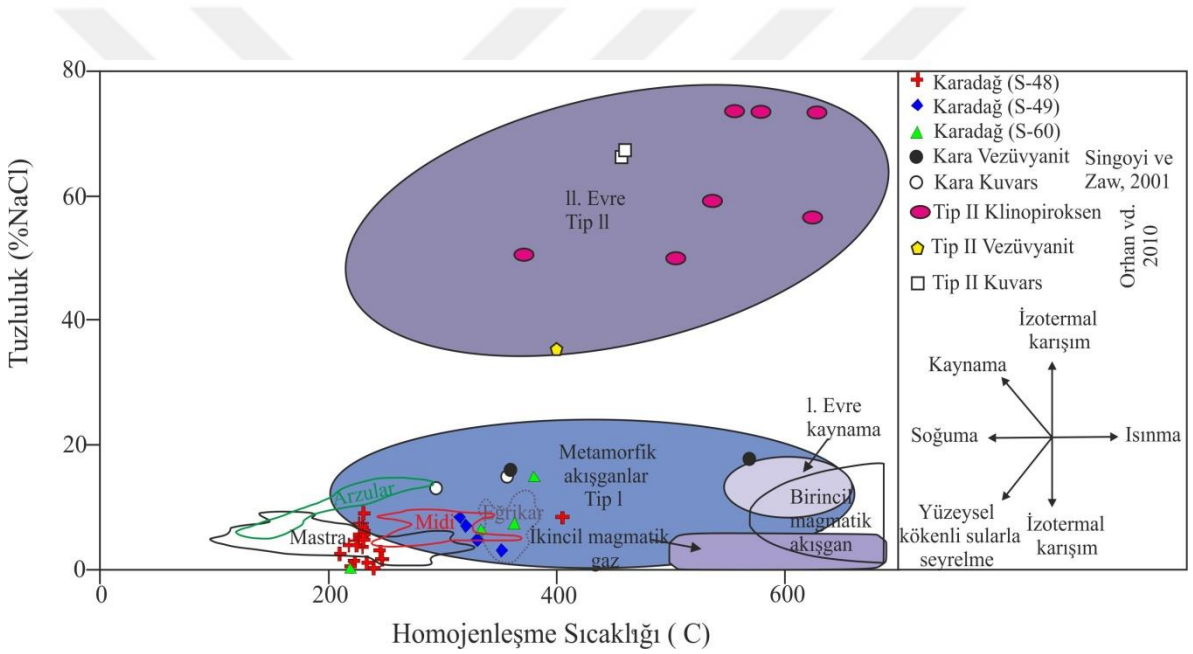
Şekil 4.3. Karadağ Fe-Cu skarn cevherleşmesine ait sıvı kapanımların homojenleşme sıcaklığına ( ^{\circ}\text{C} ) ile tuzluluk (% NaCl) değerlerinin dağılımı (farklı kökenli hidrotermal akışkanların ortalama sıcaklık ve tuzluluk alanları Bodnar, (1999)'dan; Eğrikar verileri Sipahi ve diğ. (2017)'den; sıvıların gelişim yönsemeleri Wilkinson (2001); Midi, Mastra ve Arzular sahalarının verileri Akaryalı (2016)'dan alınmıştır).
