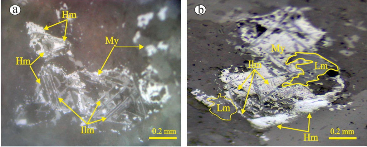
Şekil 3.26. İlmenitin parlak kesitlerde görünüm. a) İskeletimsi dokuda kısmen hematitleşen manyetit üzerindeki ilmenitler (Örn. No: 13) ve b) Kısmen hematitleşen yarı özşekilli bir manyetit tanesi üzerinde ilmenit oluşumları (Örn. No: 13). Hm: Hematit, My: Manyetit, Gng: Gang, Lm: Limonit
