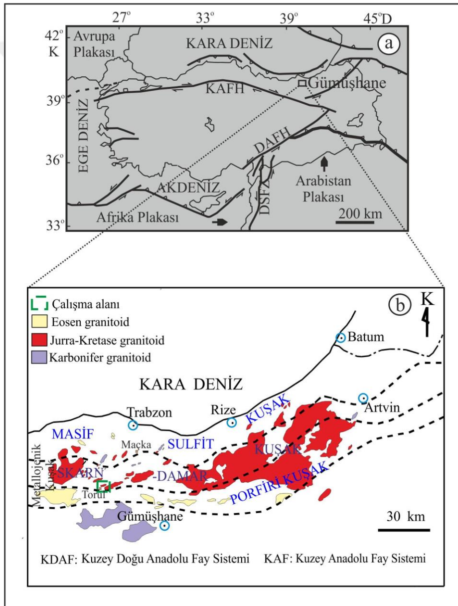
Şekil 1.4. a) MTA 2011'den değiştirilerek b) Karadeniz Bölgesi'ndeki Metalojenik Kuşakları gösteren harita (Pejatoviç, 1971).
