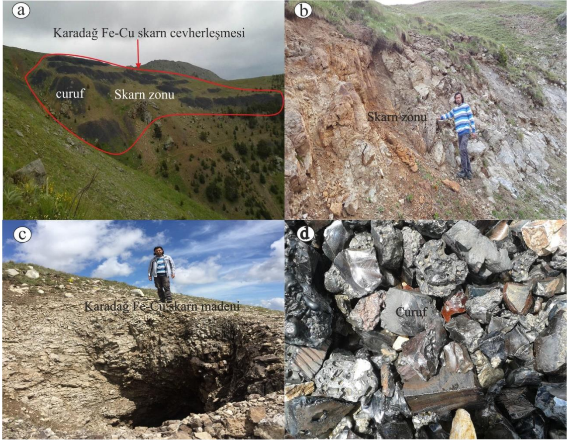
Şekil 3.19. a) Karadağ Fe-Cu skarn cevherleşmesine ait arazi görünümü b) Skarn zonuunun arazideki görünümü c) Karadağ Fe-Cu skarn cevherleşmesindeki eski işletmelere ait maden görünümü c) Karadağ Fe-Cu skarn cevherleşmesinde eski işletmelerden arda kalan curufun yakından görünümü
