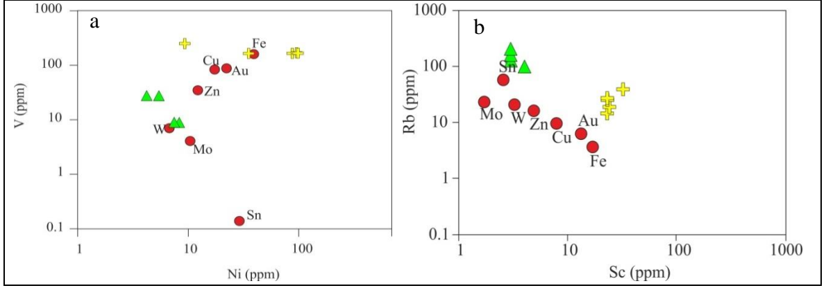
Şekil 4.2. Karadağ Fe-Cu skarn cevherleşmesindeki granitoidlerin ve Fe-, Au-, Cu-, Zn-, W-, Mo- ve Sn-skarnlara eşlik eden granitoidlerin diyagramlardaki konumları a) Ni'e karşı V ve b) Sc'a karşı Rb (Meinert, 1995; Meinert ve diğ., 2005'ten değiştirilerek). Semboller için Şekil 3.15a'ya bakınız.
