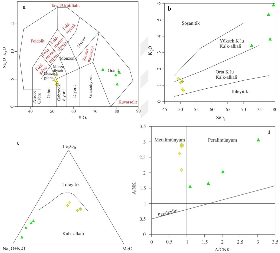
Şekil 3.15. Karadağ Fe-Cu skarn cevherleşmesine ait granitoidik kayaç örneklerinin sınıflama diyagramındaki yerleri a) SiO_2 'e karşı Na_2O+K_2O diyagramındaki (Middlemost, 1994) ve b) SiO_2 'e karşı K_2O (Le Maitre, 1989) ve c) AFM (Irvine ve Baragar, 1971) ve d) Shand (1947) değiştirilerek kullanılmıştır
