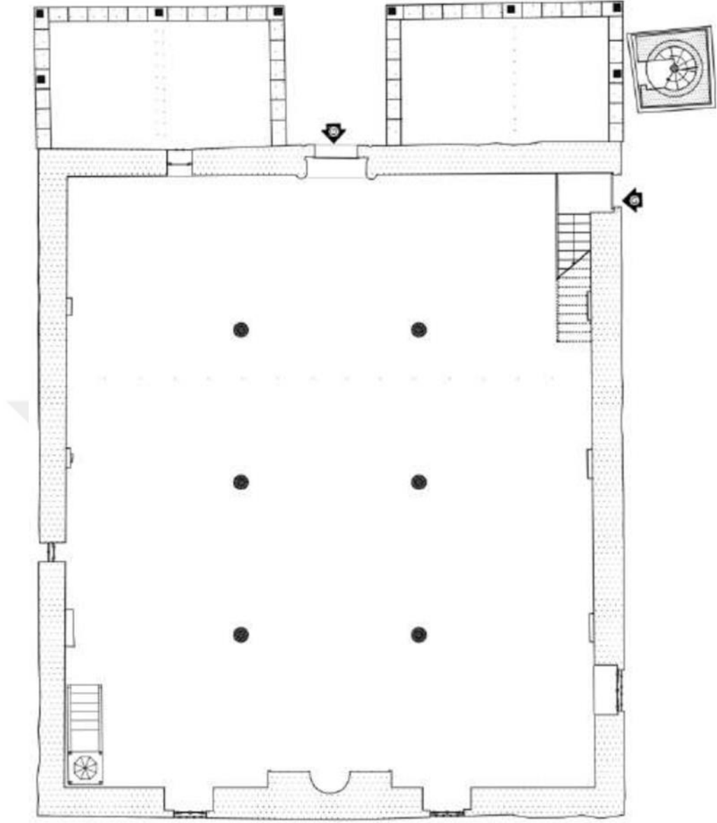
Şekil 65. Böğet Hanı Cami Planı (V.G.M.A.)
