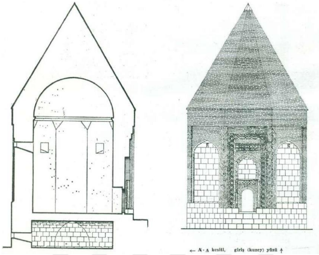
Şekil 90. Selime Sultan Türbesi Kesit ve Cephe (Orhan Cezmi Tuncer)
