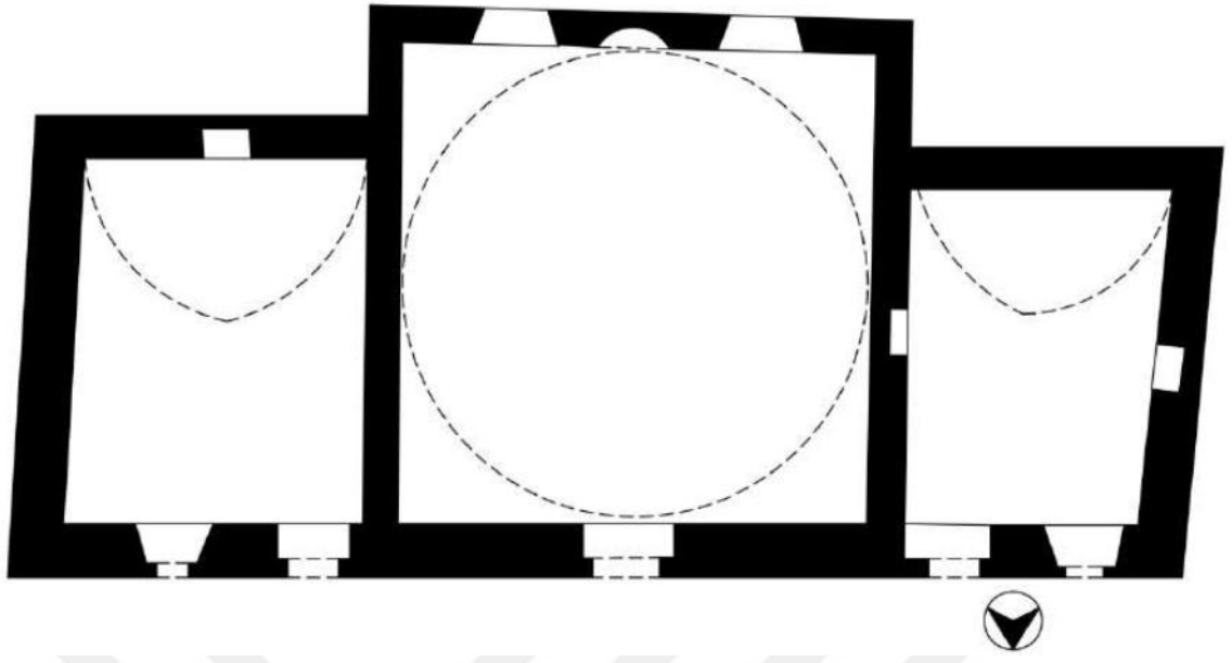
Şekil 131. Cemaleddin Aksarayi Zaviyesi Planı (Bekir Deniz)
