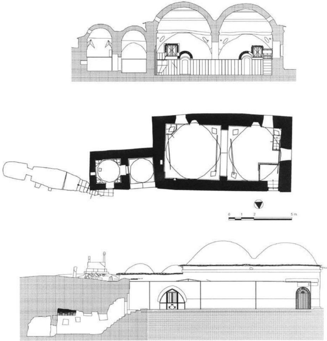
Şekil 140. Somuncu Baba Zaviyesi Planı, Kesiti ve Cephe Görünüşü (V.G.M.A.)
