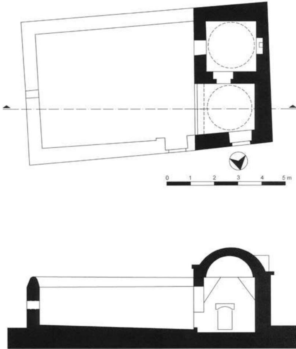
Şekil 135. Şeyh Hamza Zaviyesi (Osman Nuri Dülgerler)
