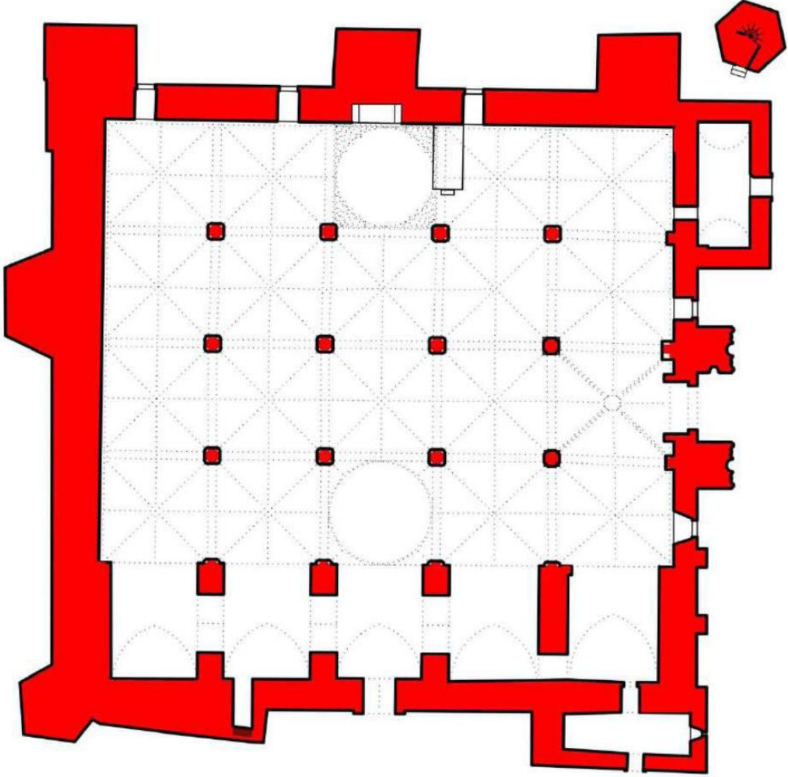
Şekil 1. Ulu Camii Planı (V.G.M.A.)
