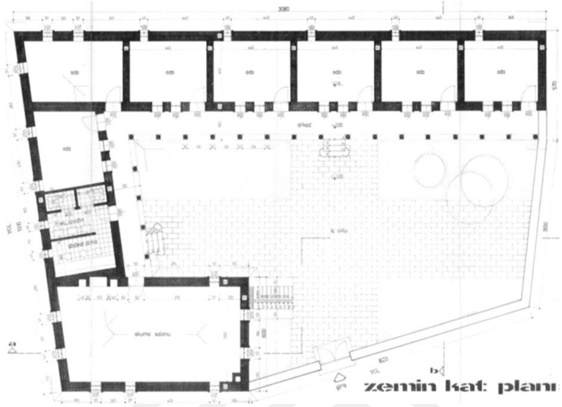
Şekil 28. Bedriyye Medresesi Planı (V.G.M.A.)
