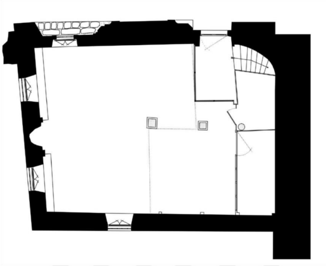
Şekil 18. Hacı Yusuf (Cıncıklı Mescit) Mescidi Planı (V.G.M.A.)
