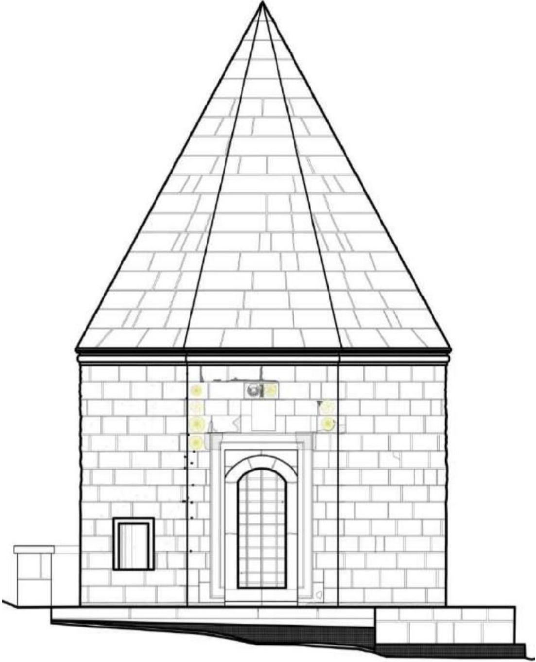
Şekil 115. Kılıç Arslan Türbesi (V.G.M.A.)
