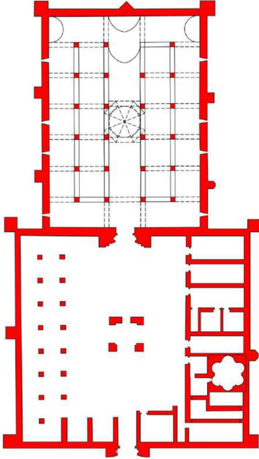
Şekil 36. Pervane (Alay Han) Kervansarayı Planı (V.G.M.A.)
