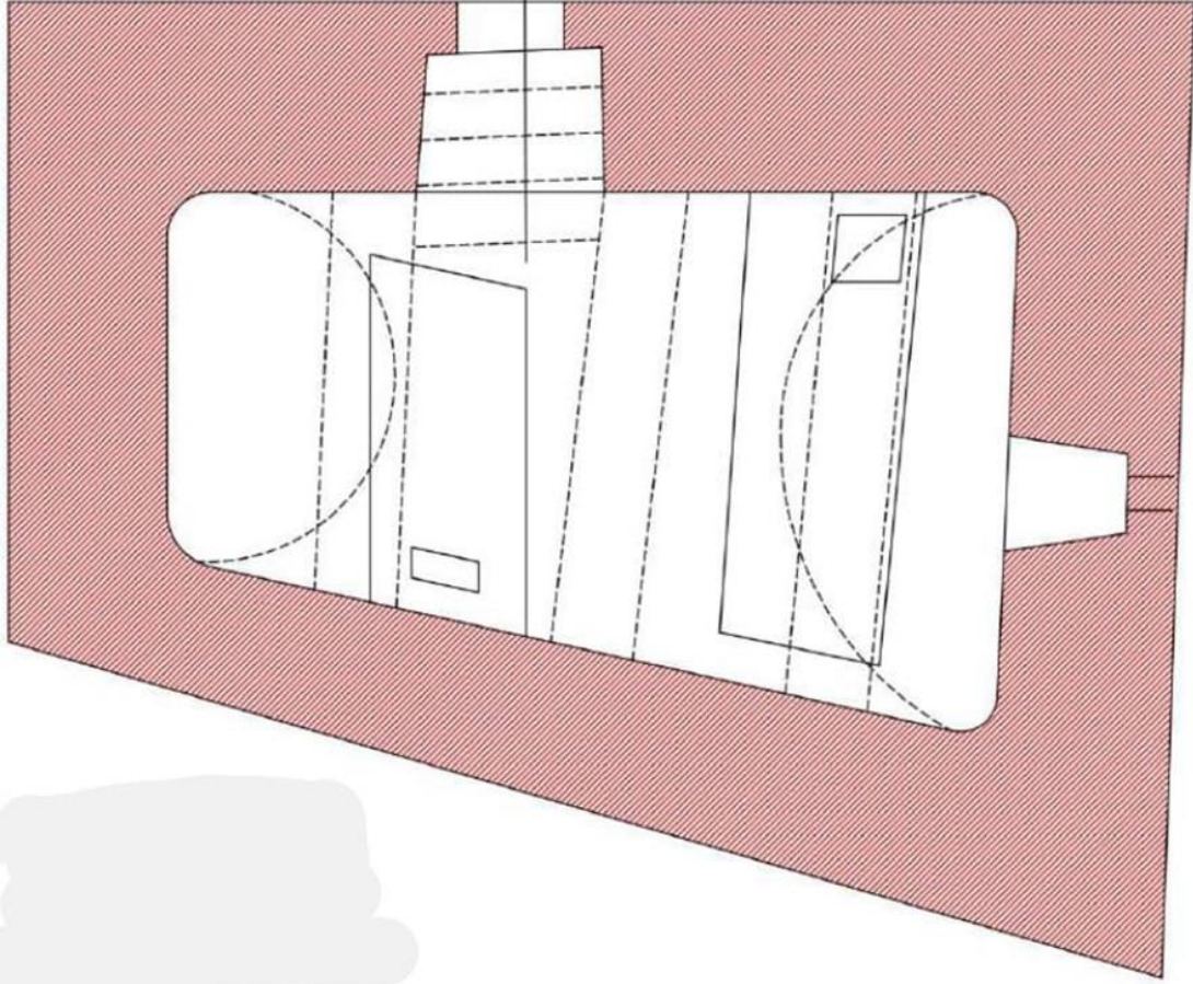
Şekil 110. Yassıviran Mevkii Türbesi Planı (Zekai Erdal)
