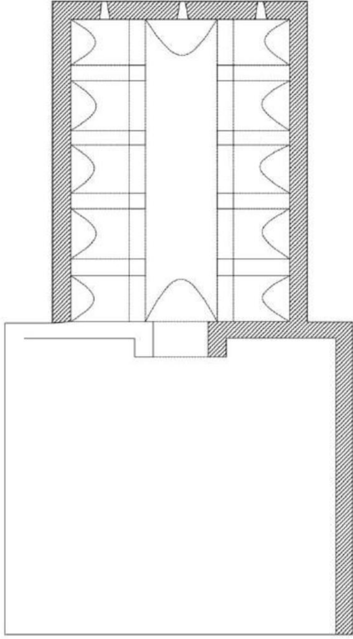
Şekil 55. Sıraçakıl Hanı Planı (Kurt Erdmann)
