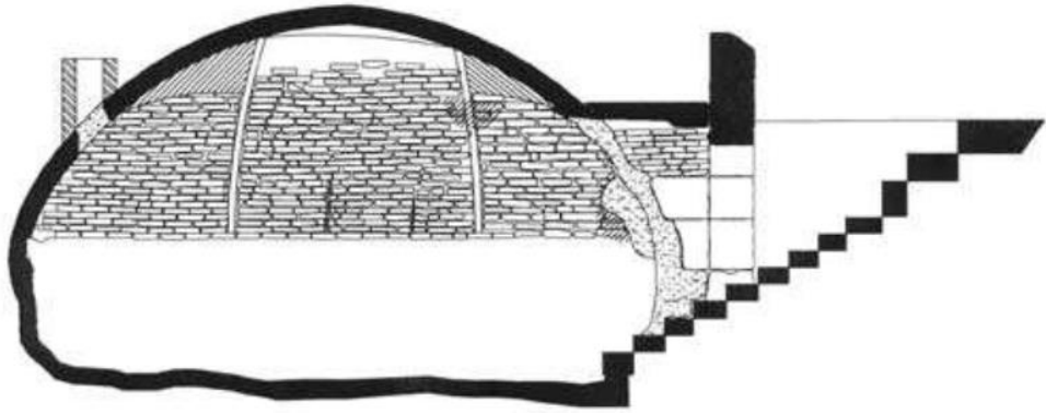
Şekil 95. Çaput Baba Türbesi Planı ve Kesiti (V.G.M.A.)
