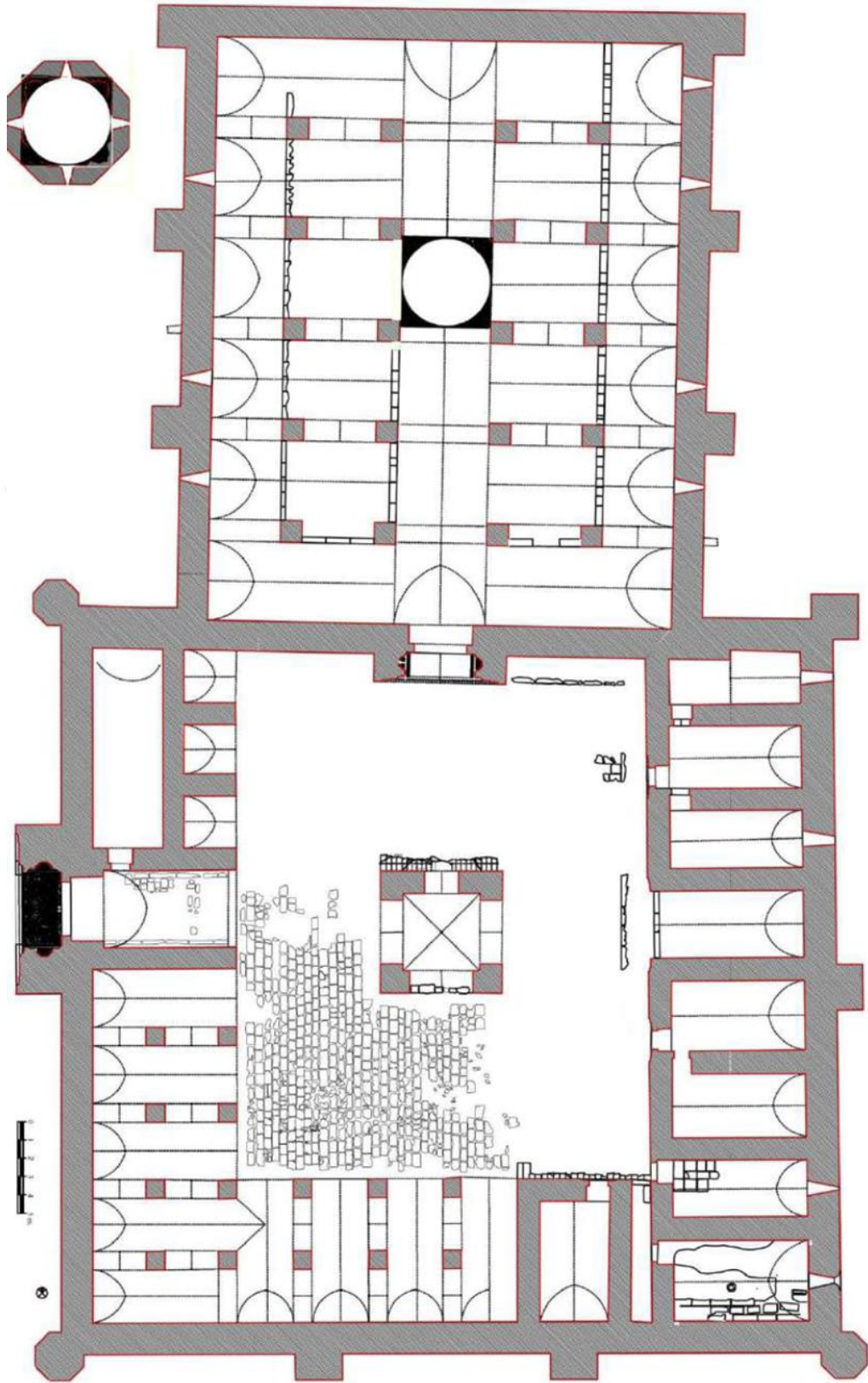
Şekil 46. Ağzıkara Han Planı (V.G.M.A.)
