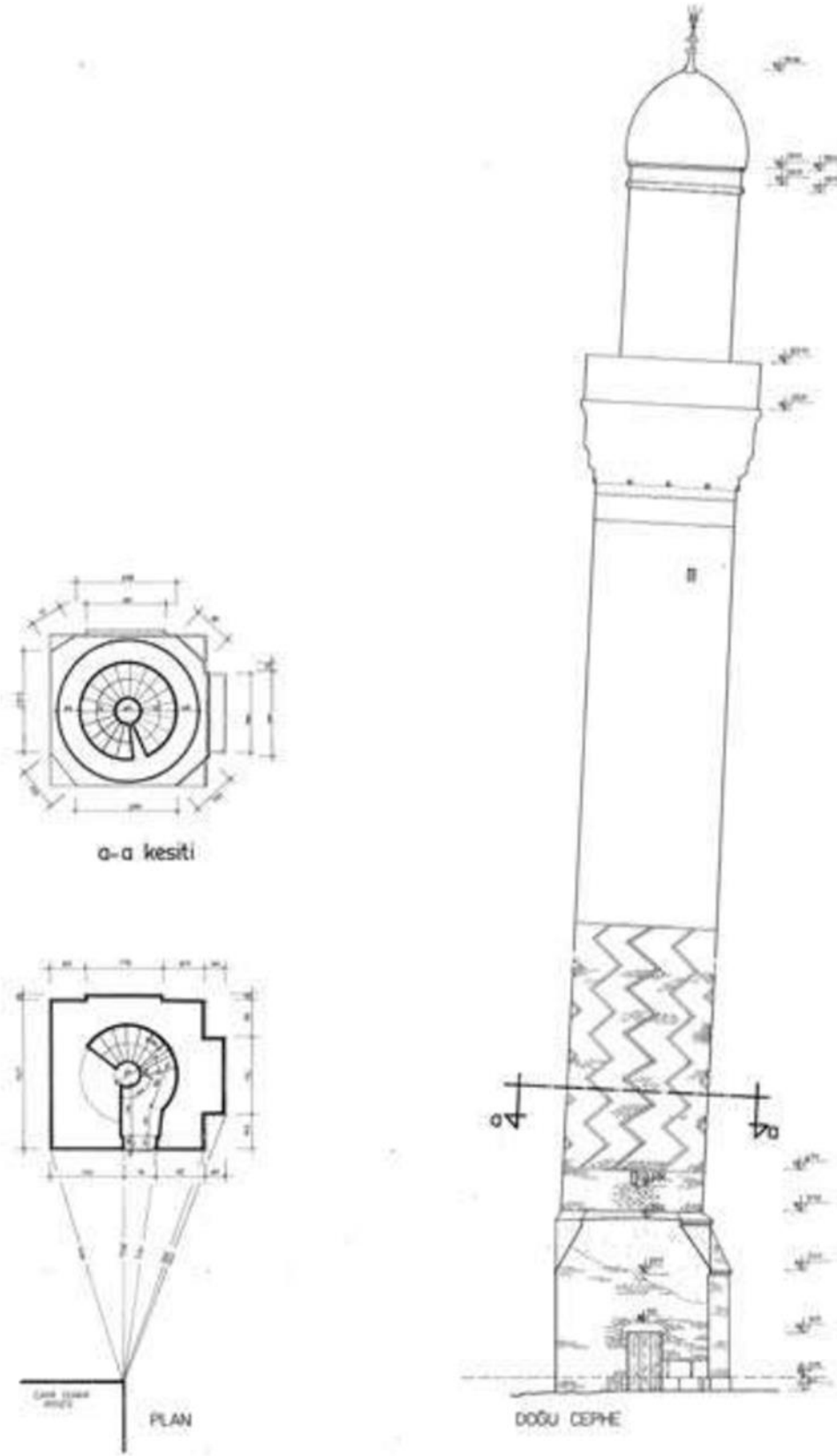
Şekil 13. Eğri (Kızıl) Minare Planı ve Çizimi (V.G.M.A.)
