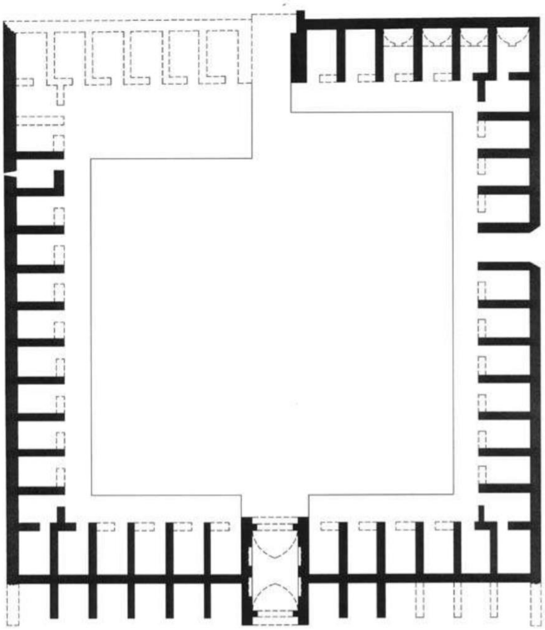
Şekil 39. Kılıç Arslan Hanı (E. Nihal Çetintürk)
