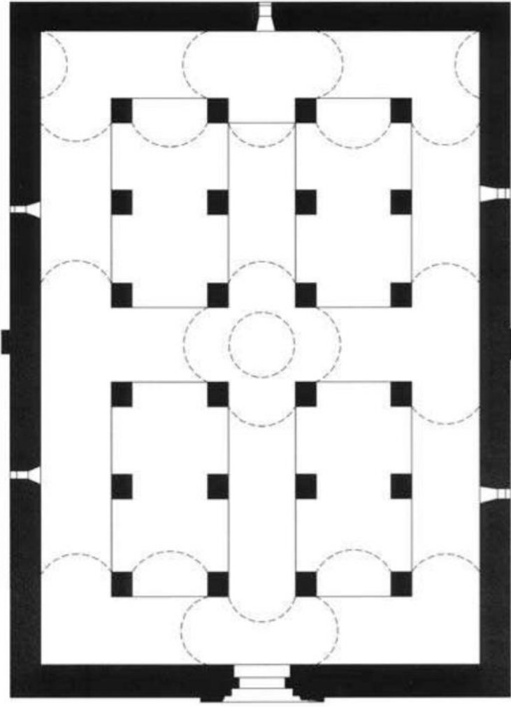
Şekil 43. Öresin (Tepesi Delik Han) Han Planı (V.G.M.A.)
