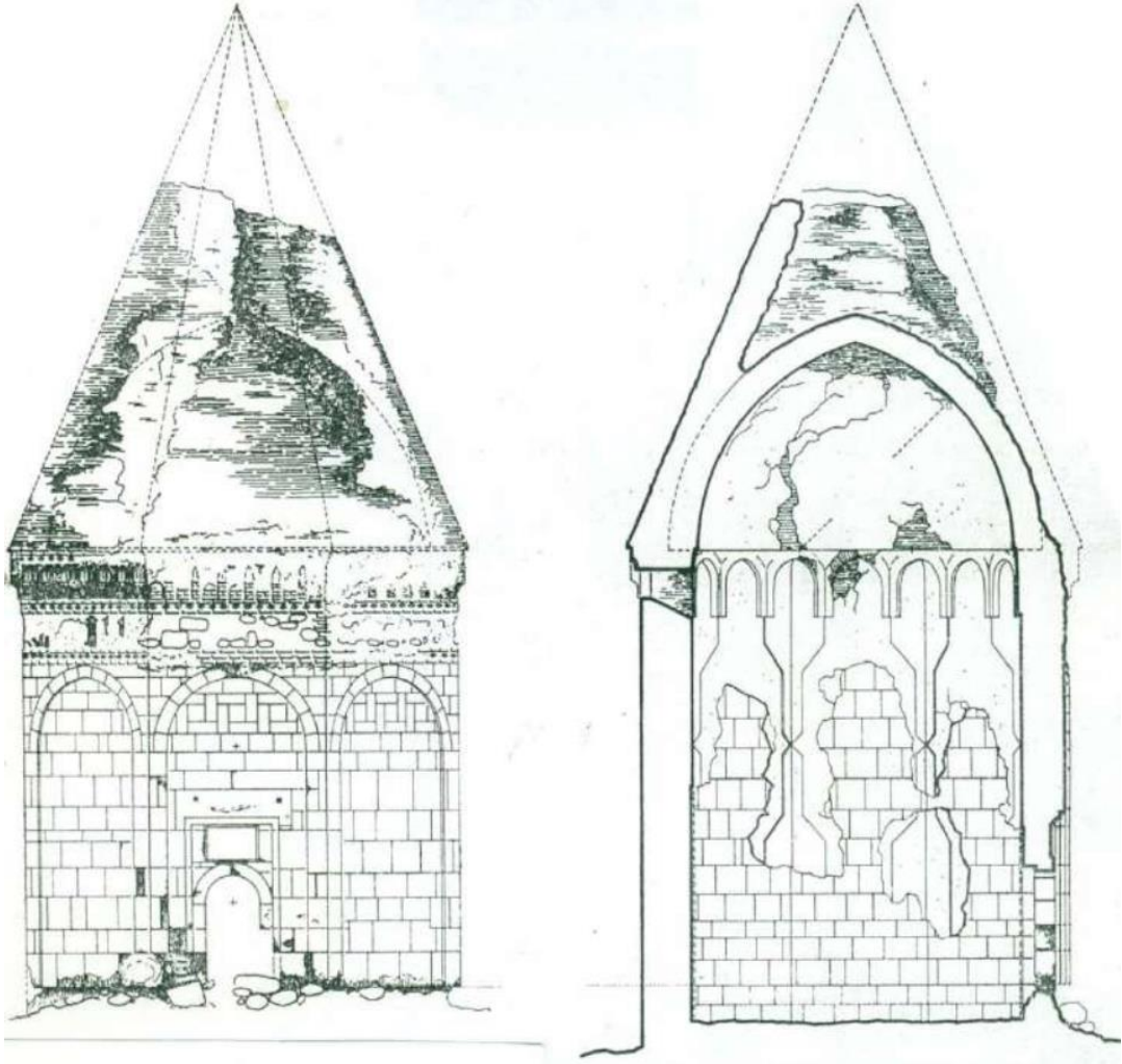
Şekil 81. Bekar Sultan Kümbeti Kesit ve Cephe Görünüşü (Orhan Cezmi Tuncer)
