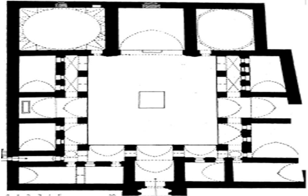
Şekil 21. Zinciriye Medresesi Planı (Ahmet Kuran)
