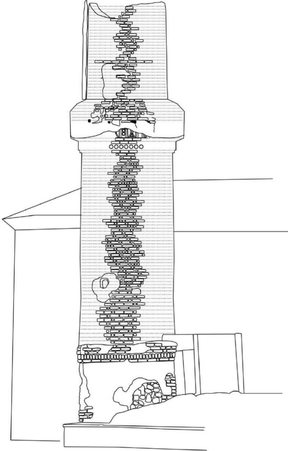
Şekil 10. Yıkık Minare Çizimi (V.G.M.A.)
