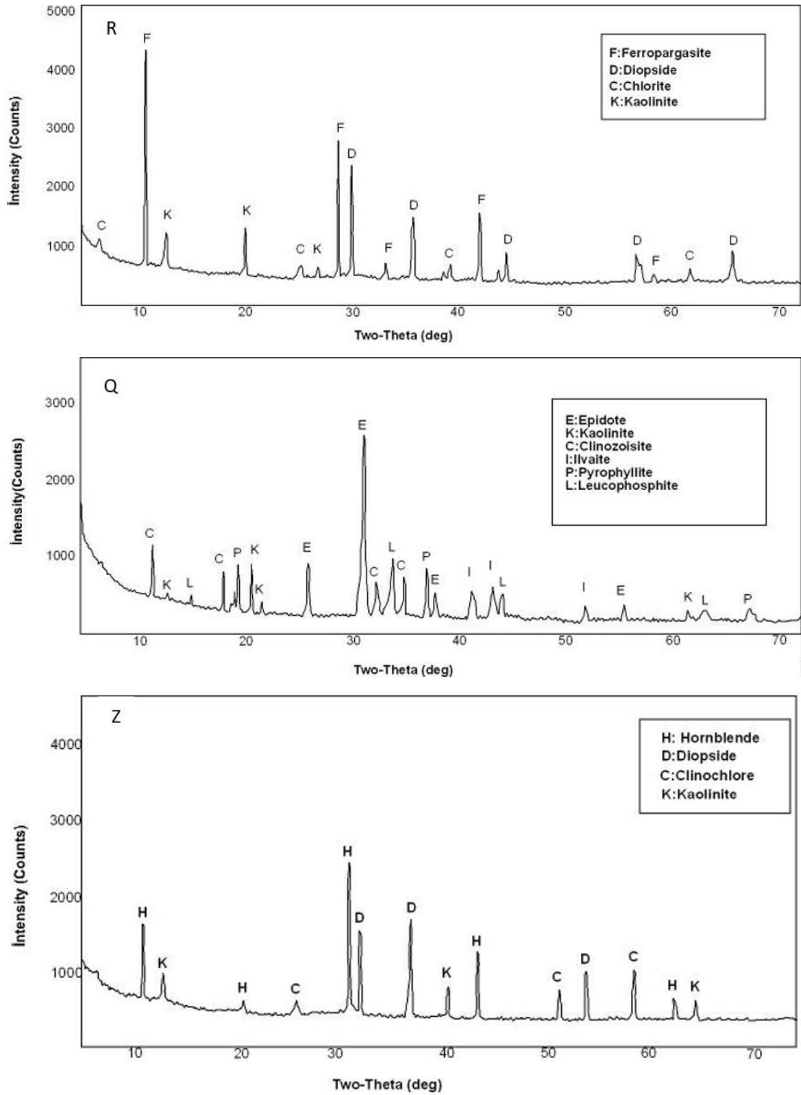
Şekil 21. Gabro Pegmatit içerisinde seçilmiş minerallerin XRD çözümlmeleri
