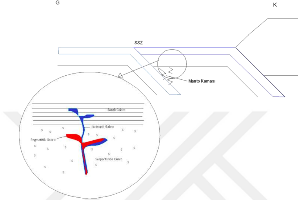
Şekil 33. Karaorgan Pegmatitik Gabrolarının gelişiminde düşünülen jeotektonik model
