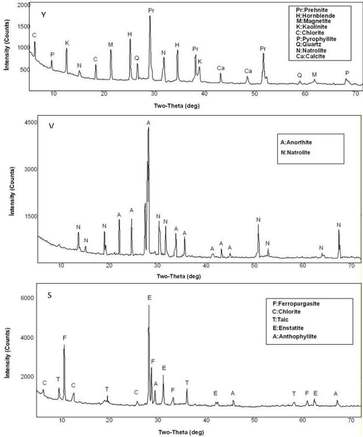
Şekil 20. Gabro Pegmatit içerisinde seçilmiş minerallerin XRD çözümlmeleri
