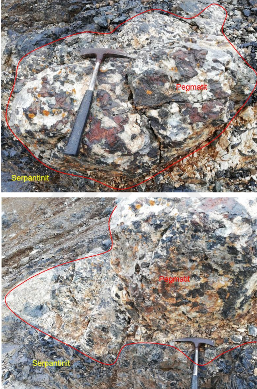
Şekil 16. Serpantinıt ierisine yerleşen Pegmatit stokları (üstte ve altta)
