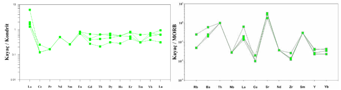
Şekil 31. Pegmatitik gabroların C1 kondrite normalleşmiş NTE (solda) ve MORB a normalleşmiş İz Element dağılımları (sağda)
