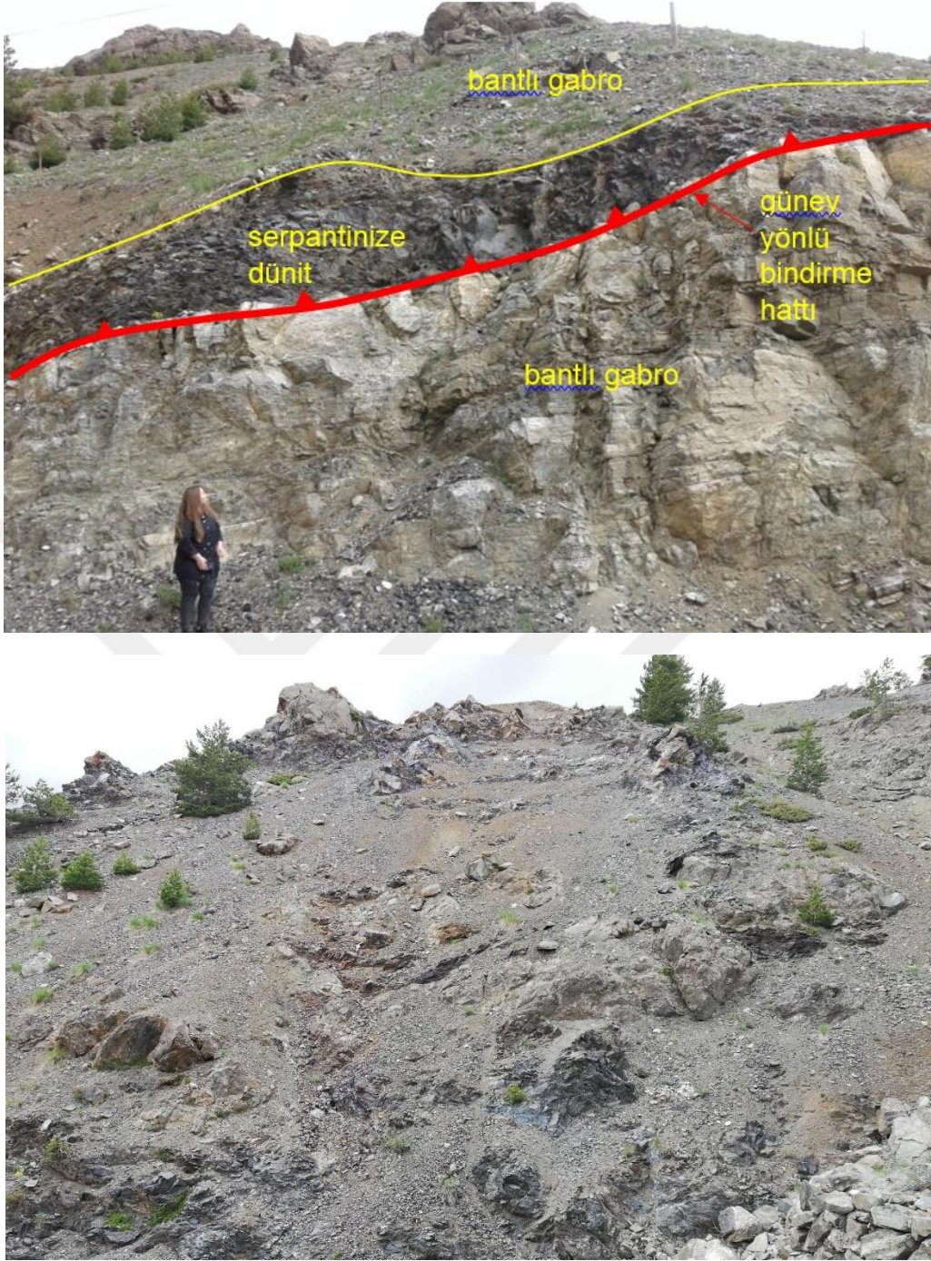
Şekil 11. Bantlı gabroların arazideki görünüşleri. Bantlı gabrolar ve bunları tektonik olarak üzerleyen serpantinize dünitler (üstte), tektonizma ile doğrultuları bozulmuş bantlı gabrolar (altta). Her iki fotoğraf güneyden kuzey yönüne doğru çekilmiştir.
