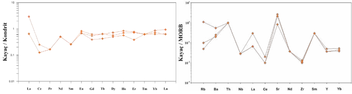
Şekil 29. Bantlı gabroların C1 kondrite normalleşmiş NTE (solda) ve MORB a normalleşmiş İz Element dağılımları (sağda)
