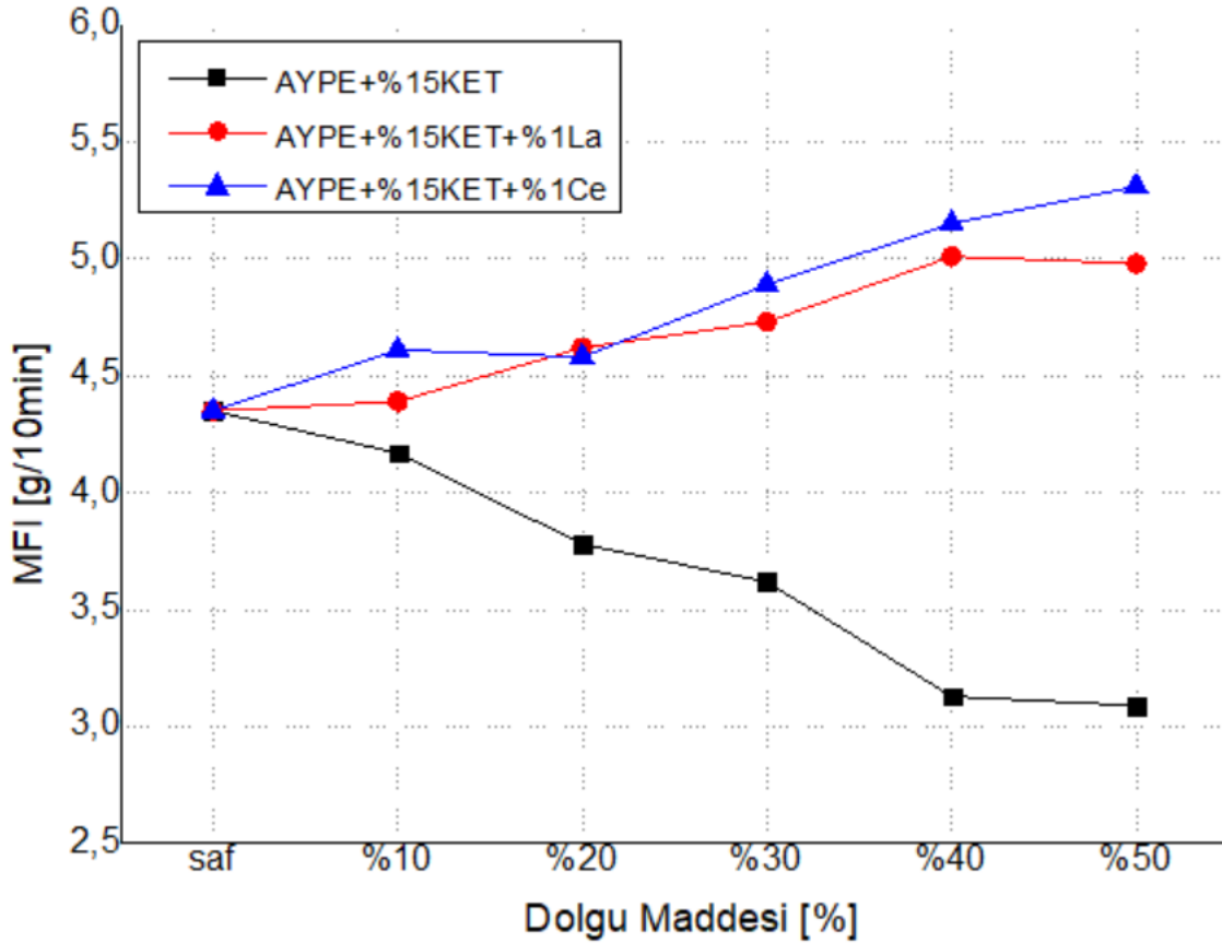
Şekil 6.4. Dolgu maddesinin çeşidi ve miktarına bağlı olarak YYPE'nin kütesel akışkanlığındaki değişim
