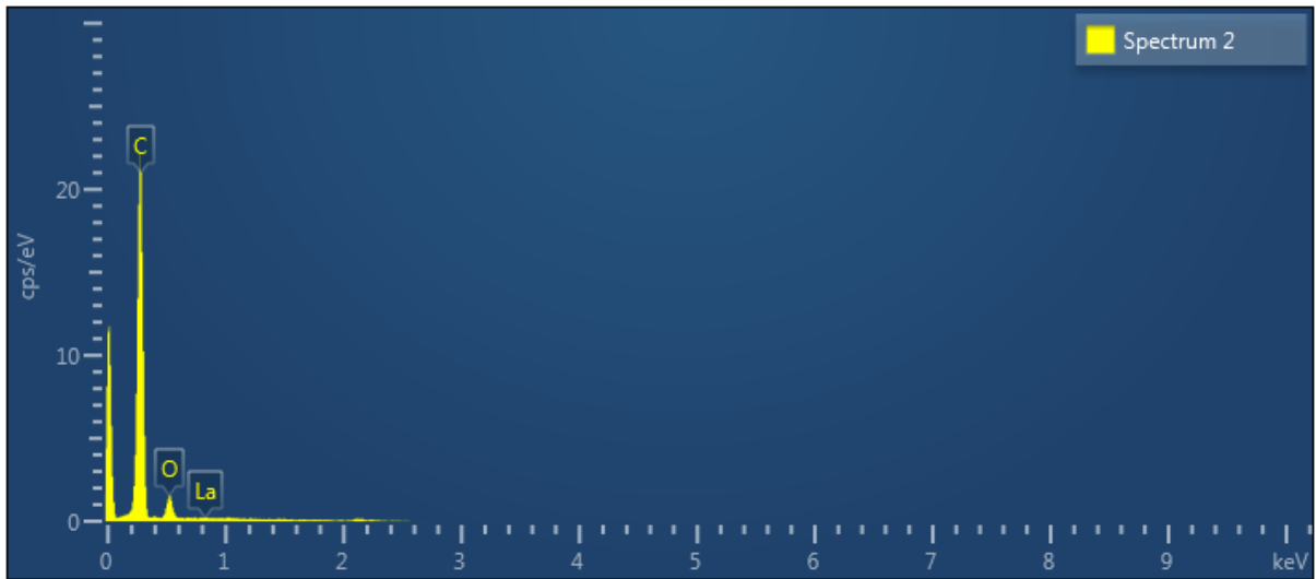
Resim 6.15. EDS analizine ait spektrum sonucu
