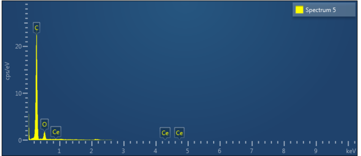
Resim 6.18. EDS analizine ait spektrum sonucu
