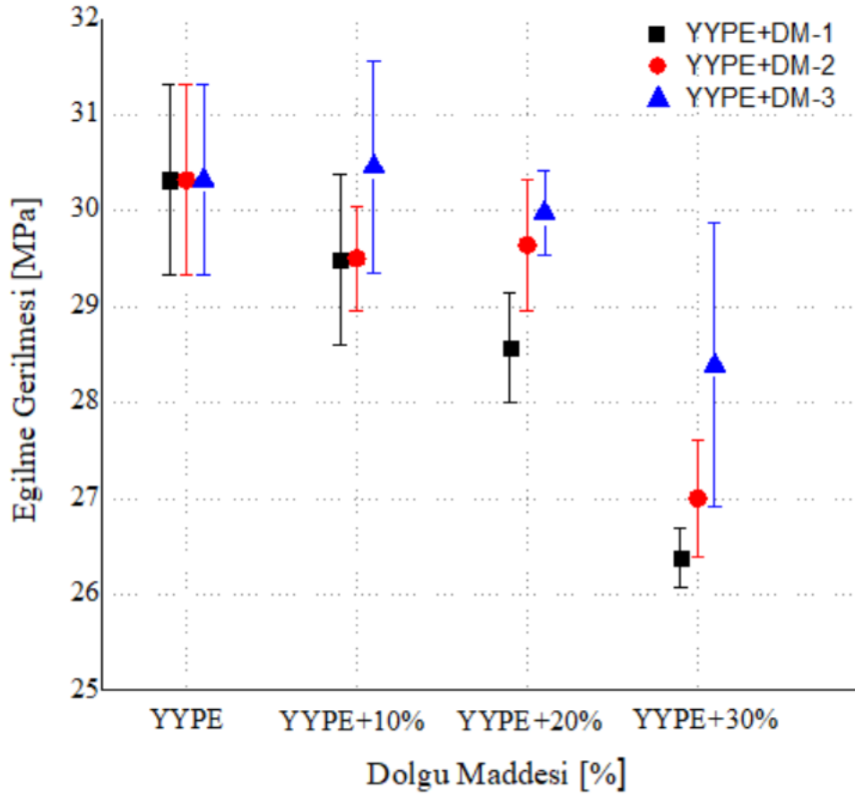
Şekil 6.10. Dolgu maddesi çeşidi ve ağırlıkça oranına bağlı olarak YYPE'nin eğilme gerilmesindeki değişim
