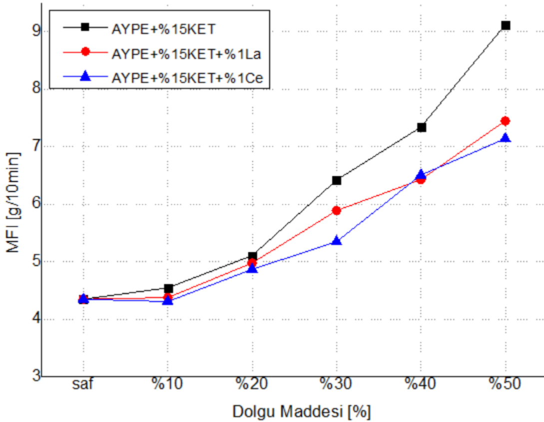
Şekil 6.2. Farklı dolgu maddeleri ve oranlarına bağı olarak YYPE’nin eriyik akış indeksindeki değ işim
